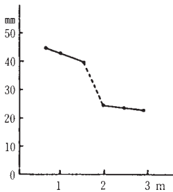
図6-1 深度～地中変位
