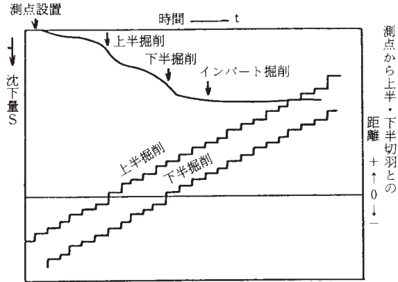
図 6 - 11 地表沈下量経時変化
