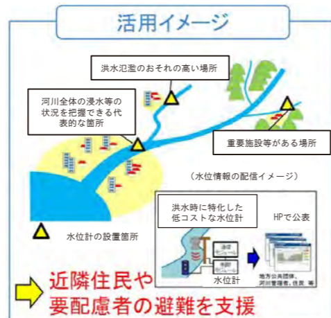
危機管理型水位計*13 <出典：国土交通省資料>
