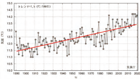
福島 年平均気温 1890-2020
