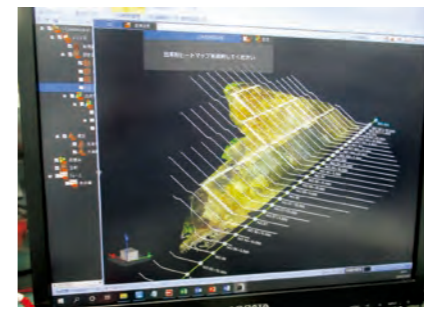
3次元設計データの活用
