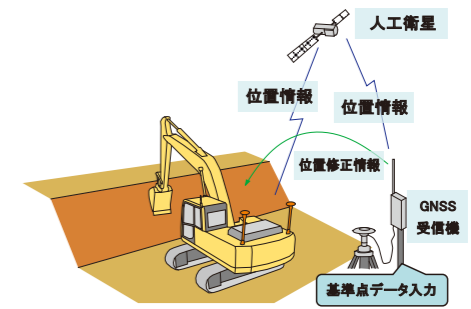
ICT建設機械による施工イメージ
