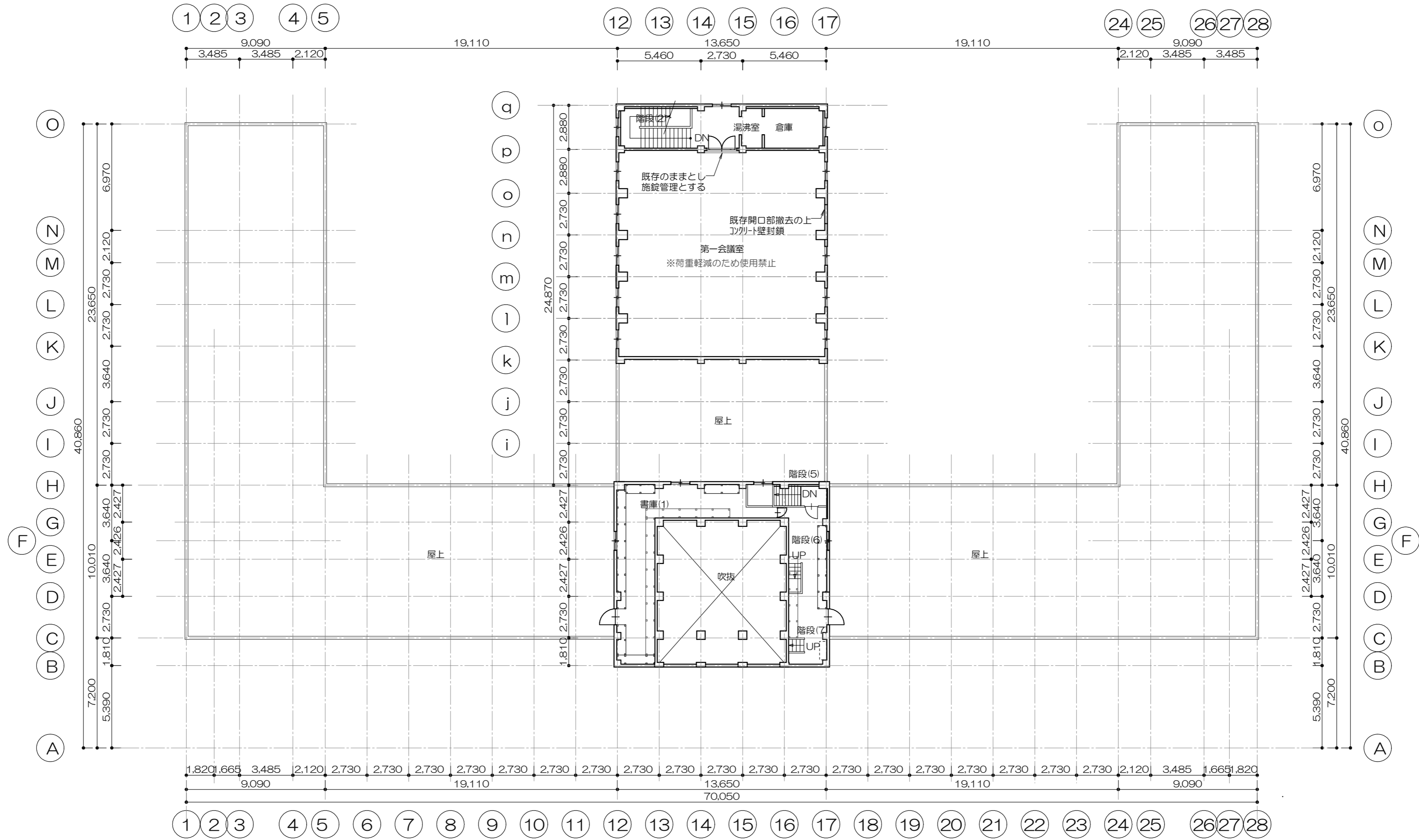
改修後 3階平面図 S=1/200
