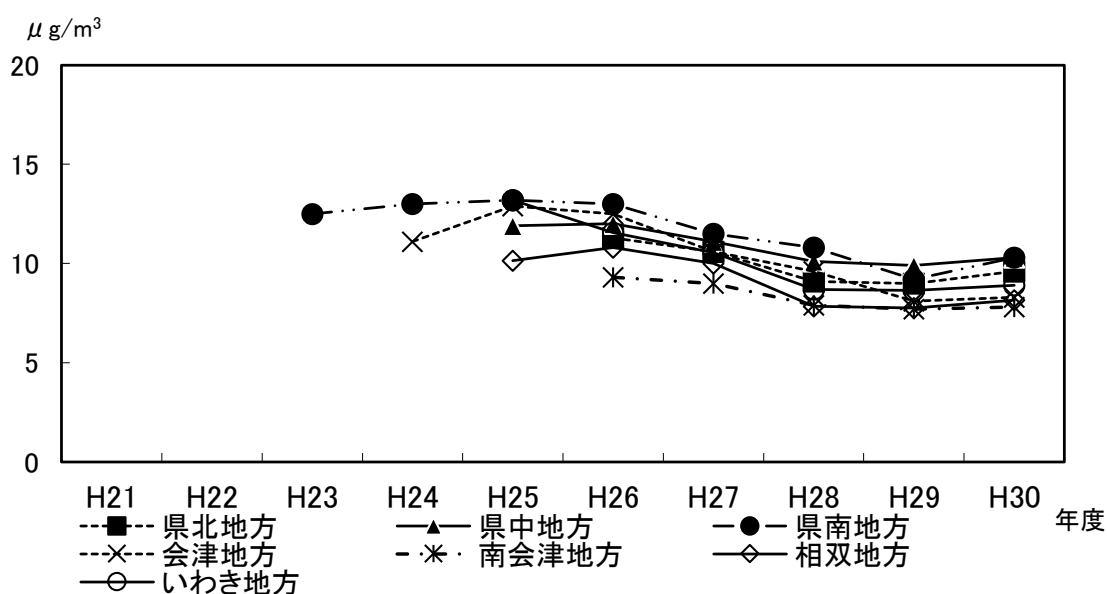
図-11 微小粒子状物質(年平均値)の経年変化
