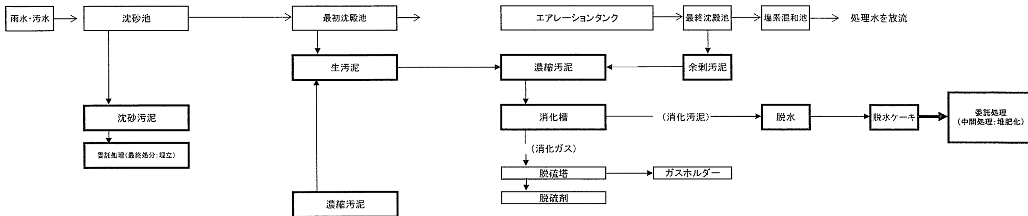
【高松浄化センター】処理フロー
