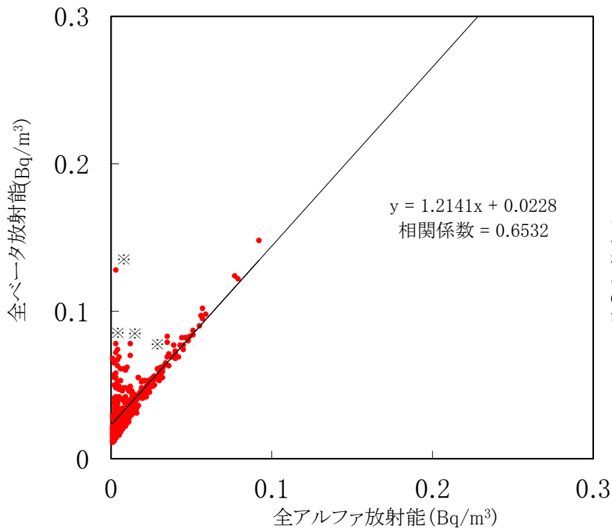
大気浮遊じんの全アルファ・全ベータ放射能の相関図 (MP-3) (令和8年1月～令和8年3月)
