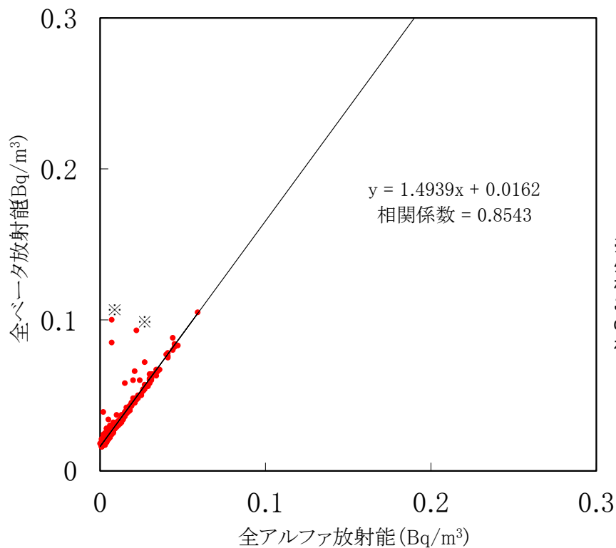
大気浮遊じんの全アルファ・全ベータ放射能の相関図 (MP-8) (令和8年1月～令和8年3月)
