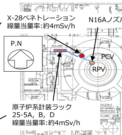
2号機R/B2階
