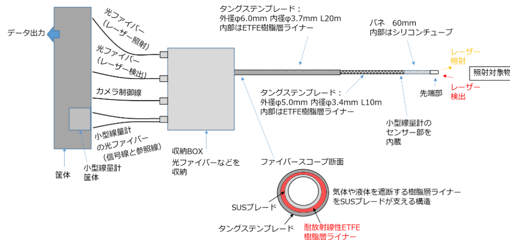
調査装置の全体図（概略）
