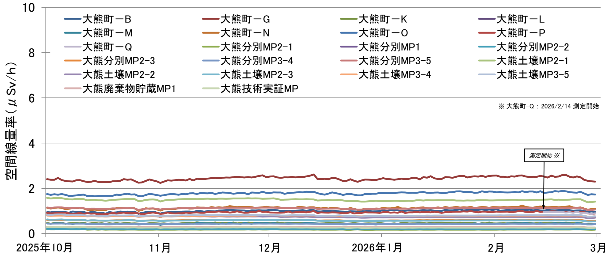
空間線量率の推移(連続測定)(2025年10月1日～2026年2月28日)
