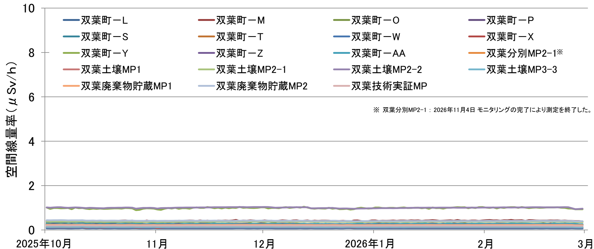
空間線量率の推移(連続測定)(2025年10月1日～2026年2月28日)
