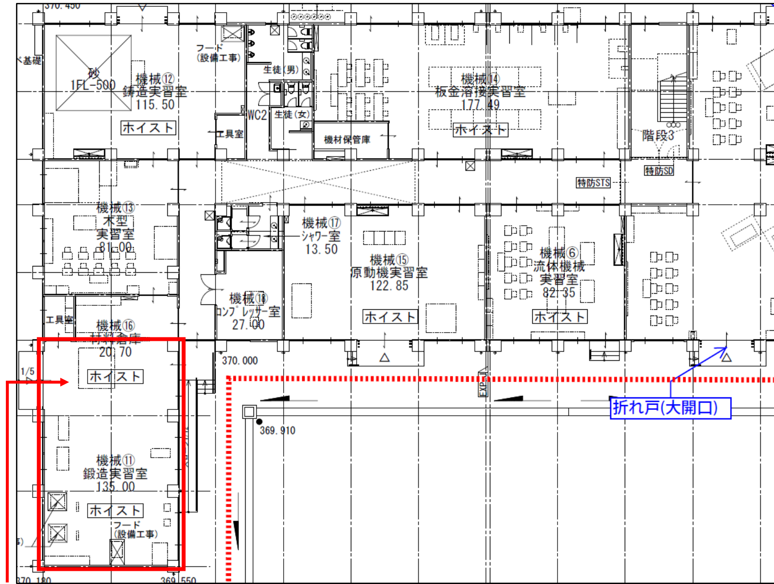
福島県立白河実業高等学校 新実習棟平面図
