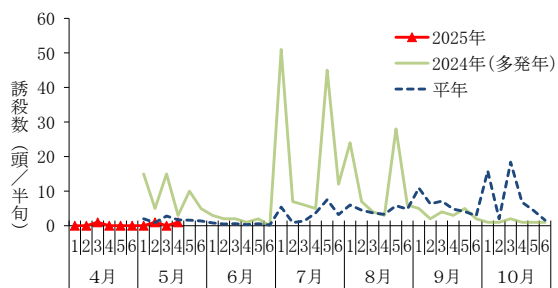
図6 フェロモントラップによるオオタバコガ誘殺状況 (新地町:キク) ※4月から調査開始
