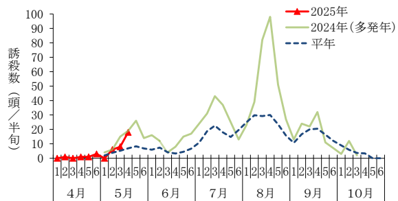
図1 フェロモントラップによるオオタバコガ誘殺状況 (伊達市保原町:キク) ※4月から調査開始
