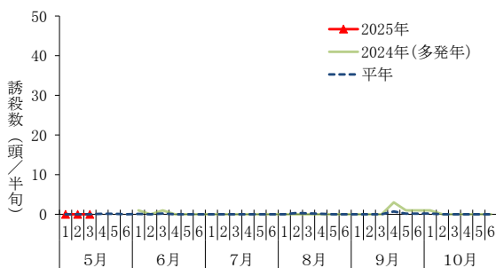
図5 フェロモントラップによるオオタバコガ誘殺状況 (南会津町界:トマト)
