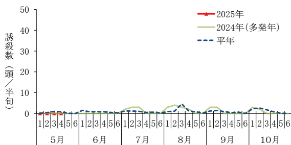
図2 フェロモントラップによるオオタバコガ誘殺状況 (中島村:トマト) 平均2015年は矢吹町上宮崎、2016～18年は泉崎村
