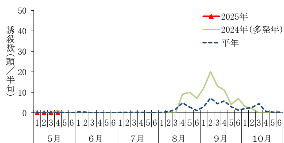
図3 フェロモントラップによるオオタバコガ誘殺状況 (喜多方市加納:トマト) ※2024年は会津美里町徳馬
