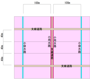
標準区画割図
