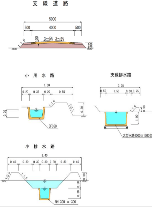
標準区構造図
