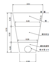
吸水渠
