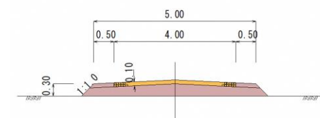
標準断面図（パイプライン）
