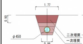
標準断面図（パイプライン）
