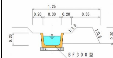
標準断面図（小用水路）
