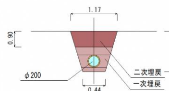
標準断面図（パイプライン）
