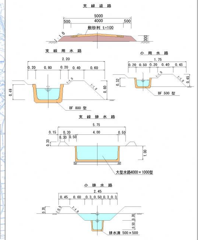
標準構造図
