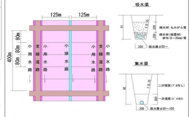
標準構造図
