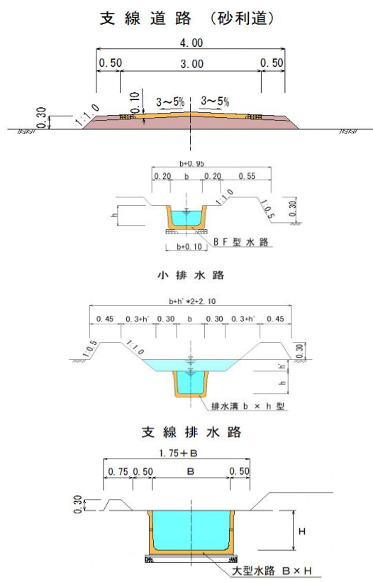
標準構造図
