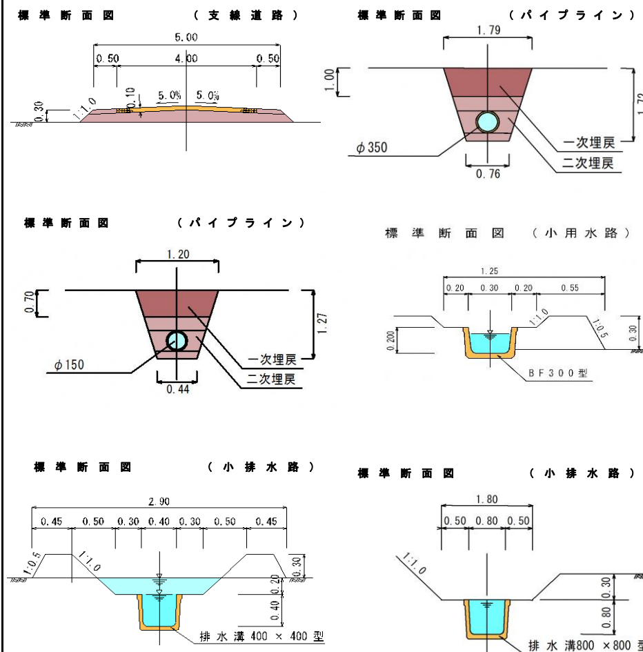
標準構造図
