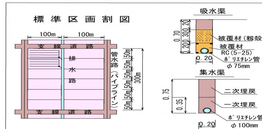
標準区画割図
