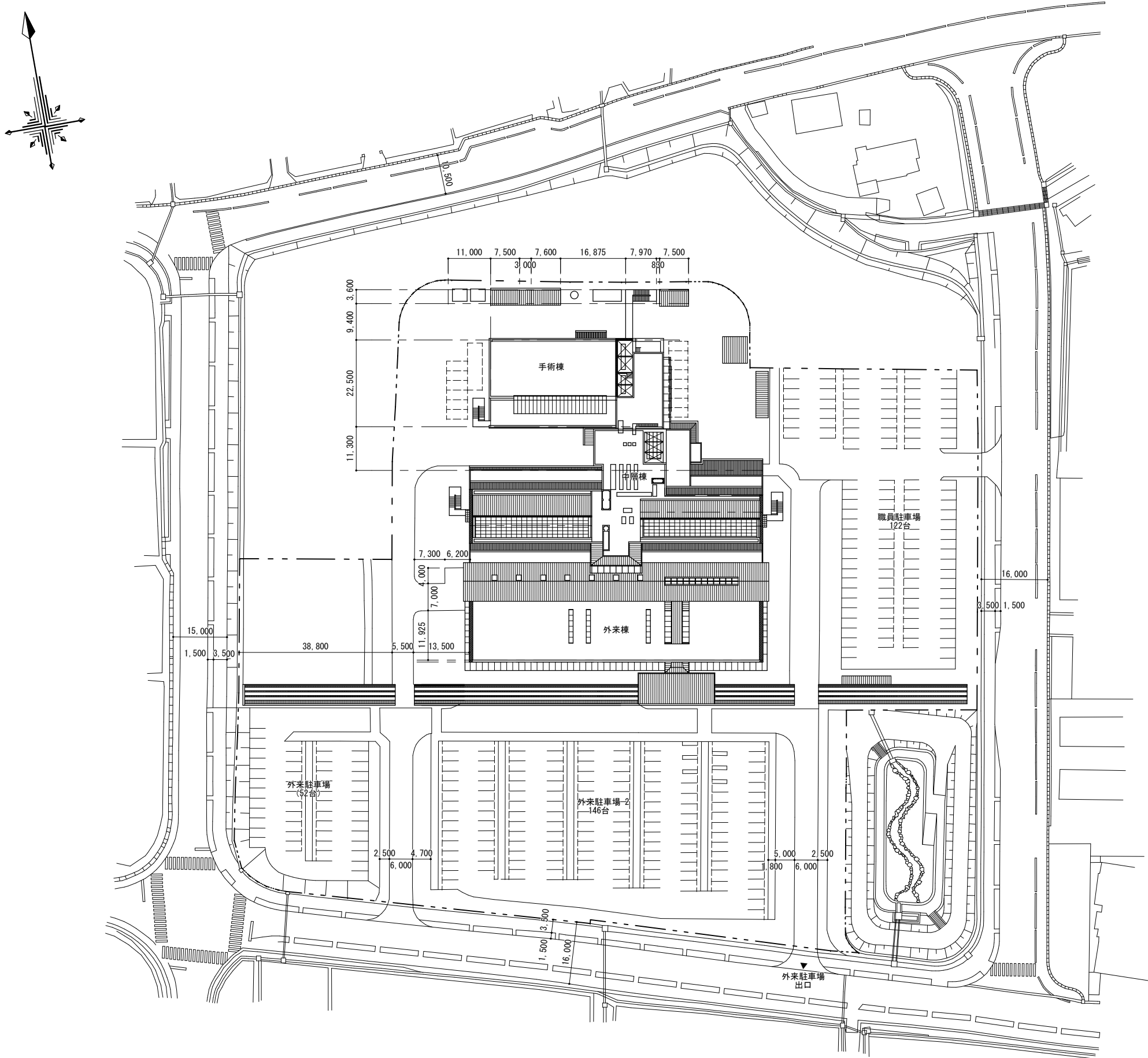
配置図 S=1:800
