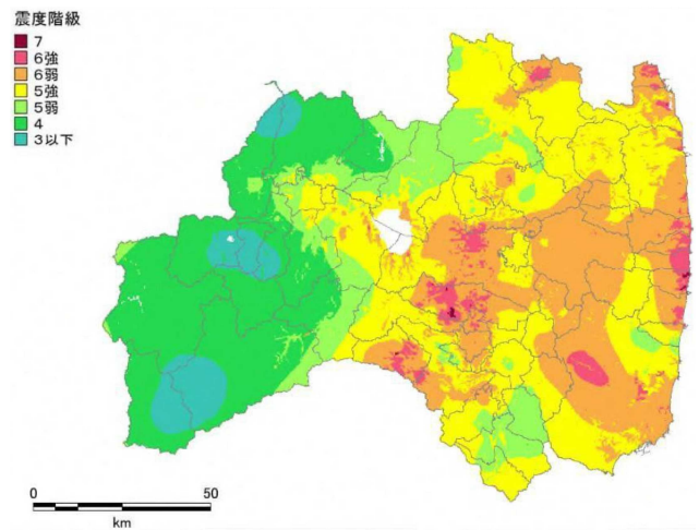
図 震度分布
