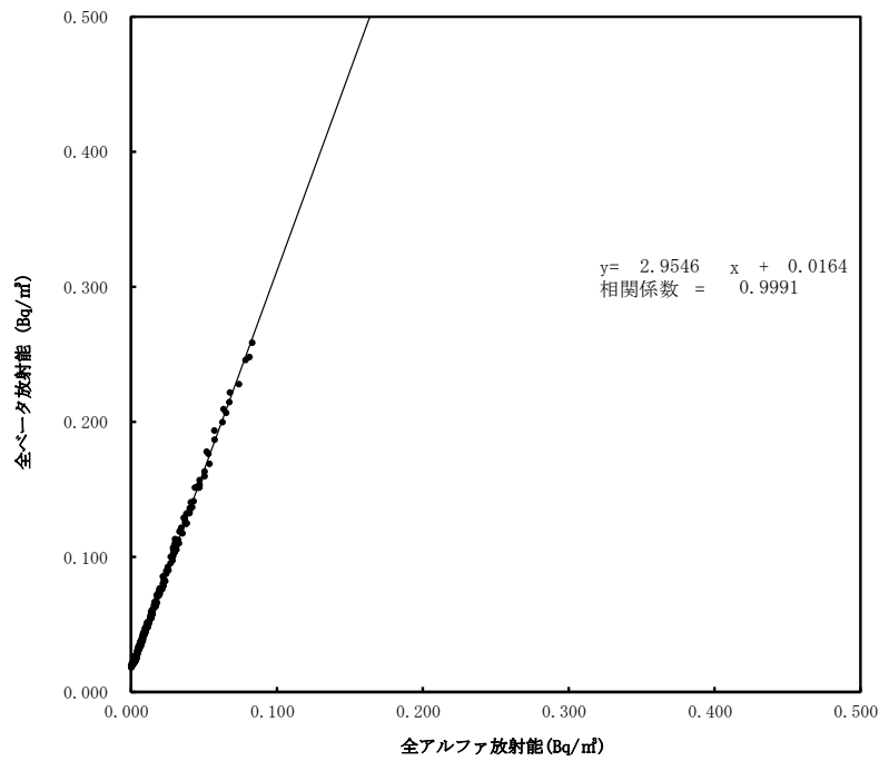
大気浮遊じんの全アルファ・全ベータ放射能の相関図 (6時間連続集じん・6時間放置後) (令和6年7月～9月) (檜葉町繁岡)
