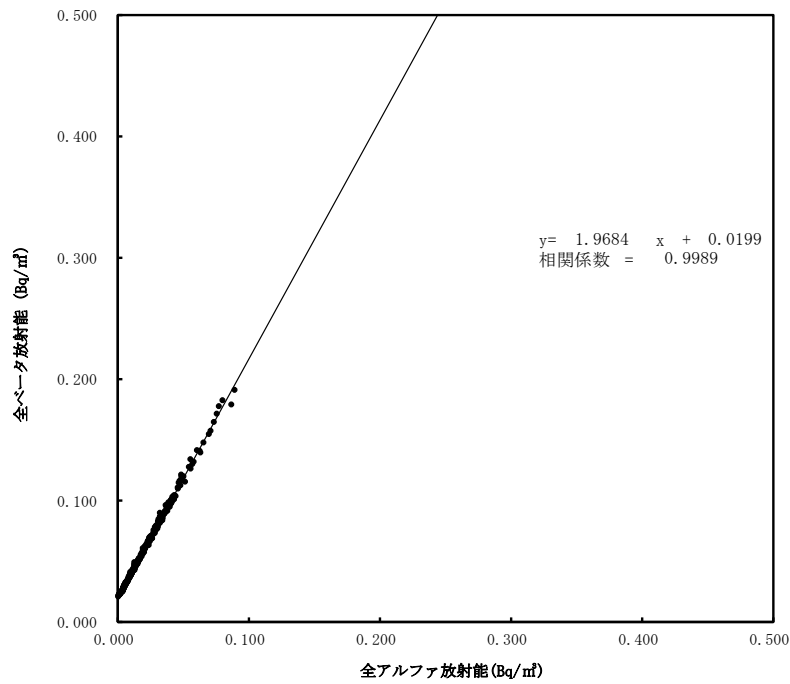
大気浮遊じんの全アルファ・全ベータ放射能の相関図 (6時間連続集じん・6時間放置後) (令和6年7月～9月) (広野町小滝平)
