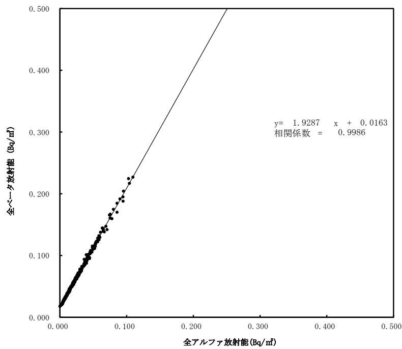
大気浮遊じんの全アルファ・全ベータ放射能の相関図 (6時間連続集じん・6時間放置後) (令和6年7月～9月) (檜葉町木戸ダム)
