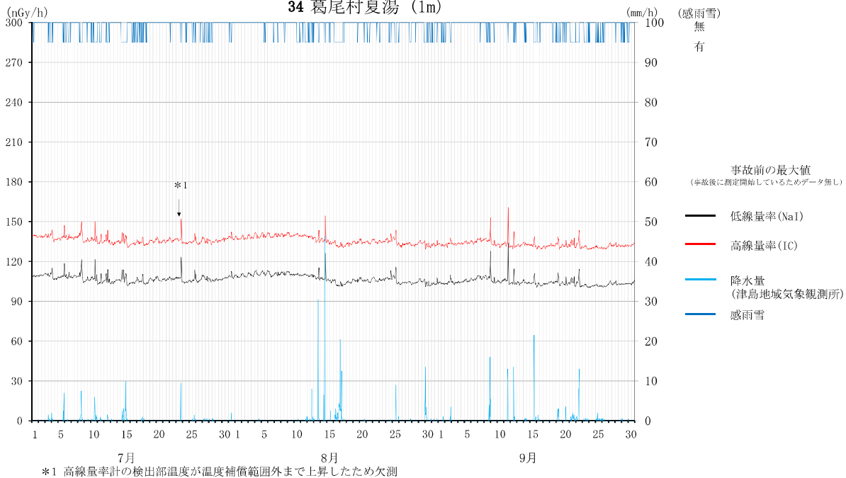
空間線量率の変動グラフ 34 葛尾村夏湯 (1m)
