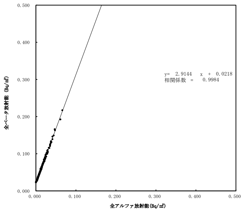
大気浮遊じんの全アルファ・全ベータ放射能の相関図 (6時間連続集じん・6時間放置後) (令和6年7月～9月) (飯館村伊丹沢)
