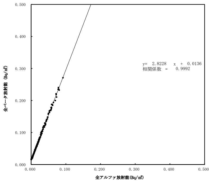
大気浮遊じんの全アルファ・全ベータ放射能の相関図 (6時間連続集じん・6時間放置後) (令和6年7月～9月) (富岡町富岡)
