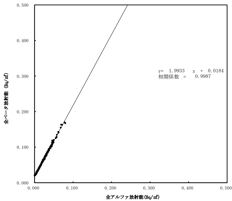
大気浮遊じんの全アルファ・全ベータ放射能の相関図 (6時間連続集じん・6時間放置後) (令和6年7月～9月) (南相馬市泉沢)
