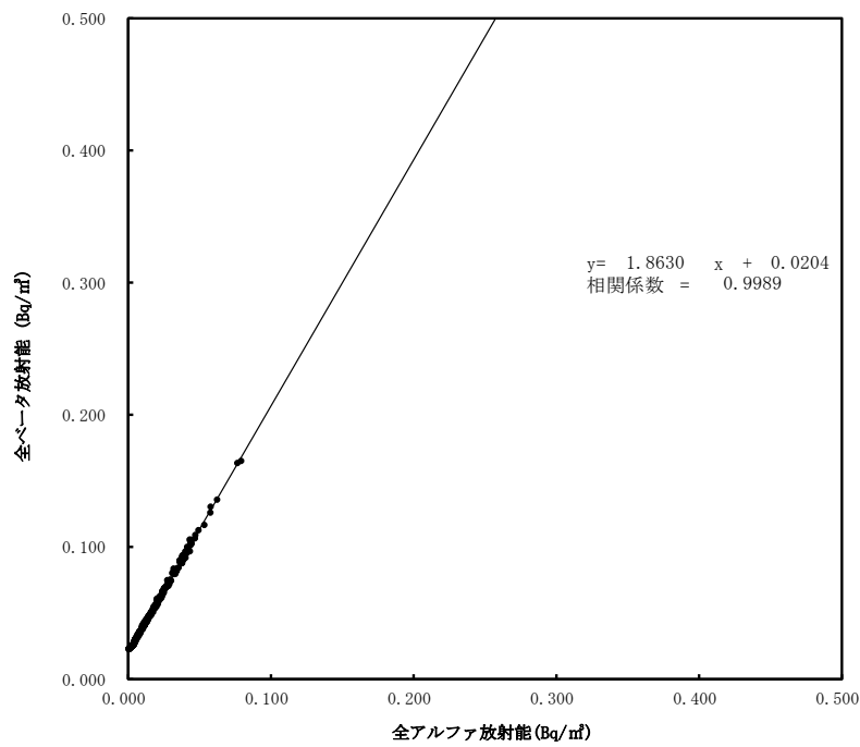
大気浮遊じんの全アルファ・全ベータ放射能の相関図 (6時間連続集じん・6時間放置後) (令和6年7月～9月) (田村市都路馬洗戸)
