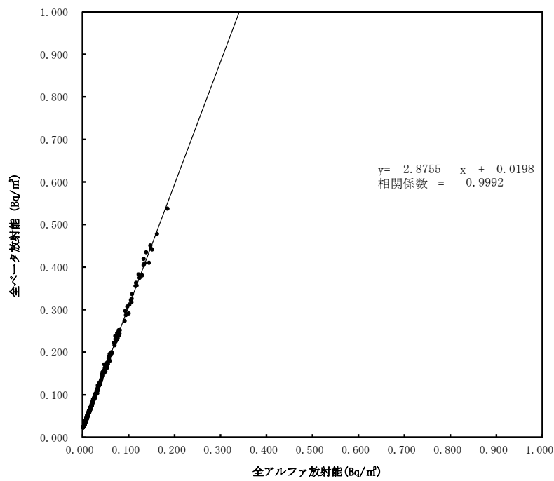
大気浮遊じんの全アルファ・全ベータ放射能の相関図 (6時間連続集じん・6時間放置後) (令和6年7月～9月) (大熊町大野)
