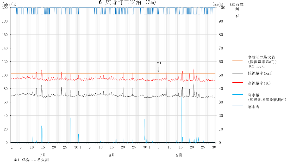
空間線量率の変動グラフ 6 広野町二ツ沼 (3m)
