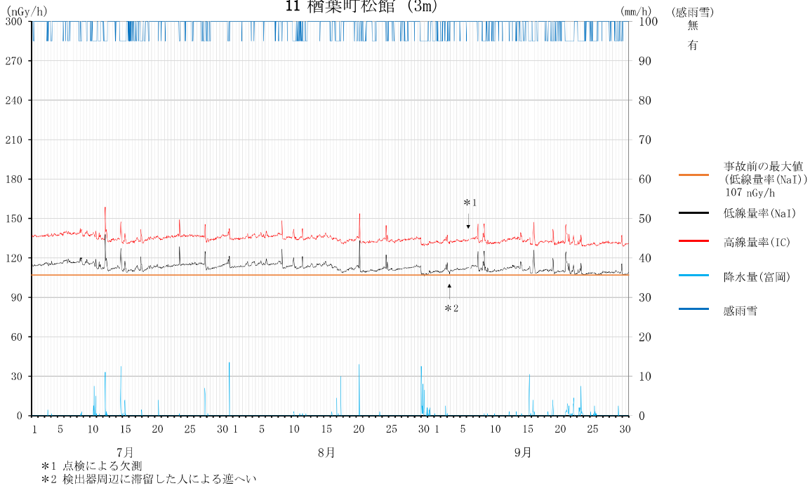
空間線量率の変動グラフ 11 檜葉町松館 (3m)
