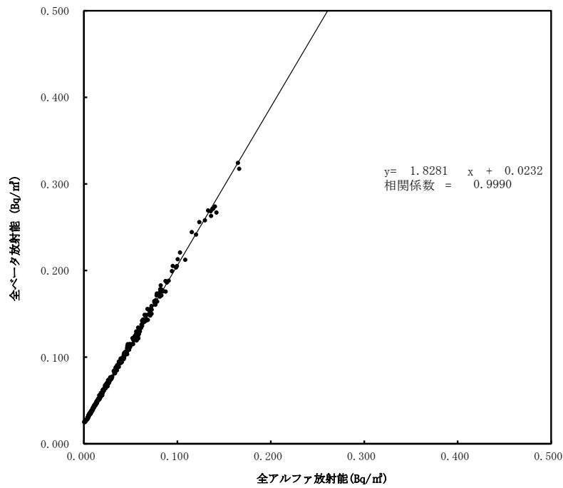
大気浮遊じんの全アルファ・全ベータ放射能の相関図 (6時間連続集じん・6時間放置後) (令和6年7月～9月) (いわき市小川)
