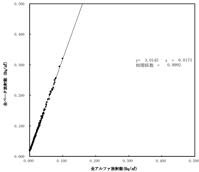
大気浮遊じんの全アルファ・全ベータ放射能の相関図 (6時間連続集じん・6時間放置後) (令和6年7月～9月) (大熊町夫沢)
