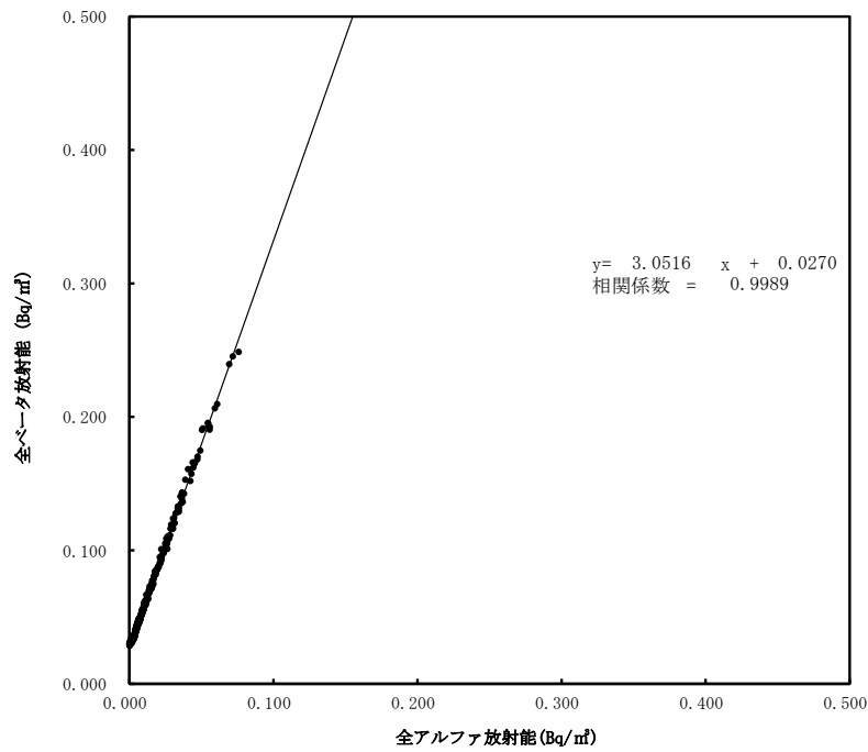
大気浮遊じんの全アルファ・全ベータ放射能の相関図 (6時間連続集じん・6時間放置後) (令和6年7月～9月) (南相馬市萱浜)
