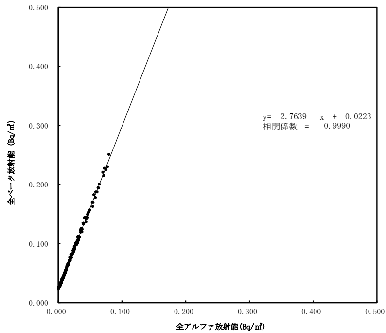
大気浮遊じんの全アルファ・全ベータ放射能の相関図 (6時間連続集じん・6時間放置後) (令和6年7月～9月) (川俣町山木屋)
