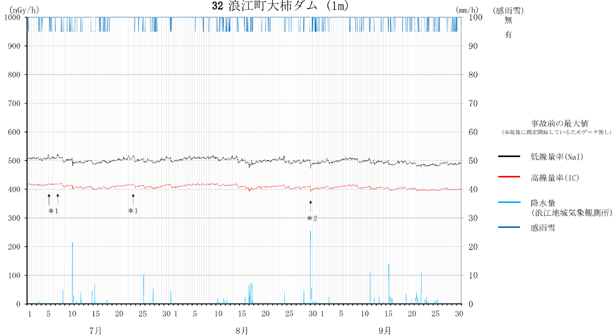
空間線量率の変動グラフ 32 浪江町大柵ダム (1m)
