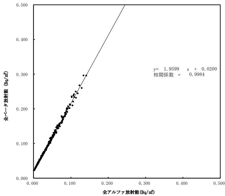
大気浮遊じんの全アルファ・全ベータ放射能の相関図 (6時間連続集じん・6時間放置後) (令和6年7月～9月) (浪江町大柿ダム)
