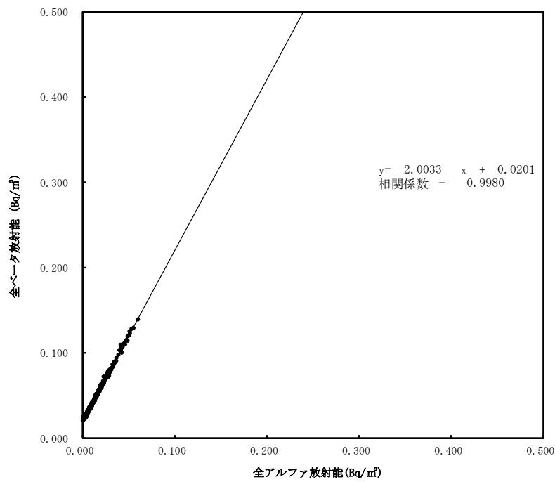
大気浮遊じんの全アルファ・全ベータ放射能の相関図 (6時間連続集じん・6時間放置後) (令和6年7月～9月) (双葉町郡山)
