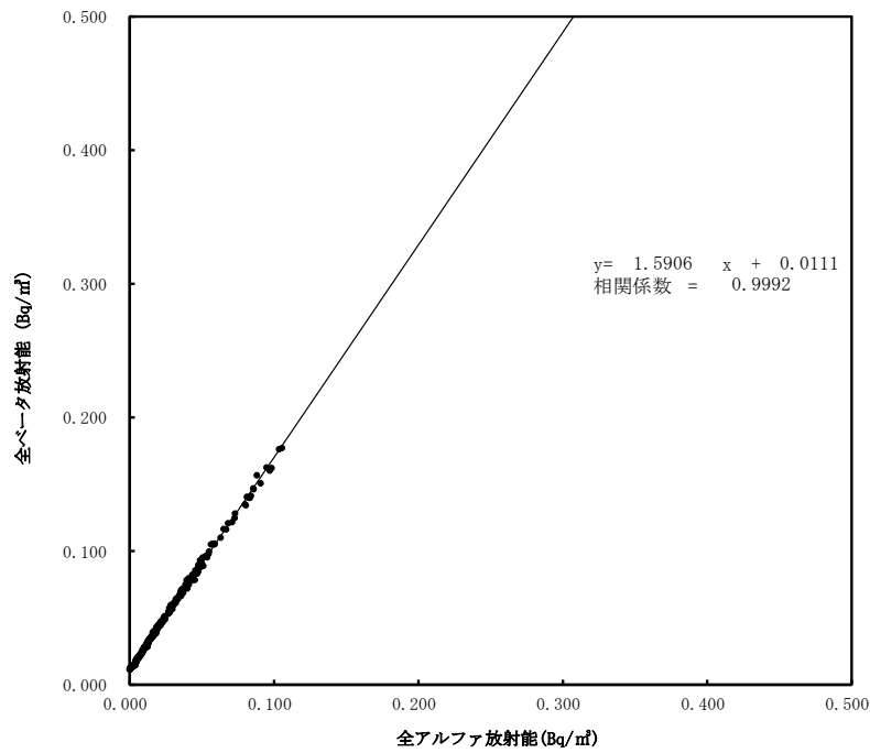
大気浮遊じんの全アルファ・全ベータ放射能の相関図 (6時間連続集じん・6時間放置後) (令和6年7月～9月) (浪江町幾世橋)
