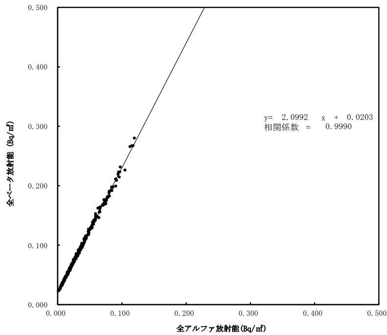
大気浮遊じんの全アルファ・全ベータ放射能の相関図 (6時間連続集じん・6時間放置後) (令和6年7月～9月) (川内村下川内)
