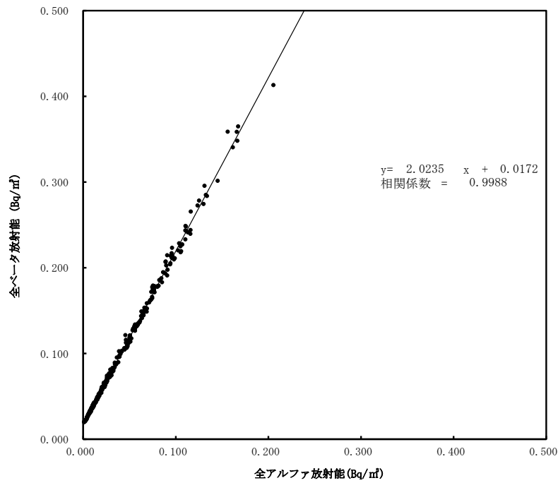
大気浮遊じんの全アルファ・全ベータ放射能の相関図 (6時間連続集じん・6時間放置後) (令和6年7月～9月) (葛尾村夏湯)
