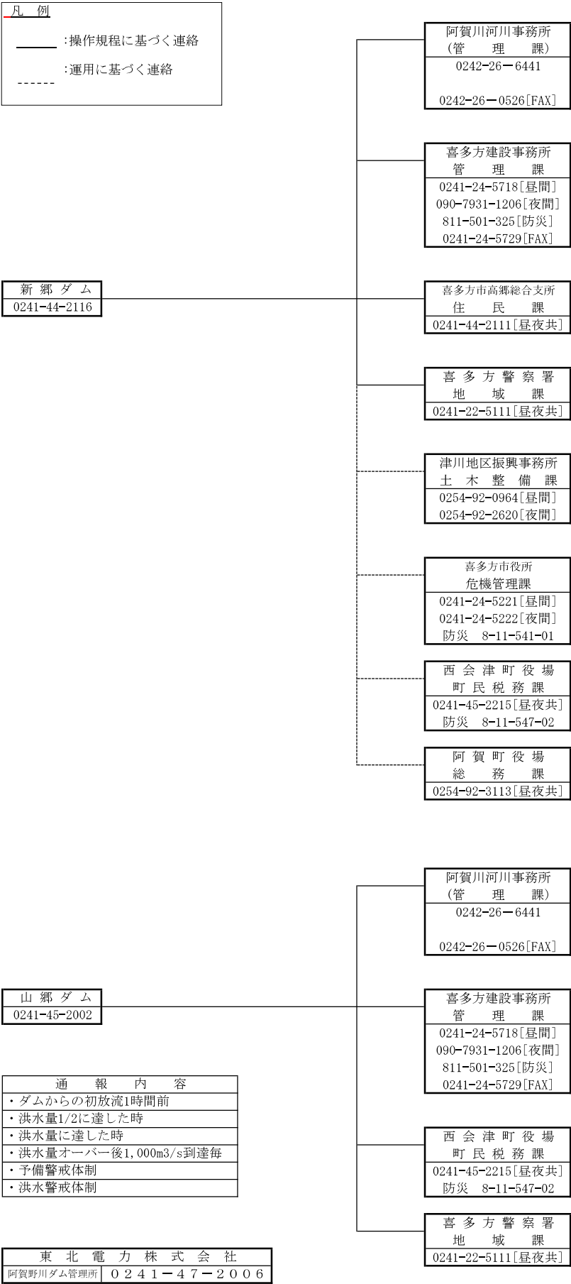
阿賀川関係ダムからの放流連絡系統図（１）
