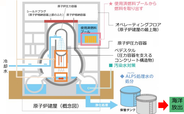
出典：経済産業省「廃炉・汚染水・処理水対策ポータルサイト」を一部加工して作成
