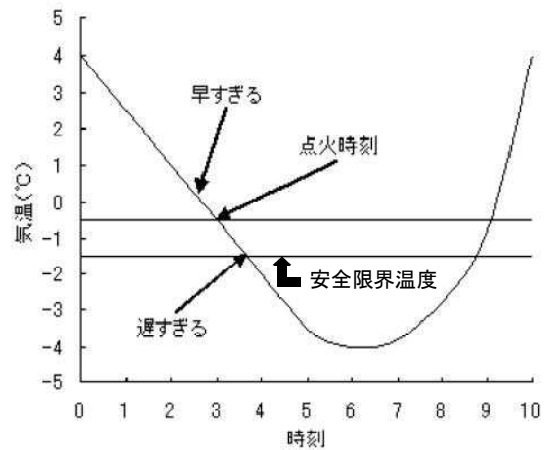
図5 危険限界温度と点火時刻
