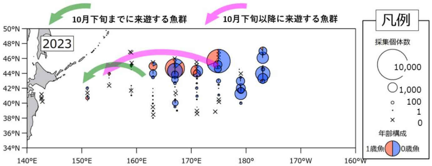
図2 2023年6~7月に行った表層トロールによるサンマ資源量直接推定調査の結果
