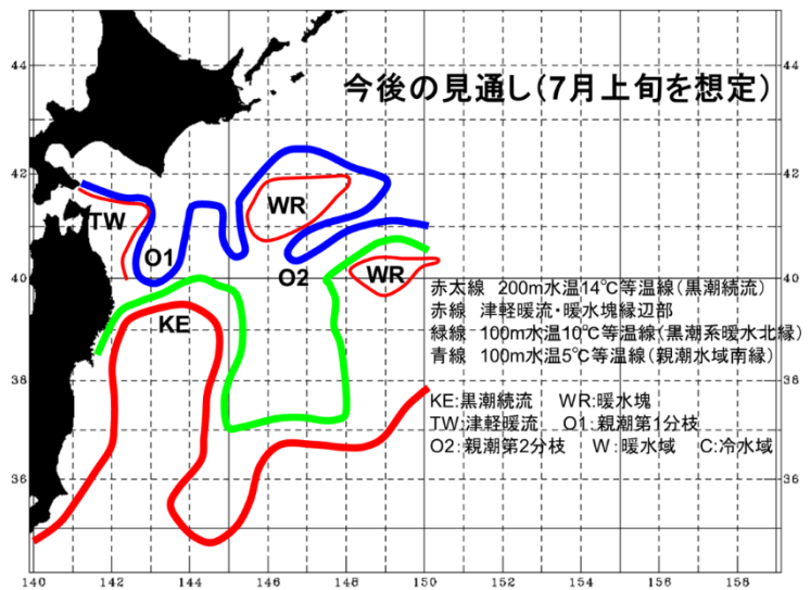
図1 7月上旬予測水温分布図
