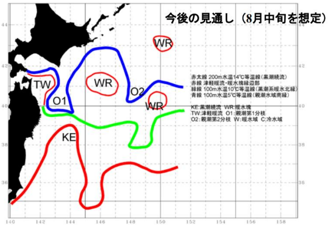
図1 8月中旬予測水温分布図
