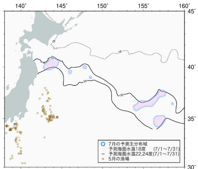
図2 2023年7月のカツオ主分布域の予測
