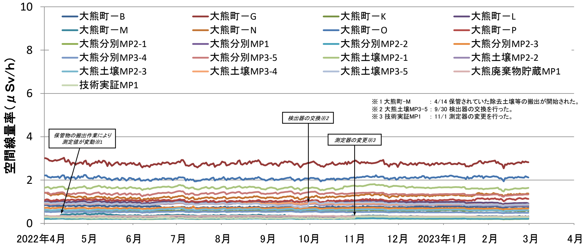
空間線量率の推移(連続測定)(2022年4月1日～2023年2月28日)
