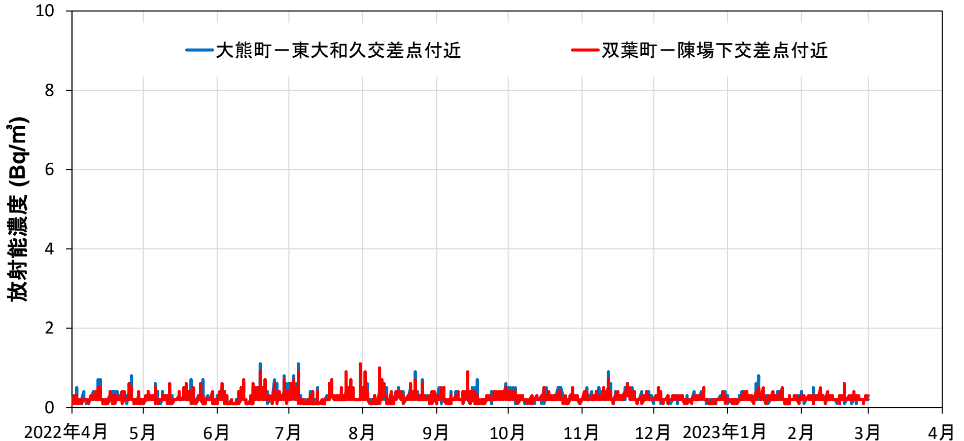
中間貯蔵施設区域境界における大気中の \beta 線の放射能濃度(連続測定) (2022年4月1日~2023年2月28日)
