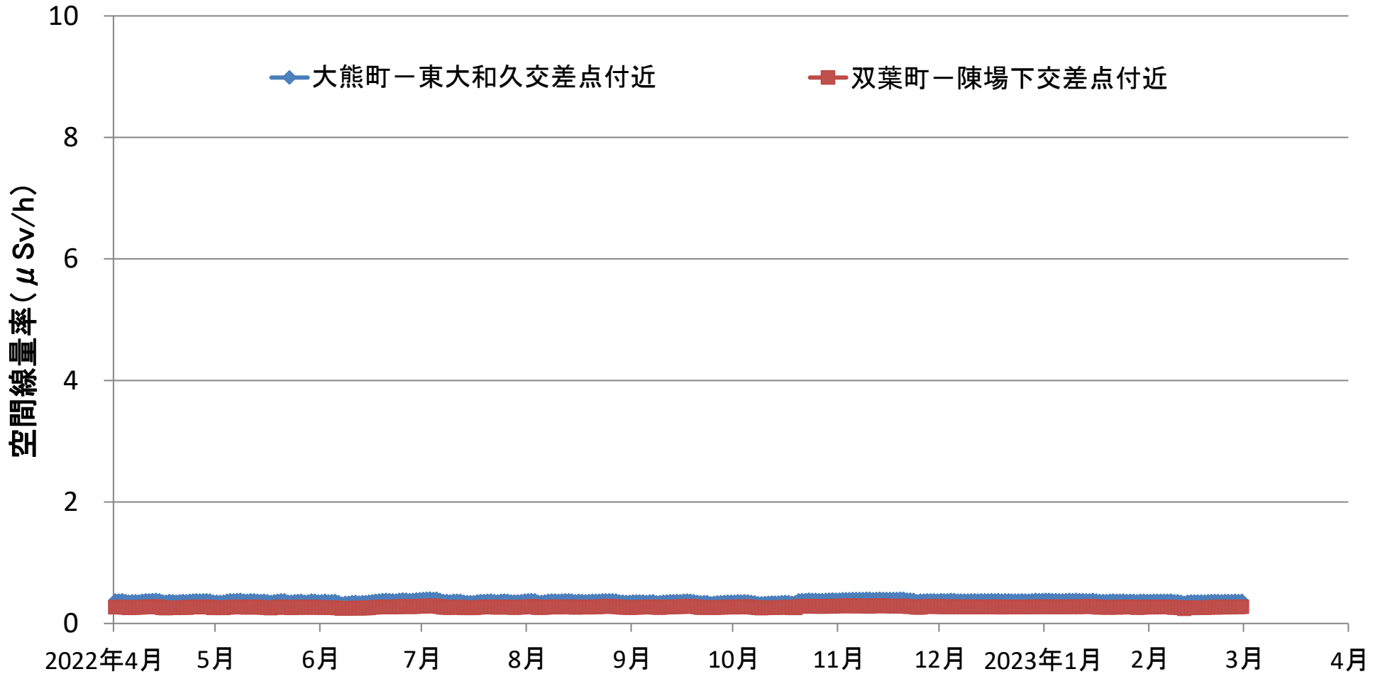
中間貯蔵施設区域境界における空間線量率の推移(連続測定) (2022年4月1日～2023年2月28日)
