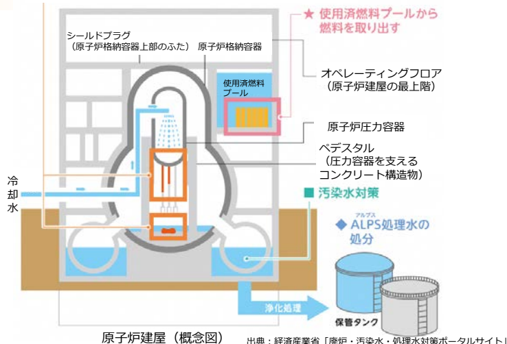
原子炉建屋（概念図）
