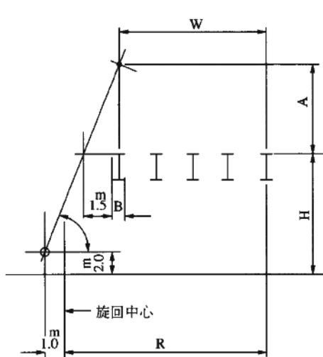
図18. 3 作業半径算定式
