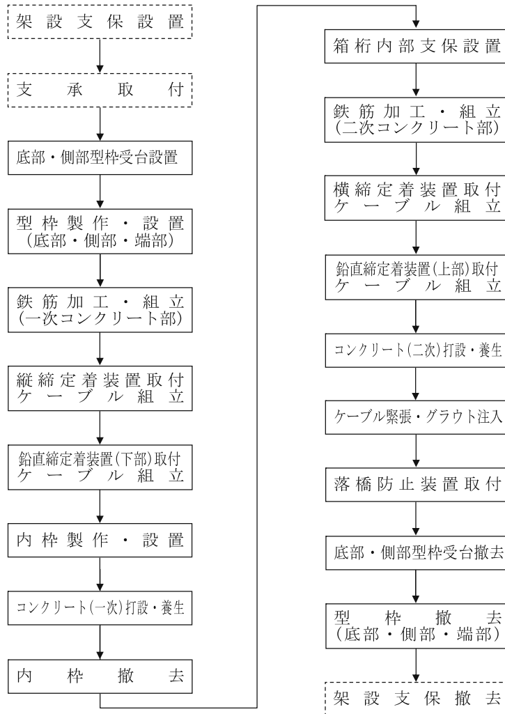
図2-1 施工フロー
