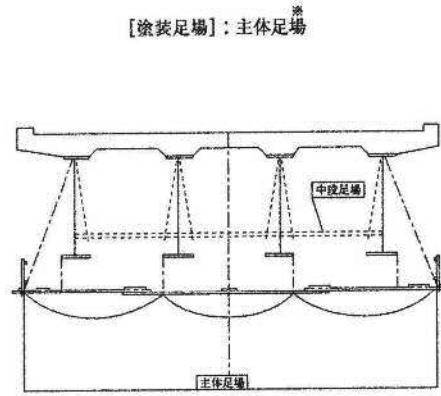
※ 板張防護 (含朝顔) ※桁高1.5m以上の場合は中段足場 (点線部) を設ける
