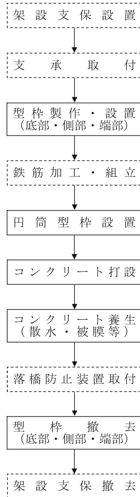
図2-1 施工フロー
