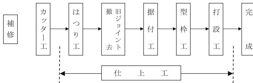
図4-1 施工フロー(鋼フィンガージョイント等)
