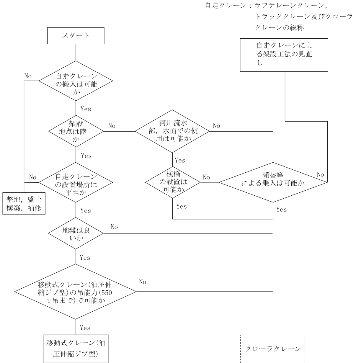
図18.1 機種選定図
