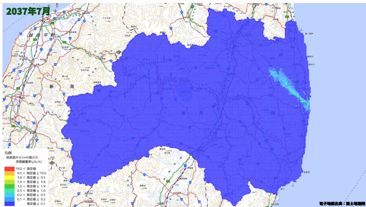
空間線量率分布将来予測解析結果(2037 年 7 月)
