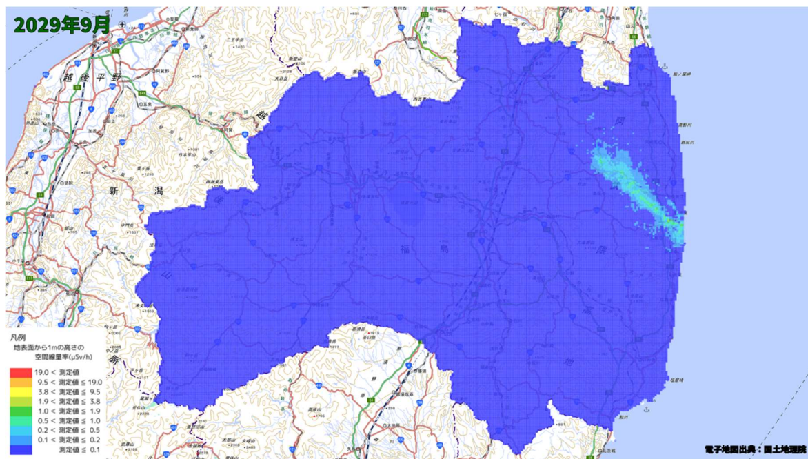
空間線量率分布将来予測解析結果(2029 年 9 月)
