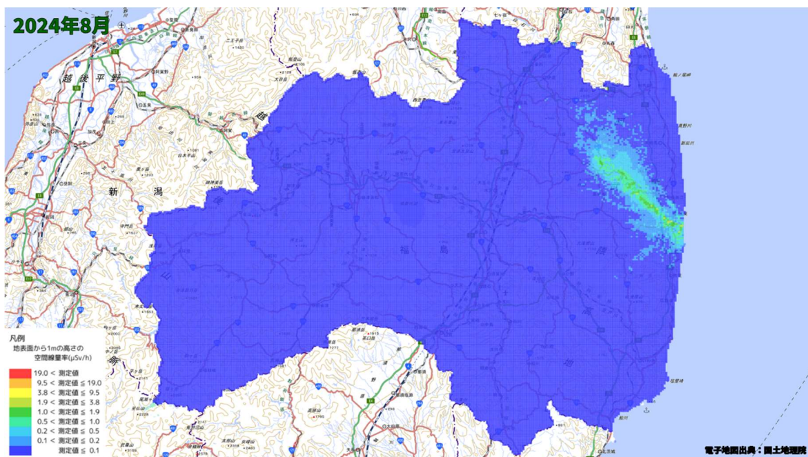
空間線量率分布将来予測解析結果(2024 年 8 月)
