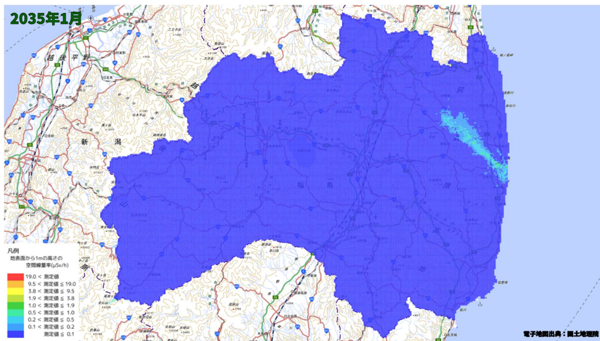
空間線量率分布将来予測解析結果(2035 年 1 月)
