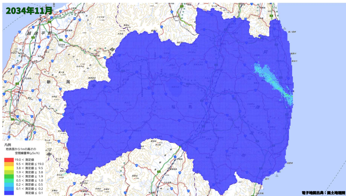
空間線量率分布将来予測解析結果(2034 年 11 月)
