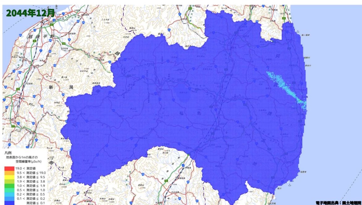
空間線量率分布将来予測解析結果(2044 年 12 月)
