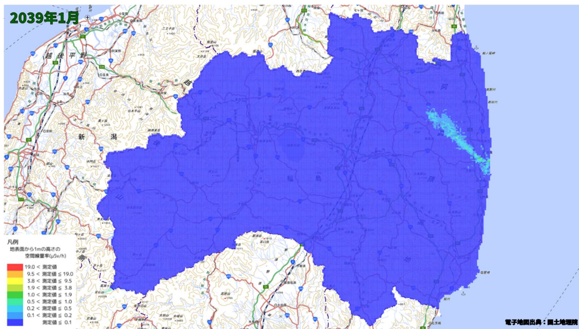
空間線量率分布将来予測解析結果(2039 年 1 月)
