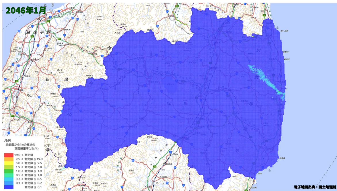
空間線量率分布将来予測解析結果(2046 年 1 月)
