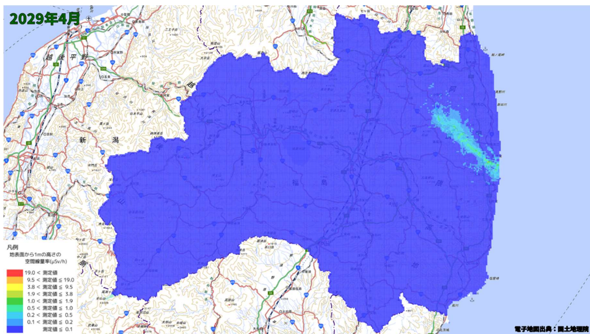
空間線量率分布将来予測解析結果(2029 年 4 月)
