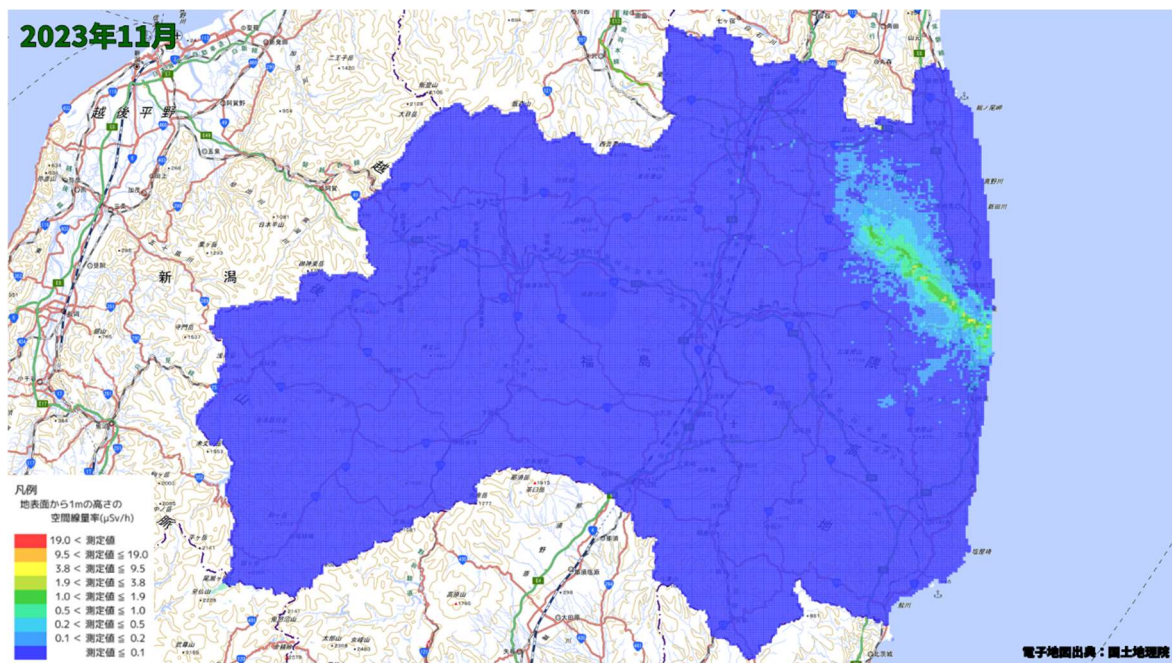
空間線量率分布将来予測解析結果(2023 年 11 月)
