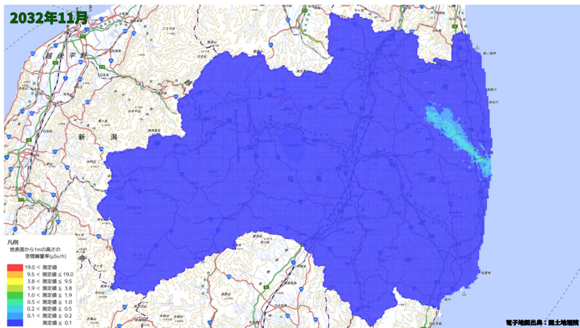
空間線量率分布将来予測解析結果(2032 年 11 月)
