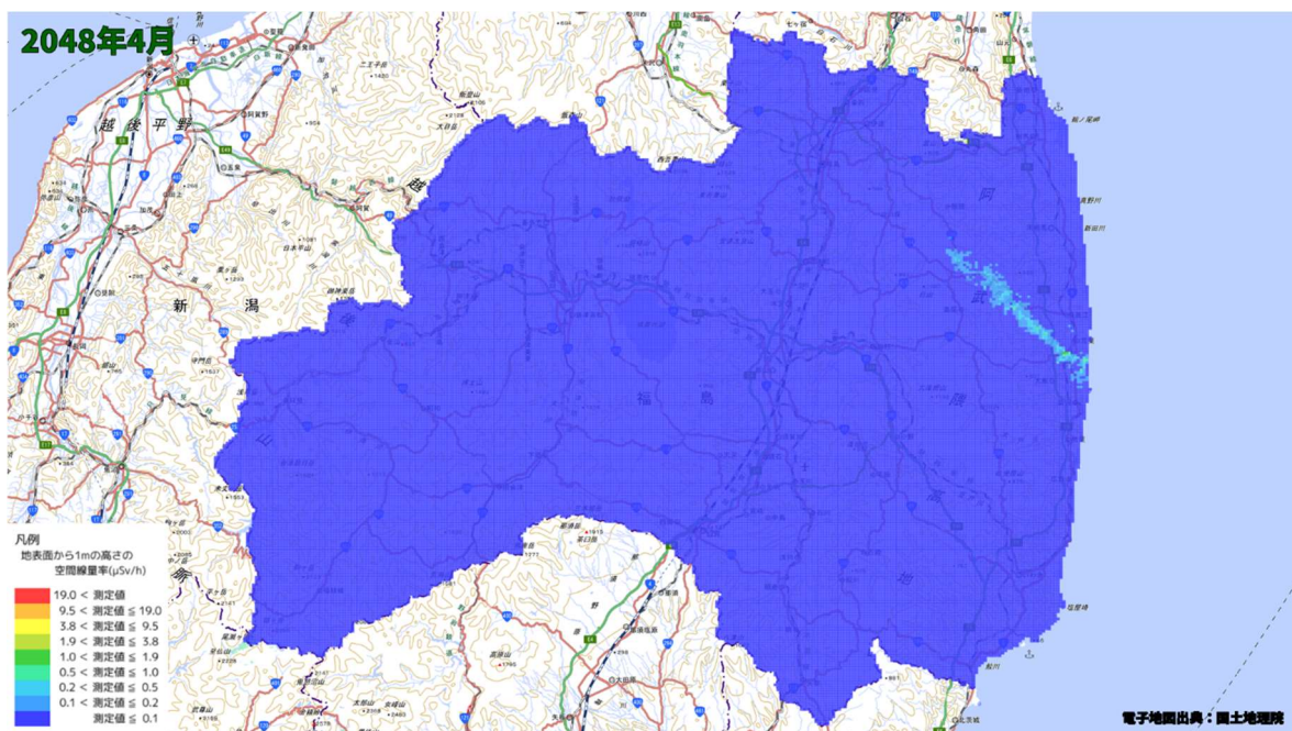
空間線量率分布将来予測解析結果(2048 年 4 月)
