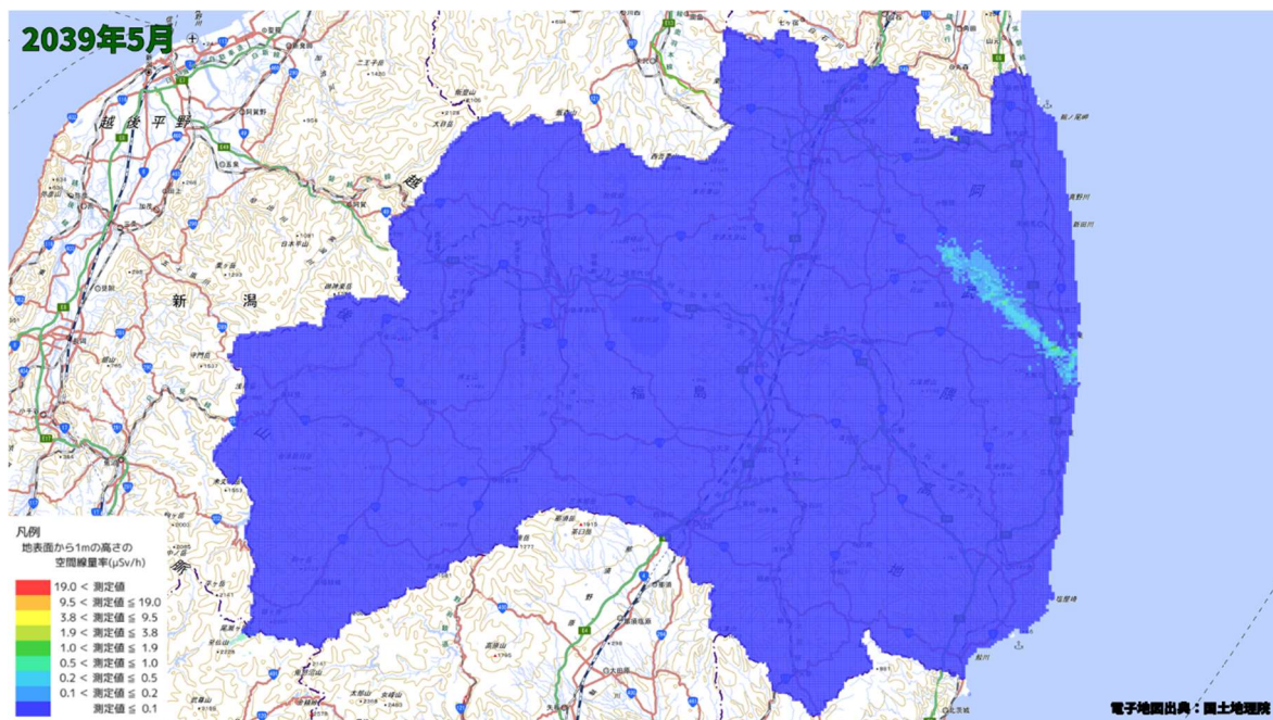
空間線量率分布将来予測解析結果(2039 年 5 月)
