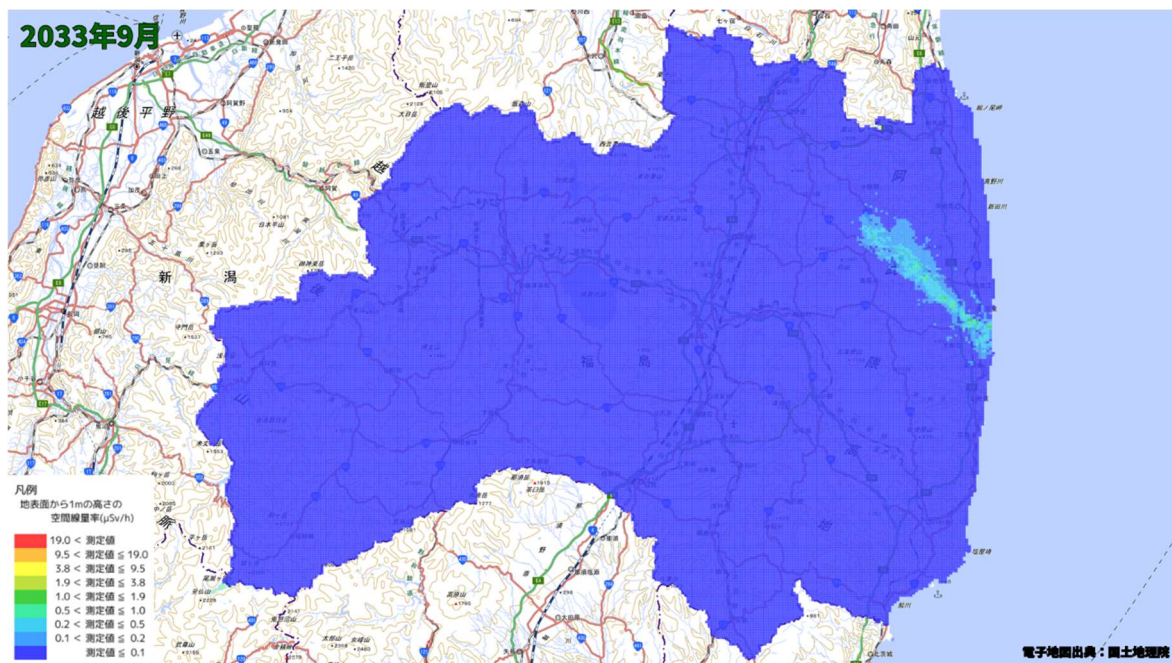
空間線量率分布将来予測解析結果(2033 年 9 月)
