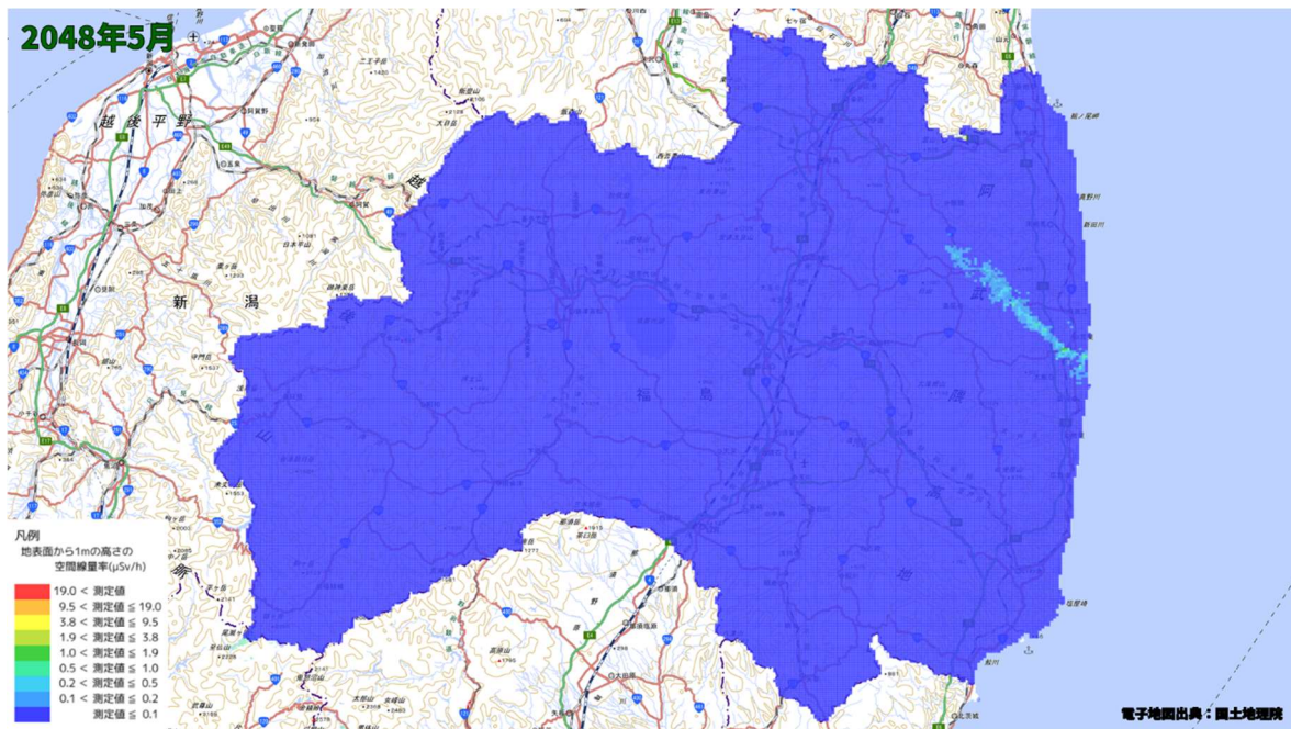
空間線量率分布将来予測解析結果(2048 年 5 月)
