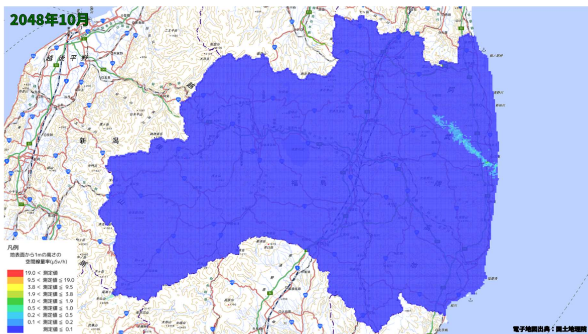
空間線量率分布将来予測解析結果(2048 年 10 月)
