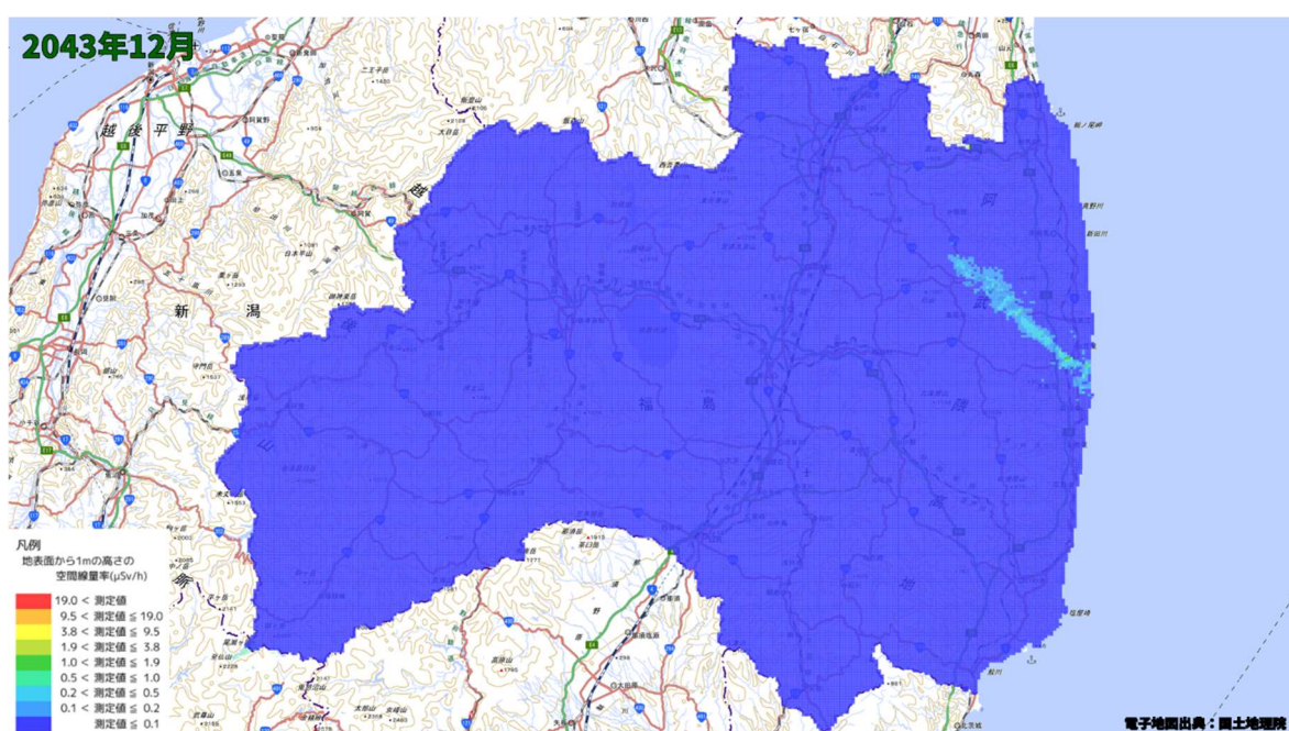
空間線量率分布将来予測解析結果(2043 年 12 月)
