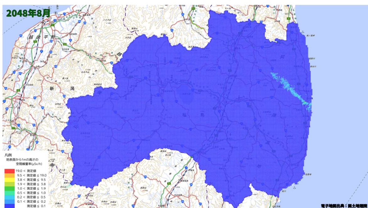
空間線量率分布将来予測解析結果(2048 年 8 月)
