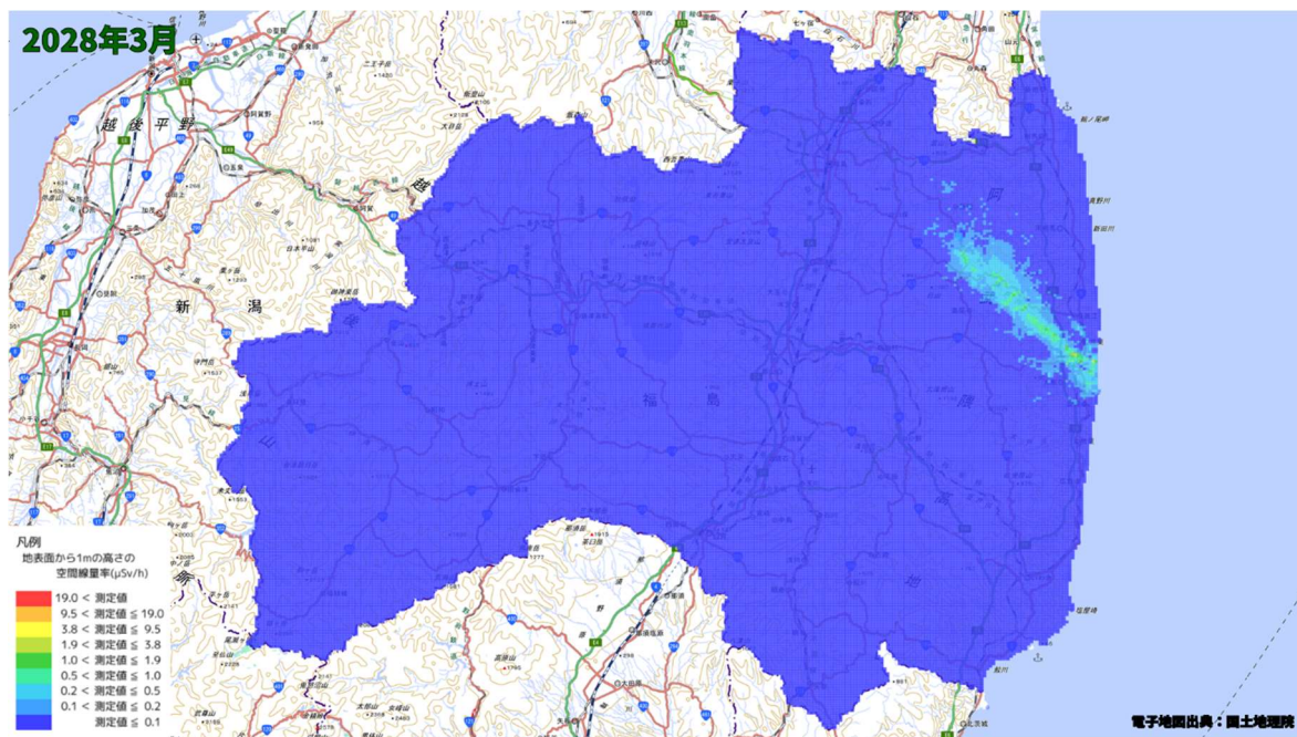
空間線量率分布将来予測解析結果(2028 年 3 月)
