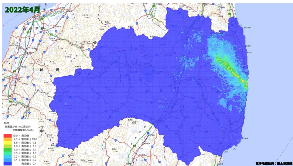
空間線量率分布将来予測解析結果(2022 年 4 月)
