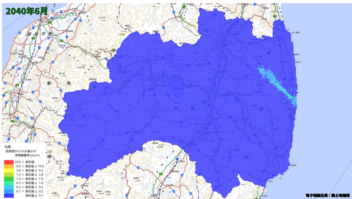
空間線量率分布将来予測解析結果(2040 年 6 月)
