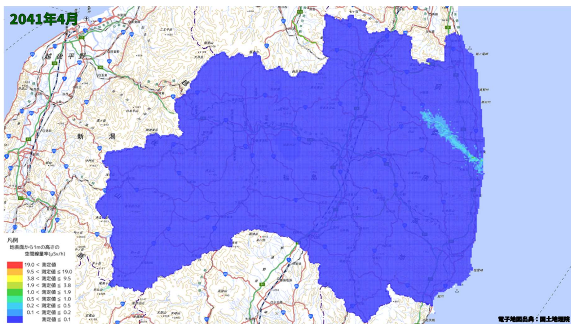
空間線量率分布将来予測解析結果(2041 年 4 月)
