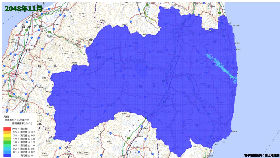
空間線量率分布将来予測解析結果(2048 年 11 月)
