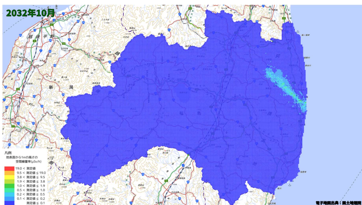
空間線量率分布将来予測解析結果(2032 年 10 月)
