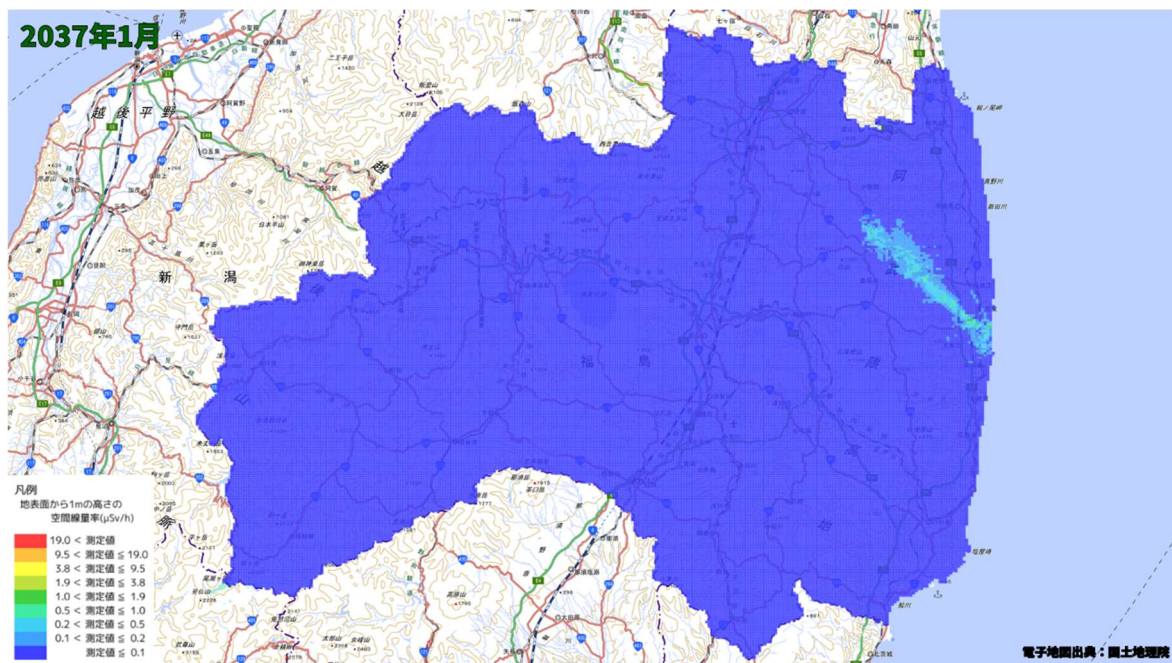
空間線量率分布将来予測解析結果(2037 年 1 月)
