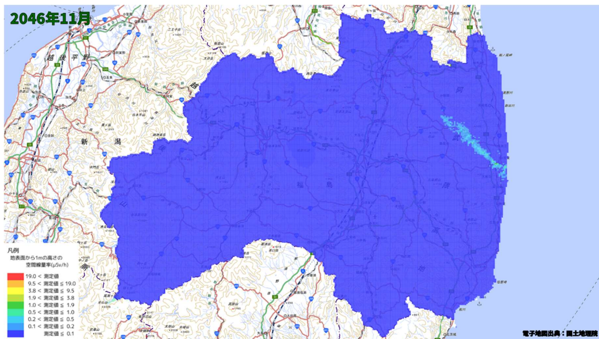
空間線量率分布将来予測解析結果(2046 年 11 月)
