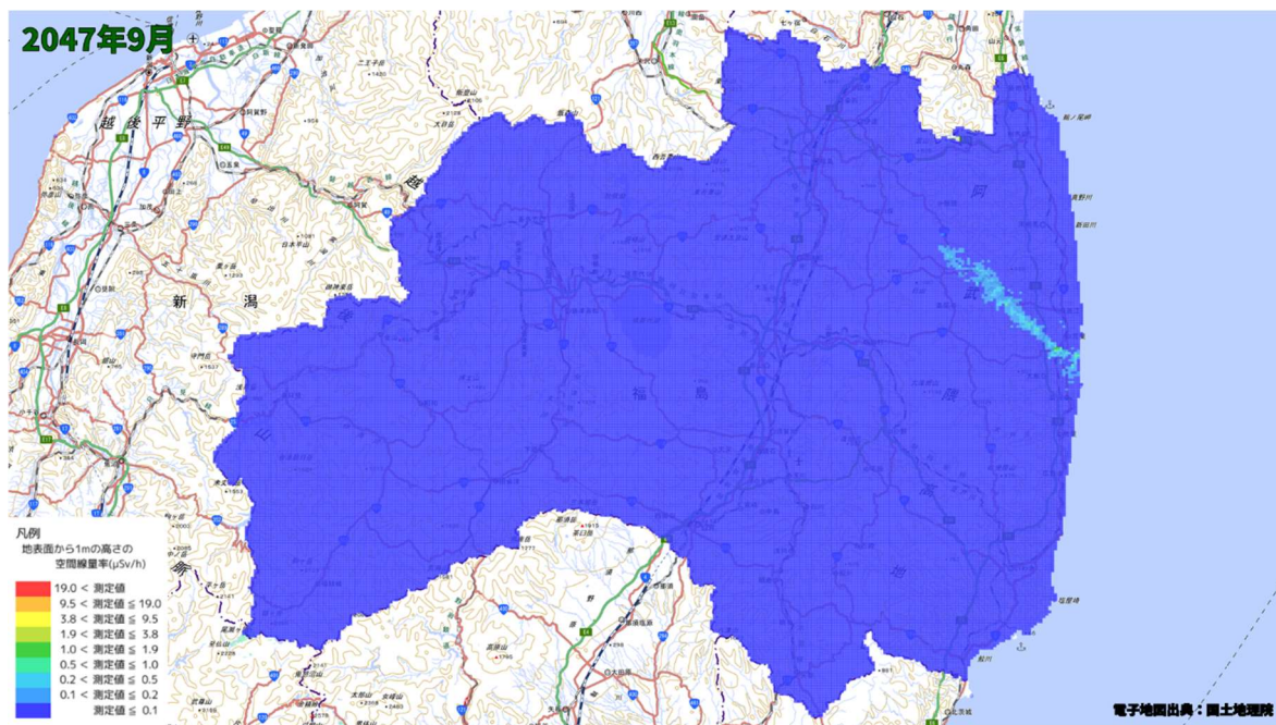
空間線量率分布将来予測解析結果(2047 年 9 月)
