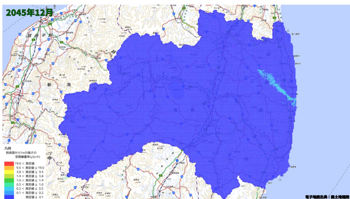
空間線量率分布将来予測解析結果(2045 年 12 月)
