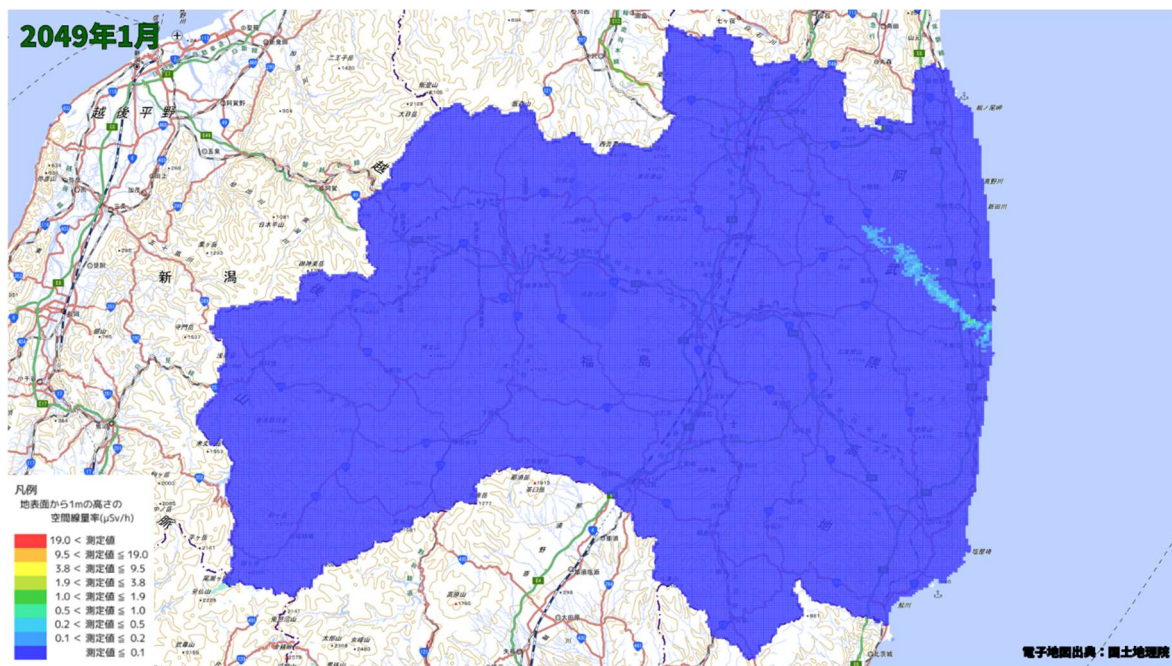
空間線量率分布将来予測解析結果(2049 年 1 月)
