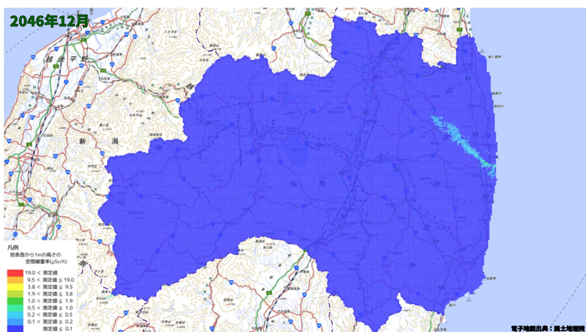
空間線量率分布将来予測解析結果(2046 年 12 月)
