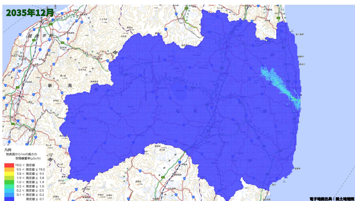
空間線量率分布将来予測解析結果(2035 年 12 月)
