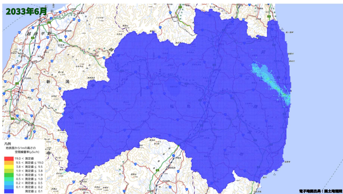
空間線量率分布将来予測解析結果(2033 年 6 月)
