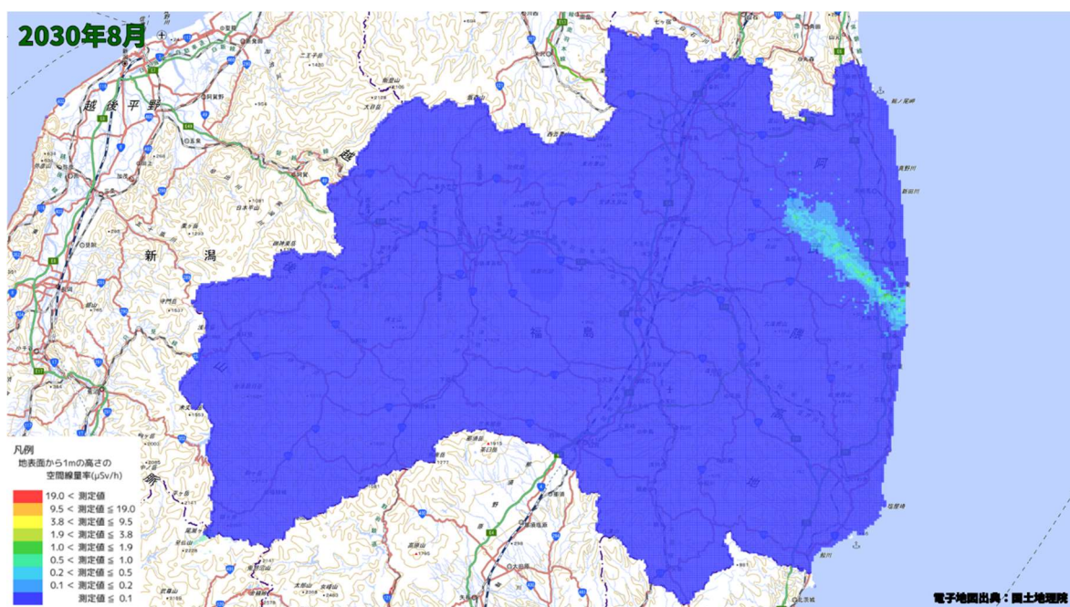
空間線量率分布将来予測解析結果(2030 年 8 月)
