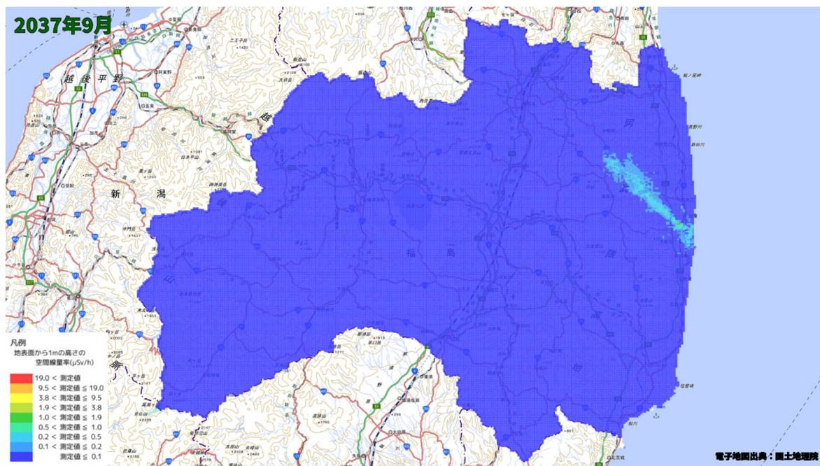
空間線量率分布将来予測解析結果(2037 年 9 月)
