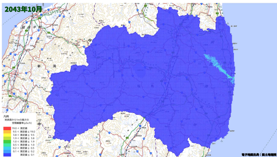
空間線量率分布将来予測解析結果(2043 年 10 月)
