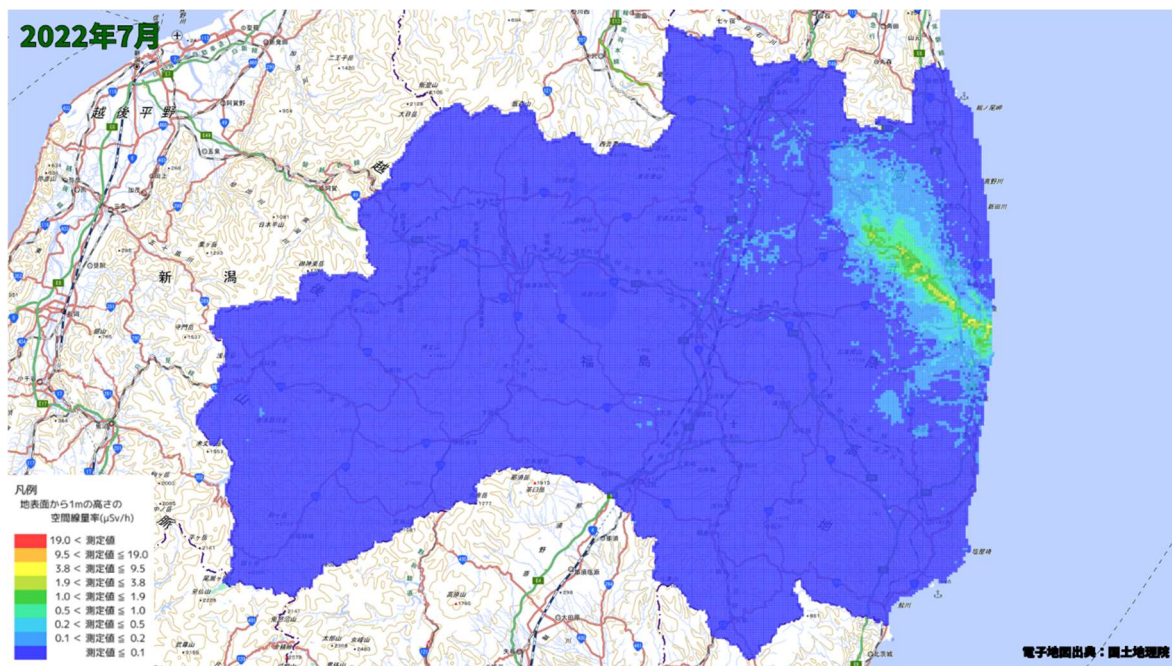
空間線量率分布将来予測解析結果(2022 年 7 月)
