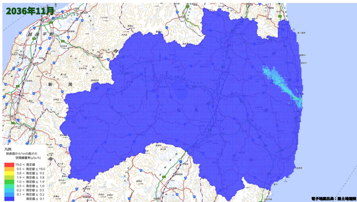
空間線量率分布将来予測解析結果(2036 年 11 月)
