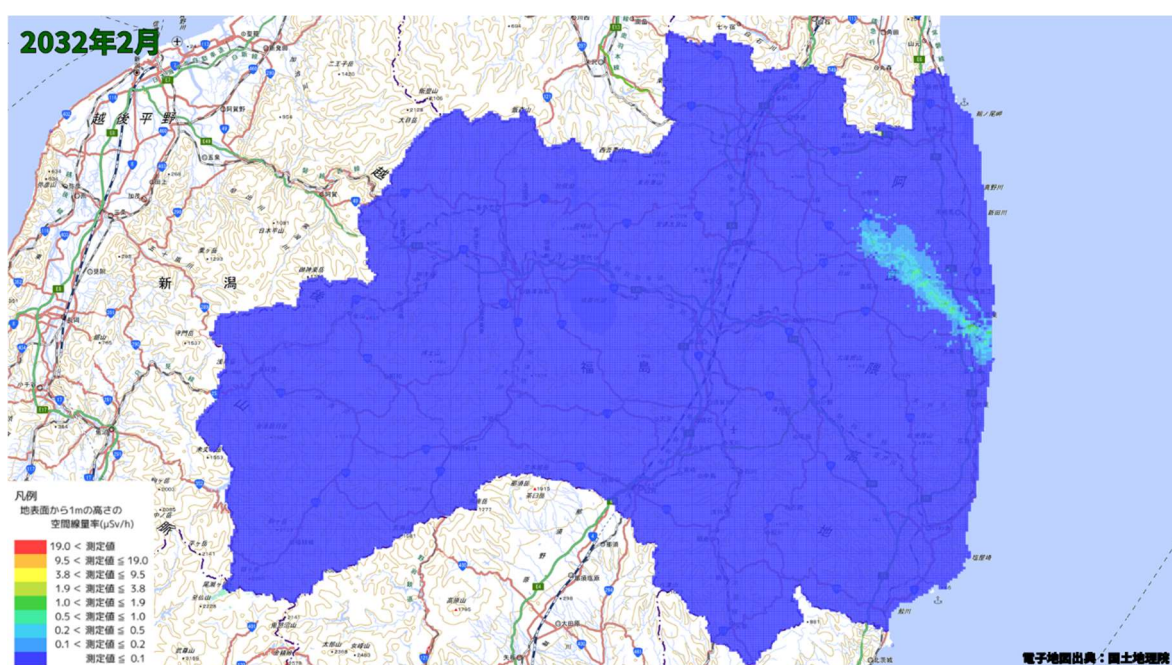
空間線量率分布将来予測解析結果(2032 年 2 月)
