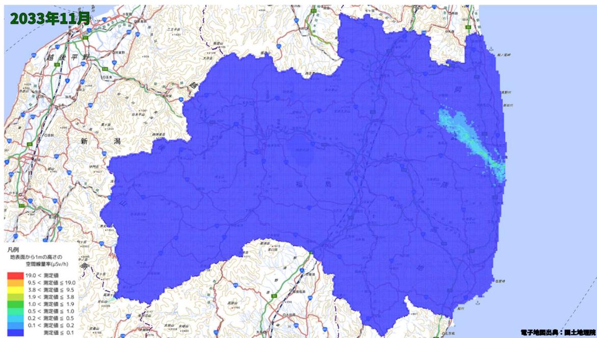
空間線量率分布将来予測解析結果(2033 年 11 月)
