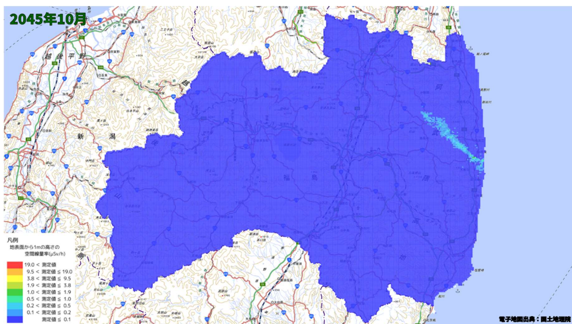
空間線量率分布将来予測解析結果(2045 年 10 月)
