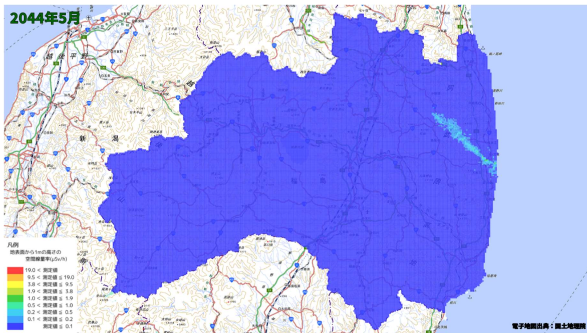
空間線量率分布将来予測解析結果(2044 年 5 月)
