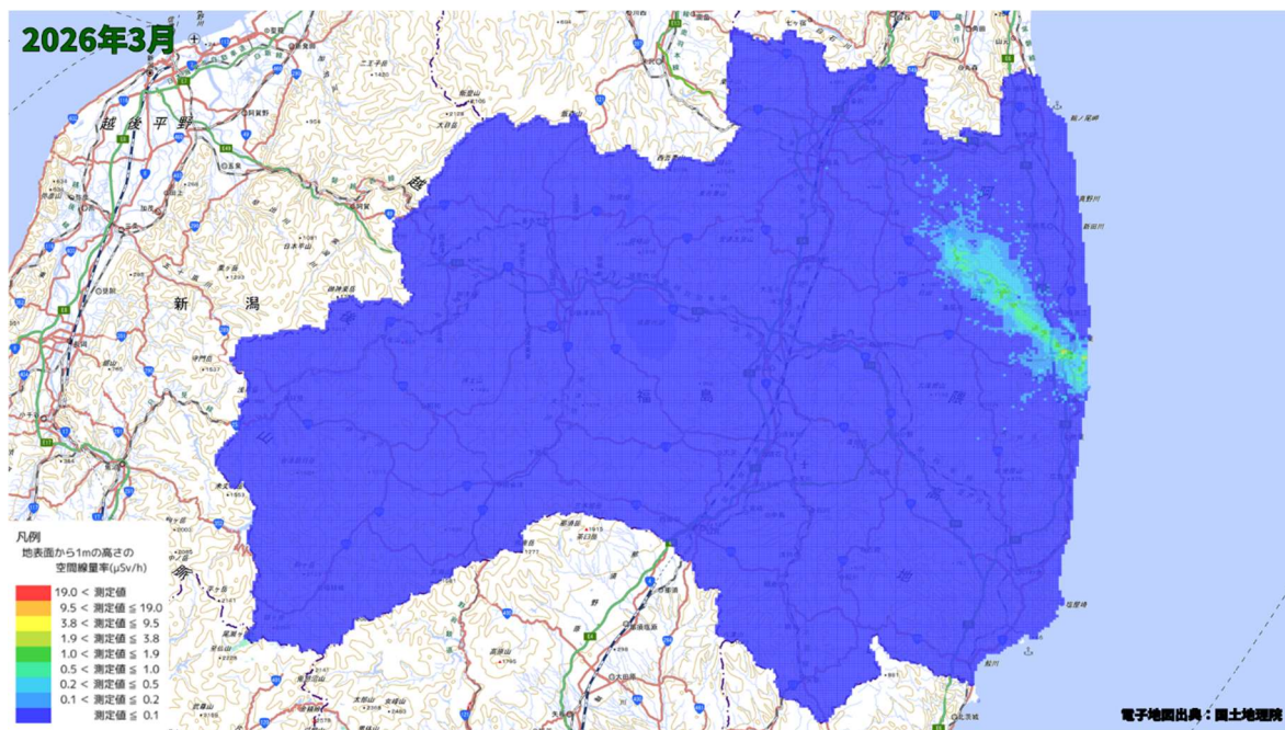
空間線量率分布将来予測解析結果(2026 年 3 月)
