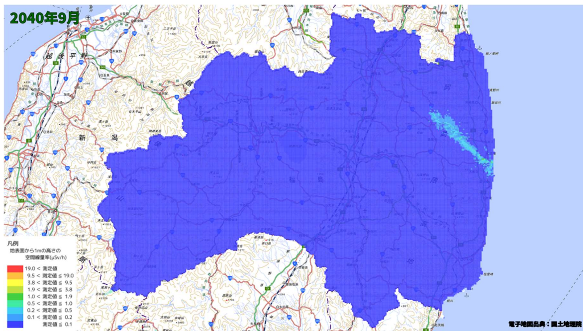
空間線量率分布将来予測解析結果(2040 年 9 月)
