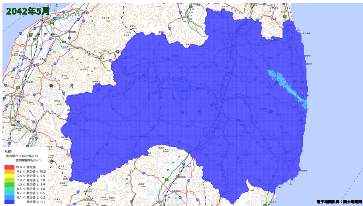
空間線量率分布将来予測解析結果(2042 年 5 月)
