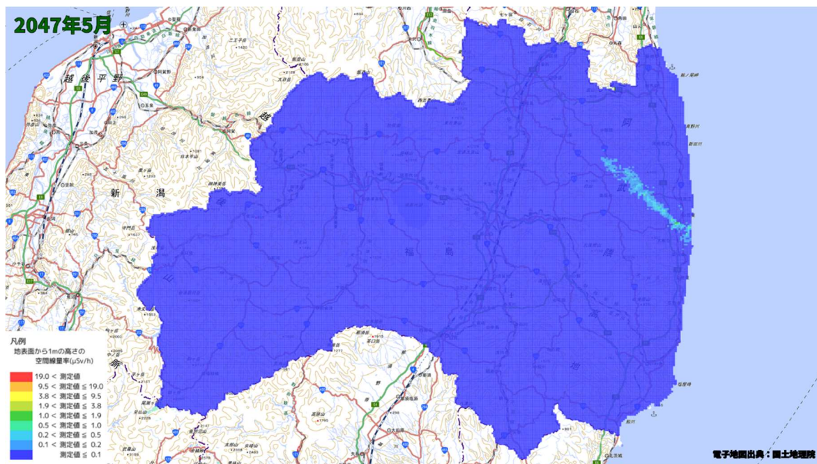
空間線量率分布将来予測解析結果(2047 年 5 月)
