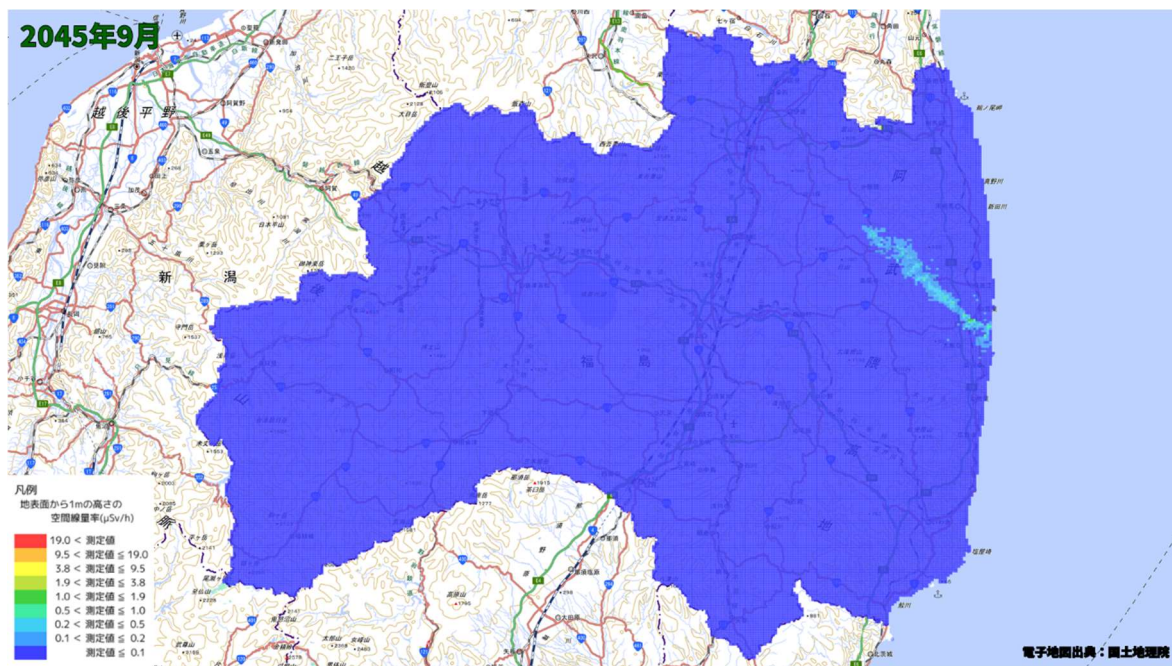
空間線量率分布将来予測解析結果(2045 年 9 月)
