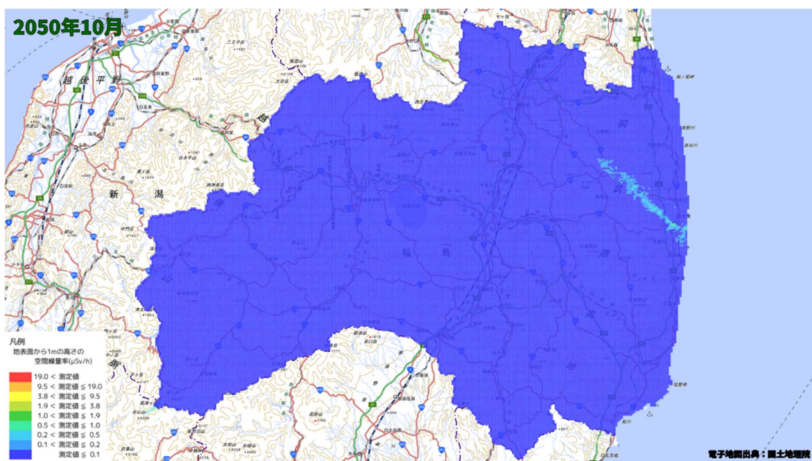
空間線量率分布将来予測解析結果(2050 年 10 月)
