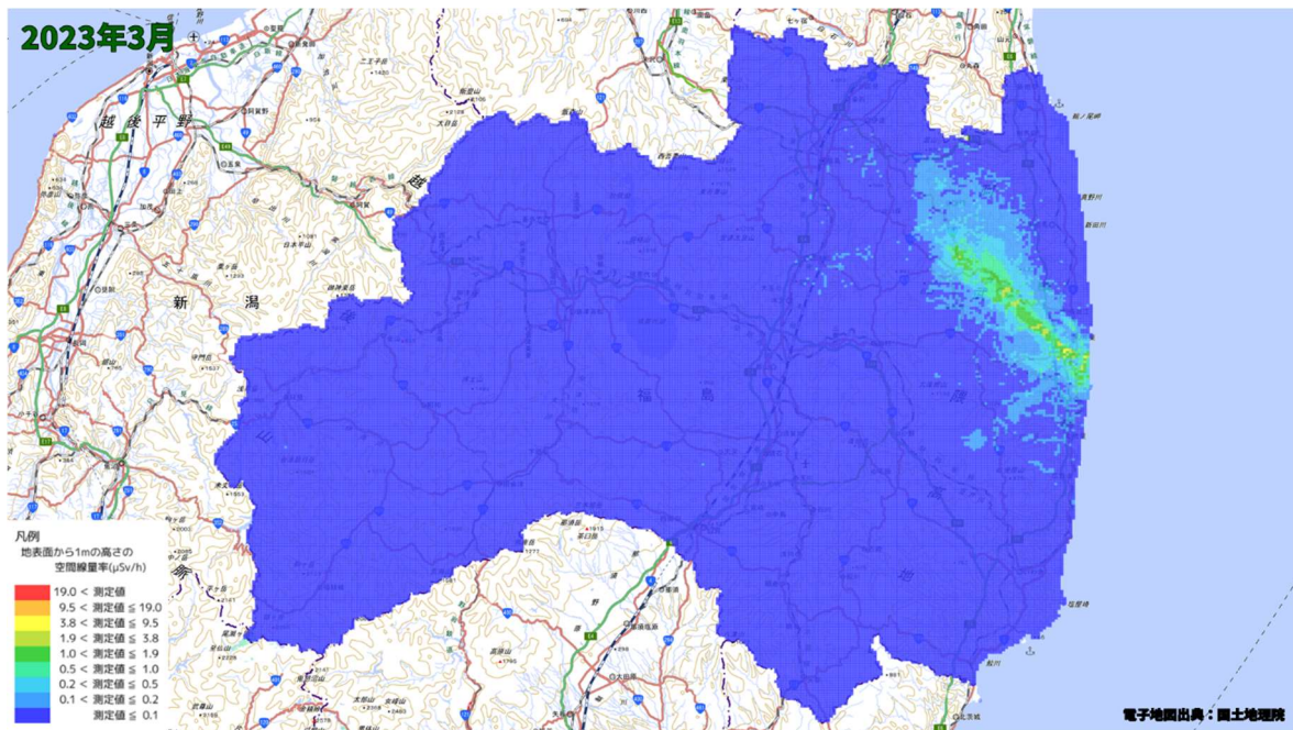
空間線量率分布将来予測解析結果(2023 年 3 月)
