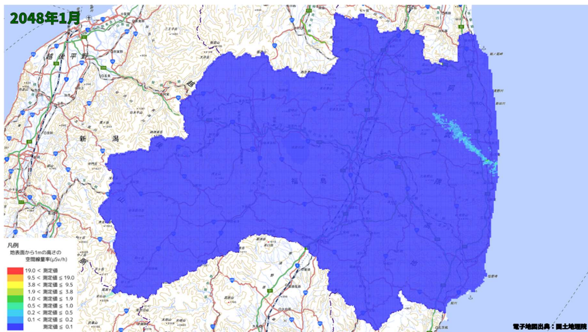
空間線量率分布将来予測解析結果(2048 年 1 月)
