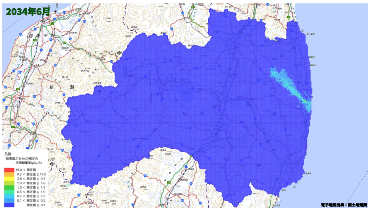
空間線量率分布将来予測解析結果(2034 年 6 月)
