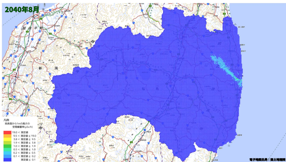
空間線量率分布将来予測解析結果(2040 年 8 月)
