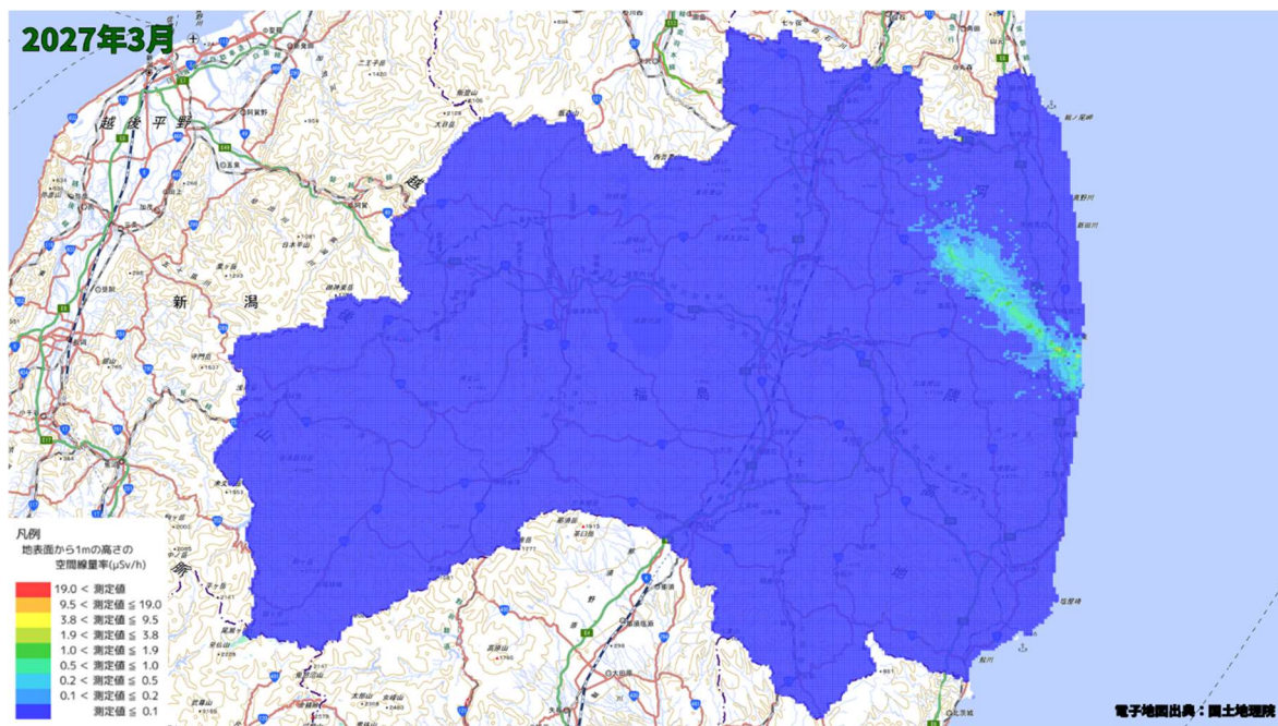
空間線量率分布将来予測解析結果(2027 年 3 月)
