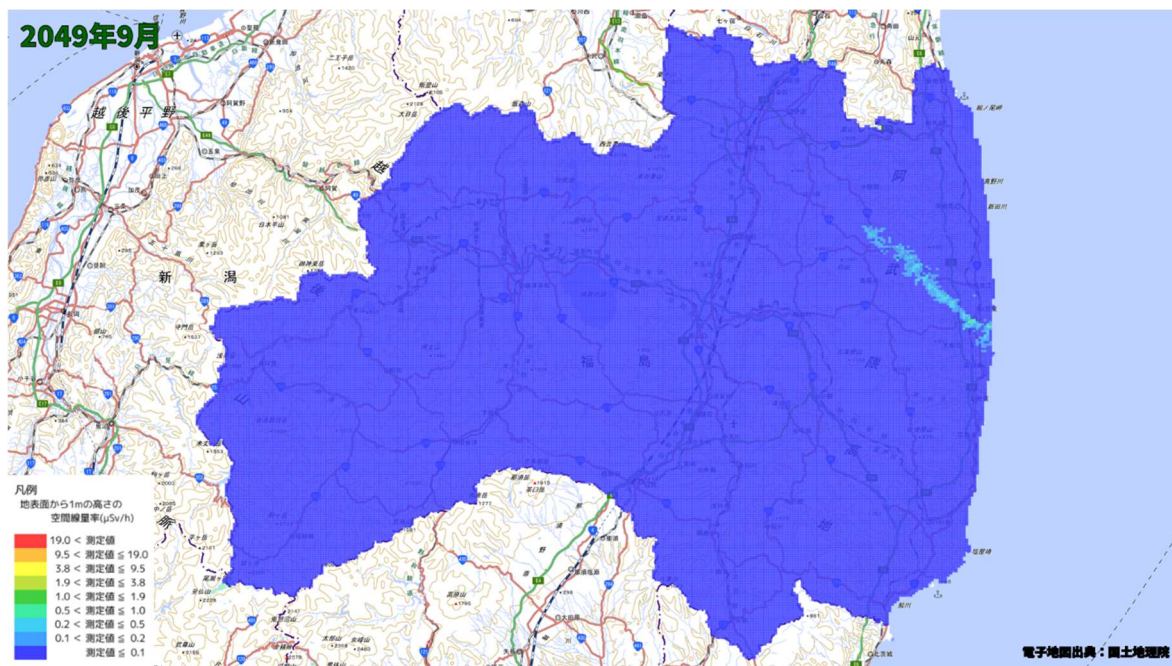
空間線量率分布将来予測解析結果(2049 年 9 月)
