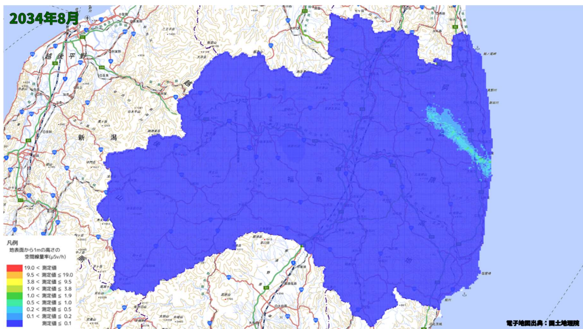
空間線量率分布将来予測解析結果(2034 年 8 月)
