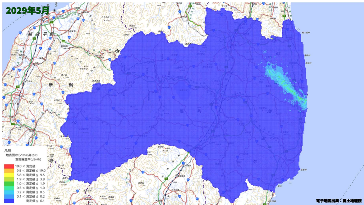
空間線量率分布将来予測解析結果(2029 年 5 月)
