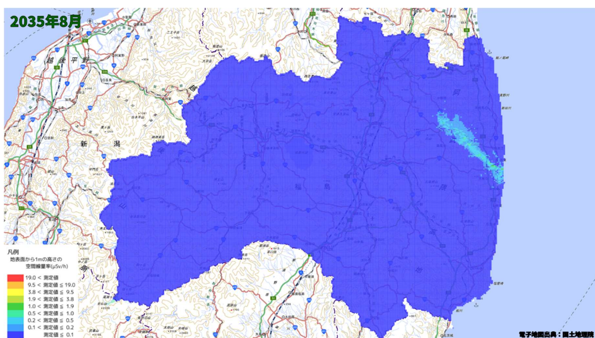
空間線量率分布将来予測解析結果(2035 年 8 月)
