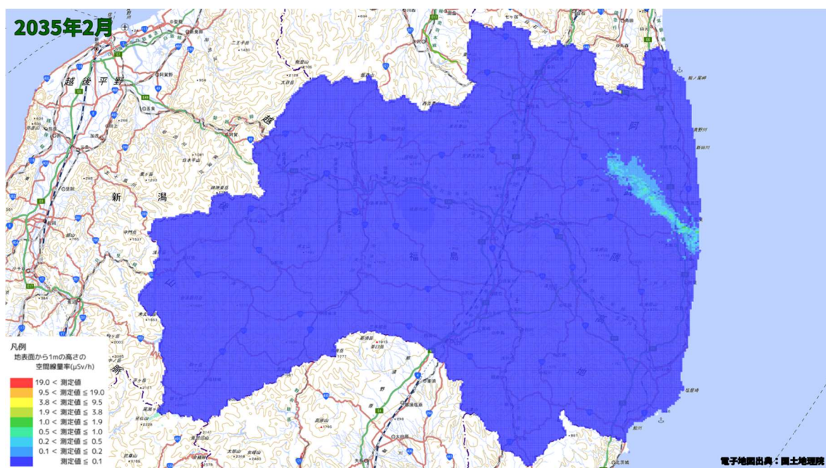
空間線量率分布将来予測解析結果(2035 年 2 月)
