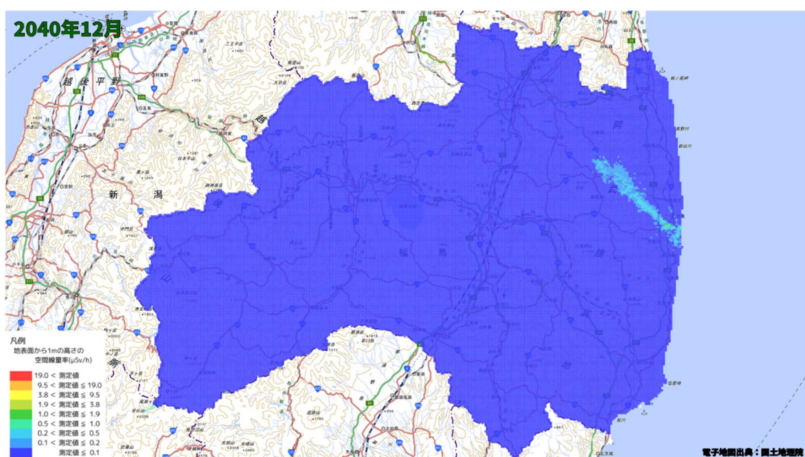
空間線量率分布将来予測解析結果(2040 年 12 月)
