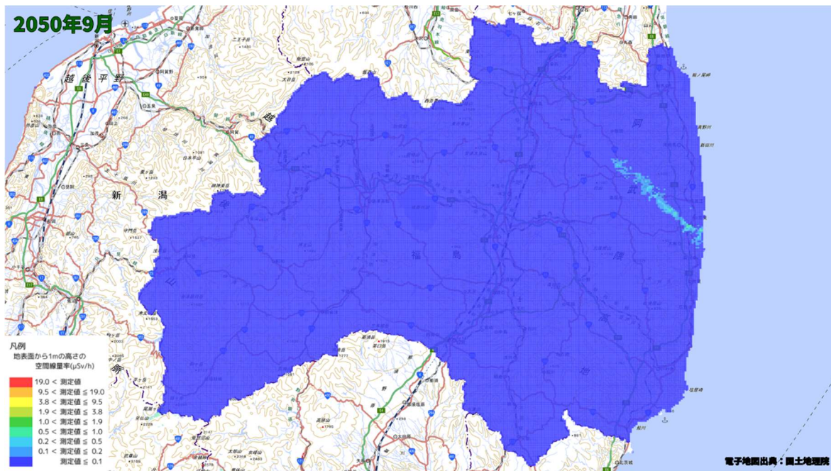
空間線量率分布将来予測解析結果(2050 年 9 月)
