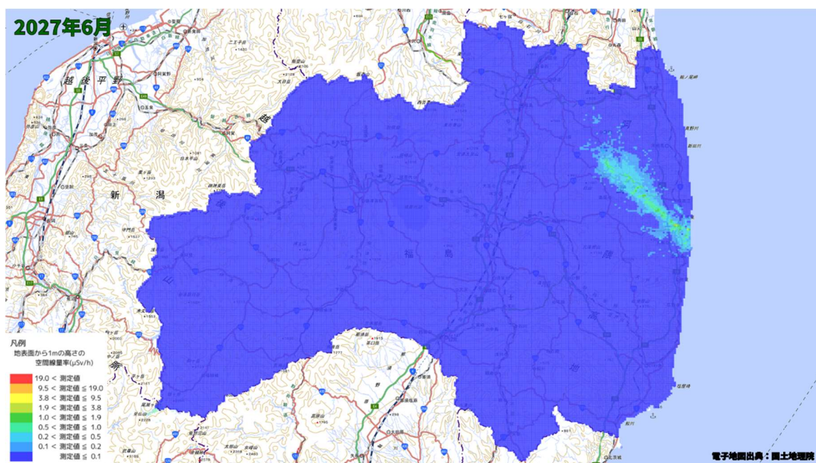
空間線量率分布将来予測解析結果(2027 年 6 月)
