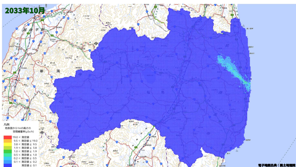
空間線量率分布将来予測解析結果(2033 年 10 月)
