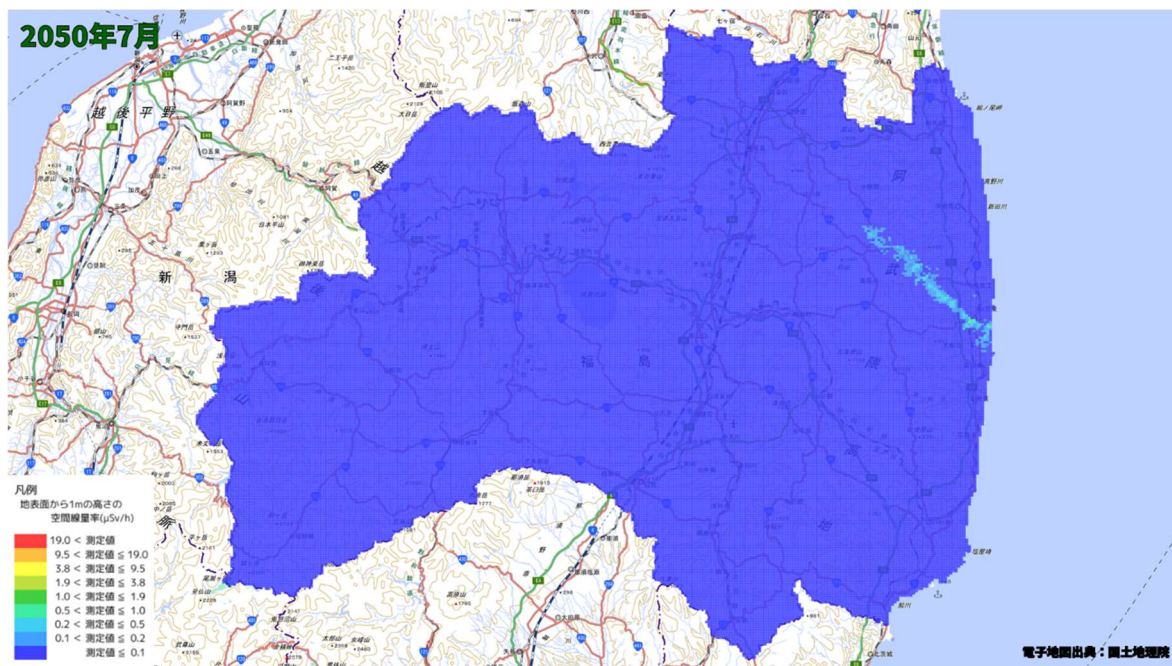
空間線量率分布将来予測解析結果(2050 年 7 月)
