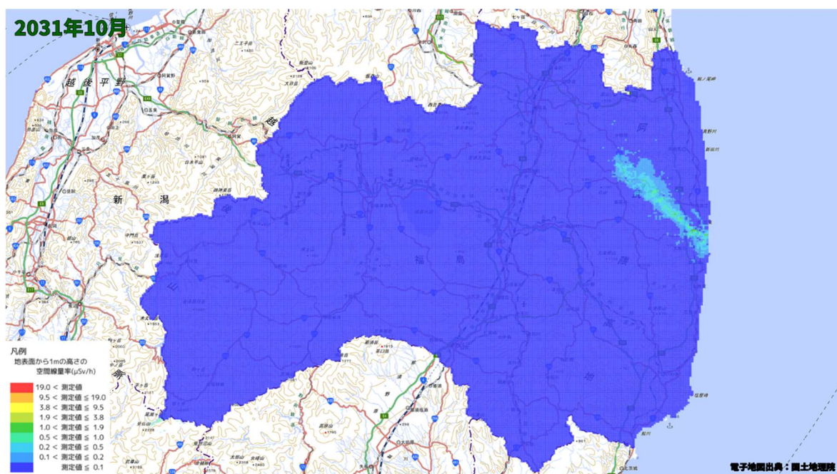
空間線量率分布将来予測解析結果(2031 年 10 月)
