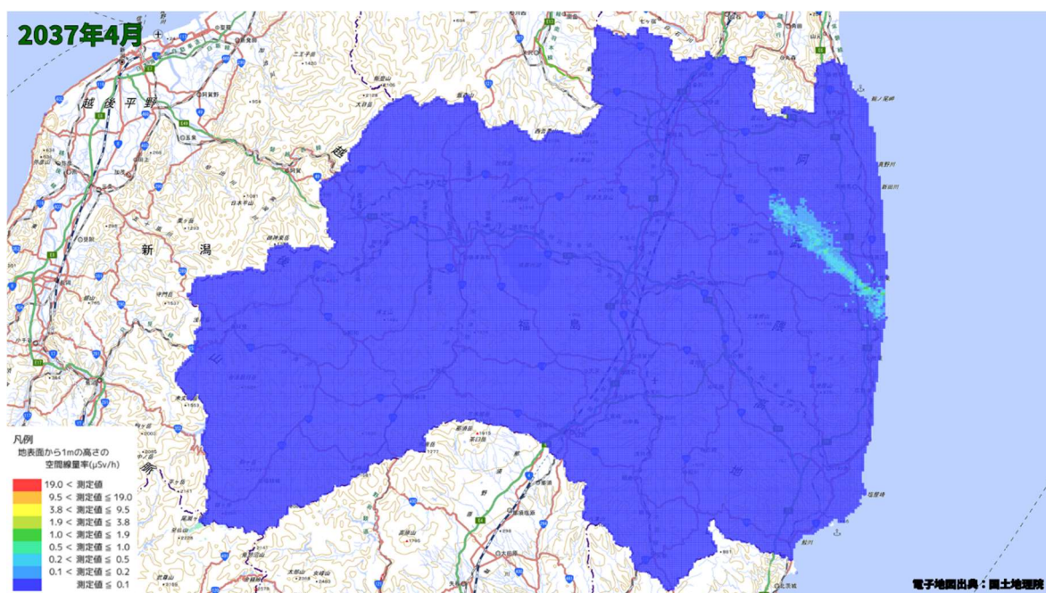
空間線量率分布将来予測解析結果(2037 年 4 月)
