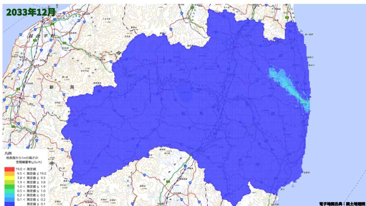
空間線量率分布将来予測解析結果(2033 年 12 月)
