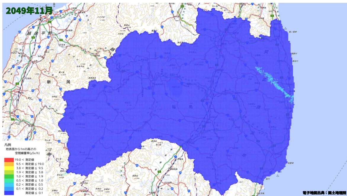
空間線量率分布将来予測解析結果(2049 年 11 月)
