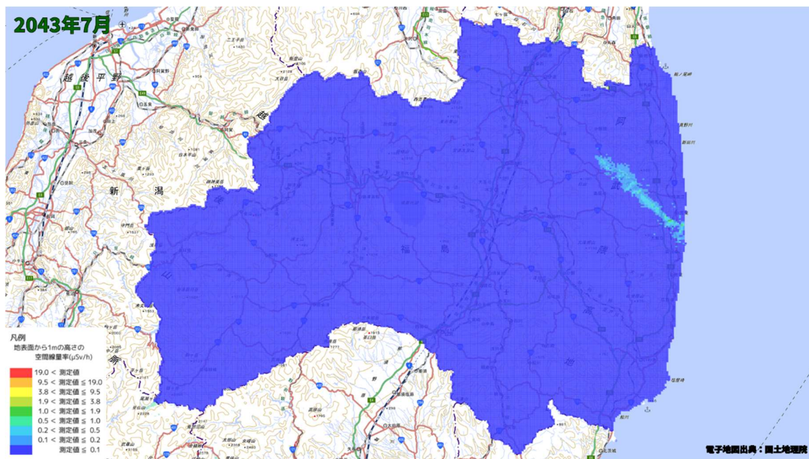
空間線量率分布将来予測解析結果(2043 年 7 月)
