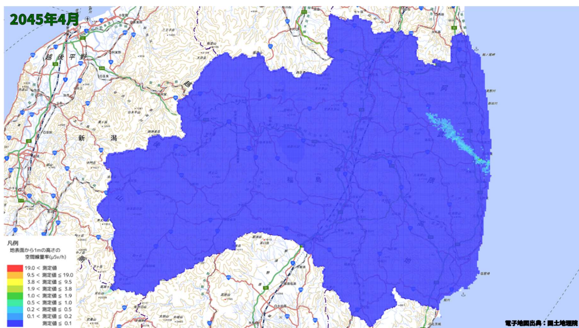
空間線量率分布将来予測解析結果(2045 年 4 月)
