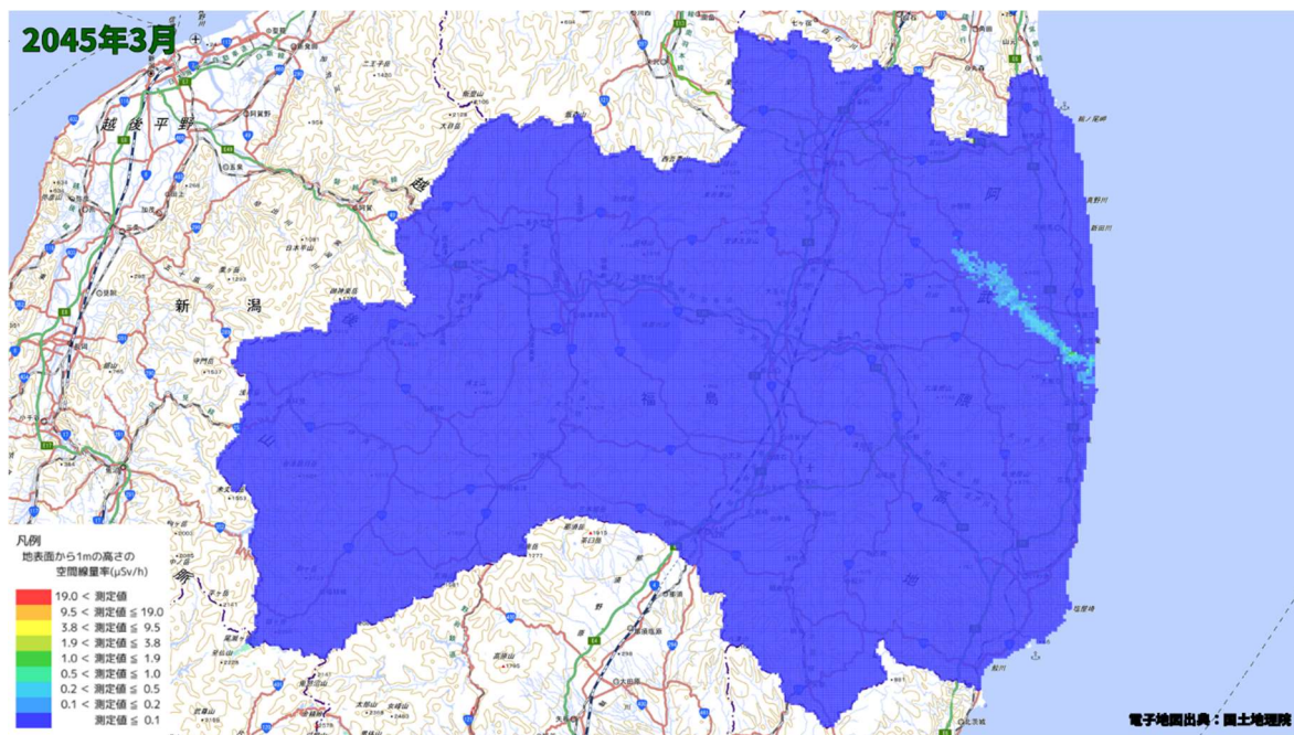
空間線量率分布将来予測解析結果(2045 年 3 月)
