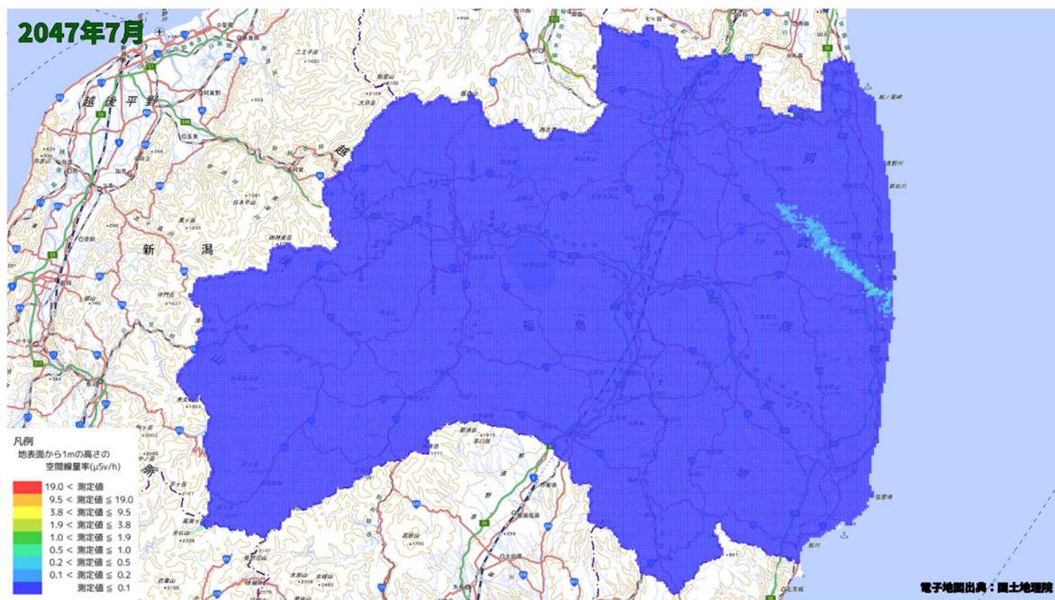
空間線量率分布将来予測解析結果(2047 年 7 月)
