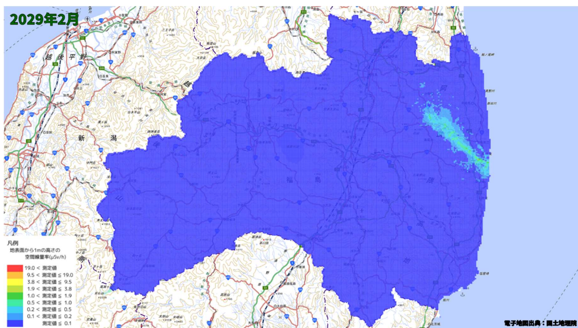
空間線量率分布将来予測解析結果(2029 年 2 月)
