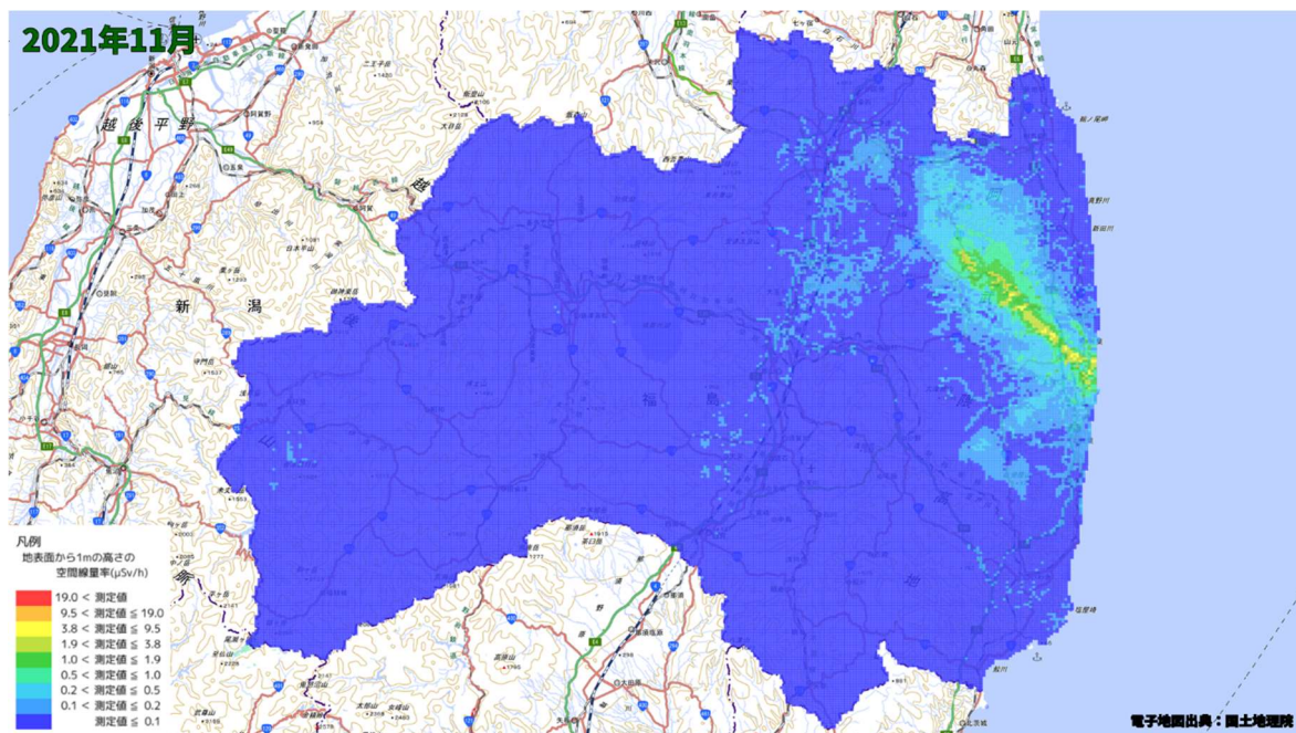
空間線量率分布将来予測解析結果(2021 年 11 月)
