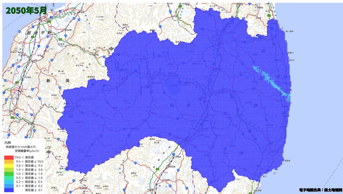
空間線量率分布将来予測解析結果(2050 年 5 月)
