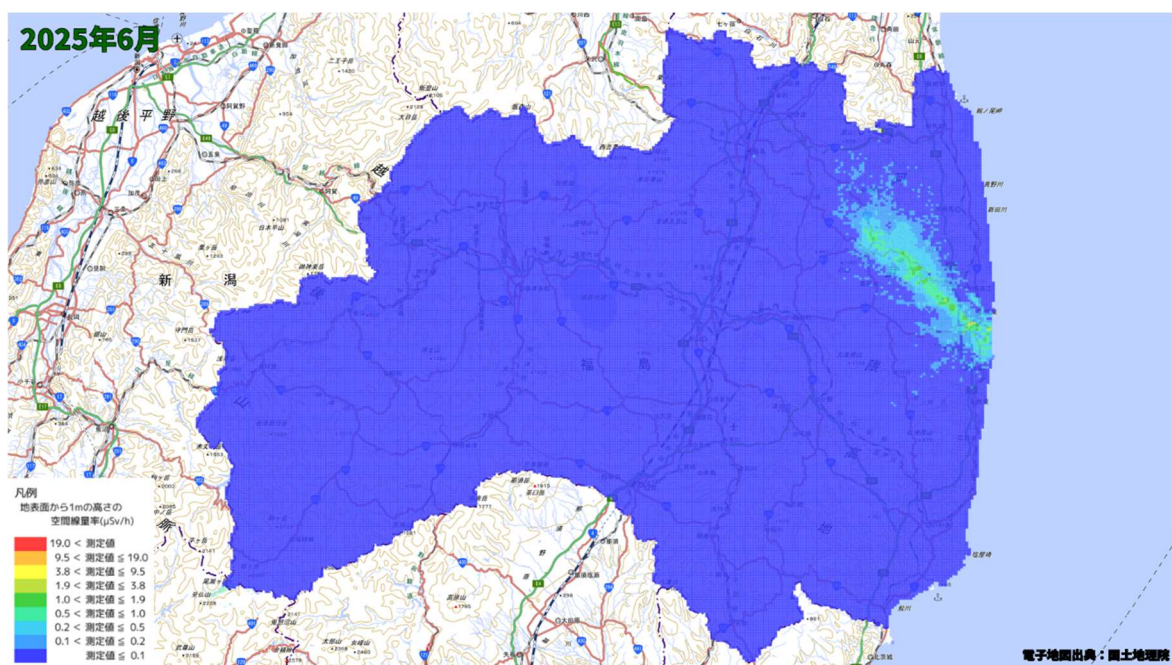
空間線量率分布将来予測解析結果(2025 年 6 月)
