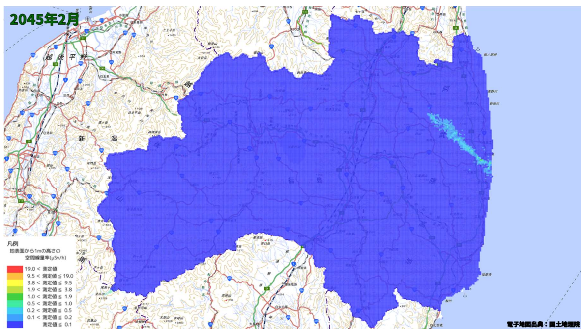
空間線量率分布将来予測解析結果(2045 年 2 月)
