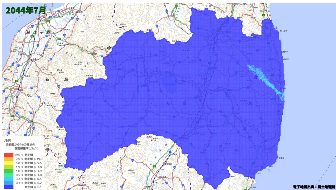
空間線量率分布将来予測解析結果(2044 年 7 月)
