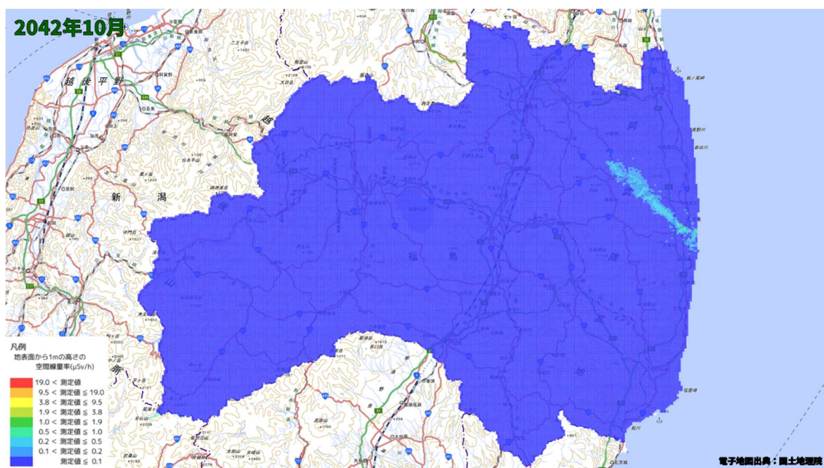
空間線量率分布将来予測解析結果(2042 年 10 月)
