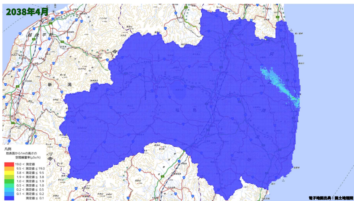
空間線量率分布将来予測解析結果(2038 年 4 月)
