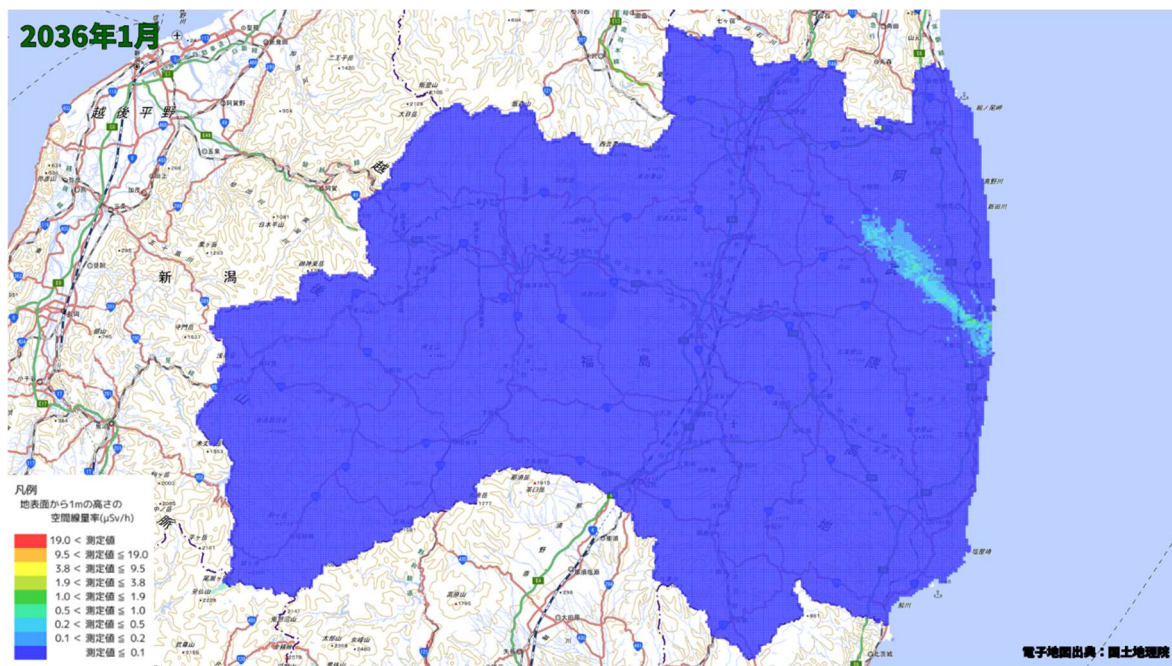
空間線量率分布将来予測解析結果(2036 年 1 月)
