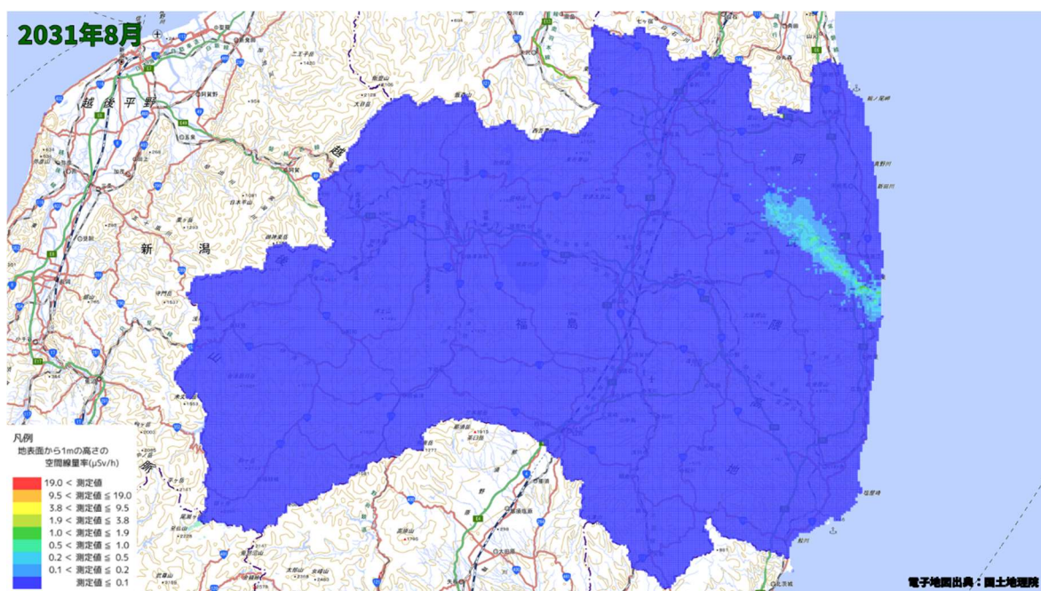
空間線量率分布将来予測解析結果(2031 年 8 月)
