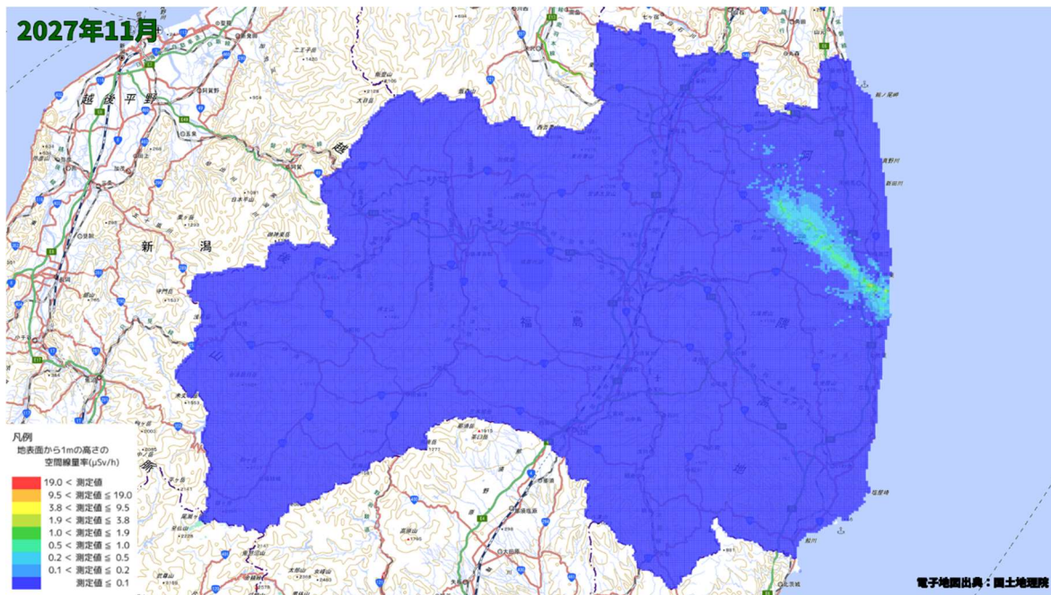
空間線量率分布将来予測解析結果(2027 年 11 月)
