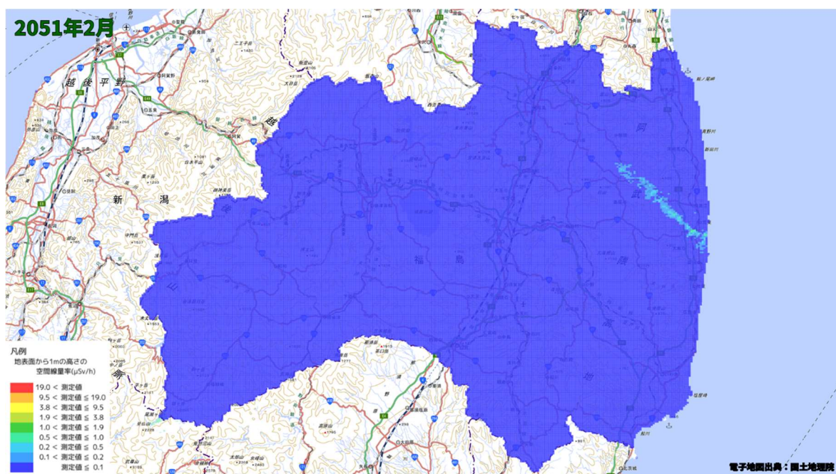
空間線量率分布将来予測解析結果(2051 年 2 月)
