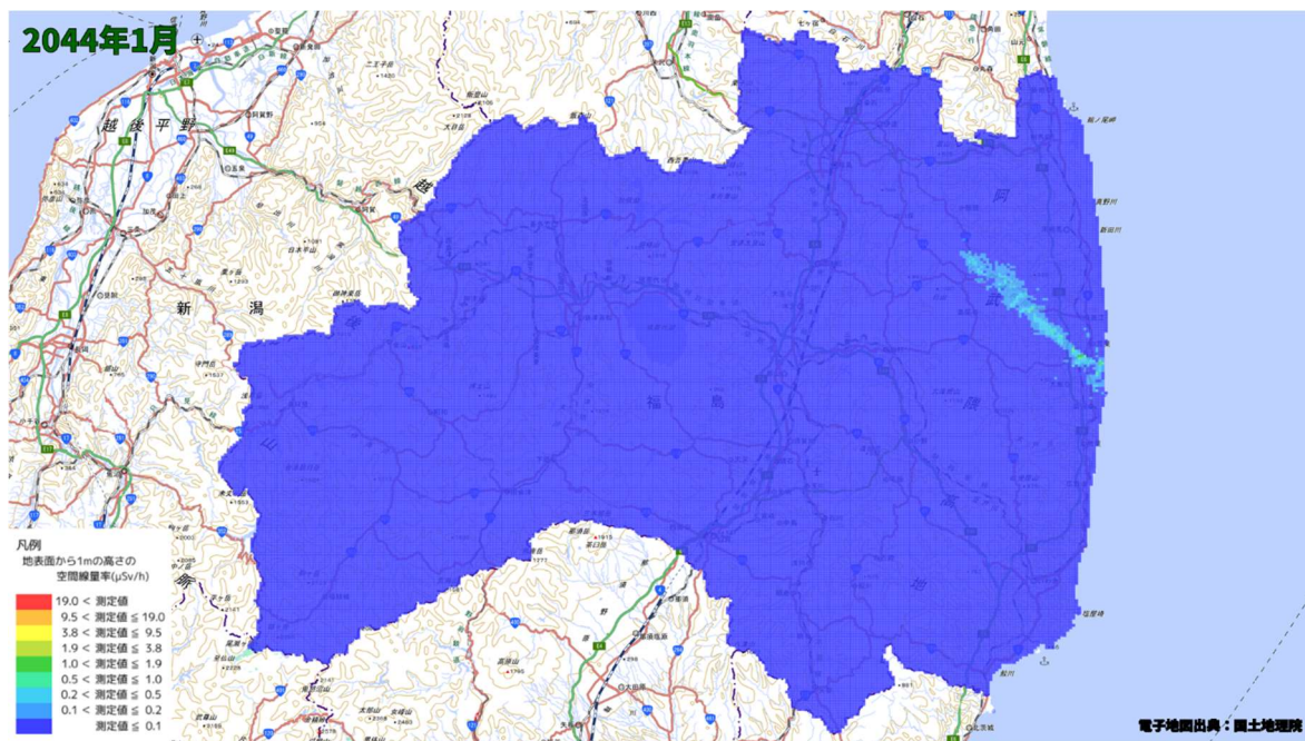
空間線量率分布将来予測解析結果(2044 年 1 月)
