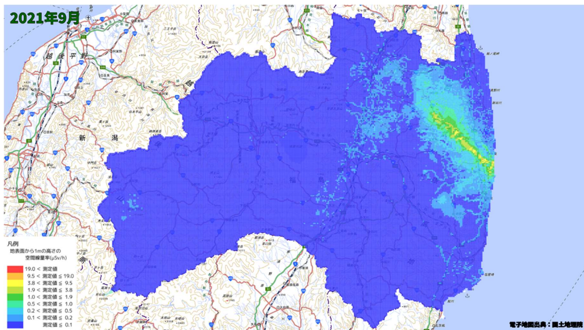
空間線量率分布将来予測解析結果(2021 年 9 月)
