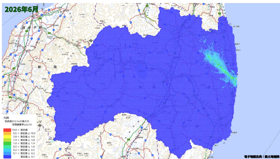
空間線量率分布将来予測解析結果(2026 年 6 月)
