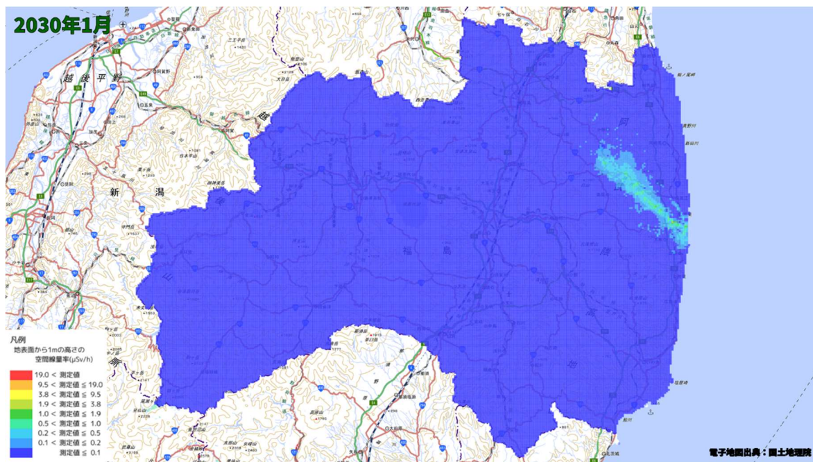
空間線量率分布将来予測解析結果(2030 年 1 月)
