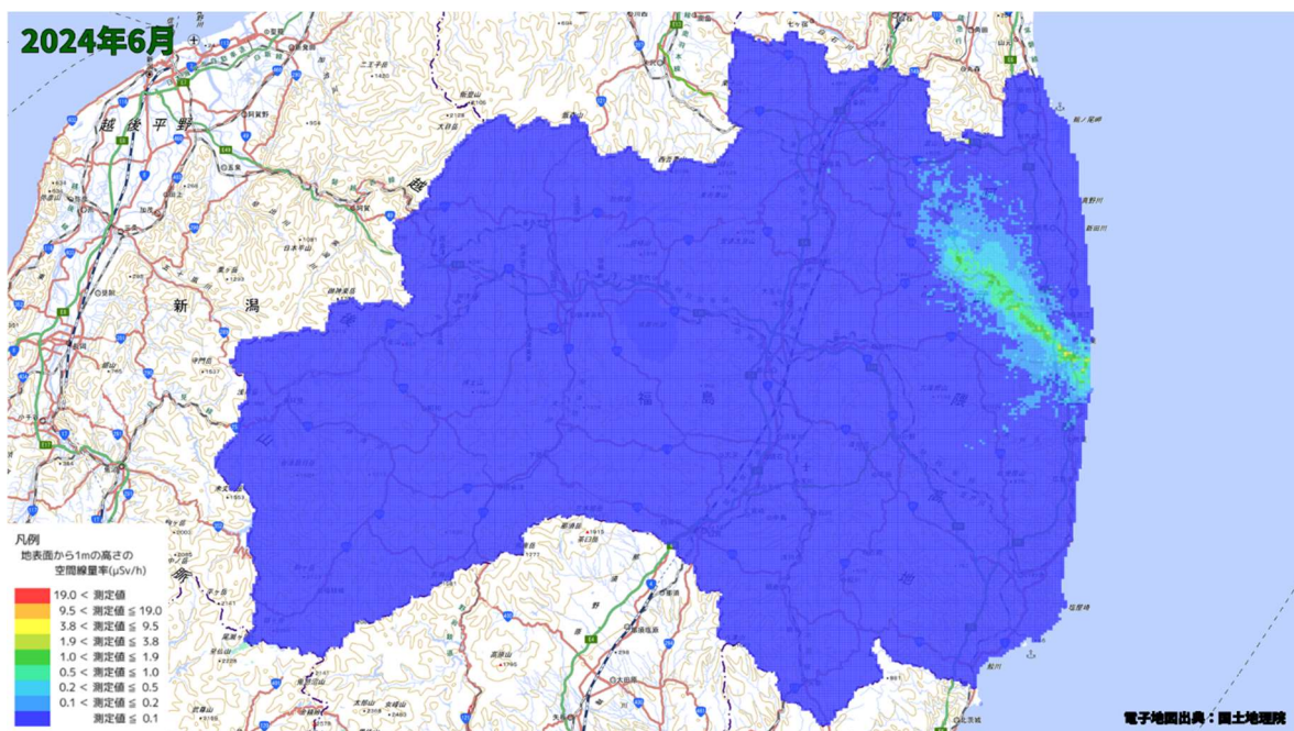
空間線量率分布将来予測解析結果(2024 年 6 月)
