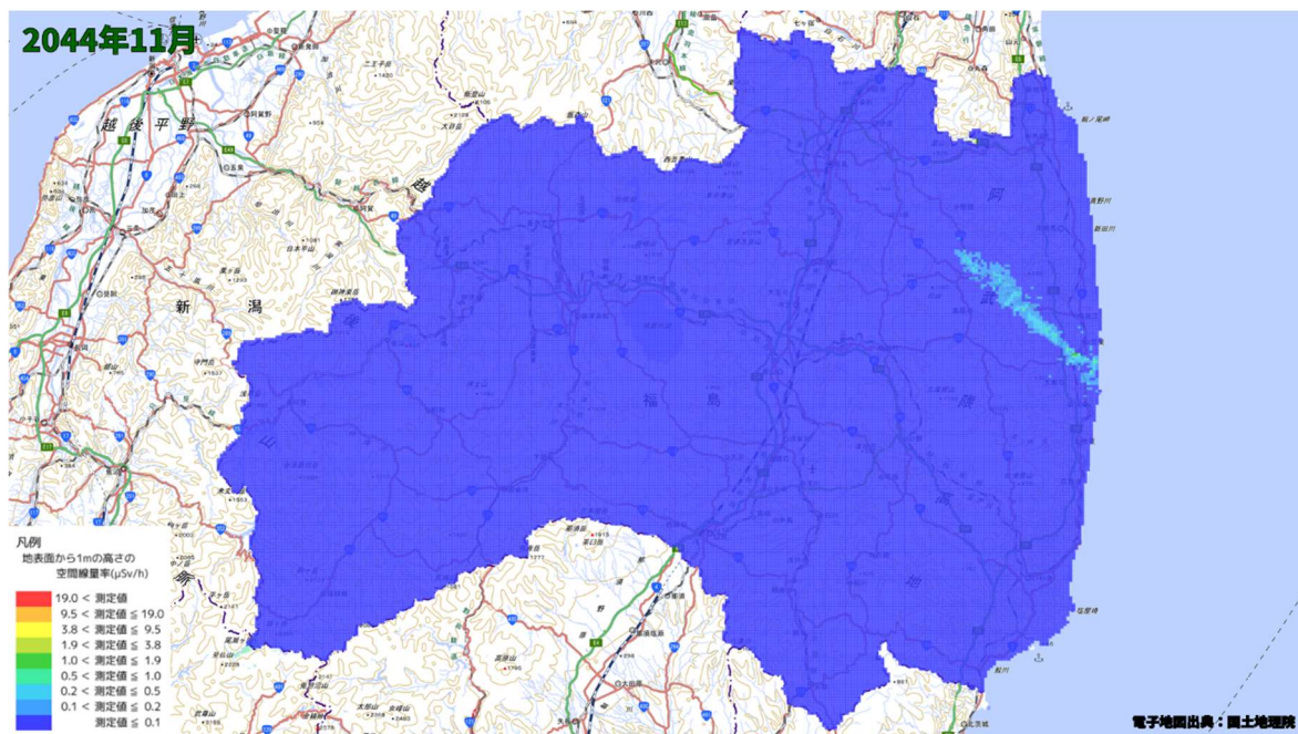
空間線量率分布将来予測解析結果(2044 年 11 月)
