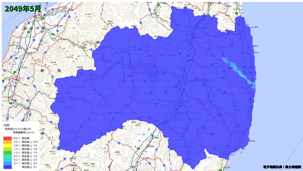
空間線量率分布将来予測解析結果(2049 年 5 月)
