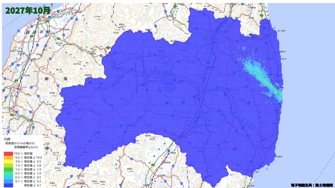
空間線量率分布将来予測解析結果(2027 年 10 月)
