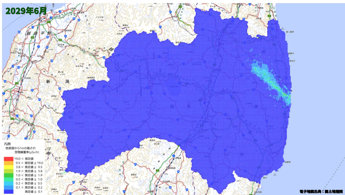
空間線量率分布将来予測解析結果(2029 年 6 月)
