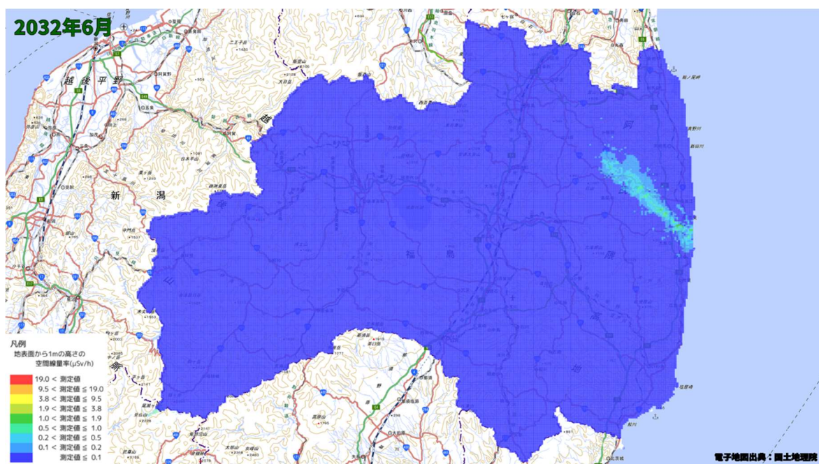
空間線量率分布将来予測解析結果(2032 年 6 月)
