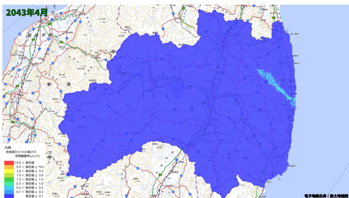
空間線量率分布将来予測解析結果(2043 年 4 月)
