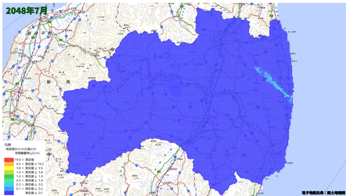
空間線量率分布将来予測解析結果(2048 年 7 月)
