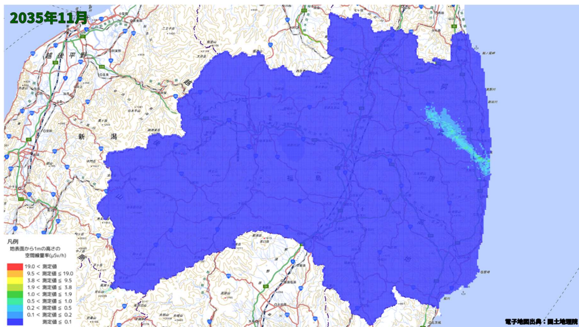
空間線量率分布将来予測解析結果(2035 年 11 月)
