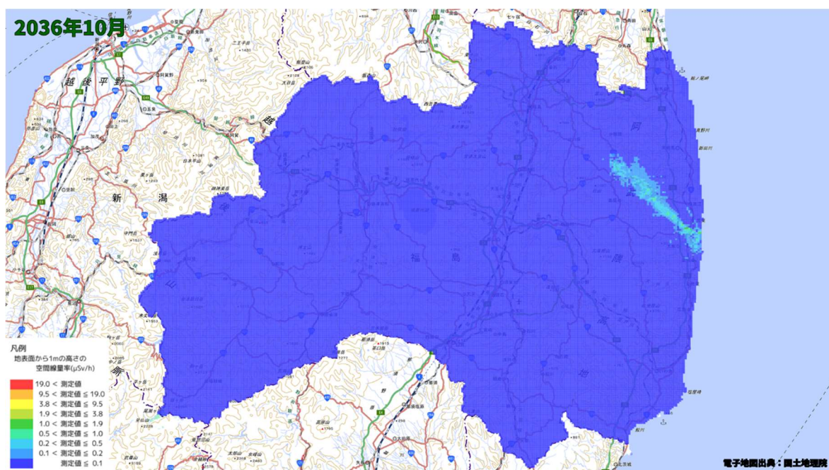
空間線量率分布将来予測解析結果(2036 年 10 月)
