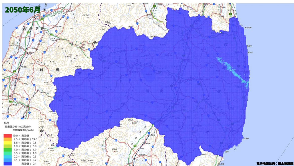
空間線量率分布将来予測解析結果(2050 年 6 月)
