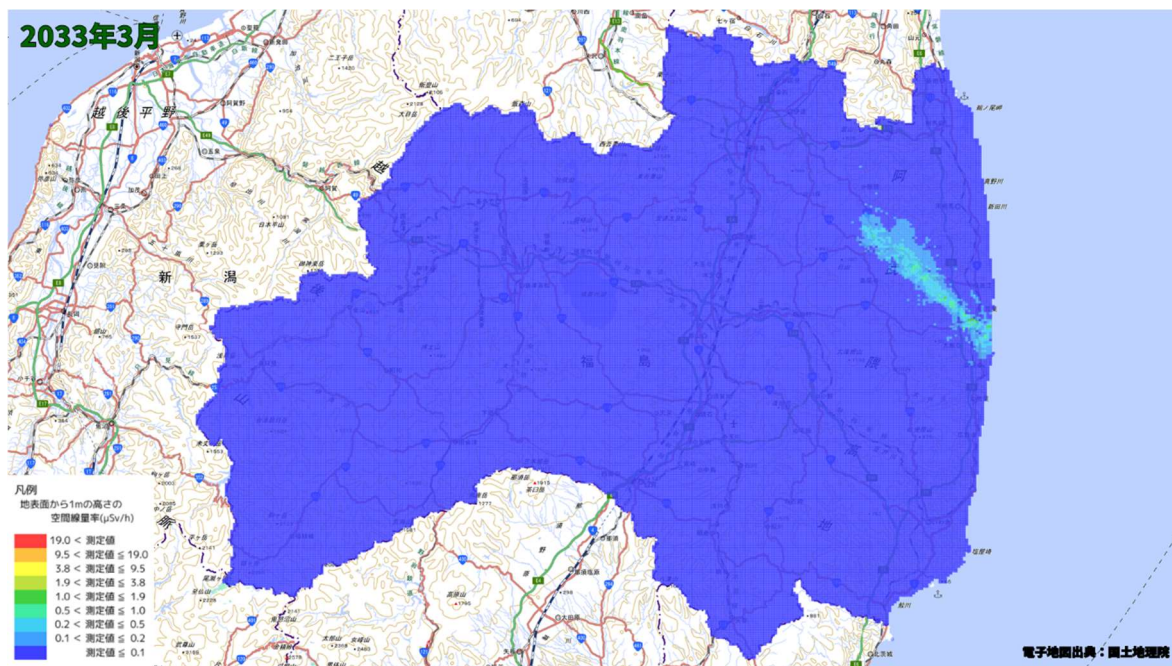
空間線量率分布将来予測解析結果(2033 年 3 月)
