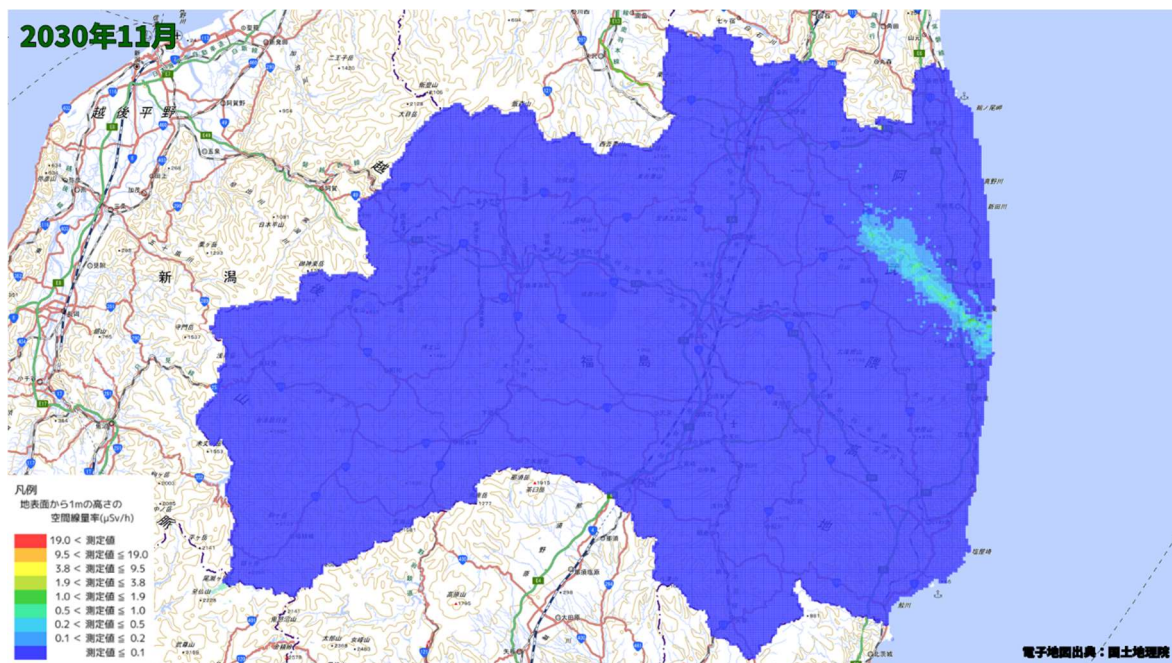
空間線量率分布将来予測解析結果(2030 年 11 月)
