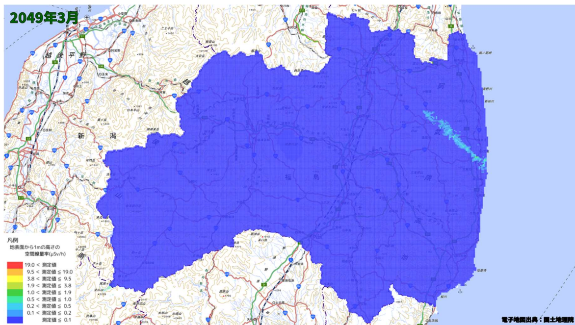
空間線量率分布将来予測解析結果(2049 年 3 月)
