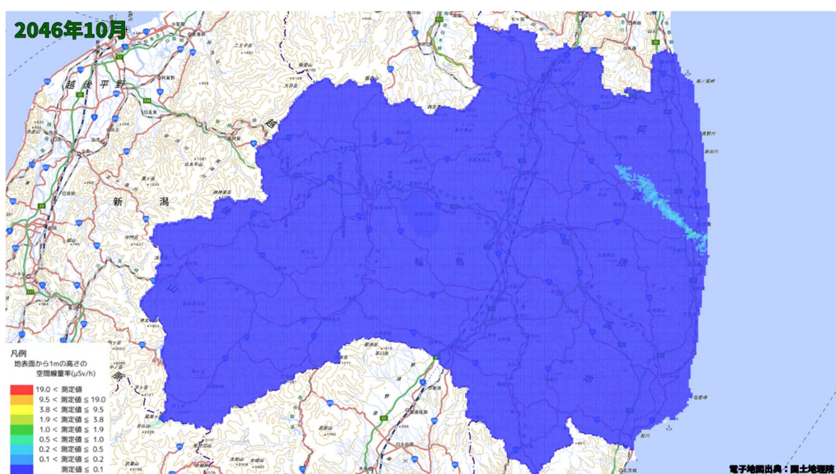
空間線量率分布将来予測解析結果(2046 年 10 月)
