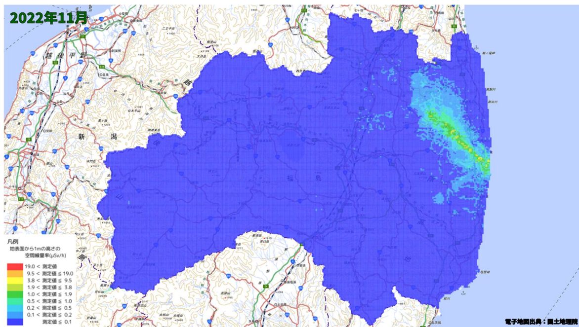
空間線量率分布将来予測解析結果(2022 年 11 月)
