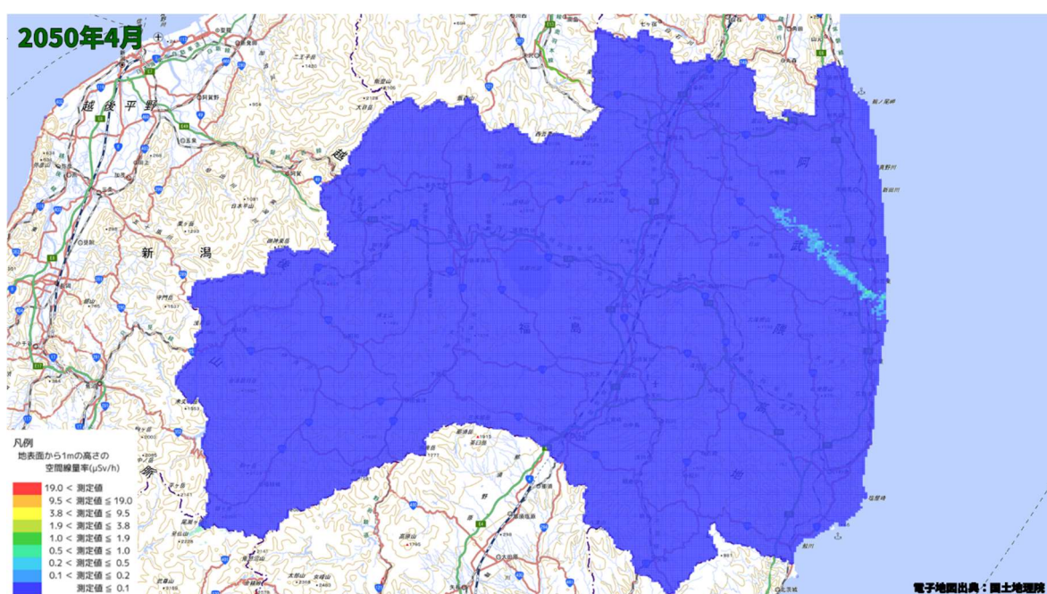
空間線量率分布将来予測解析結果(2050 年 4 月)
