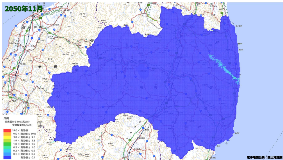
空間線量率分布将来予測解析結果(2050 年 11 月)
