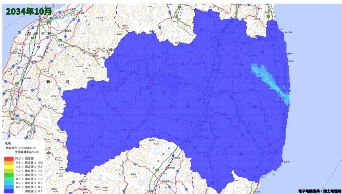
空間線量率分布将来予測解析結果(2034 年 10 月)
