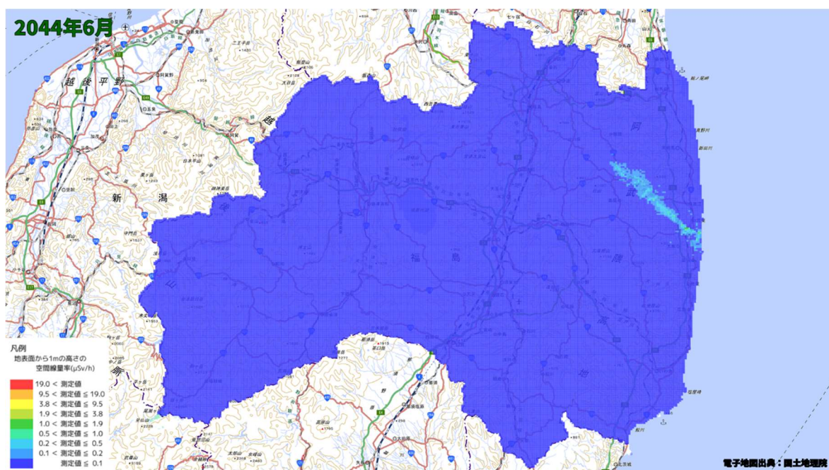
空間線量率分布将来予測解析結果(2044 年 6 月)
