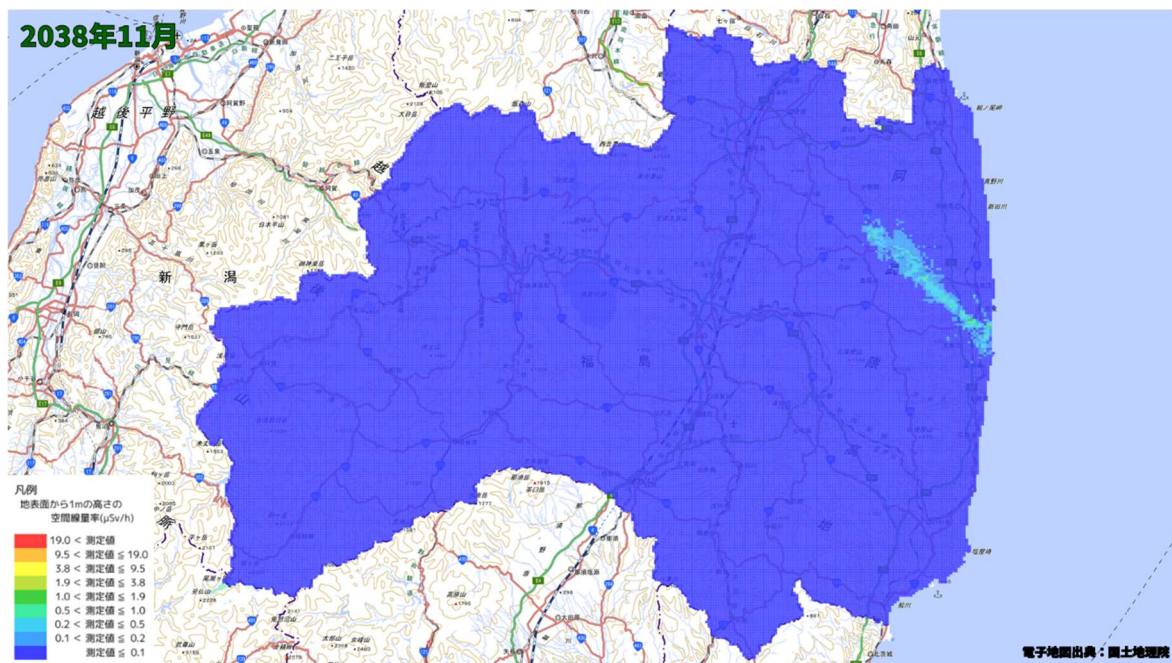
空間線量率分布将来予測解析結果(2038 年 11 月)
