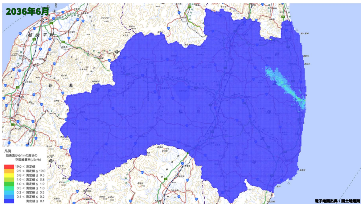
空間線量率分布将来予測解析結果(2036 年 6 月)
