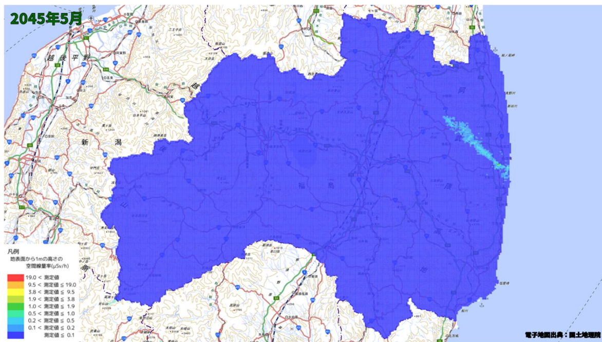
空間線量率分布将来予測解析結果(2045 年 5 月)
