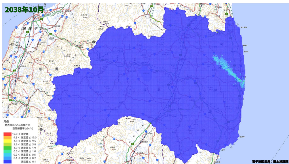
空間線量率分布将来予測解析結果(2038 年 10 月)
