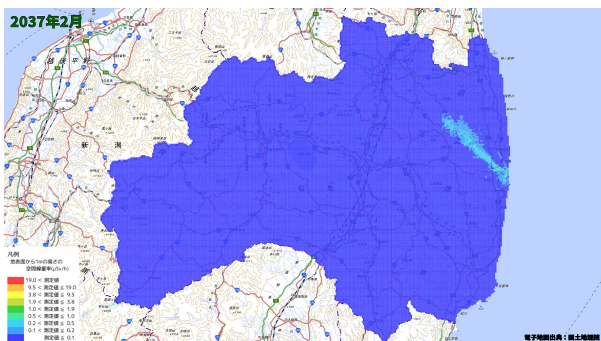
空間線量率分布将来予測解析結果(2037 年 2 月)
