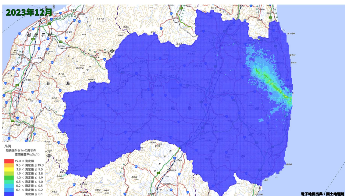
空間線量率分布将来予測解析結果(2023 年 12 月)
