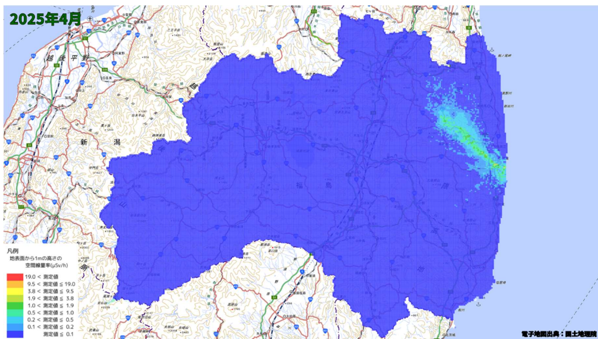
空間線量率分布将来予測解析結果(2025 年 4 月)
