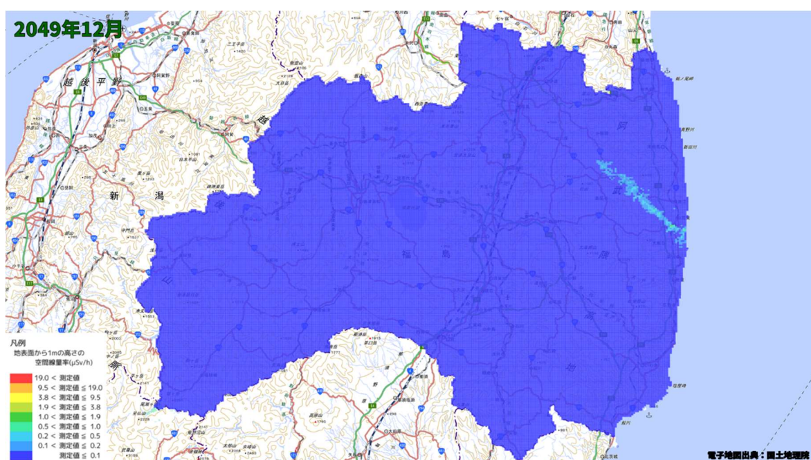
空間線量率分布将来予測解析結果(2049 年 12 月)
