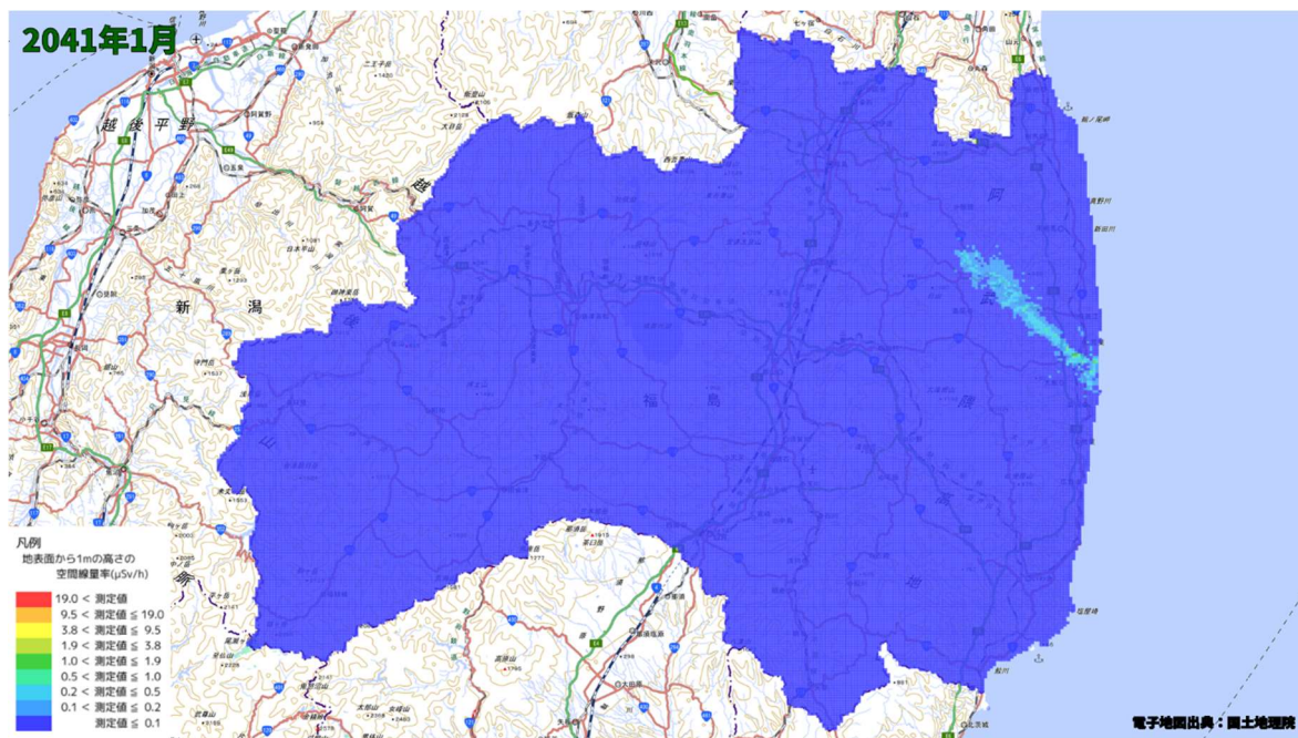
空間線量率分布将来予測解析結果(2041 年 1 月)
