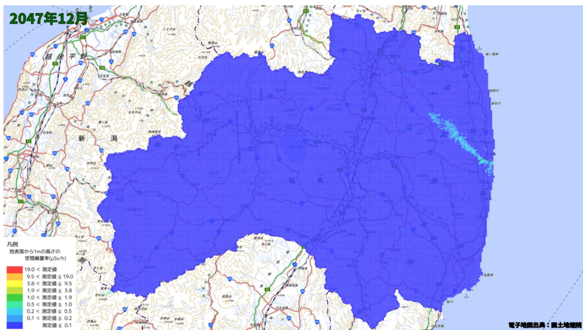
空間線量率分布将来予測解析結果(2047 年 12 月)
