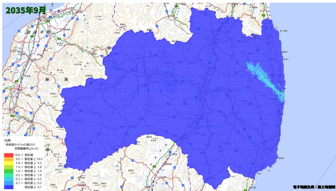
空間線量率分布将来予測解析結果(2035 年 9 月)
