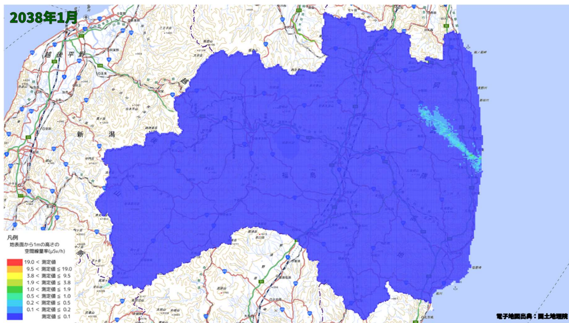
空間線量率分布将来予測解析結果(2038 年 1 月)
