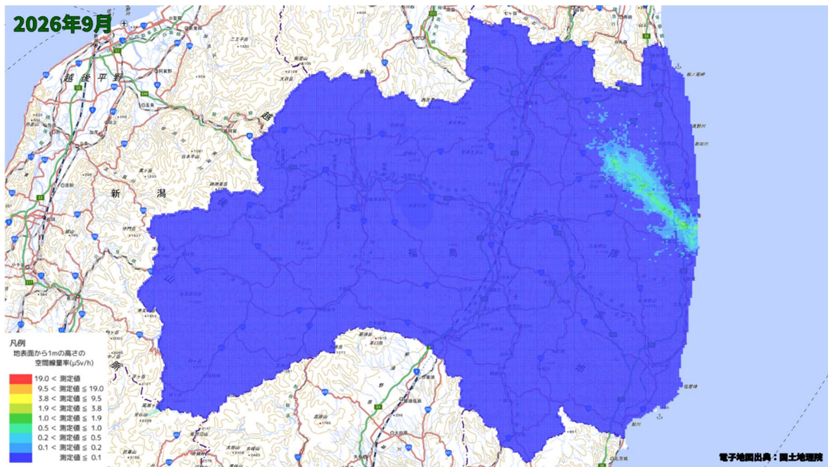
空間線量率分布将来予測解析結果(2026 年 9 月)
