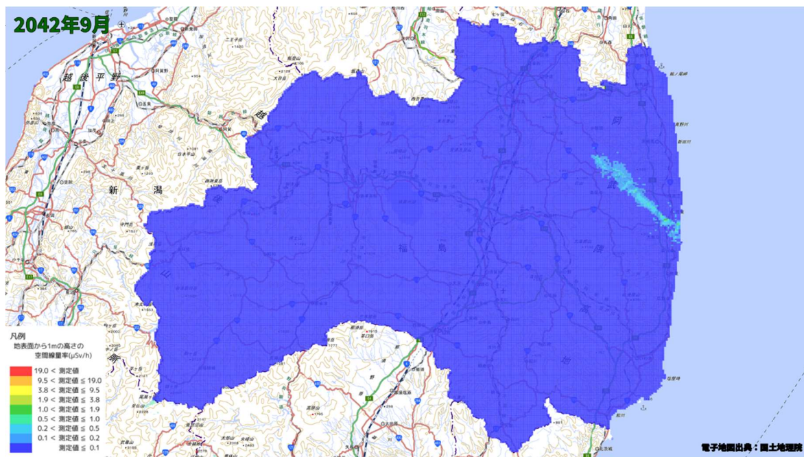
空間線量率分布将来予測解析結果(2042 年 9 月)
