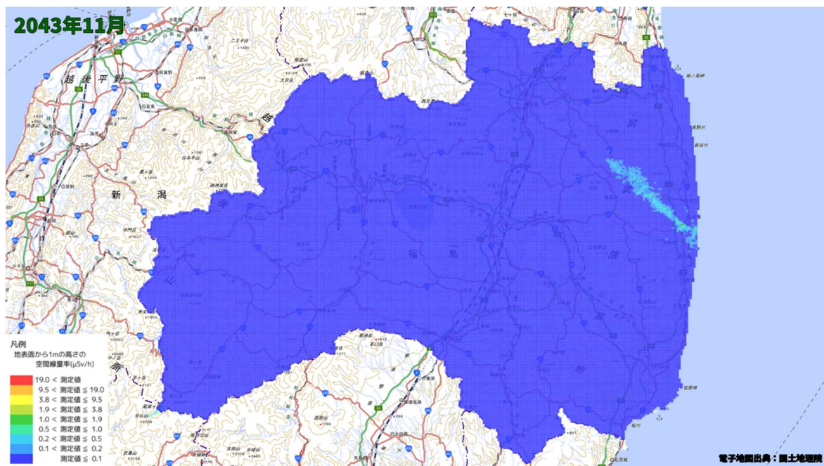
空間線量率分布将来予測解析結果(2043 年 11 月)
