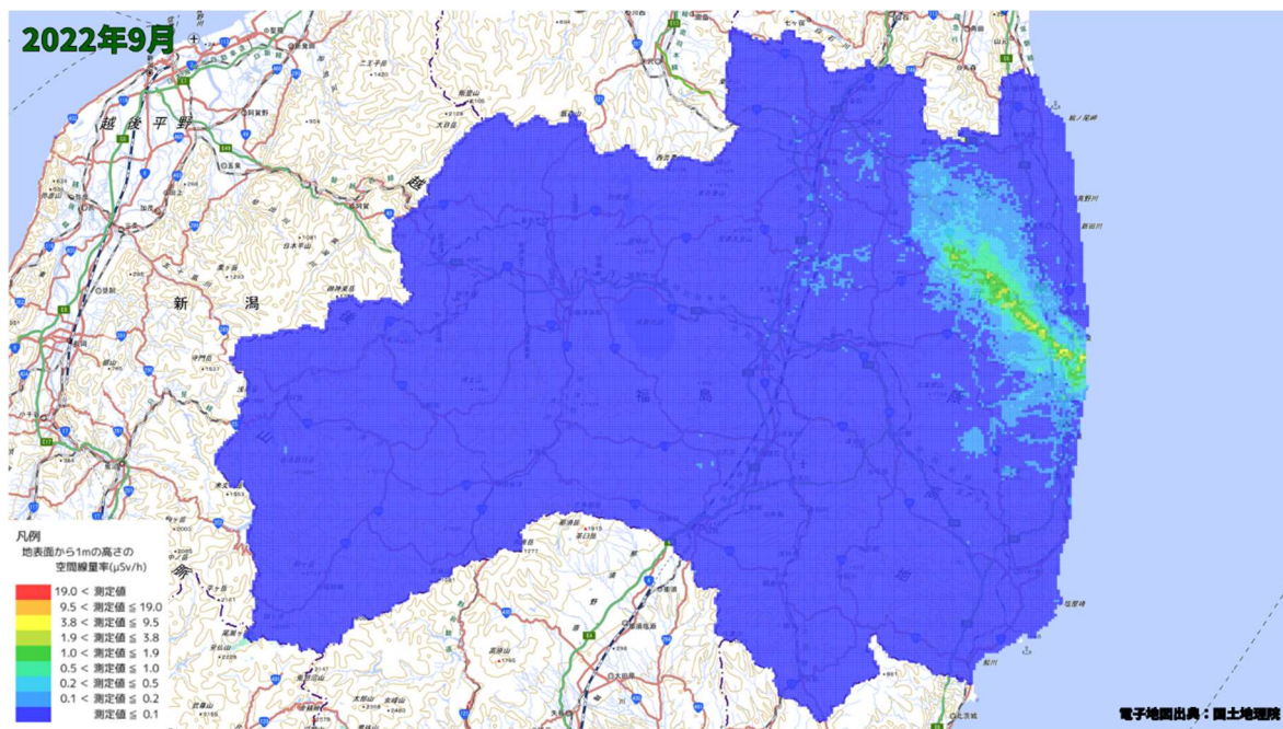
空間線量率分布将来予測解析結果(2022 年 9 月)
