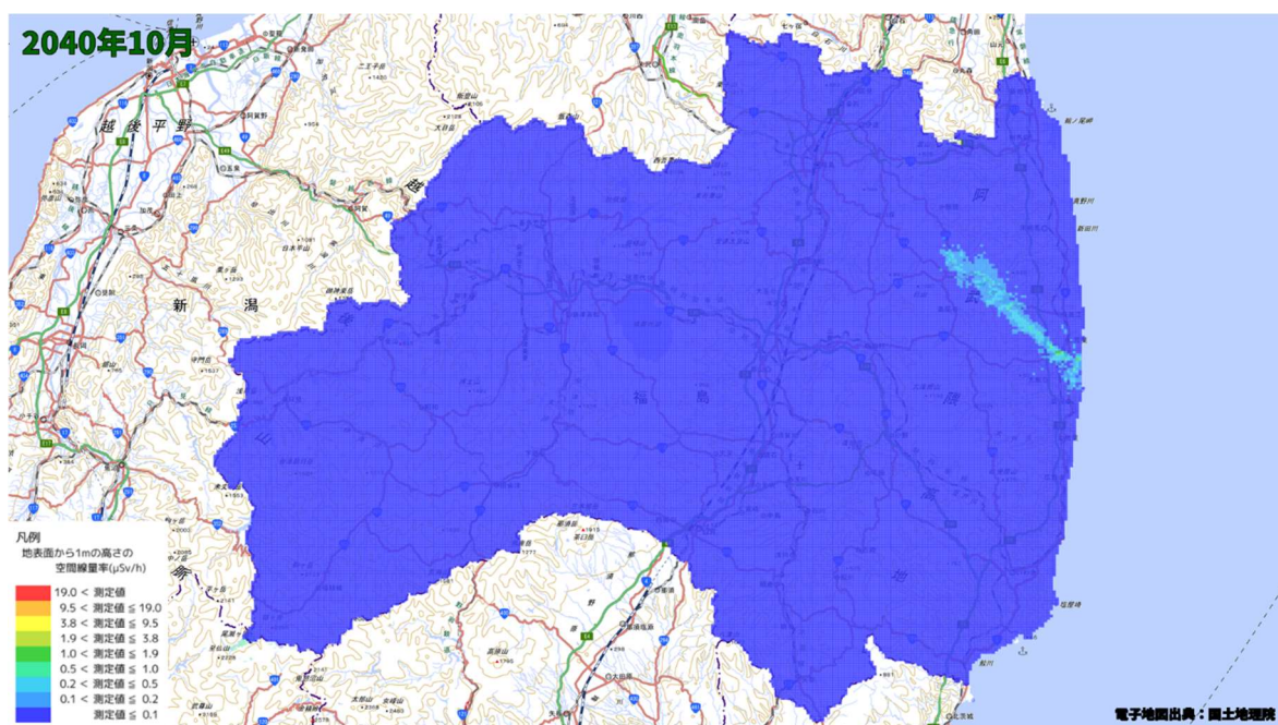
空間線量率分布将来予測解析結果(2040 年 10 月)
