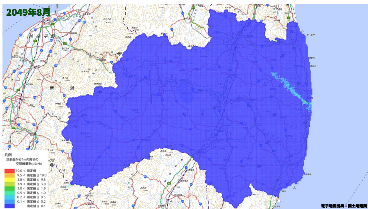
空間線量率分布将来予測解析結果(2049 年 8 月)
