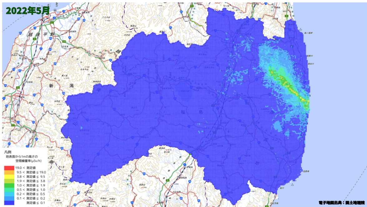
空間線量率分布将来予測解析結果(2022 年 5 月)
