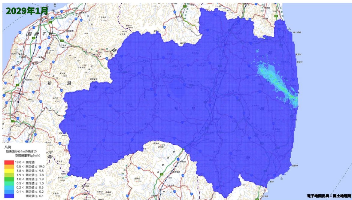
空間線量率分布将来予測解析結果(2029 年 1 月)
