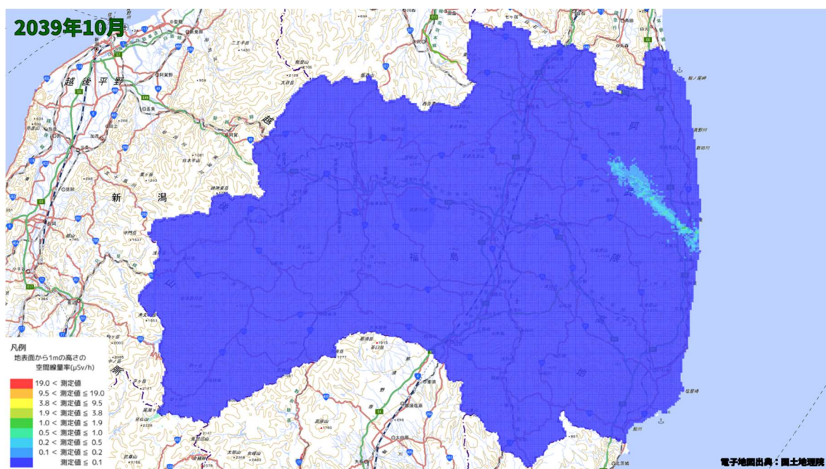
空間線量率分布将来予測解析結果(2039 年 10 月)
