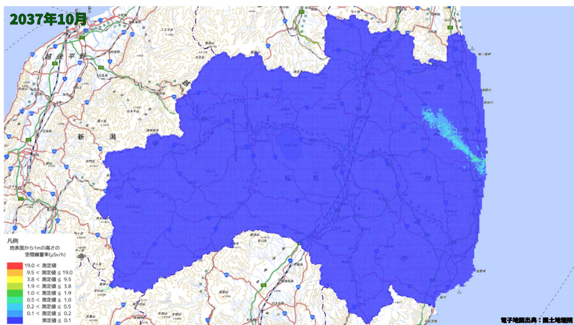
空間線量率分布将来予測解析結果(2037 年 10 月)
