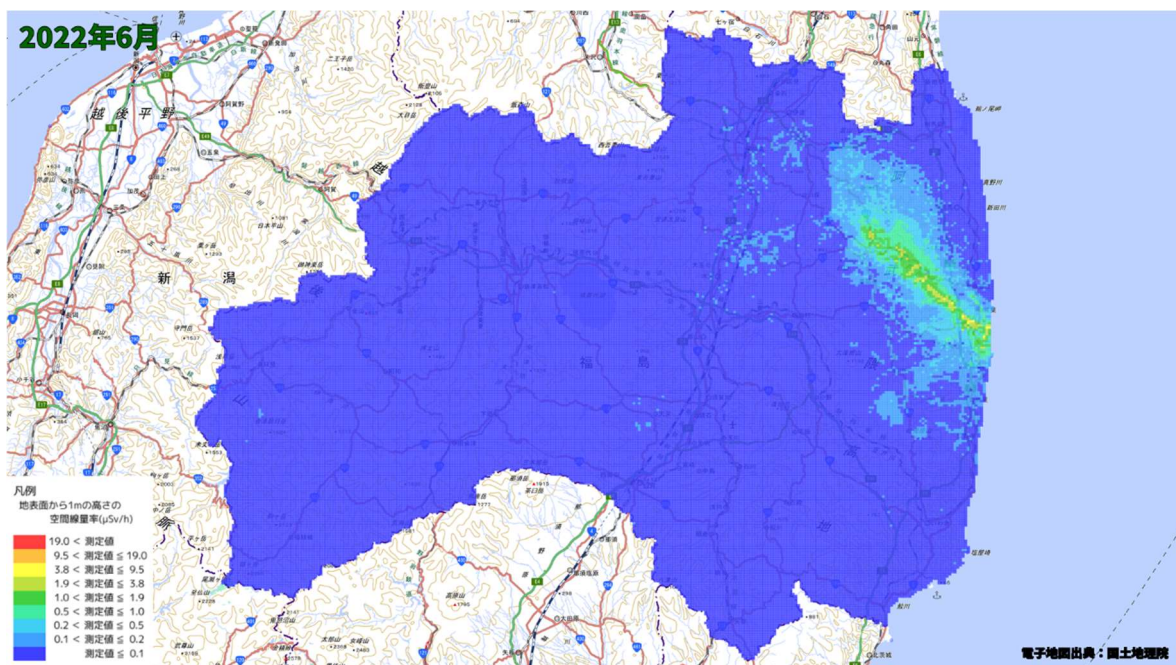
空間線量率分布将来予測解析結果(2022 年 6 月)
