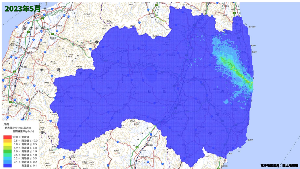
空間線量率分布将来予測解析結果(2023 年 5 月)
