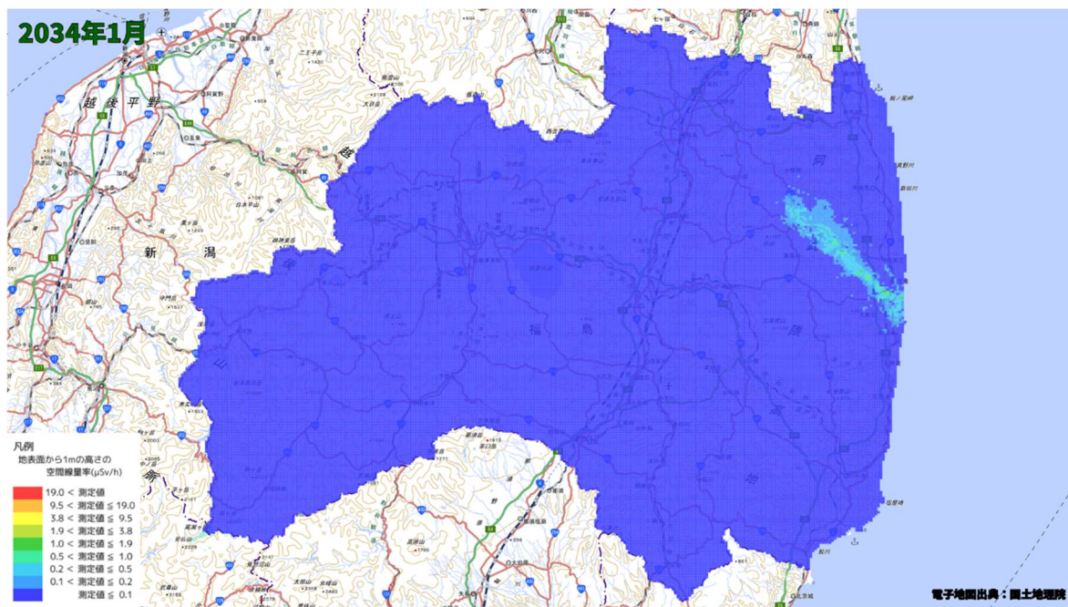
空間線量率分布将来予測解析結果(2034 年 1 月)
