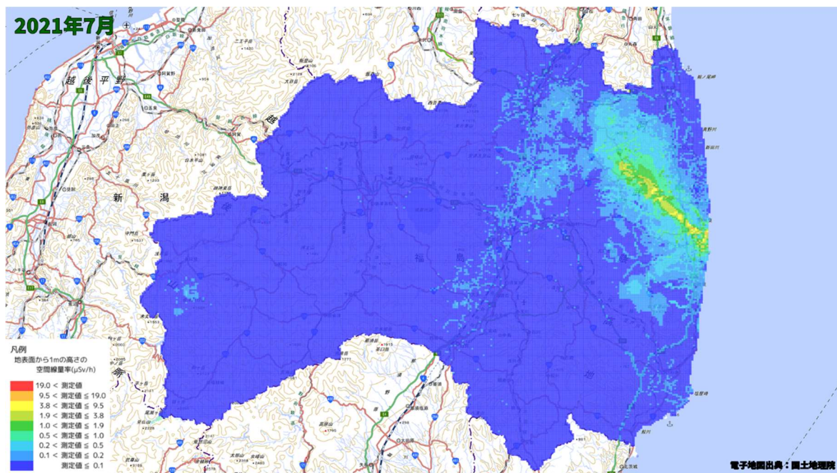
空間線量率分布将来予測解析結果(2021 年 7 月)
