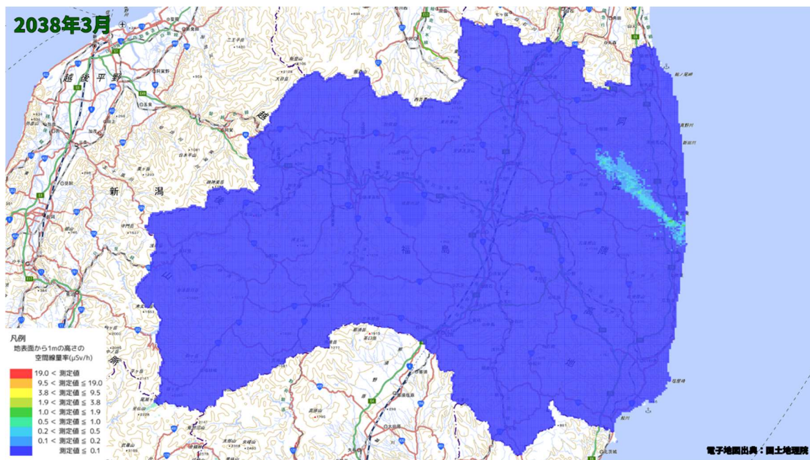
空間線量率分布将来予測解析結果(2038 年 3 月)
