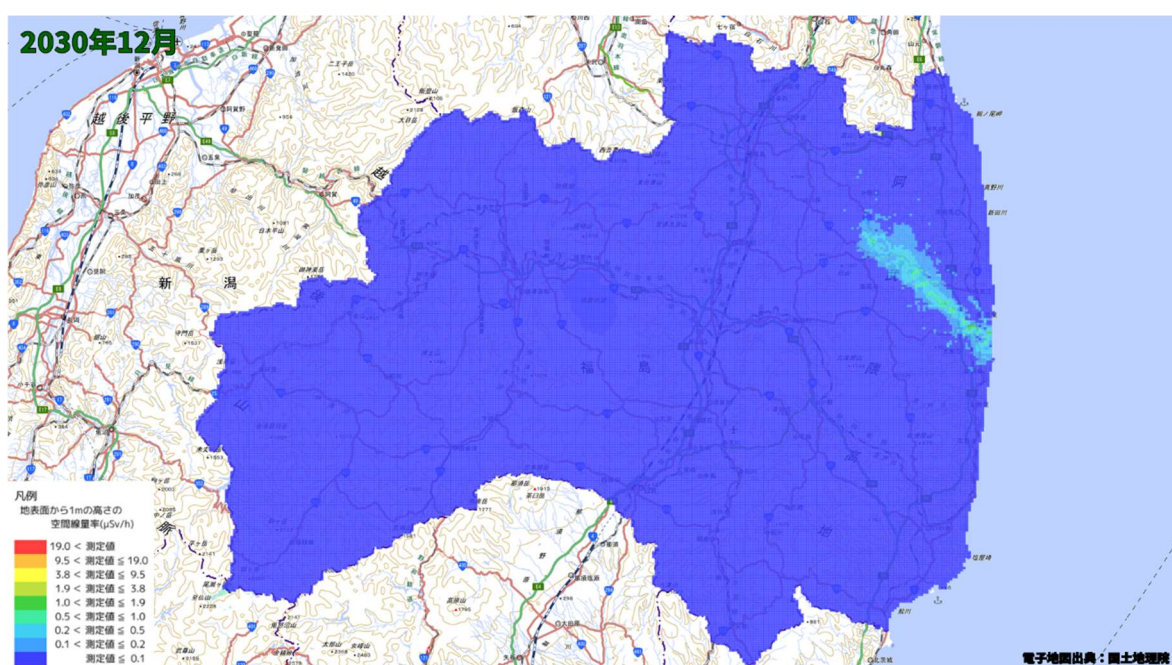
空間線量率分布将来予測解析結果(2030 年 12 月)
