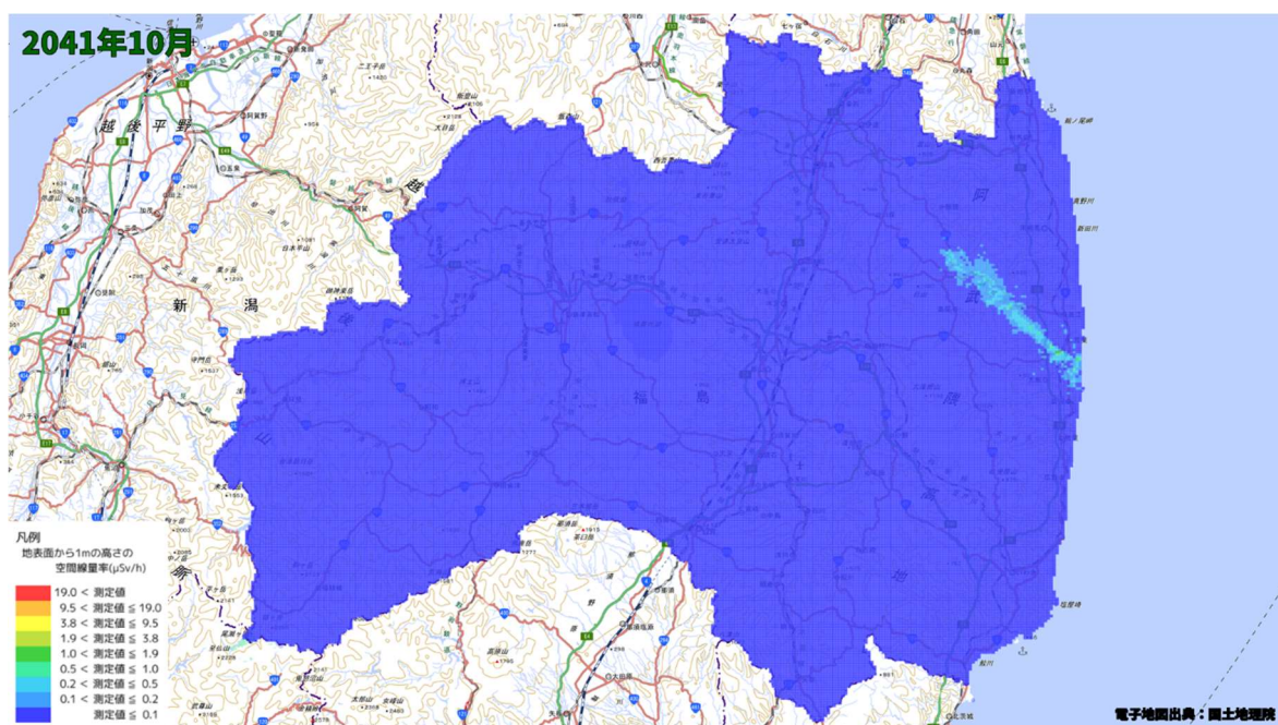
空間線量率分布将来予測解析結果(2041 年 10 月)
