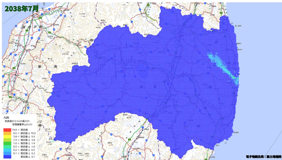
空間線量率分布将来予測解析結果(2038 年 7 月)
