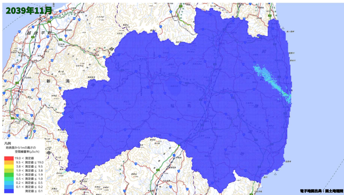
空間線量率分布将来予測解析結果(2039 年 11 月)
