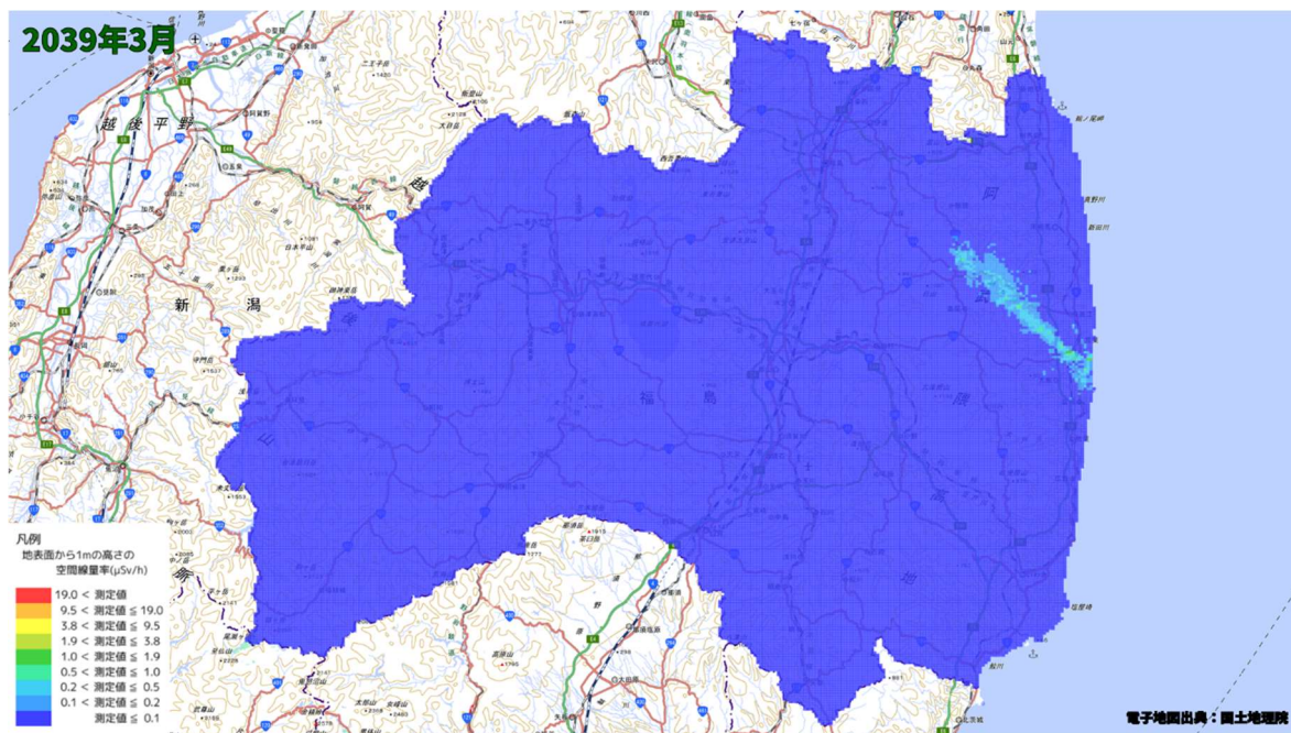
空間線量率分布将来予測解析結果(2039 年 3 月)
