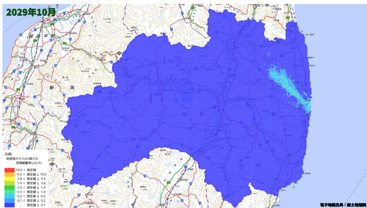
空間線量率分布将来予測解析結果(2029 年 10 月)
