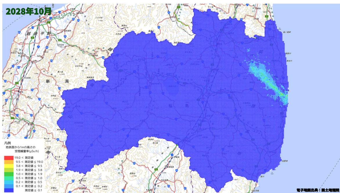
空間線量率分布将来予測解析結果(2028 年 10 月)
