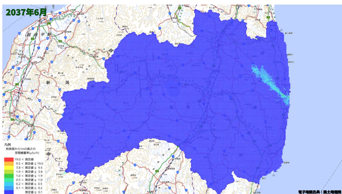
空間線量率分布将来予測解析結果(2037 年 6 月)
