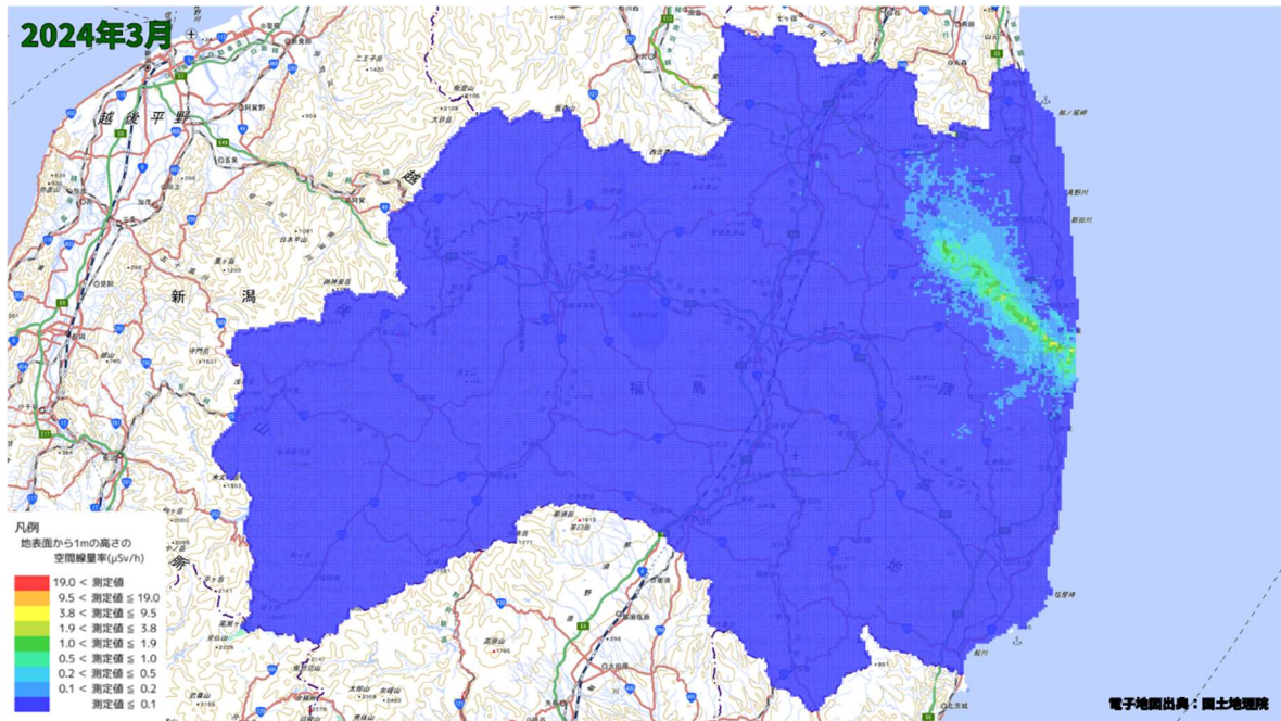
空間線量率分布将来予測解析結果(2024 年 3 月)
