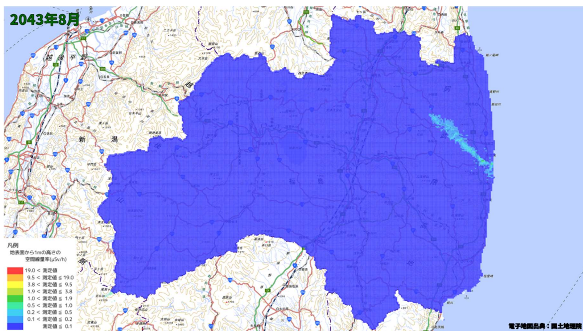
空間線量率分布将来予測解析結果(2043 年 8 月)
