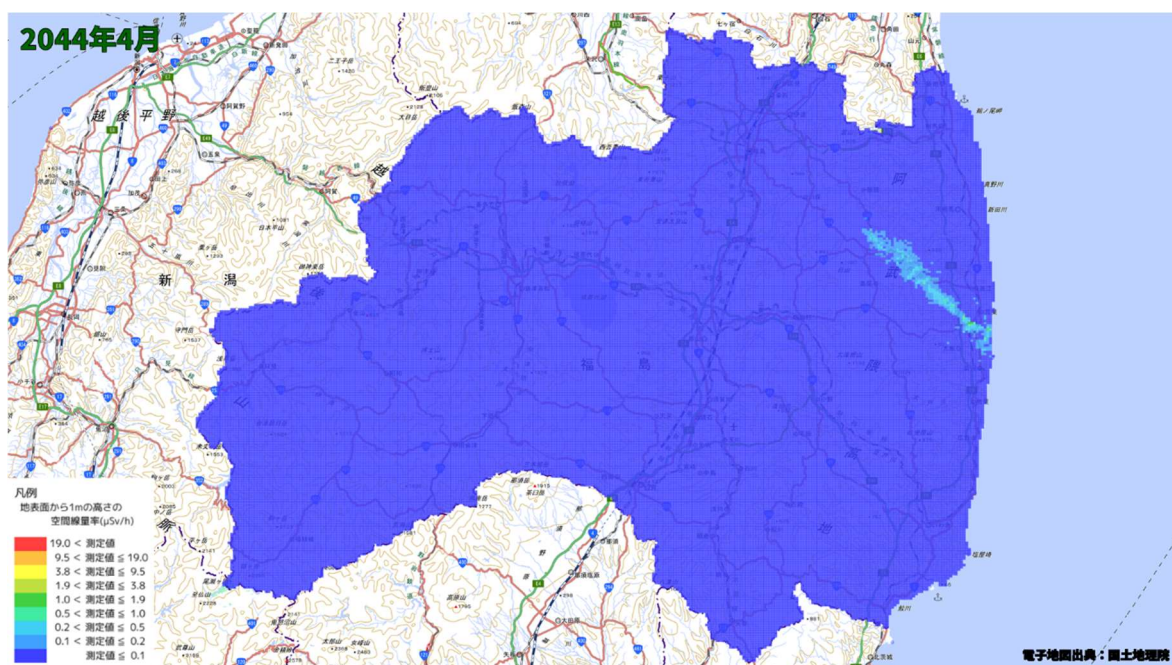
空間線量率分布将来予測解析結果(2044 年 4 月)
