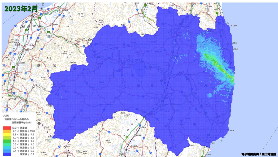
空間線量率分布将来予測解析結果(2023 年 2 月)
