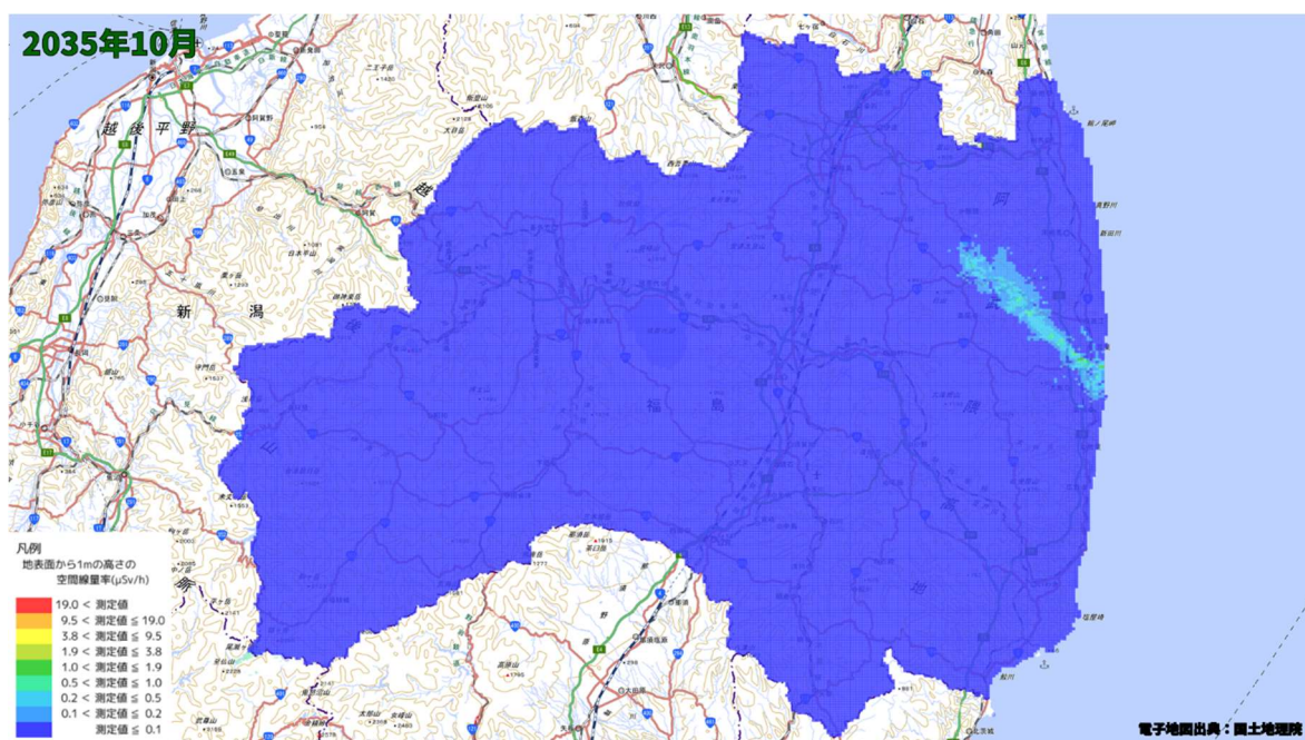
空間線量率分布将来予測解析結果(2035 年 10 月)
