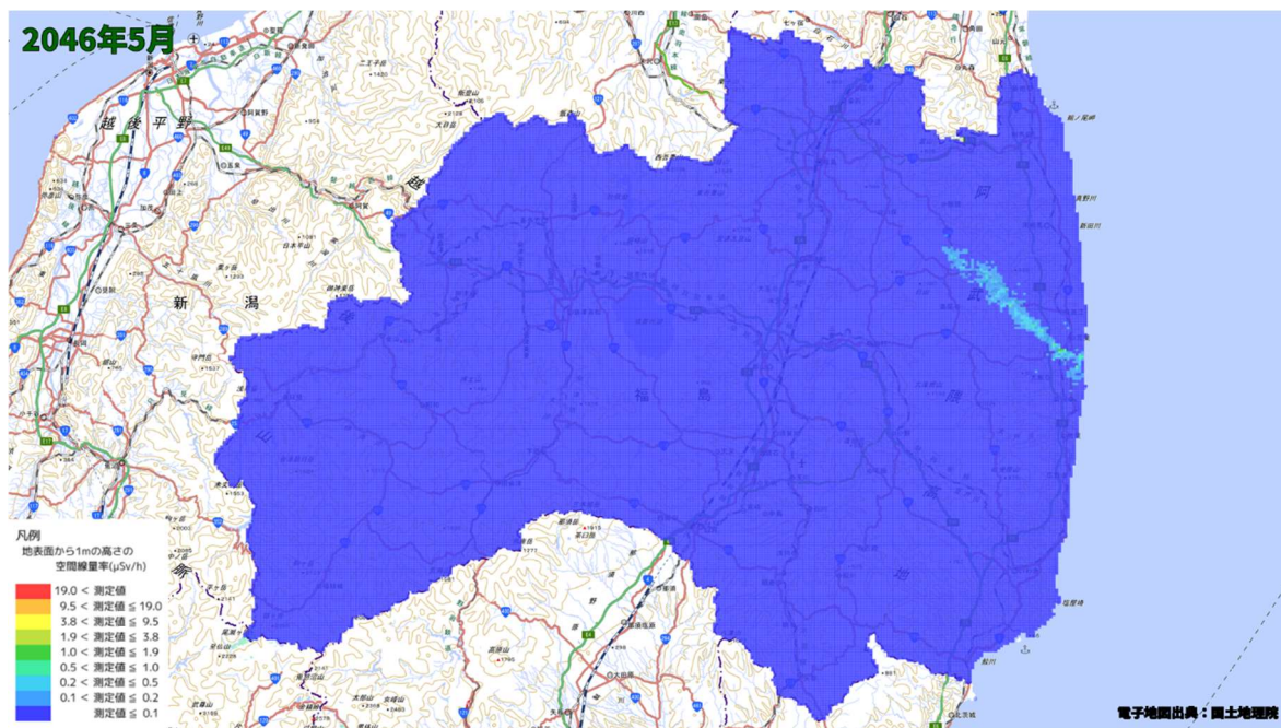
空間線量率分布将来予測解析結果(2046 年 5 月)
