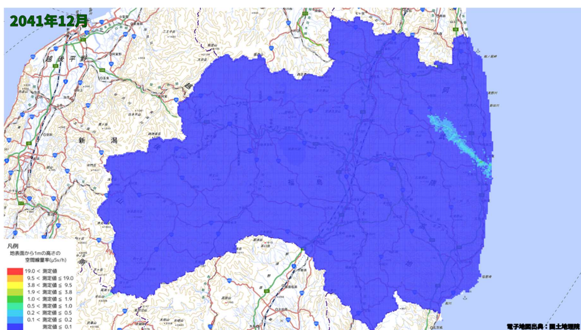
空間線量率分布将来予測解析結果(2041 年 12 月)
