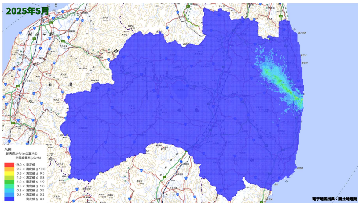
空間線量率分布将来予測解析結果(2025 年 5 月)
