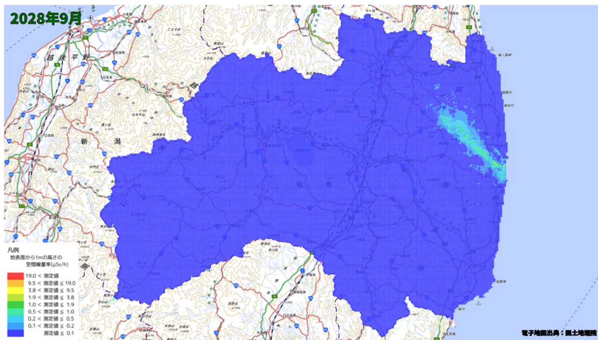
空間線量率分布将来予測解析結果(2028 年 9 月)
