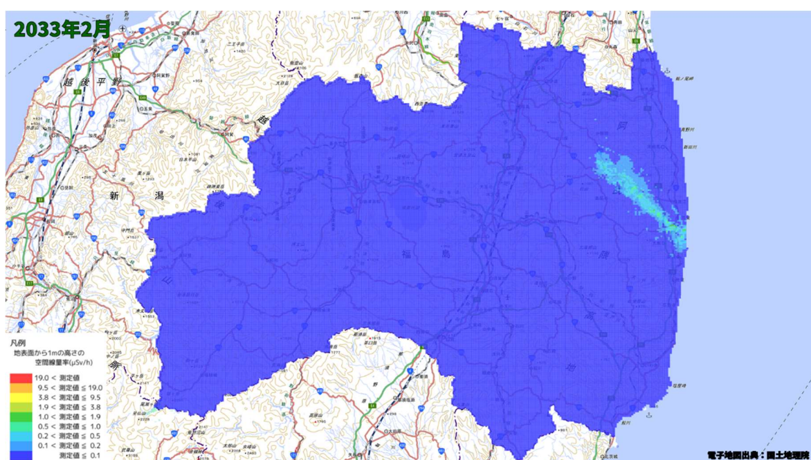
空間線量率分布将来予測解析結果(2033 年 2 月)
