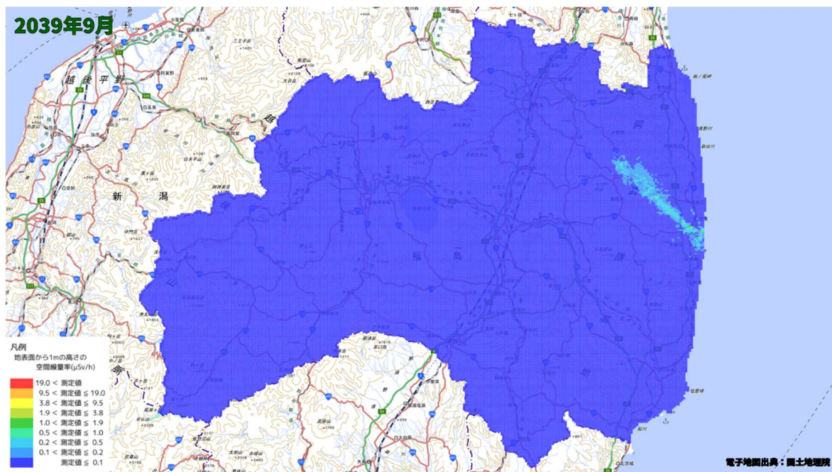
空間線量率分布将来予測解析結果(2039 年 9 月)
