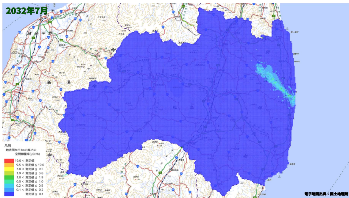
空間線量率分布将来予測解析結果(2032 年 7 月)
