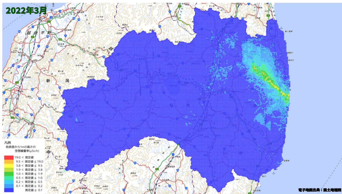
空間線量率分布将来予測解析結果(2022 年 3 月)
