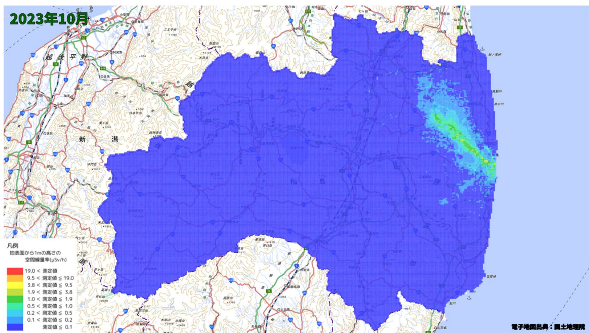
空間線量率分布将来予測解析結果(2023 年 10 月)
