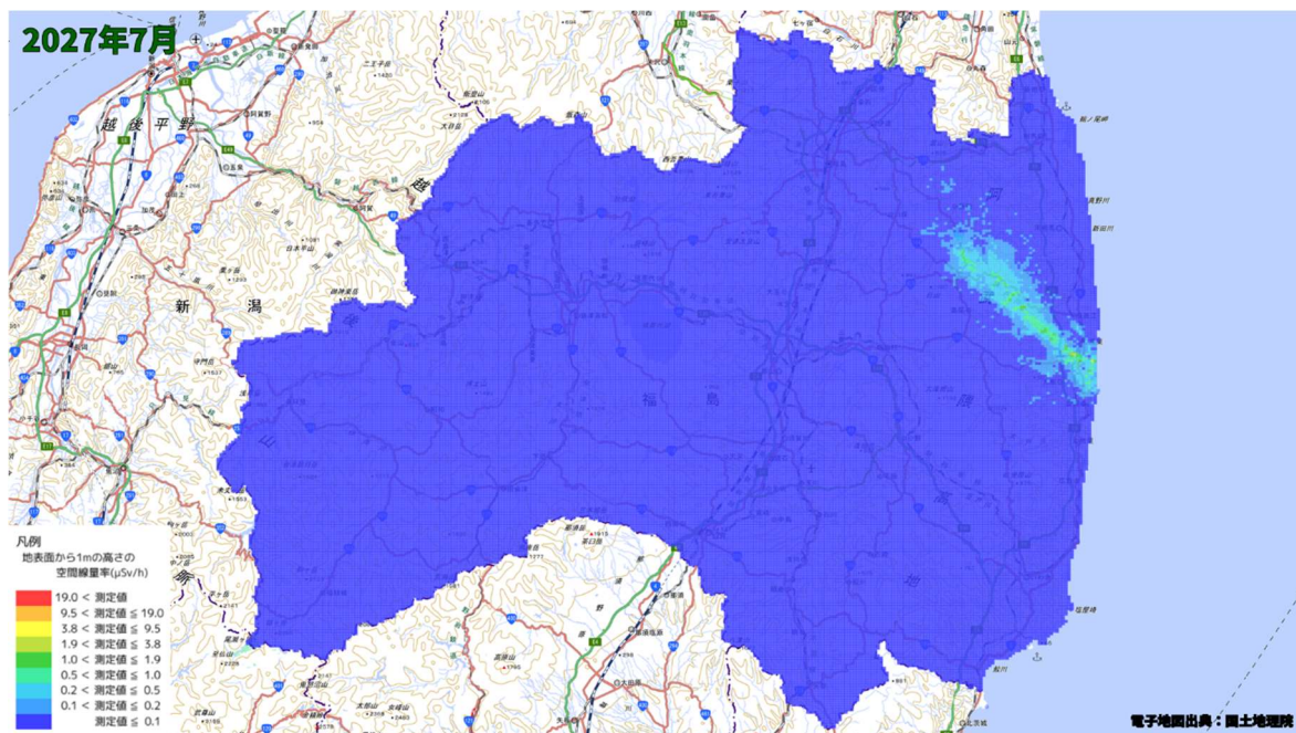
空間線量率分布将来予測解析結果(2027 年 7 月)
