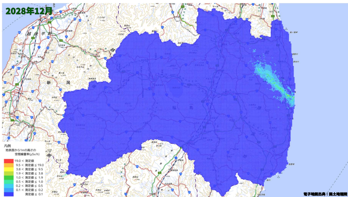
空間線量率分布将来予測解析結果(2028 年 12 月)
