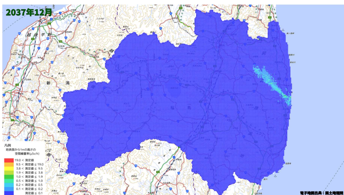
空間線量率分布将来予測解析結果(2037 年 12 月)
