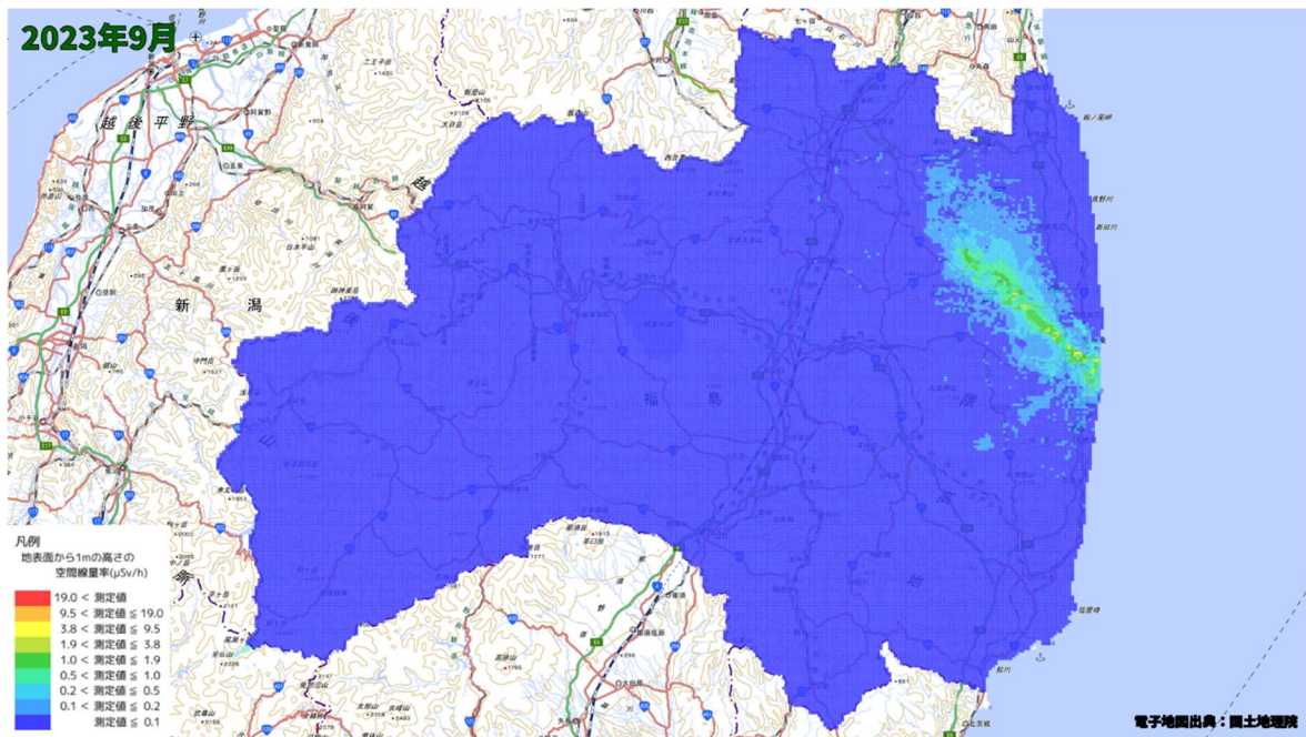
空間線量率分布将来予測解析結果(2023 年 9 月)
