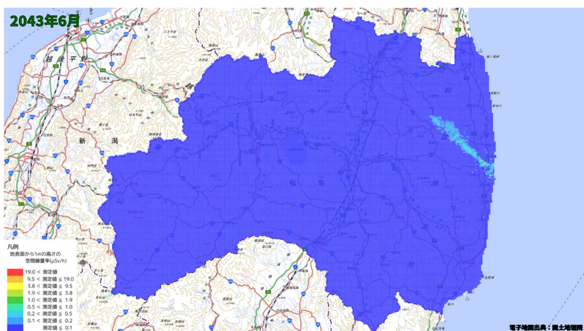
空間線量率分布将来予測解析結果(2043 年 6 月)
