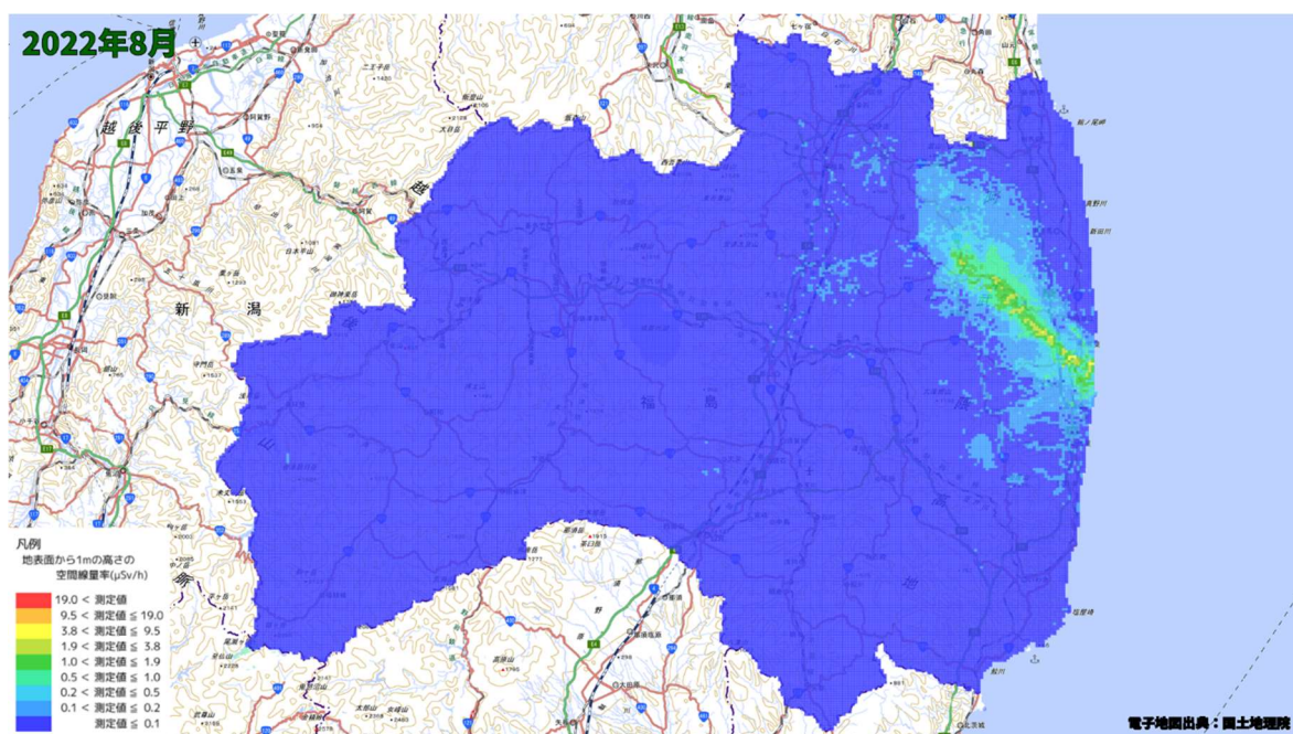
空間線量率分布将来予測解析結果(2022 年 8 月)
