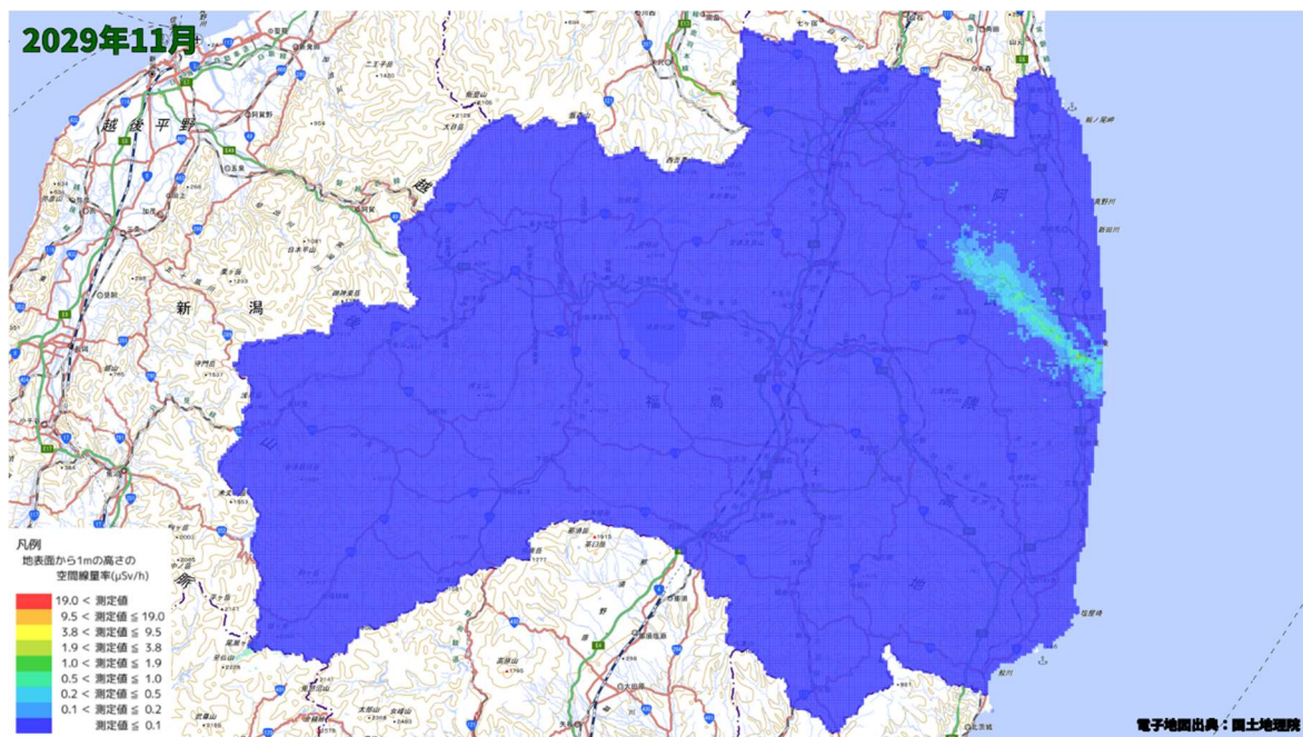
空間線量率分布将来予測解析結果(2029 年 11 月)
