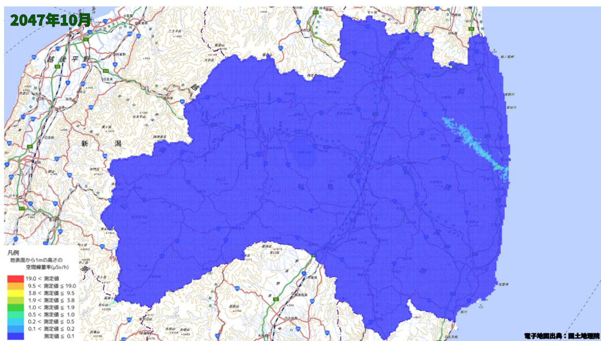
空間線量率分布将来予測解析結果(2047 年 10 月)
