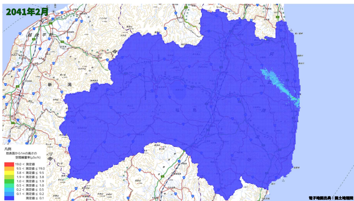
空間線量率分布将来予測解析結果(2041 年 2 月)
