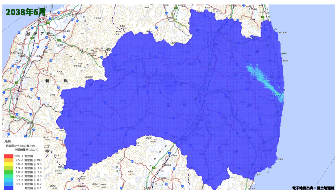
空間線量率分布将来予測解析結果(2038 年 6 月)
