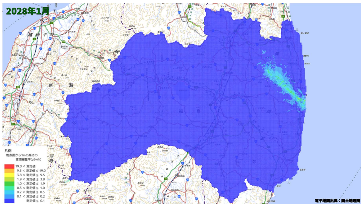
空間線量率分布将来予測解析結果(2028 年 1 月)
