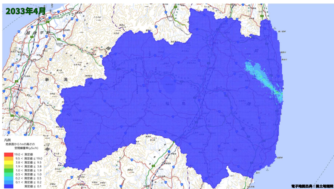
空間線量率分布将来予測解析結果(2033 年 4 月)
