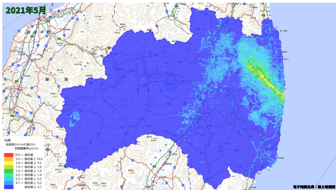
空間線量率分布将来予測解析結果(2021 年 5 月)
