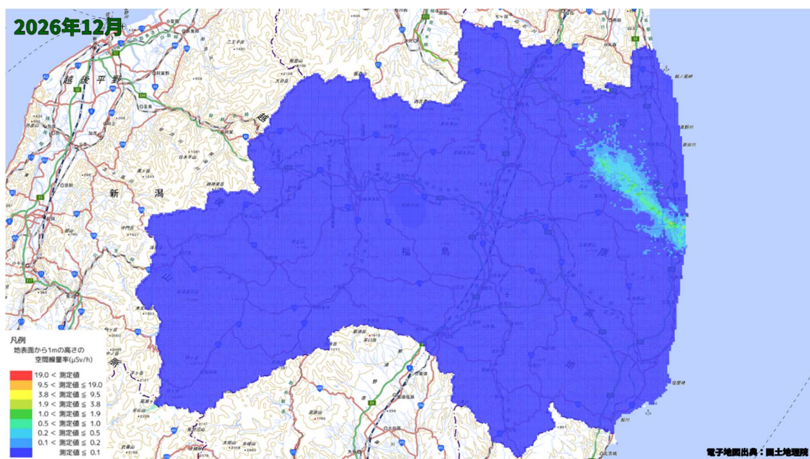
空間線量率分布将来予測解析結果(2026 年 12 月)
