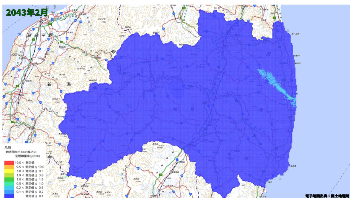
空間線量率分布将来予測解析結果(2043 年 2 月)
