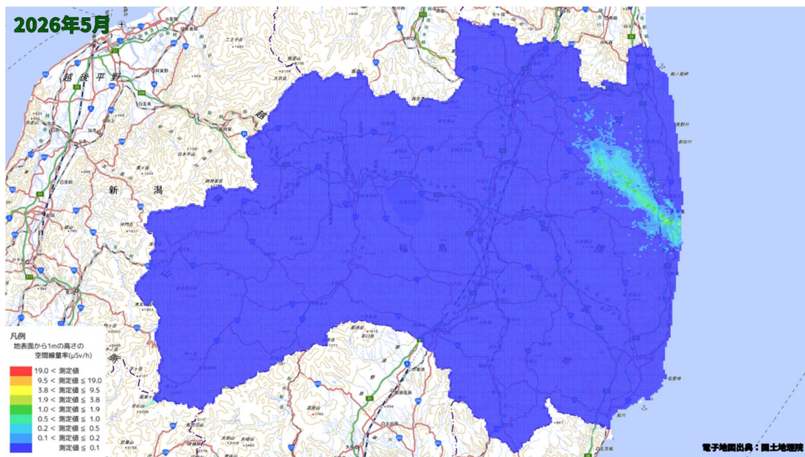
空間線量率分布将来予測解析結果(2026 年 5 月)
