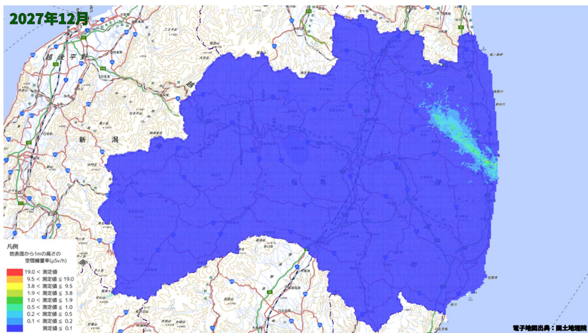
空間線量率分布将来予測解析結果(2027 年 12 月)
