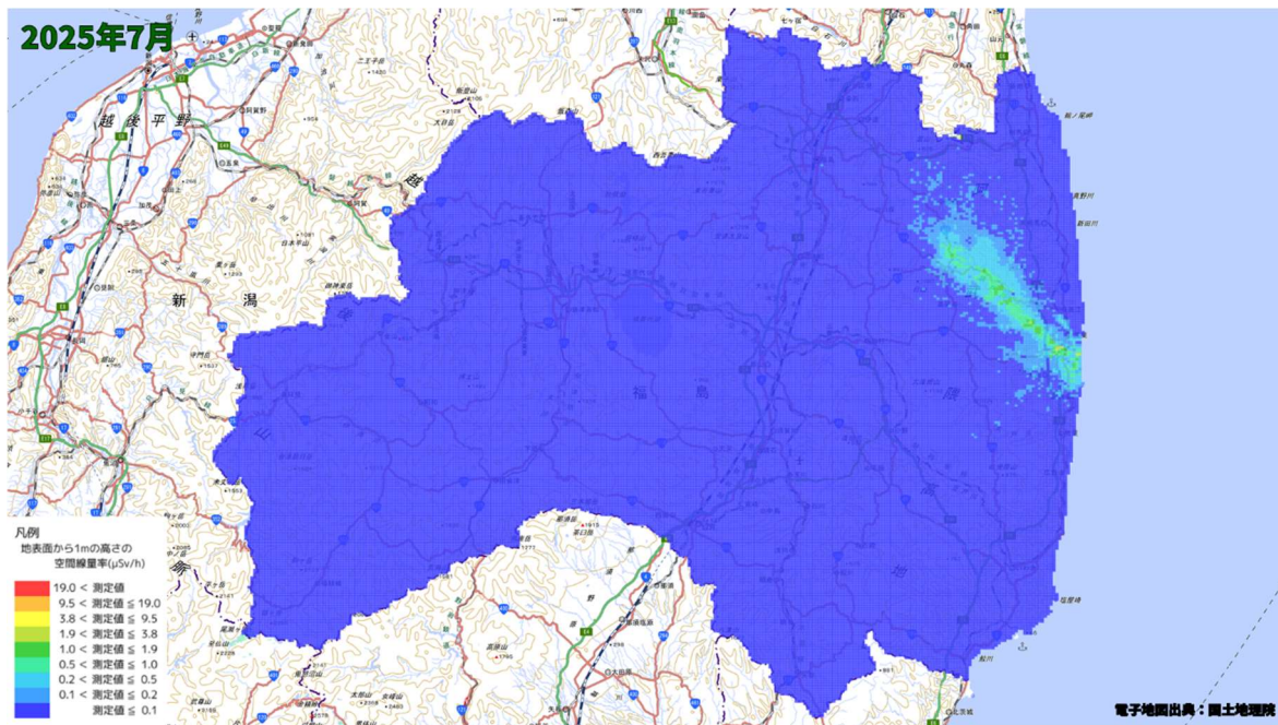
空間線量率分布将来予測解析結果(2025 年 7 月)
