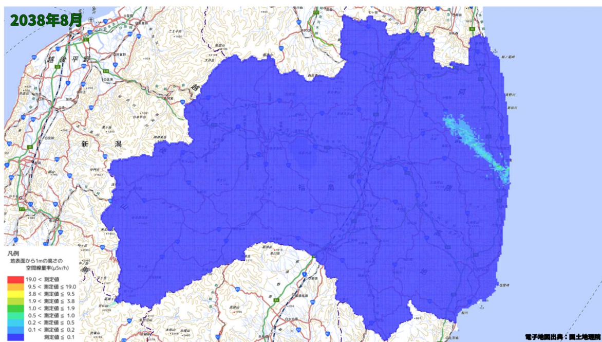
空間線量率分布将来予測解析結果(2038 年 8 月)
