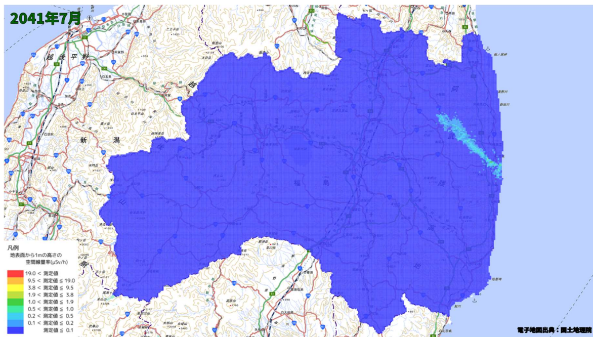
空間線量率分布将来予測解析結果(2041 年 7 月)
