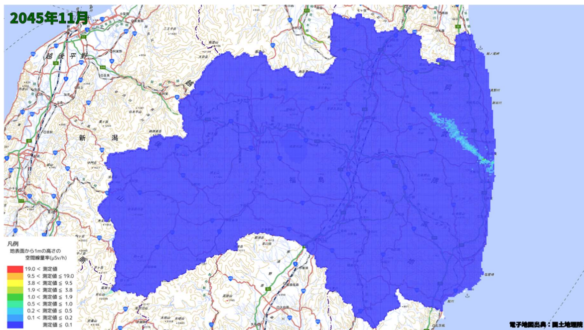
空間線量率分布将来予測解析結果(2045 年 11 月)
