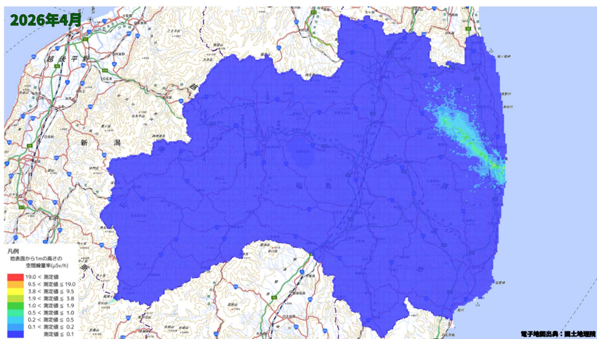
空間線量率分布将来予測解析結果(2026 年 4 月)
