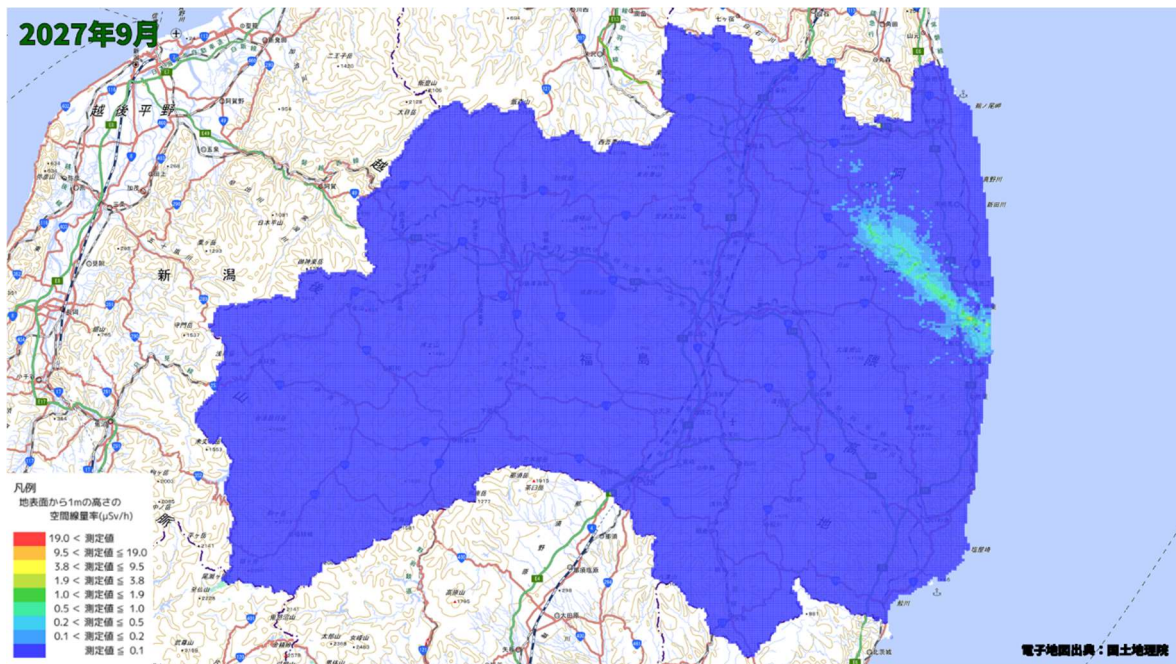
空間線量率分布将来予測解析結果(2027 年 9 月)
