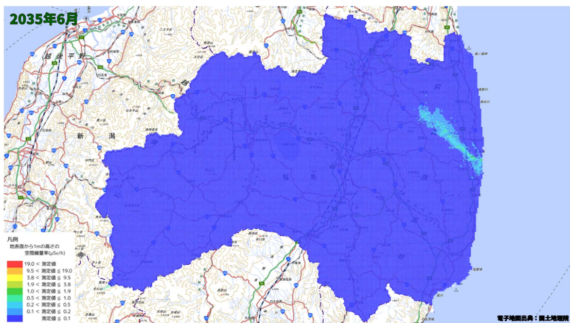
空間線量率分布将来予測解析結果(2035 年 6 月)
