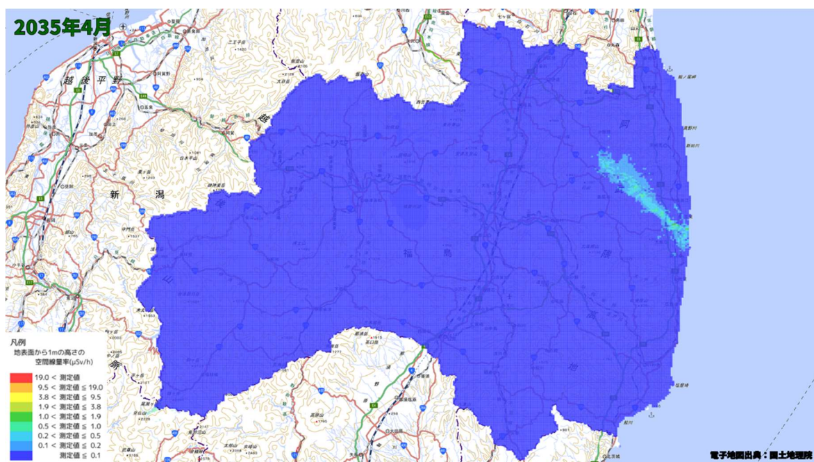
空間線量率分布将来予測解析結果(2035 年 4 月)
