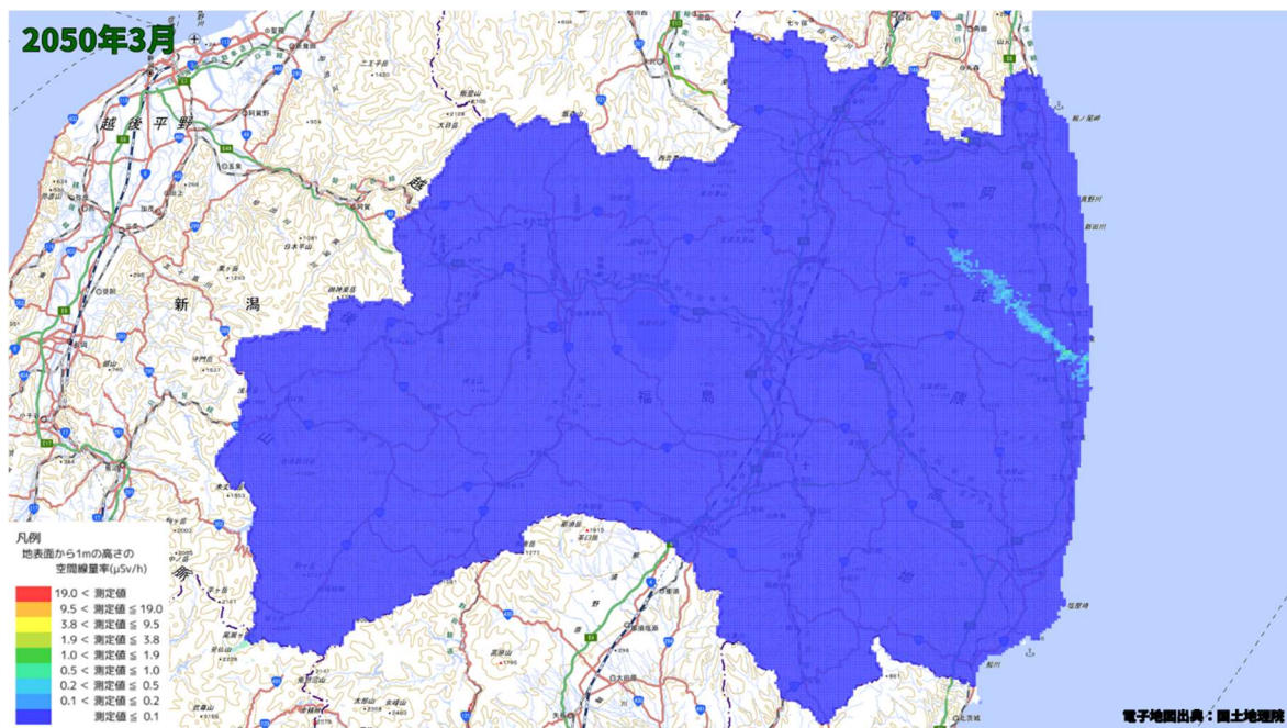
空間線量率分布将来予測解析結果(2050 年 3 月)
