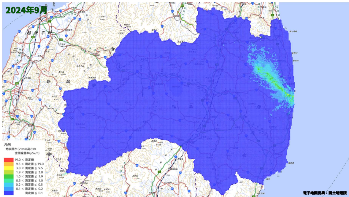
空間線量率分布将来予測解析結果(2024 年 9 月)
