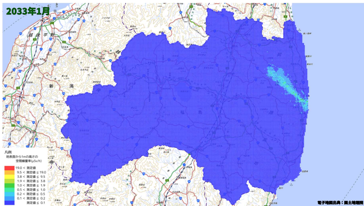
空間線量率分布将来予測解析結果(2033 年 1 月)
