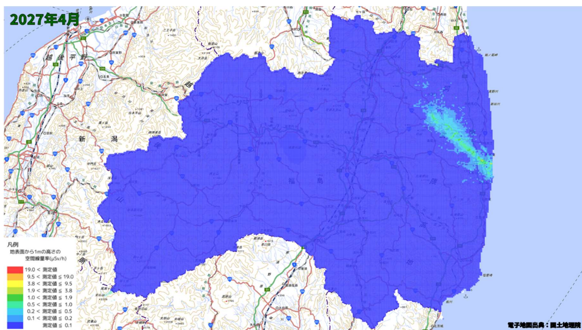
空間線量率分布将来予測解析結果(2027 年 4 月)
