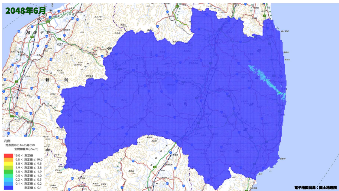
空間線量率分布将来予測解析結果(2048 年 6 月)
