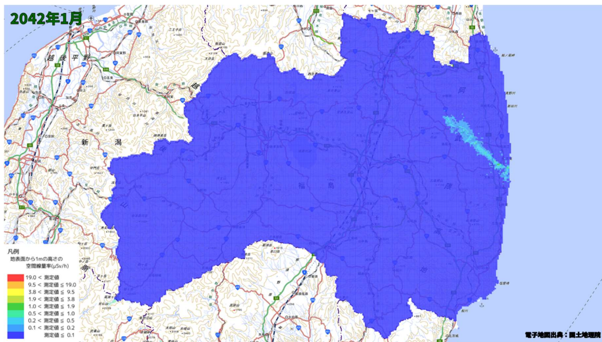
空間線量率分布将来予測解析結果(2042 年 1 月)
