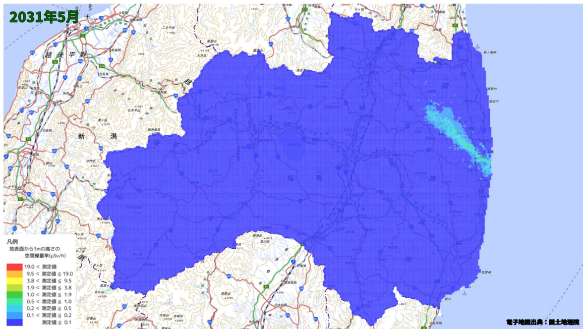
空間線量率分布将来予測解析結果(2031 年 5 月)
