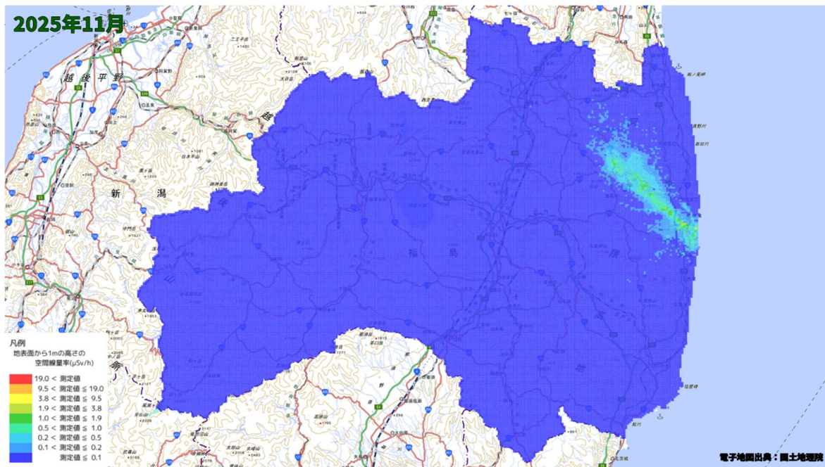
空間線量率分布将来予測解析結果(2025 年 11 月)
