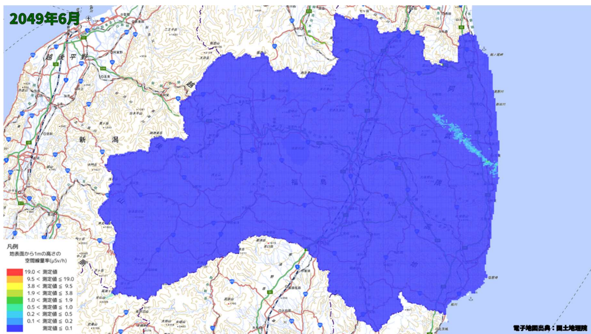
空間線量率分布将来予測解析結果(2049 年 6 月)
