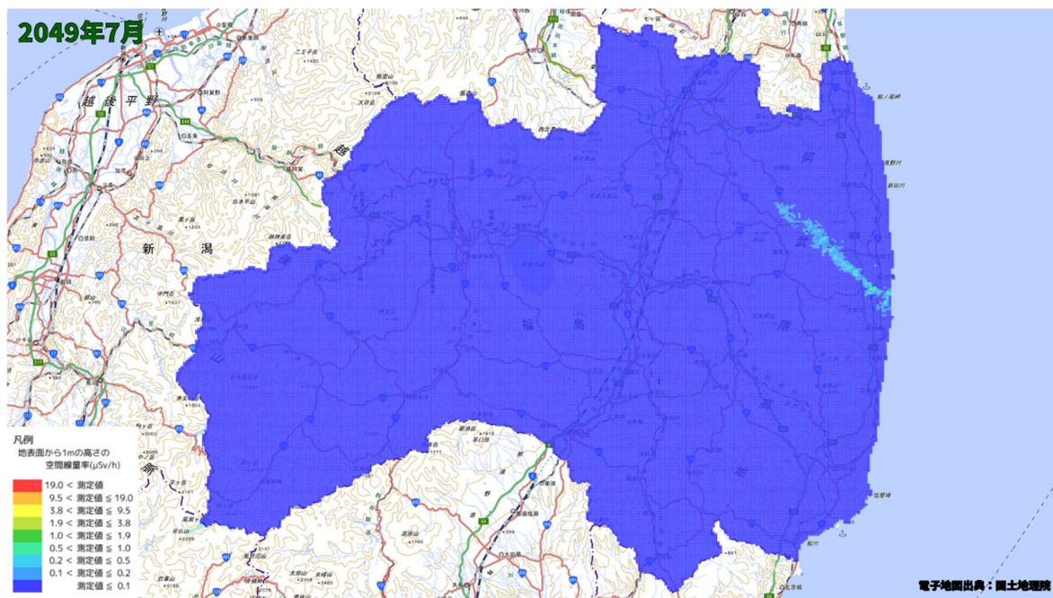
空間線量率分布将来予測解析結果(2049 年 7 月)
