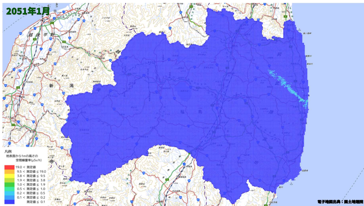
空間線量率分布将来予測解析結果(2051 年 1 月)
