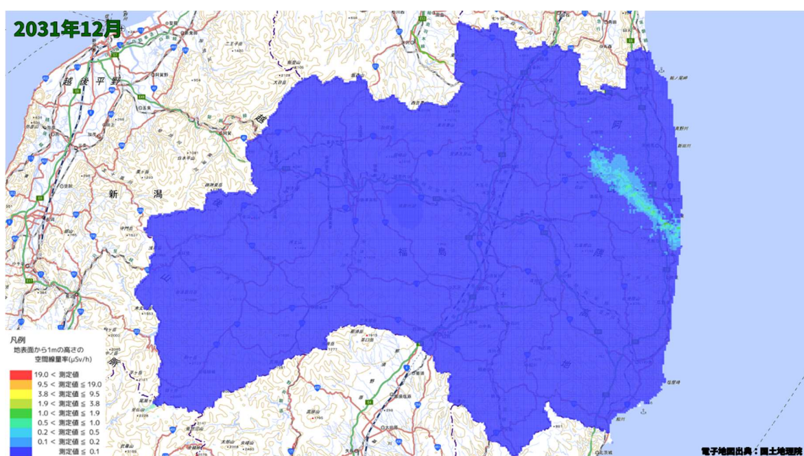
空間線量率分布将来予測解析結果(2031 年 12 月)
