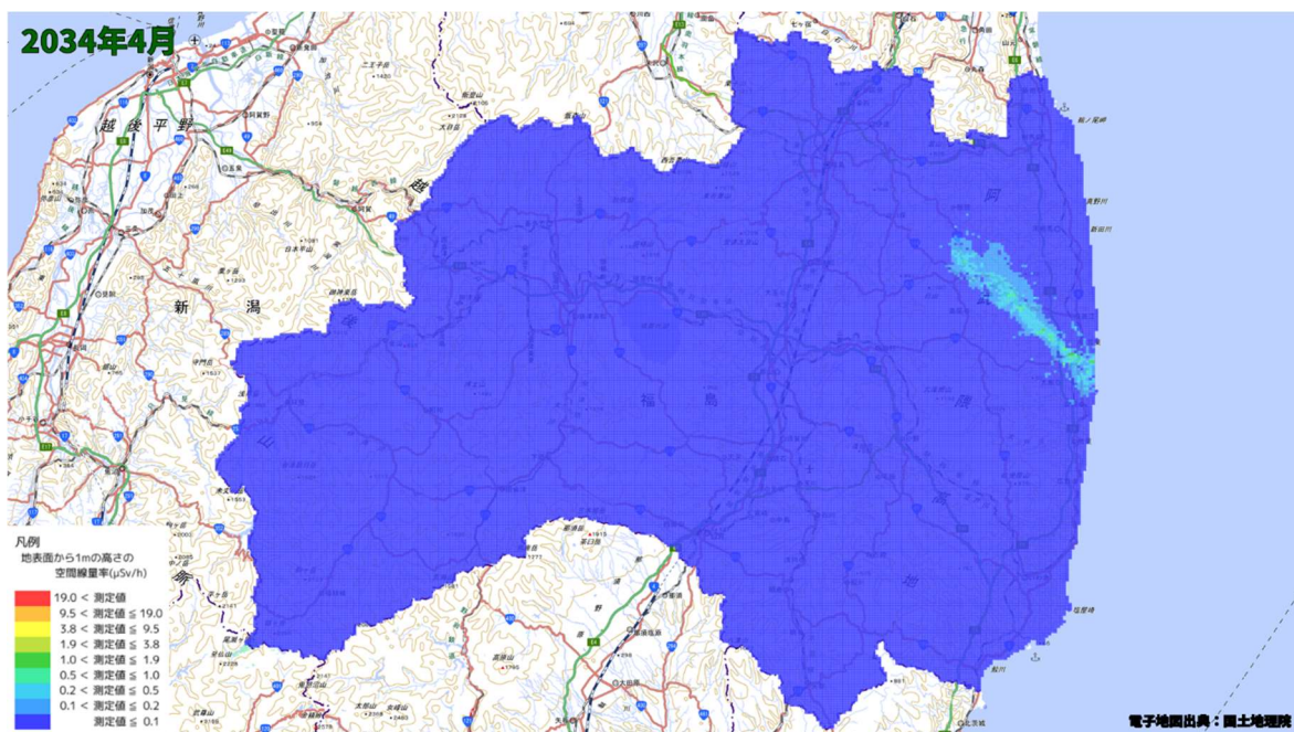
空間線量率分布将来予測解析結果(2034 年 4 月)
