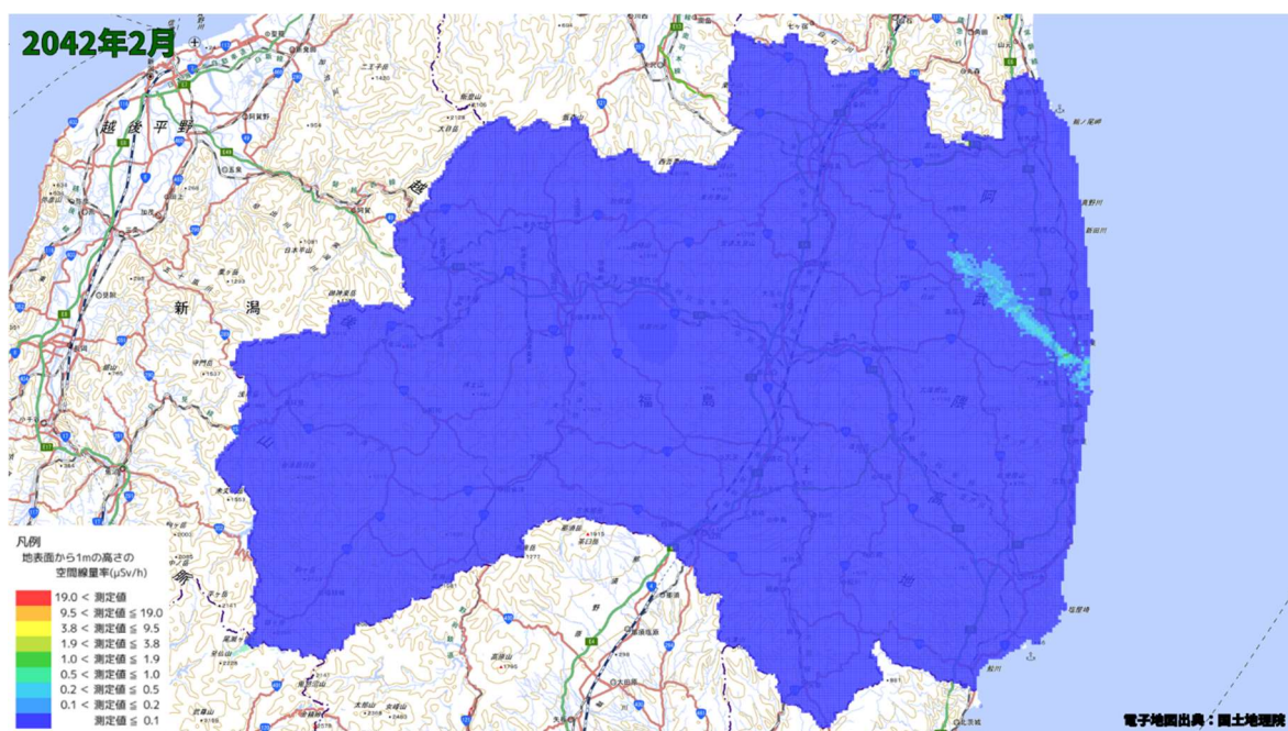
空間線量率分布将来予測解析結果(2042 年 2 月)
