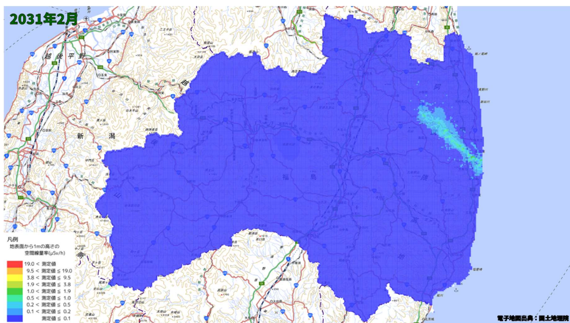
空間線量率分布将来予測解析結果(2031 年 2 月)
