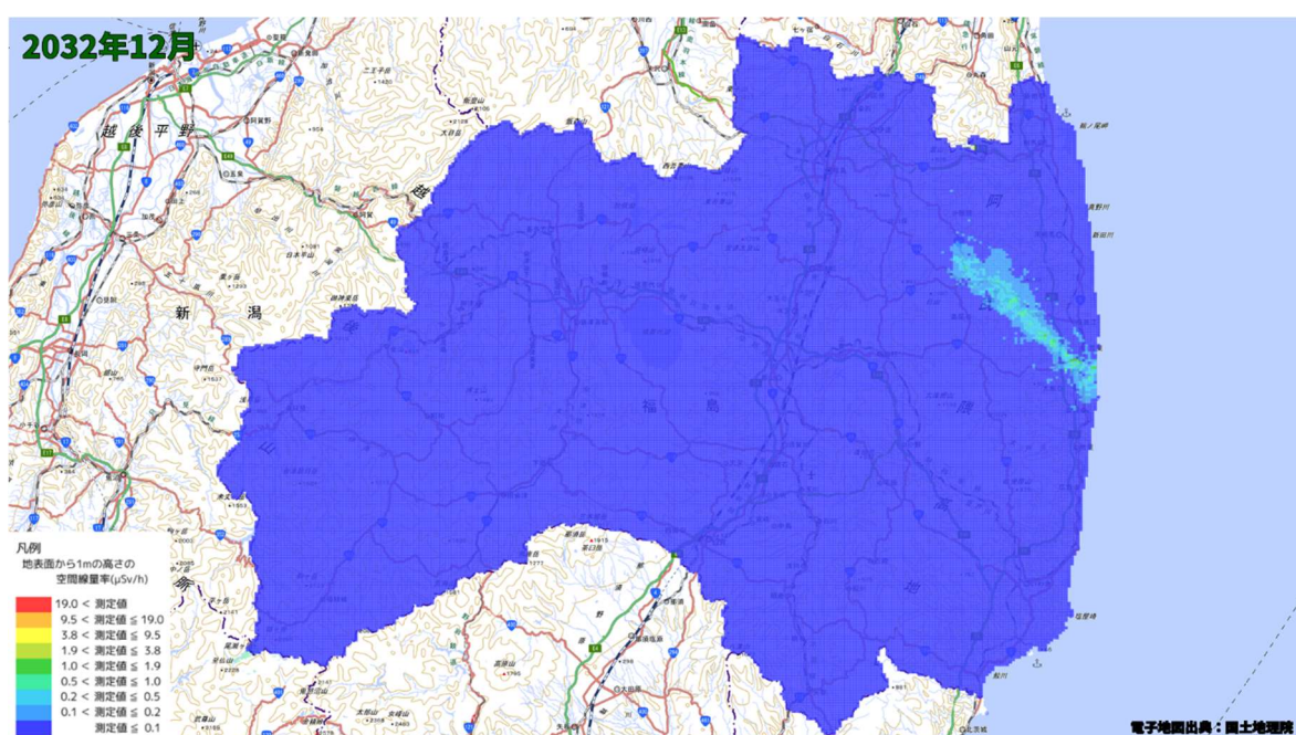
空間線量率分布将来予測解析結果(2032 年 12 月)
