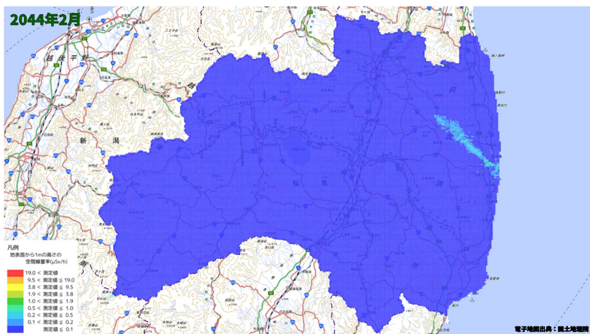
空間線量率分布将来予測解析結果(2044 年 2 月)
