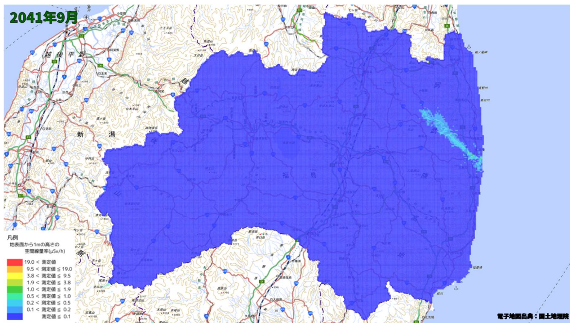
空間線量率分布将来予測解析結果(2041 年 9 月)
