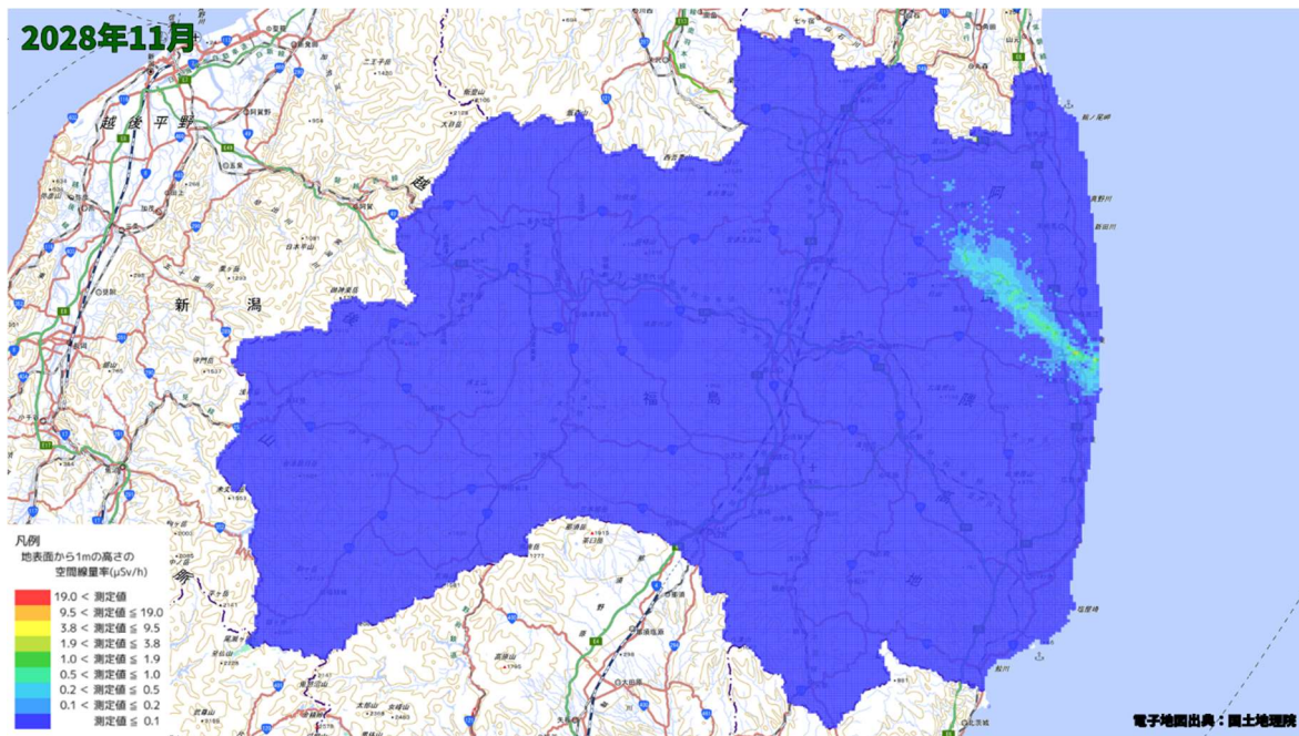
空間線量率分布将来予測解析結果(2028 年 11 月)
