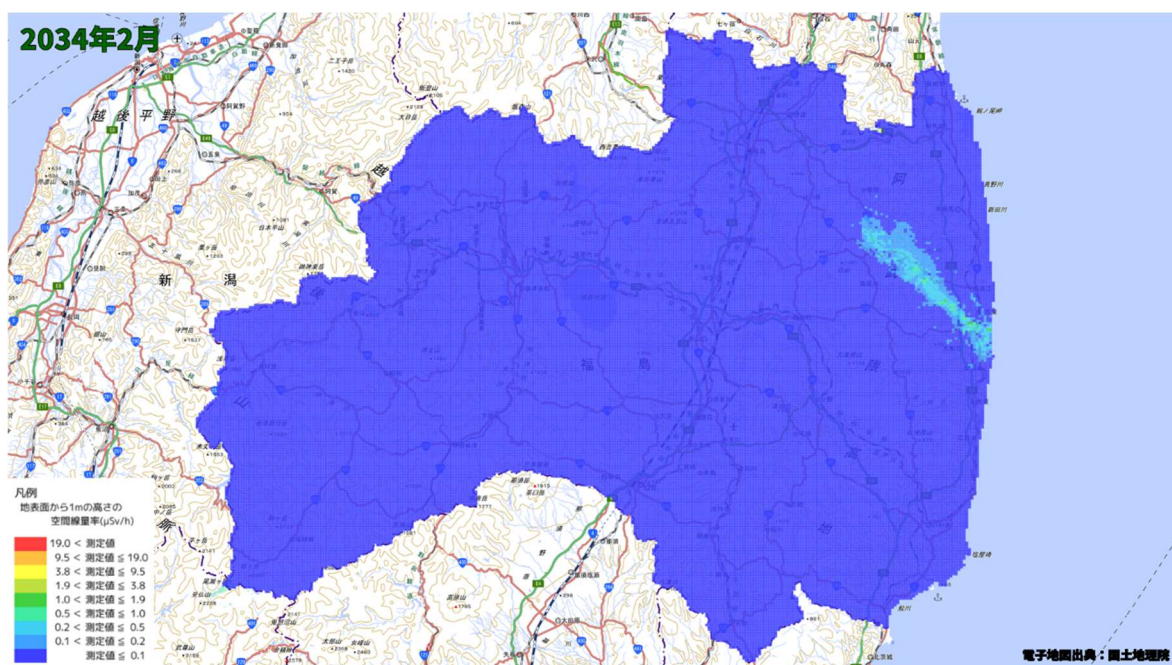
空間線量率分布将来予測解析結果(2034 年 2 月)
