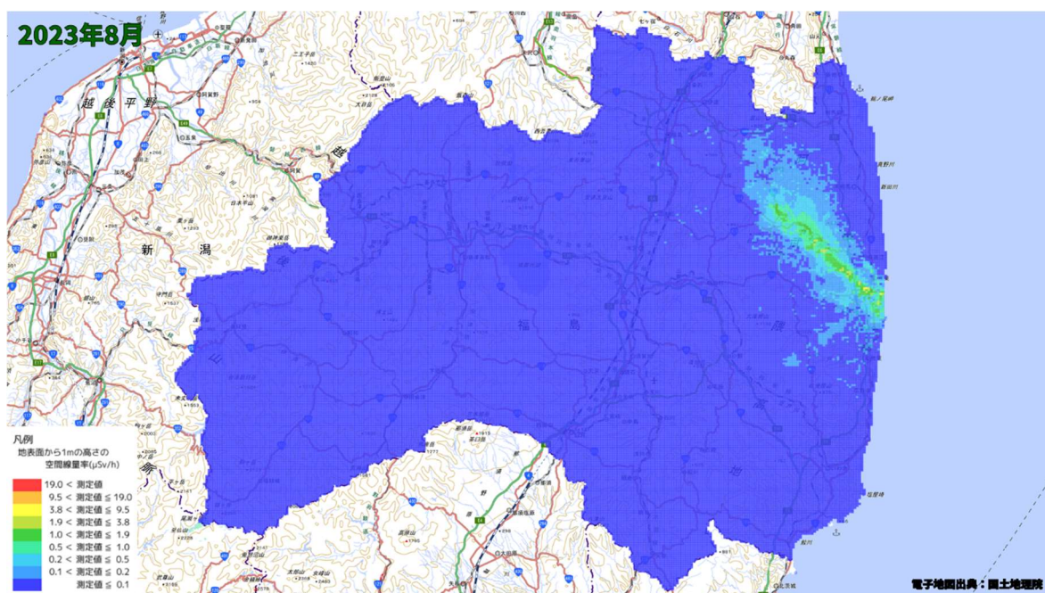
空間線量率分布将来予測解析結果(2023 年 8 月)
