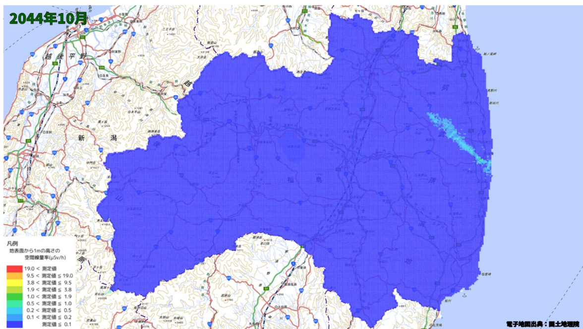
空間線量率分布将来予測解析結果(2044 年 10 月)
