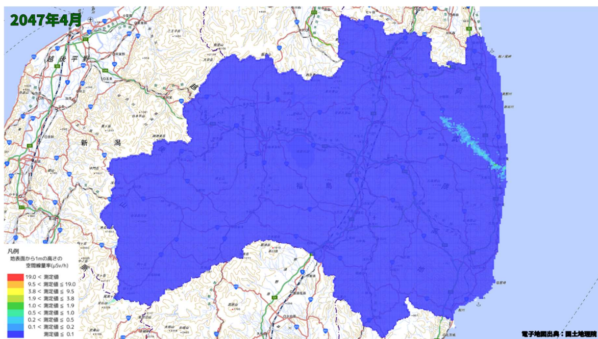
空間線量率分布将来予測解析結果(2047 年 4 月)
