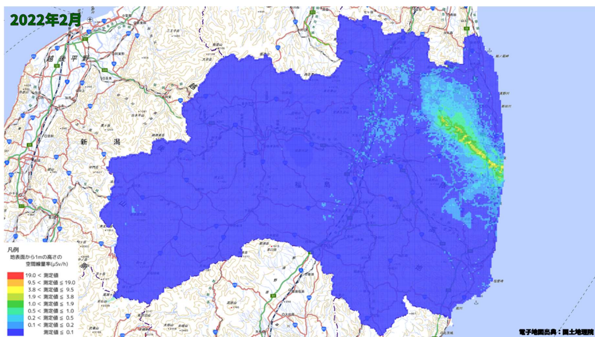
空間線量率分布将来予測解析結果(2022 年 2 月)
