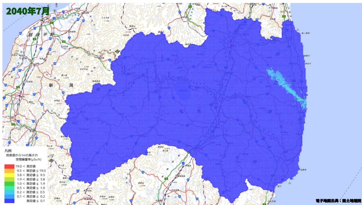
空間線量率分布将来予測解析結果(2040 年 7 月)
