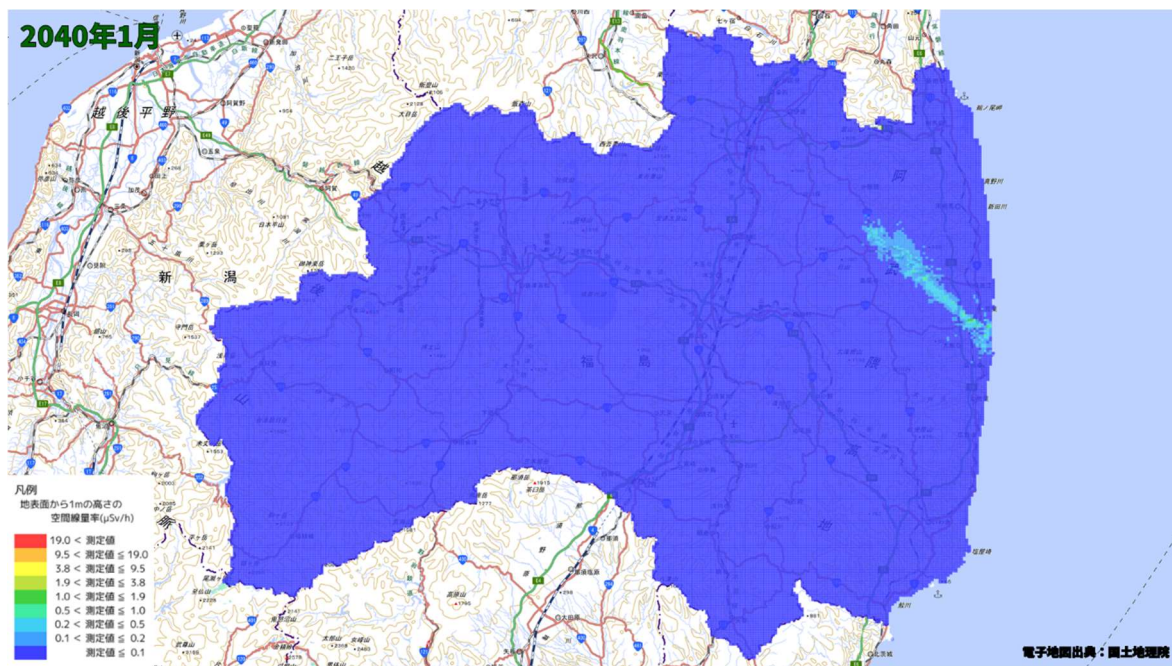
空間線量率分布将来予測解析結果(2040 年 1 月)
