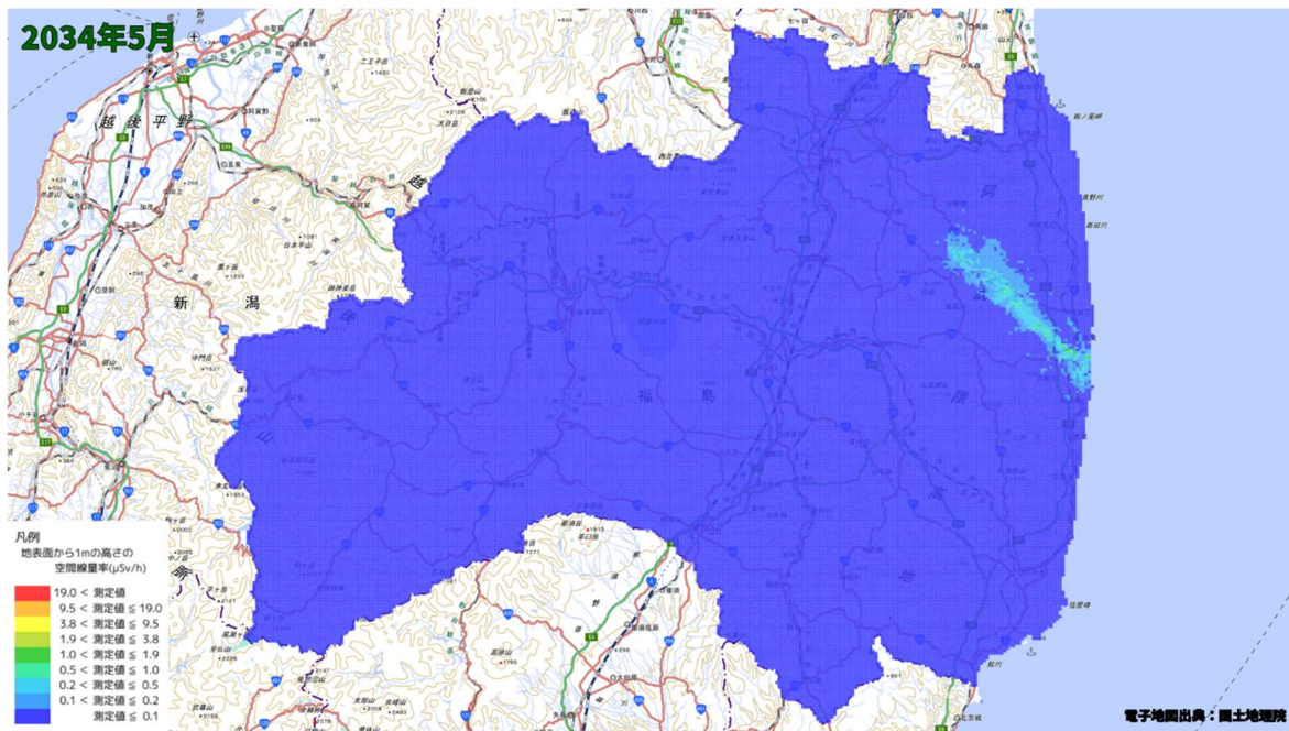
空間線量率分布将来予測解析結果(2034 年 5 月)
