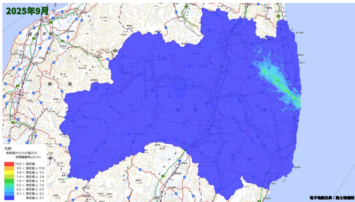
空間線量率分布将来予測解析結果(2025 年 9 月)
