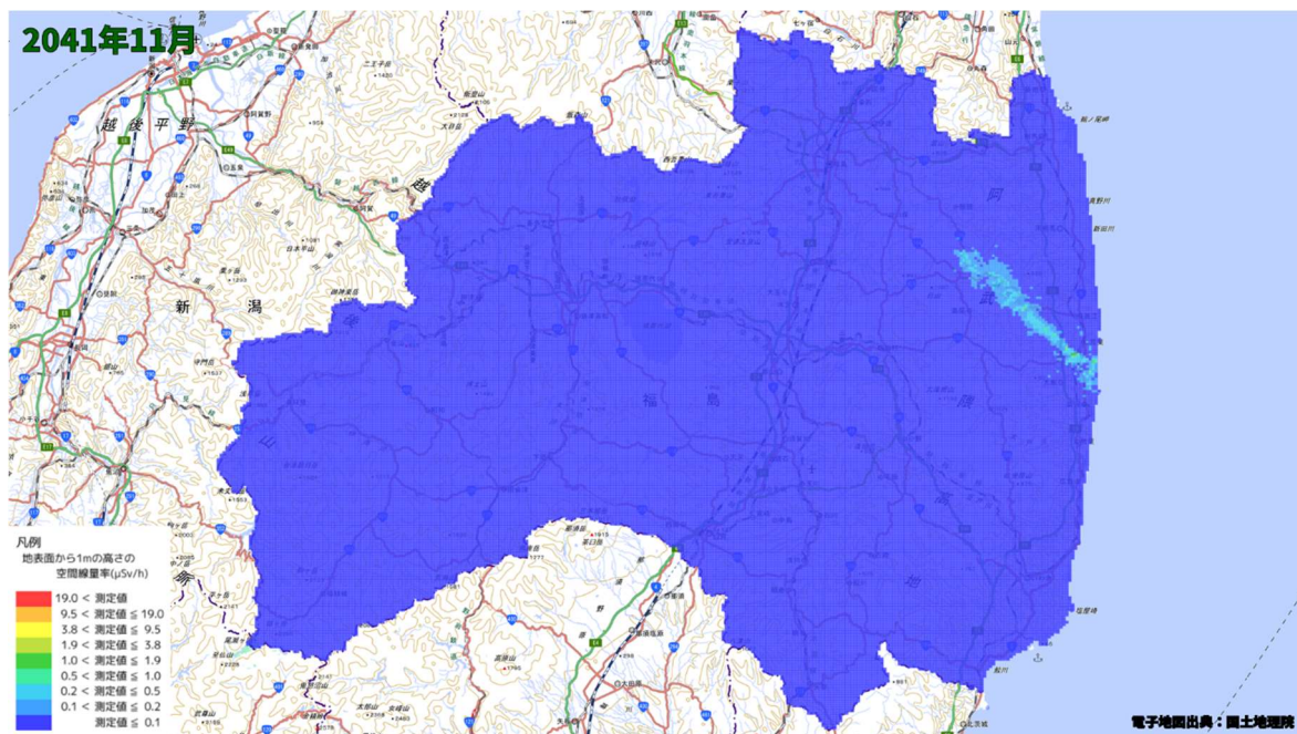
空間線量率分布将来予測解析結果(2041 年 11 月)
