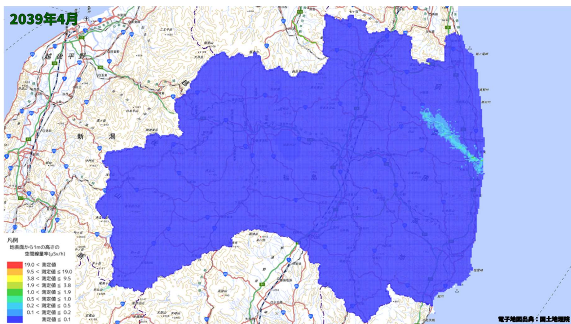
空間線量率分布将来予測解析結果(2039 年 4 月)
