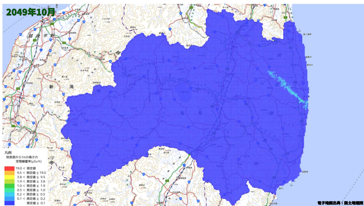
空間線量率分布将来予測解析結果(2049 年 10 月)
