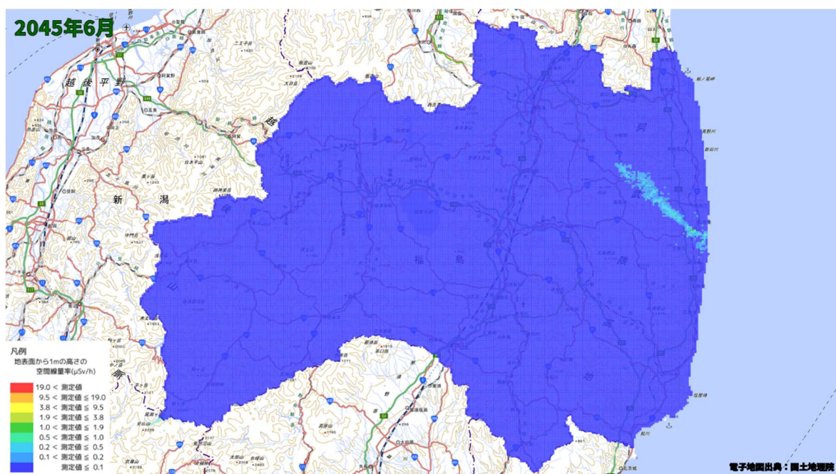
空間線量率分布将来予測解析結果(2045 年 6 月)
