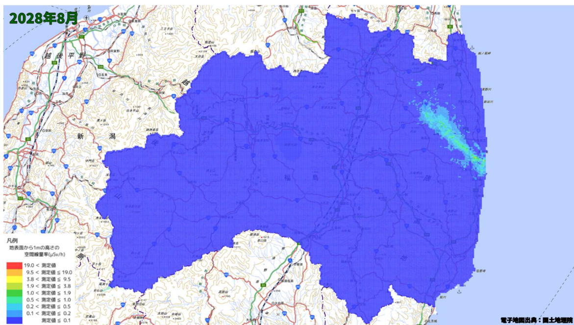
空間線量率分布将来予測解析結果(2028 年 8 月)
