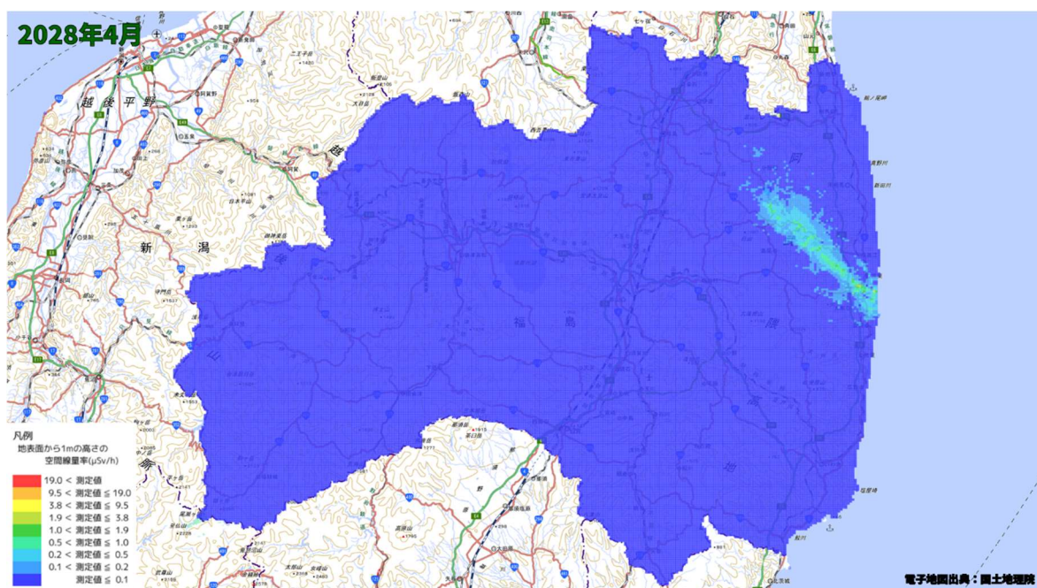
空間線量率分布将来予測解析結果(2028 年 4 月)
