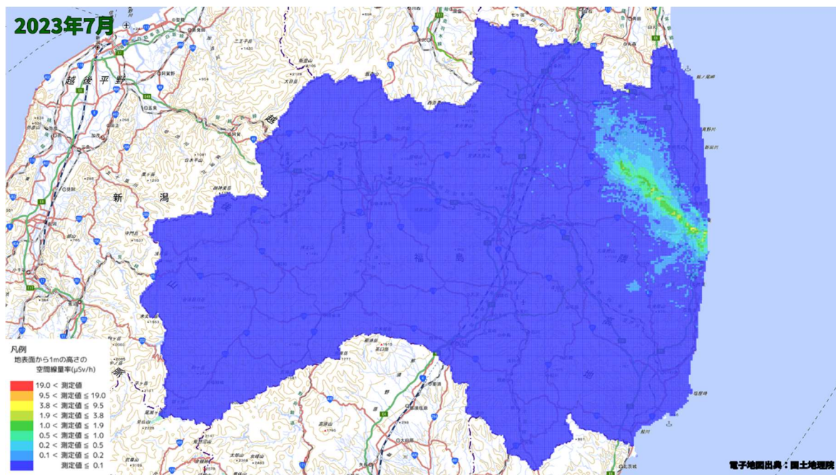
空間線量率分布将来予測解析結果(2023 年 7 月)
