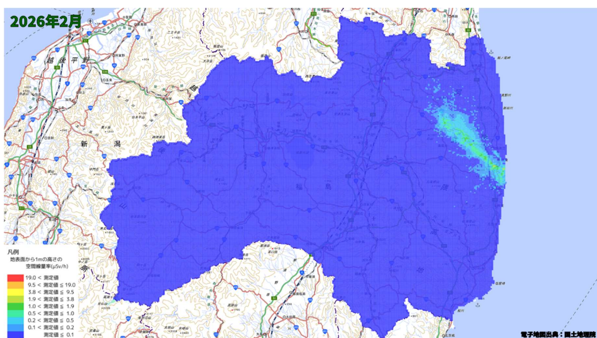
空間線量率分布将来予測解析結果(2026 年 2 月)
