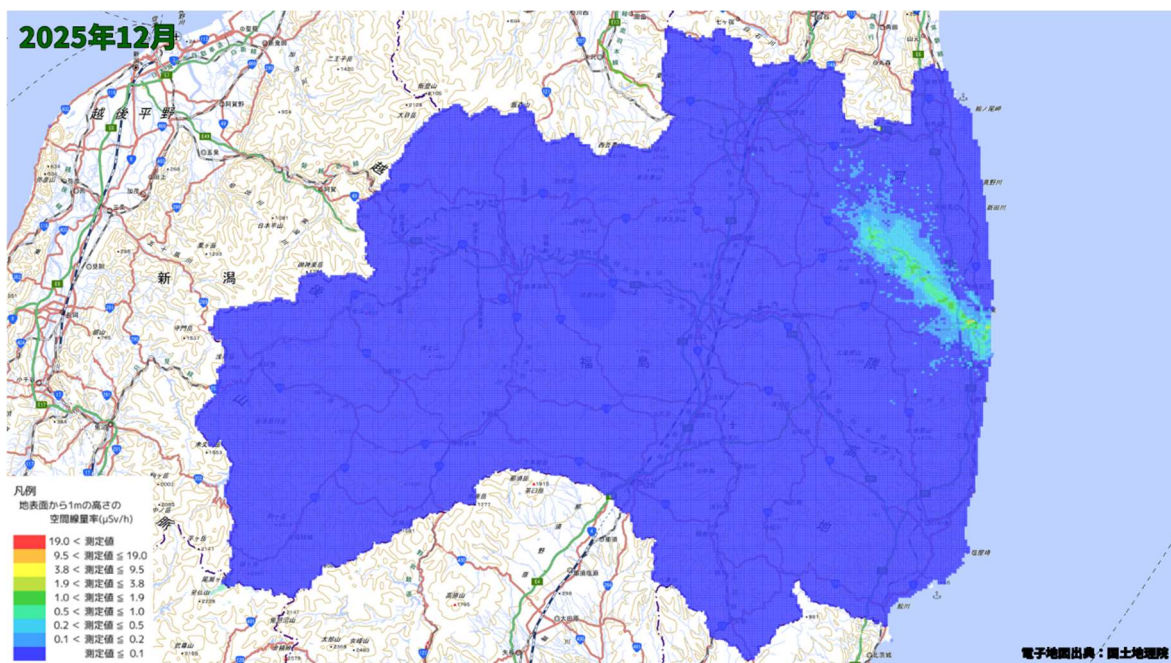
空間線量率分布将来予測解析結果(2025 年 12 月)
