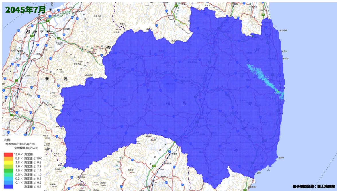
空間線量率分布将来予測解析結果(2045 年 7 月)
