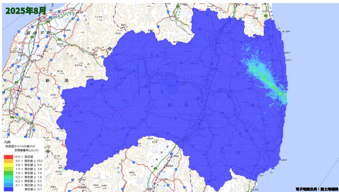
空間線量率分布将来予測解析結果(2025 年 8 月)
