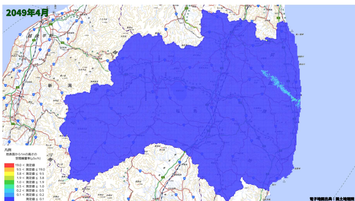
空間線量率分布将来予測解析結果(2049 年 4 月)
