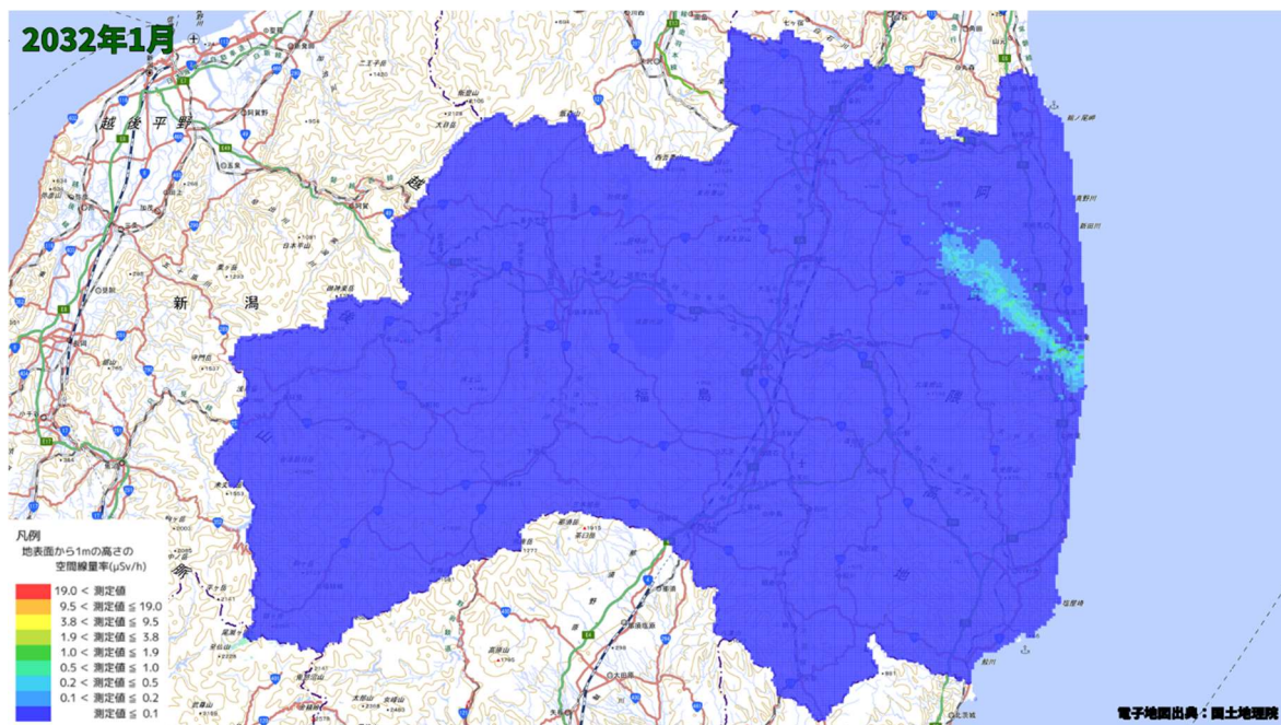
空間線量率分布将来予測解析結果(2032 年 1 月)
