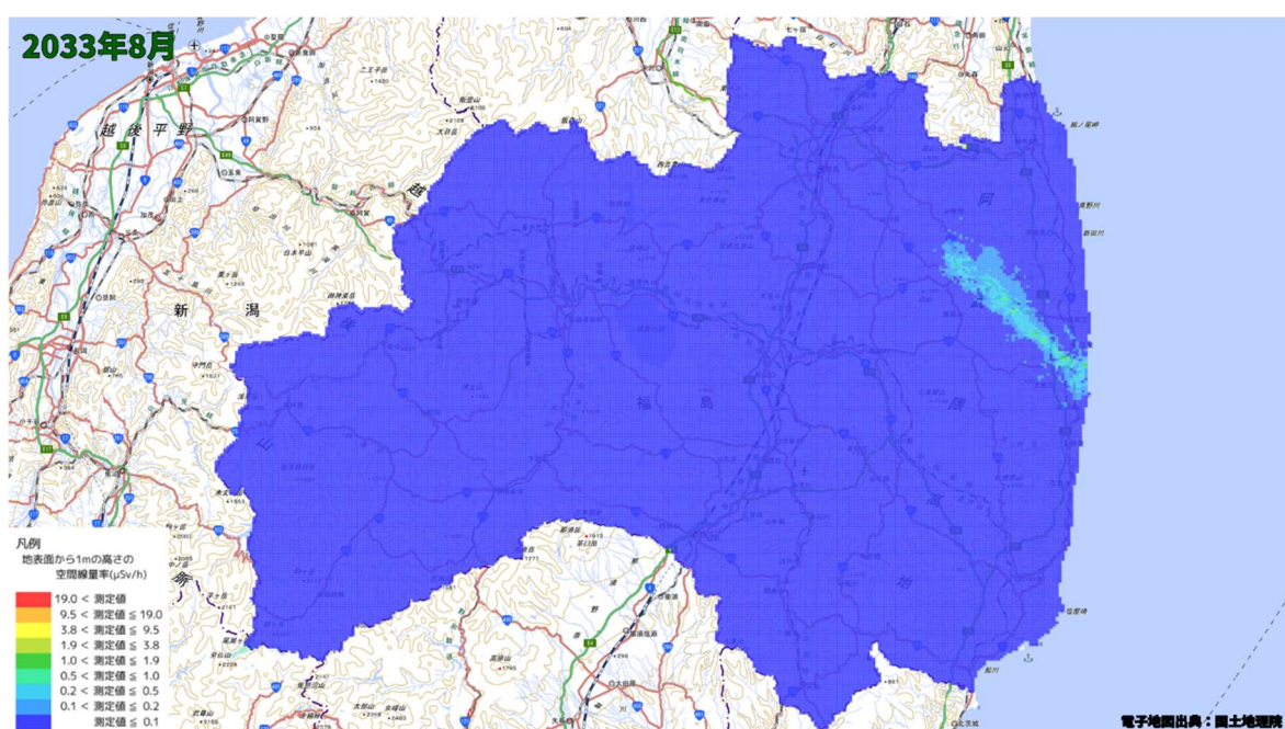
空間線量率分布将来予測解析結果(2033 年 8 月)
