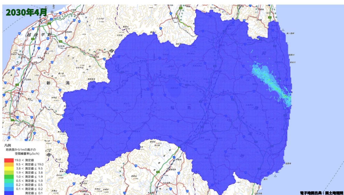
空間線量率分布将来予測解析結果(2030 年 4 月)
