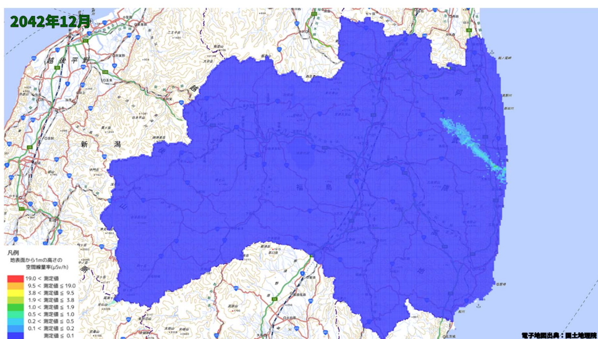
空間線量率分布将来予測解析結果(2042 年 12 月)
