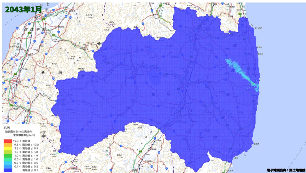
空間線量率分布将来予測解析結果(2043 年 1 月)
