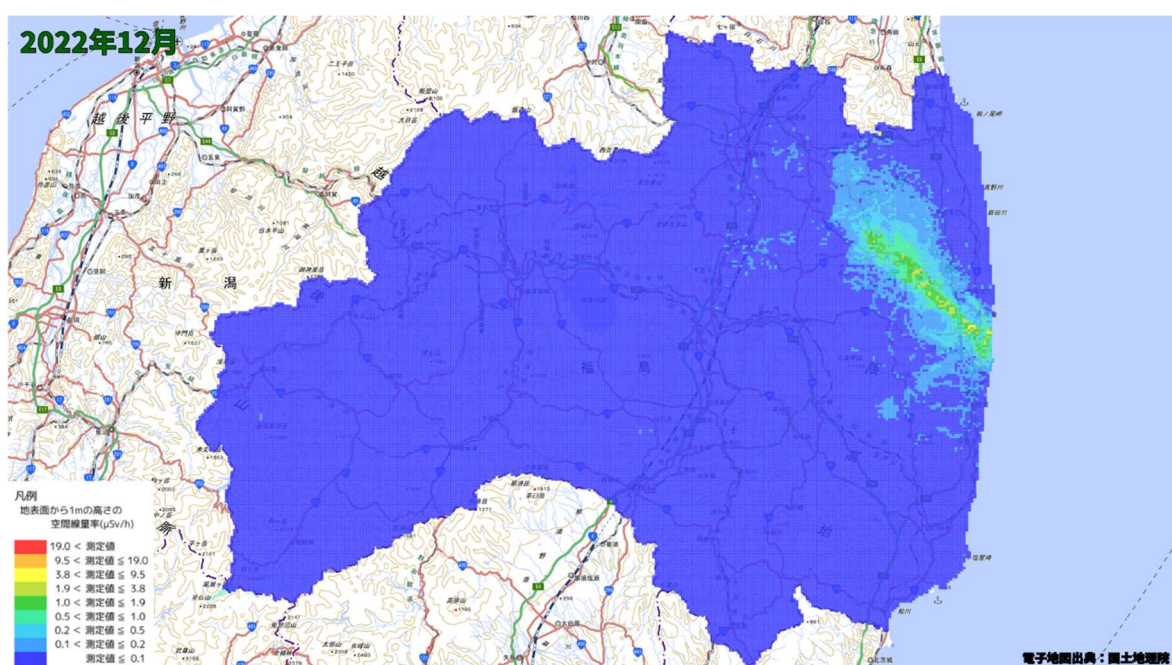
空間線量率分布将来予測解析結果(2022 年 12 月)
