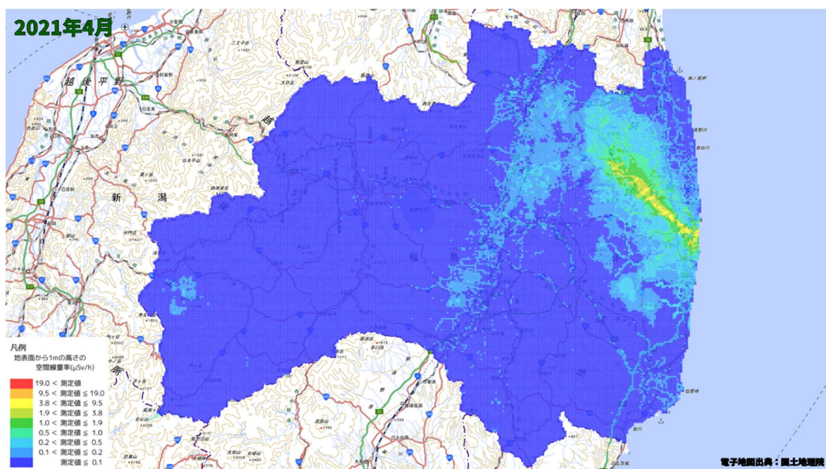
空間線量率分布将来予測解析結果(2021 年 4 月)
