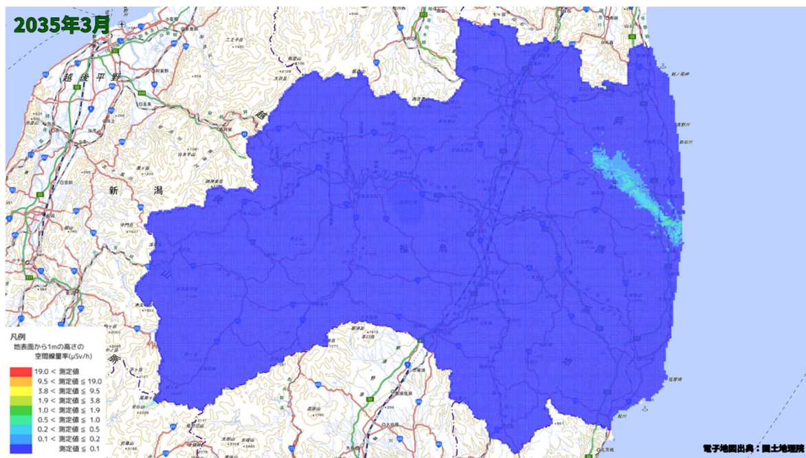
空間線量率分布将来予測解析結果(2035 年 3 月)
