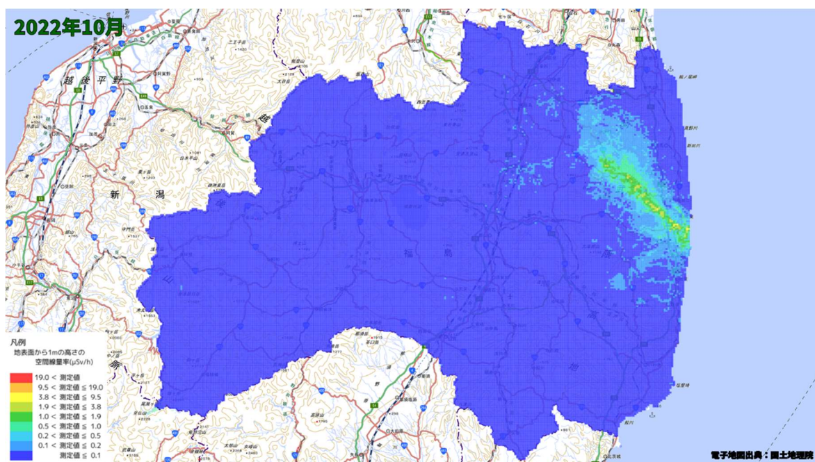
空間線量率分布将来予測解析結果(2022 年 10 月)
