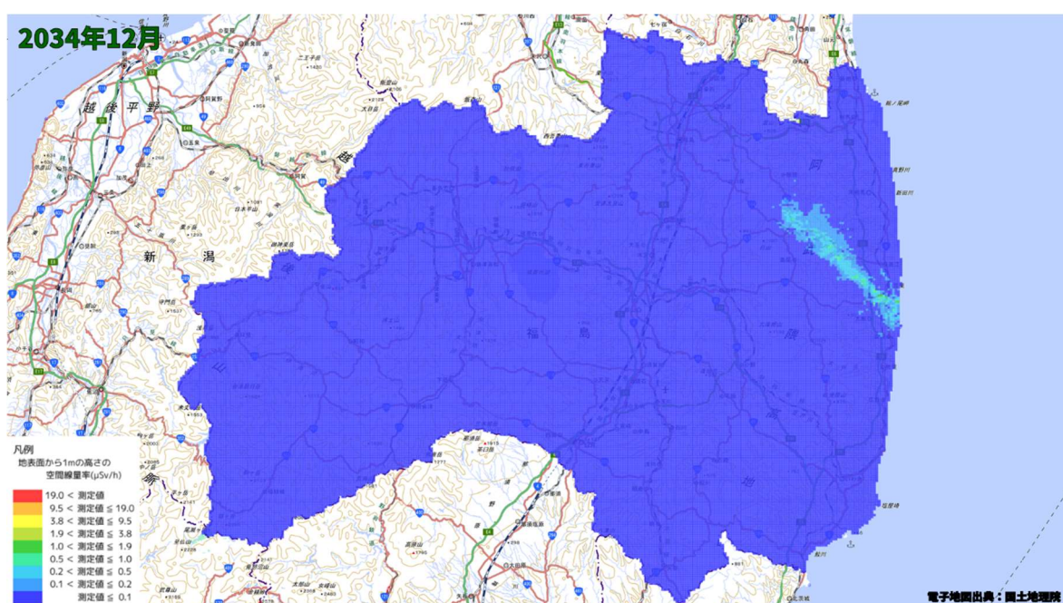
空間線量率分布将来予測解析結果(2034 年 12 月)
