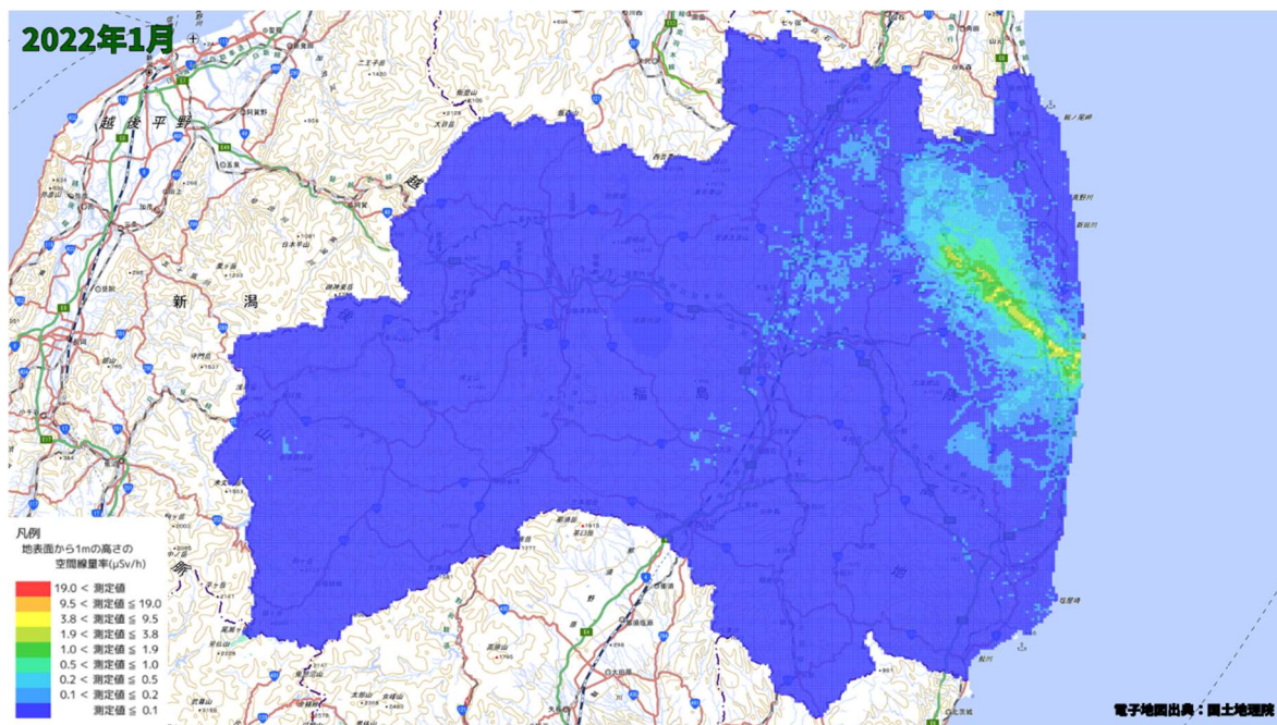
空間線量率分布将来予測解析結果(2022 年 1 月)
