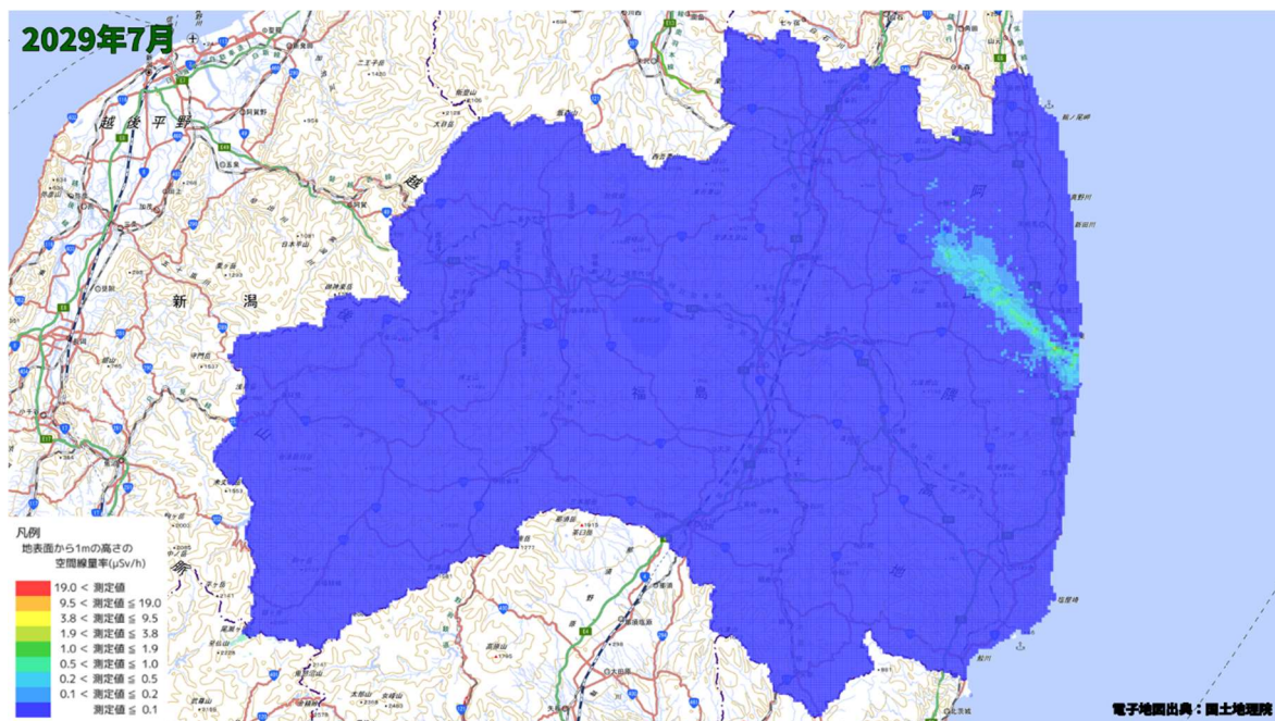
空間線量率分布将来予測解析結果(2029 年 7 月)
