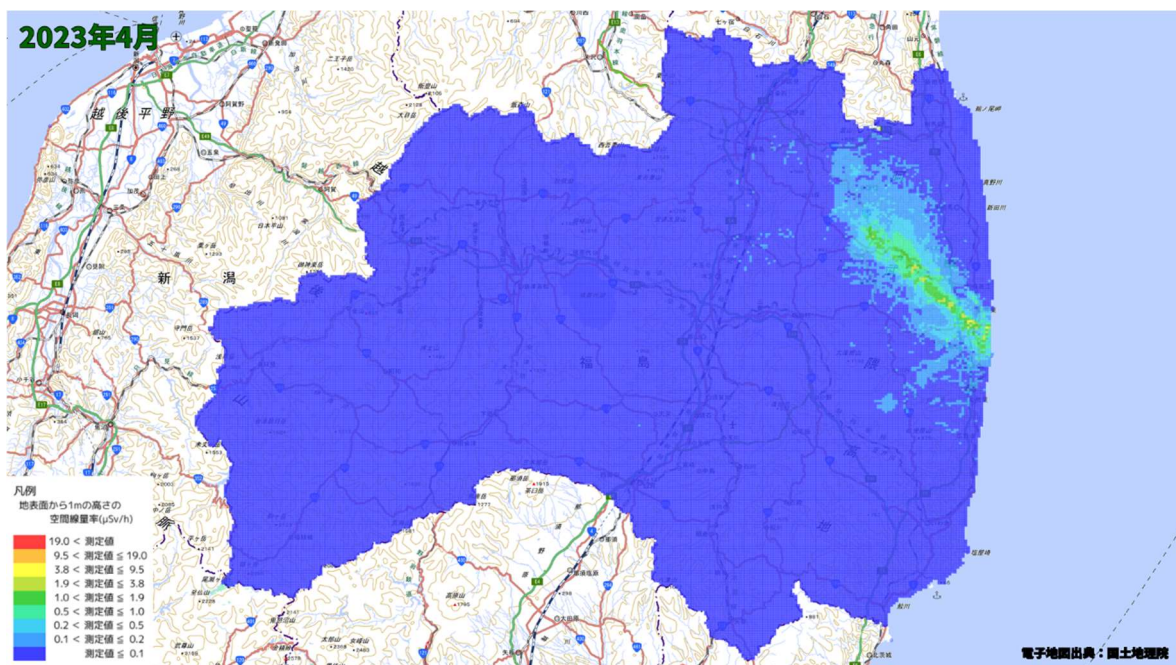
空間線量率分布将来予測解析結果(2023 年 4 月)
