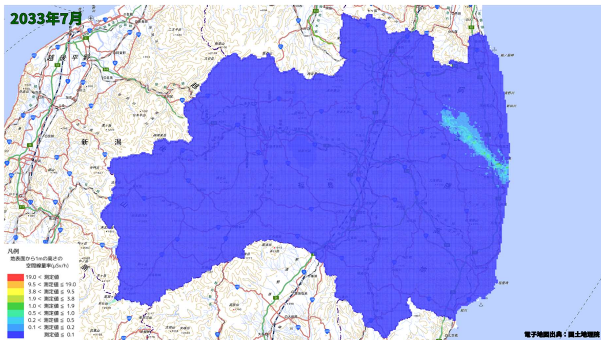
空間線量率分布将来予測解析結果(2033 年 7 月)
