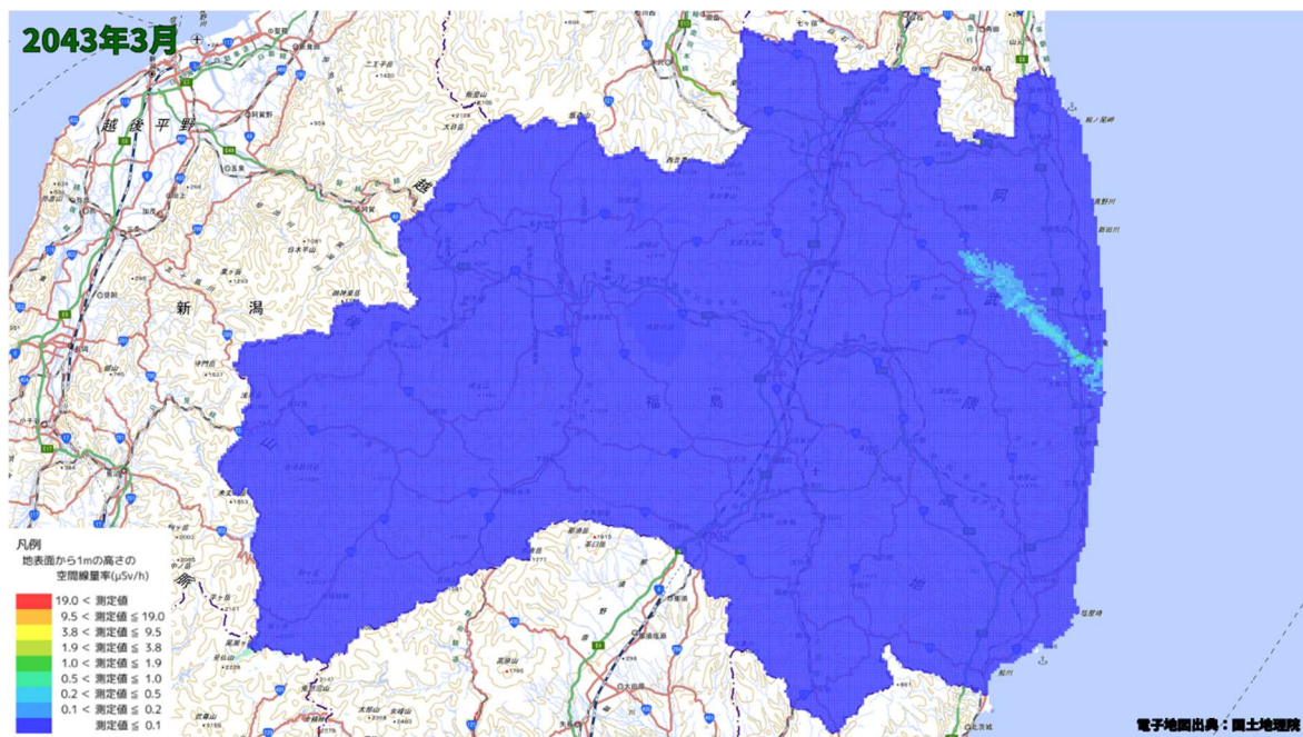
空間線量率分布将来予測解析結果(2043 年 3 月)
