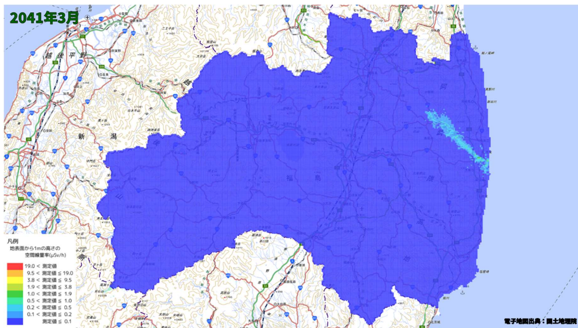
空間線量率分布将来予測解析結果(2041 年 3 月)
