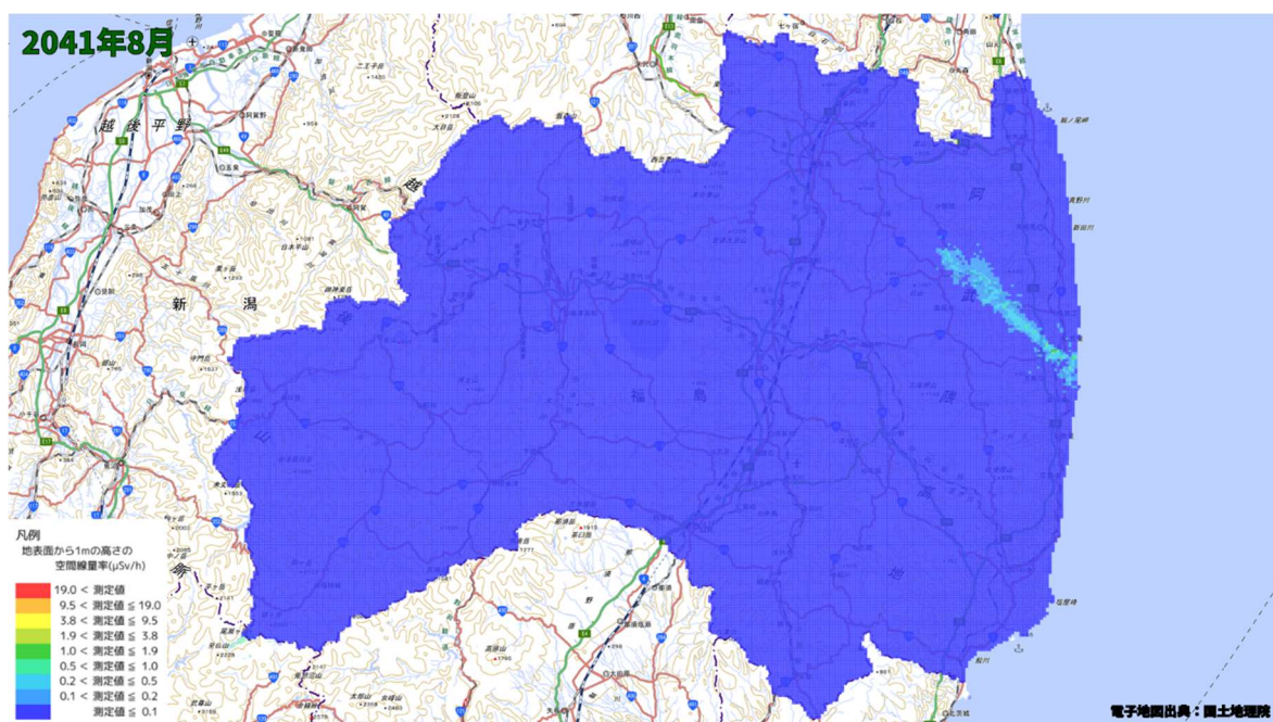
空間線量率分布将来予測解析結果(2041 年 8 月)
