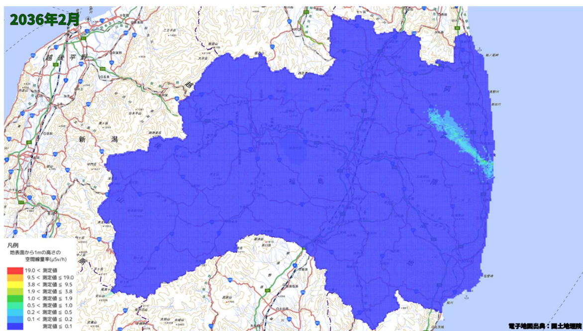
空間線量率分布将来予測解析結果(2036 年 2 月)
