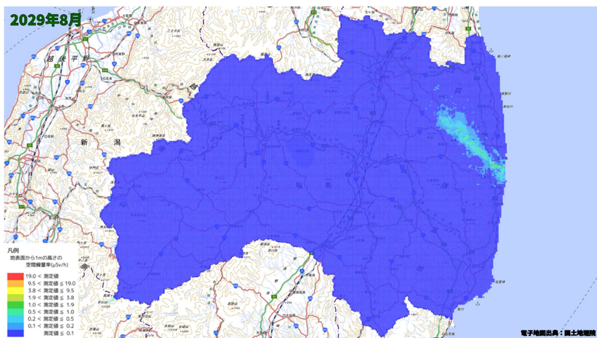
空間線量率分布将来予測解析結果(2029 年 8 月)
