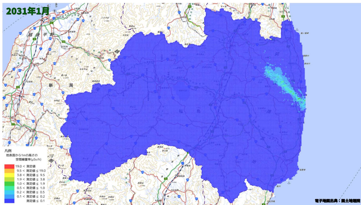
空間線量率分布将来予測解析結果(2031 年 1 月)
