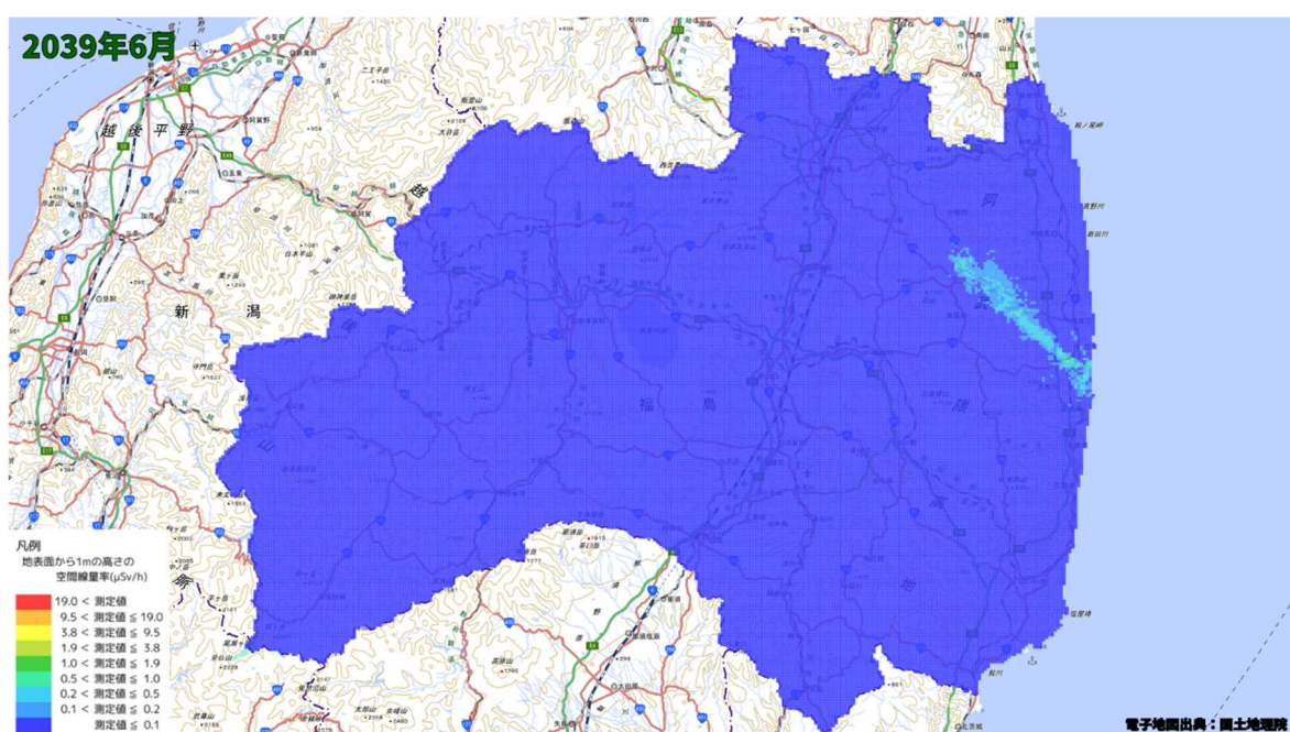
空間線量率分布将来予測解析結果(2039 年 6 月)
