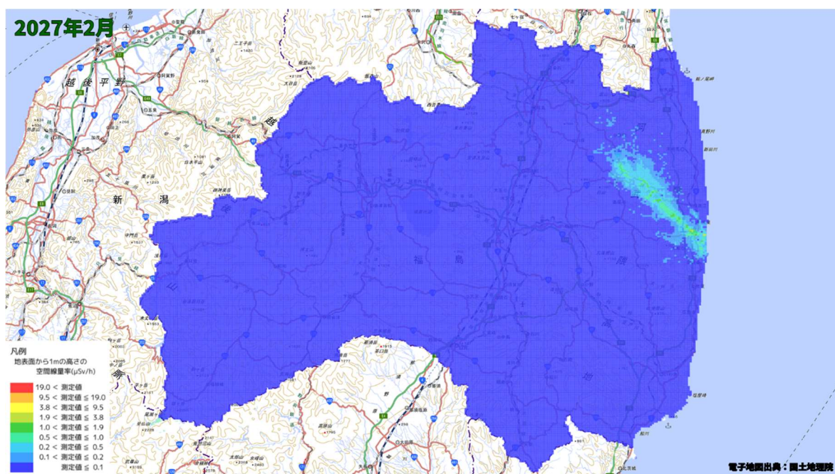
空間線量率分布将来予測解析結果(2027 年 2 月)
