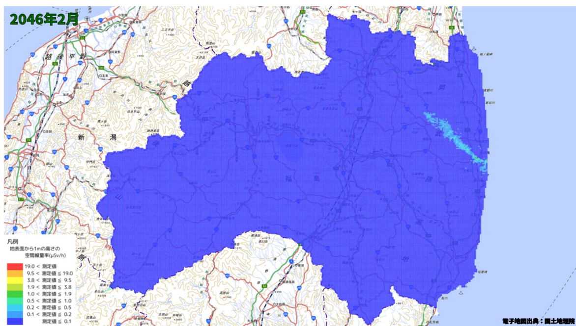
空間線量率分布将来予測解析結果(2046 年 2 月)
