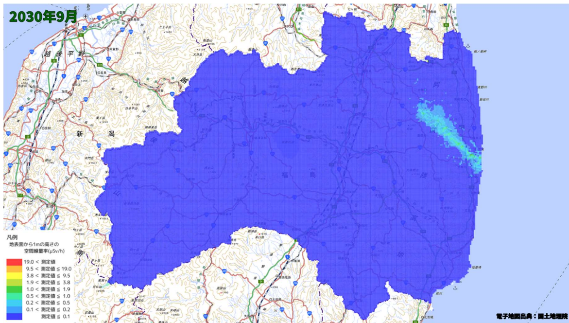
空間線量率分布将来予測解析結果(2030 年 9 月)
