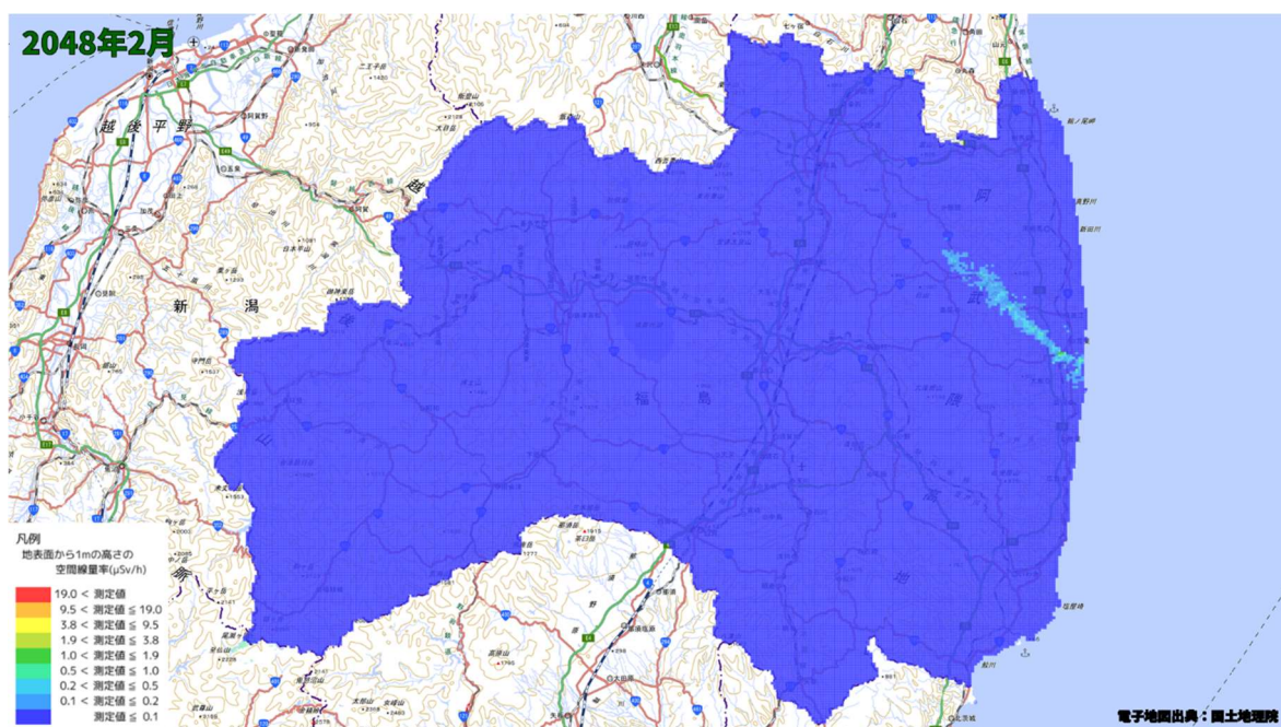
空間線量率分布将来予測解析結果(2048 年 2 月)
