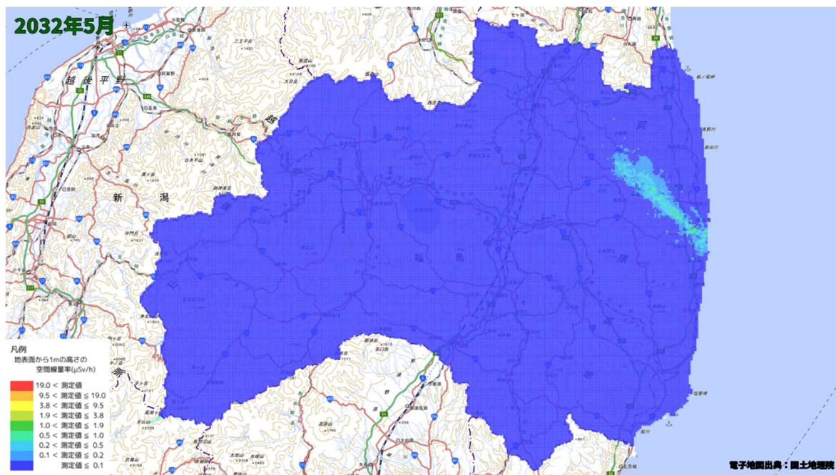
空間線量率分布将来予測解析結果(2032 年 5 月)
