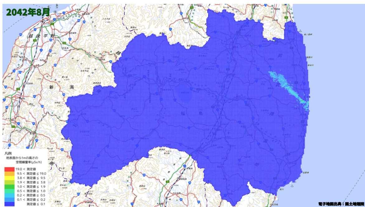
空間線量率分布将来予測解析結果(2042 年 8 月)
