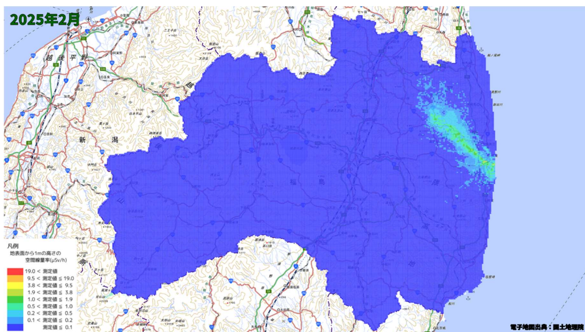
空間線量率分布将来予測解析結果(2025 年 2 月)
