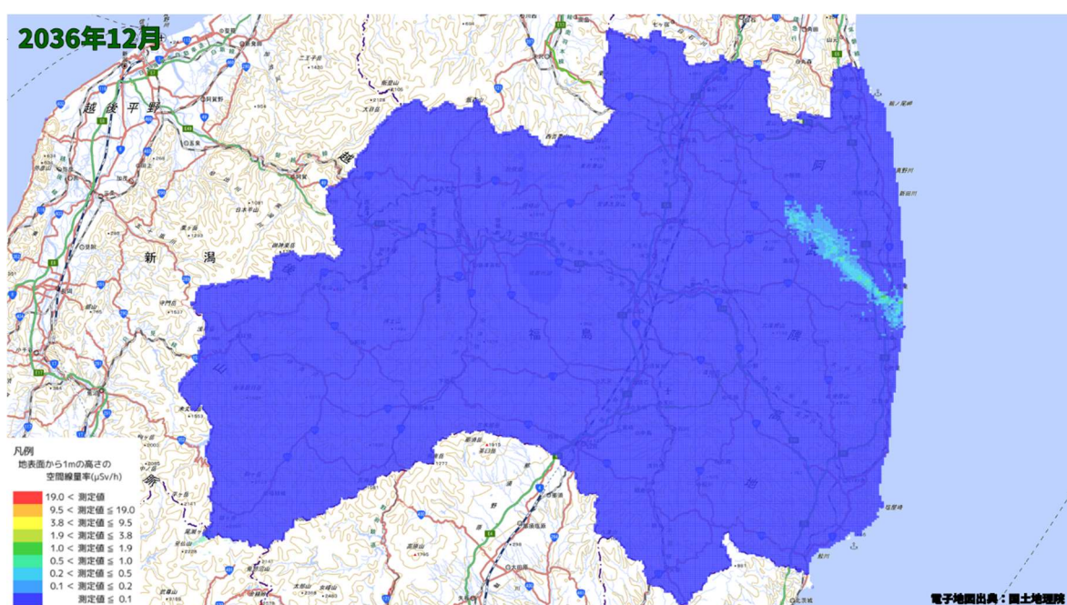
空間線量率分布将来予測解析結果(2036 年 12 月)
