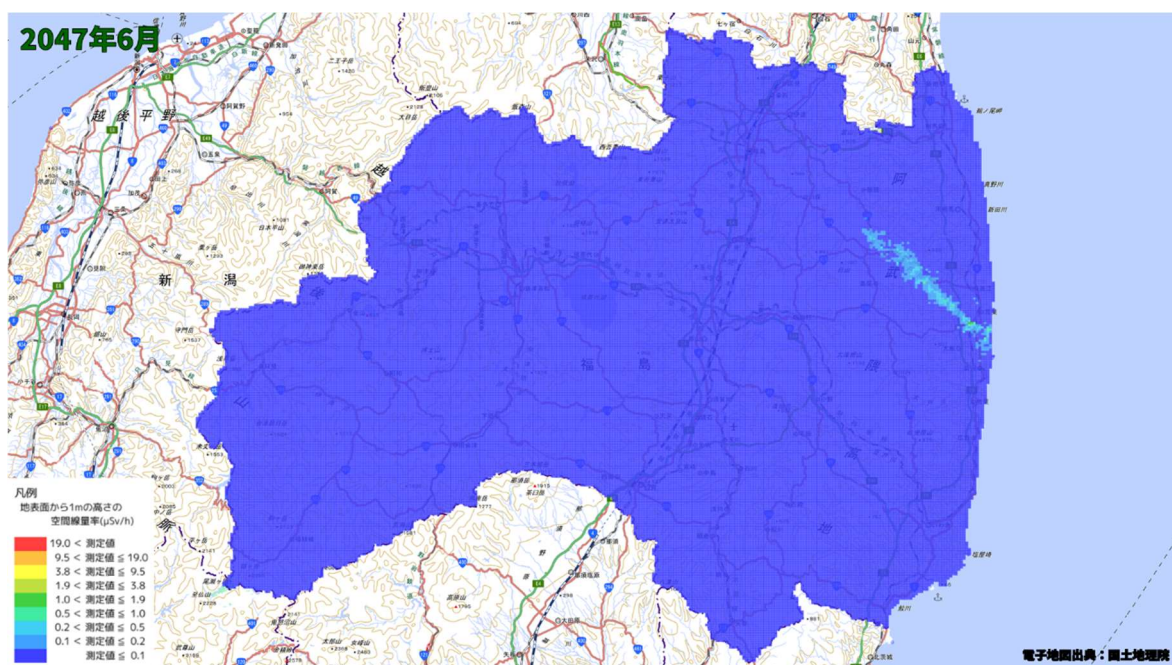
空間線量率分布将来予測解析結果(2047 年 6 月)
