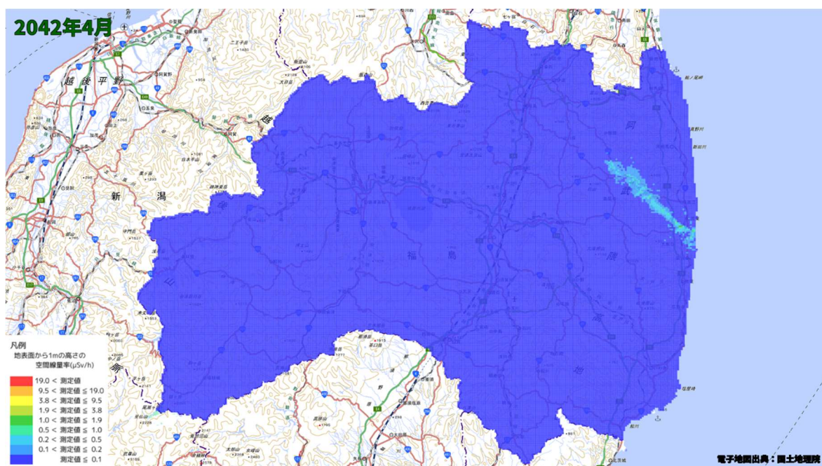
空間線量率分布将来予測解析結果(2042 年 4 月)
