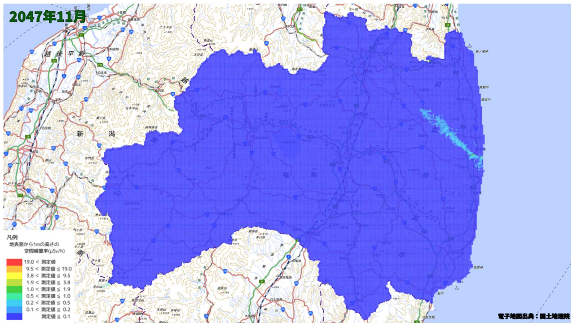
空間線量率分布将来予測解析結果(2047 年 11 月)
