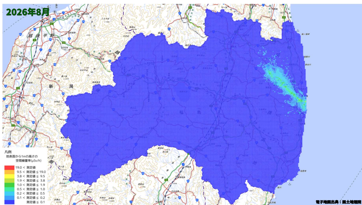
空間線量率分布将来予測解析結果(2026 年 8 月)
