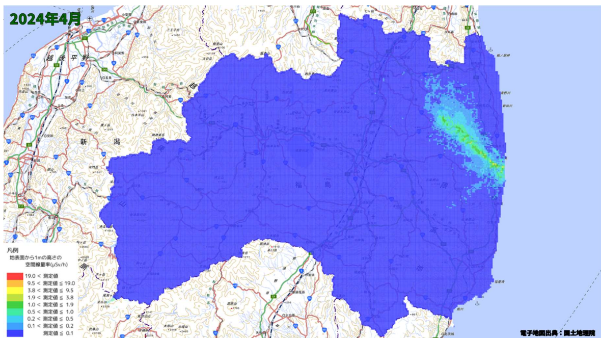
空間線量率分布将来予測解析結果(2024 年 4 月)
