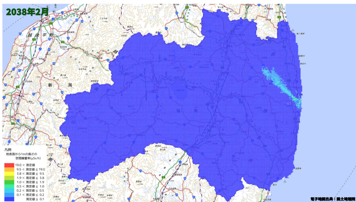
空間線量率分布将来予測解析結果(2038 年 2 月)
