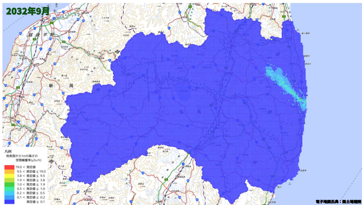
空間線量率分布将来予測解析結果(2032 年 9 月)
