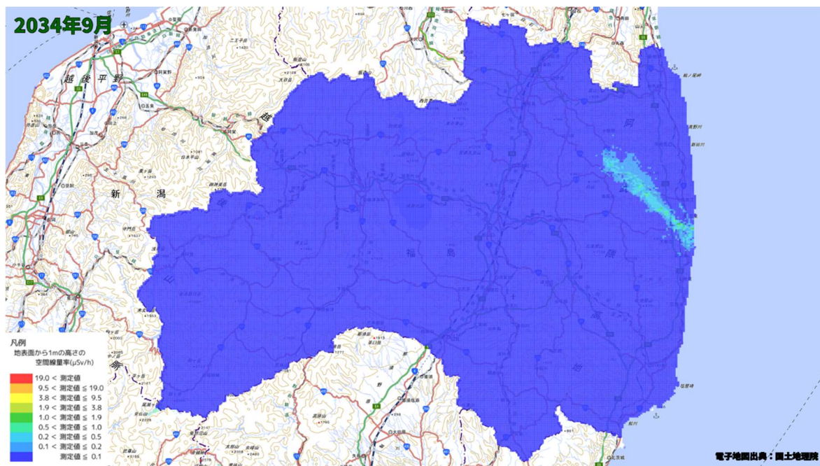
空間線量率分布将来予測解析結果(2034 年 9 月)
