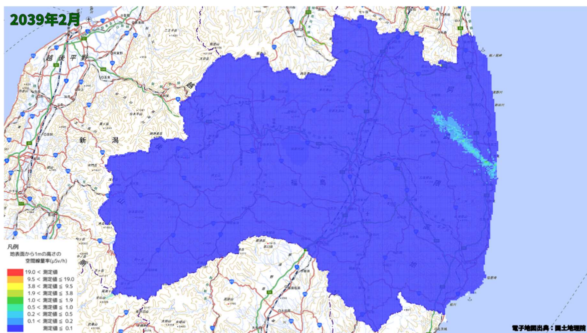
空間線量率分布将来予測解析結果(2039 年 2 月)
