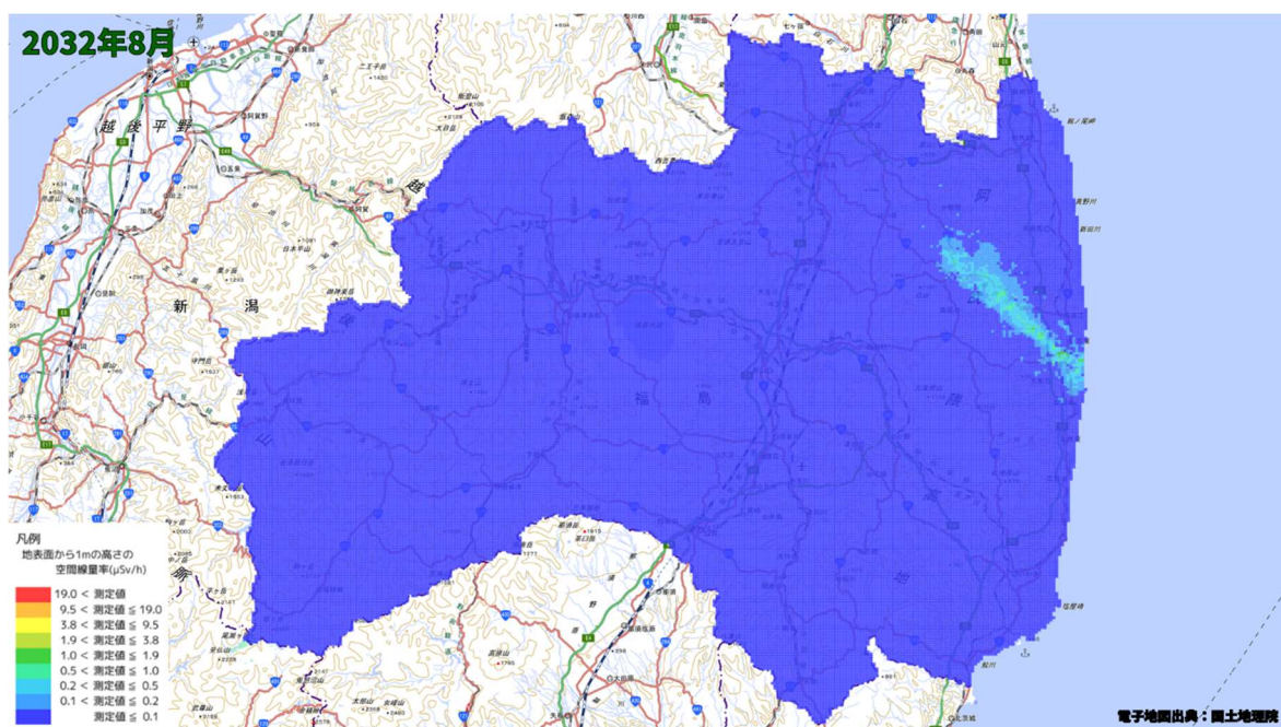
空間線量率分布将来予測解析結果(2032 年 8 月)
