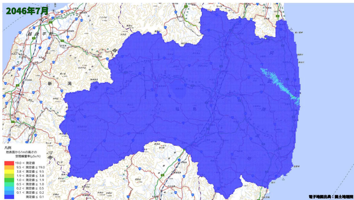
空間線量率分布将来予測解析結果(2046 年 7 月)
