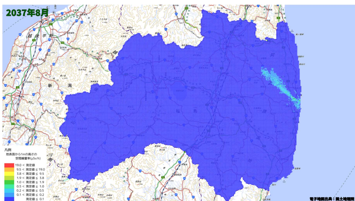
空間線量率分布将来予測解析結果(2037 年 8 月)
