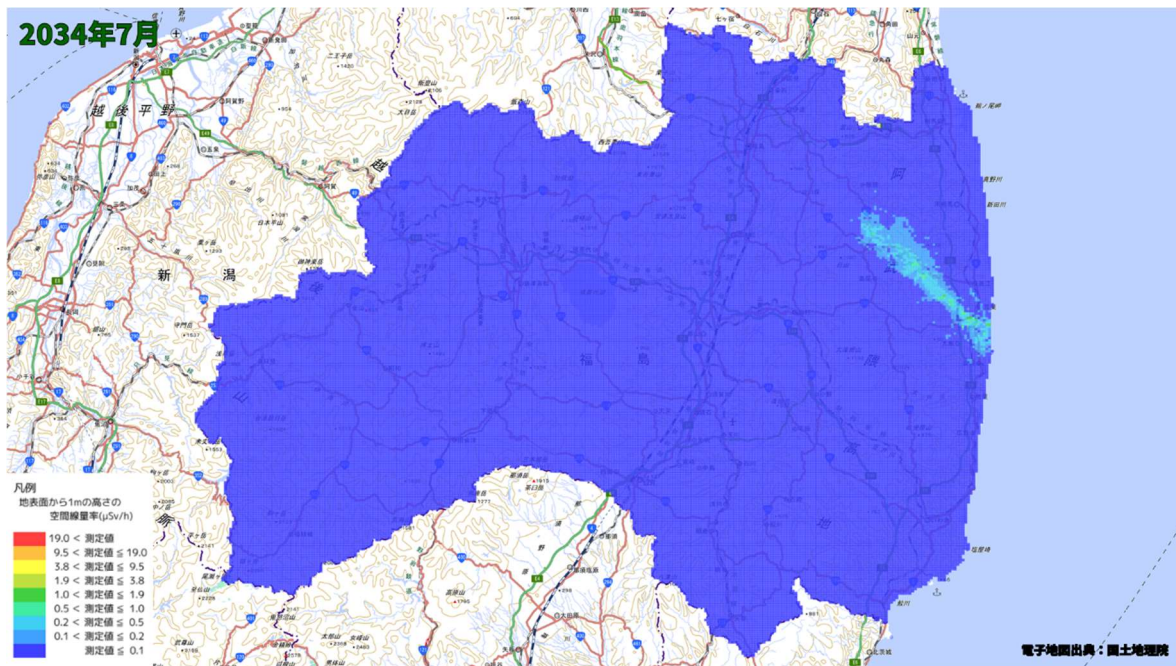
空間線量率分布将来予測解析結果(2034 年 7 月)
