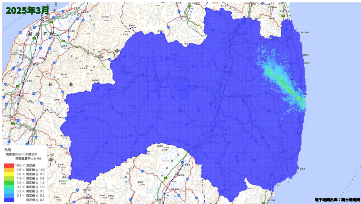
空間線量率分布将来予測解析結果(2025 年 3 月)
