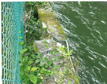
コンクリートの割れ(開水路)
