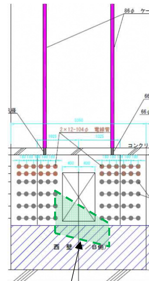
b-b断面
