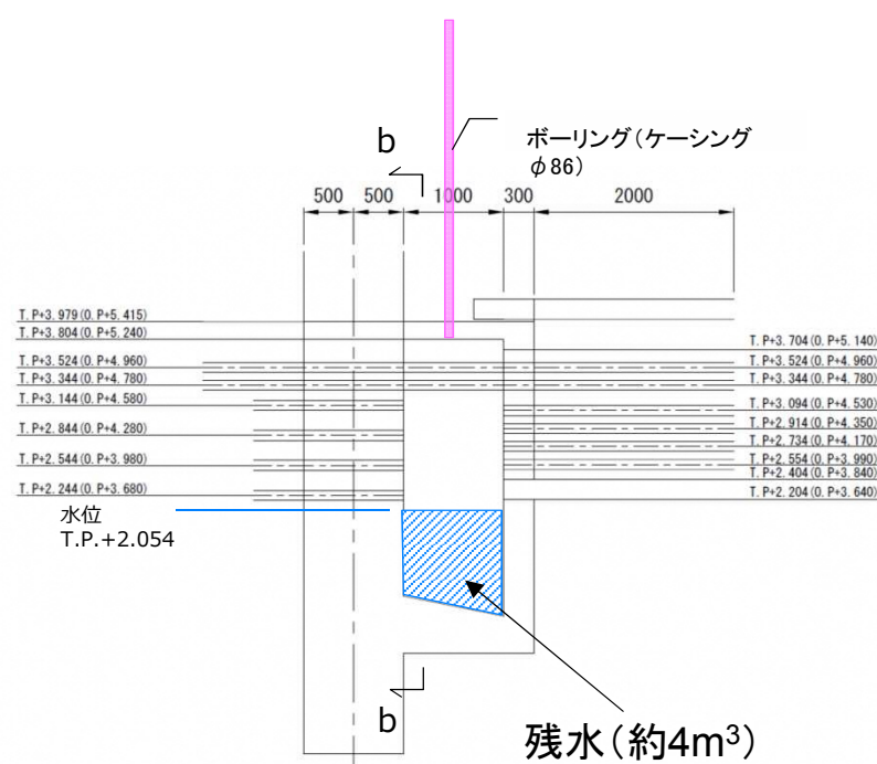
b-b断面
