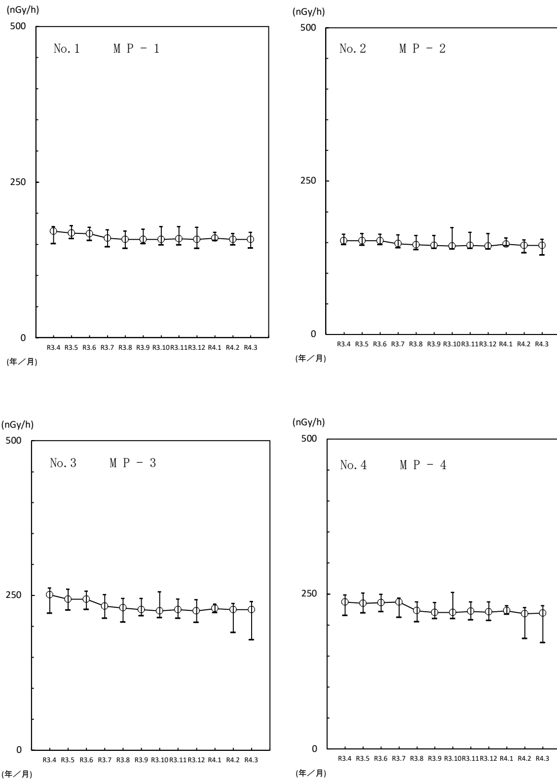
図 4. 7 空間線量率の月間平均値及び変動幅の推移
