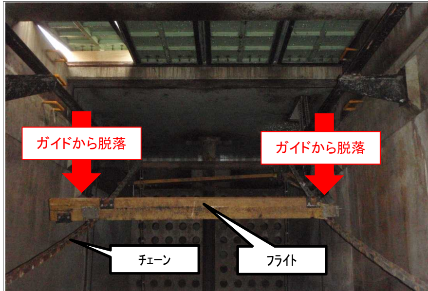
写真3-1 県北浄化センター(伊達郡国見町)汚泥掻寄機損傷
