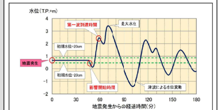
図2 影響開始時間と第一波到達時間
