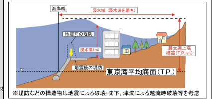
図1 最大遡上高と浸水深
