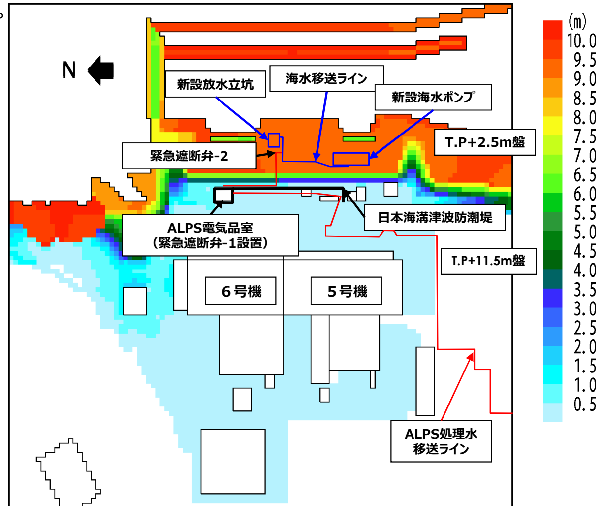
日本海溝津波による最大浸水分布図 (第93回 特定原子力施設監視・評価検討会と同条件での解析結果)
