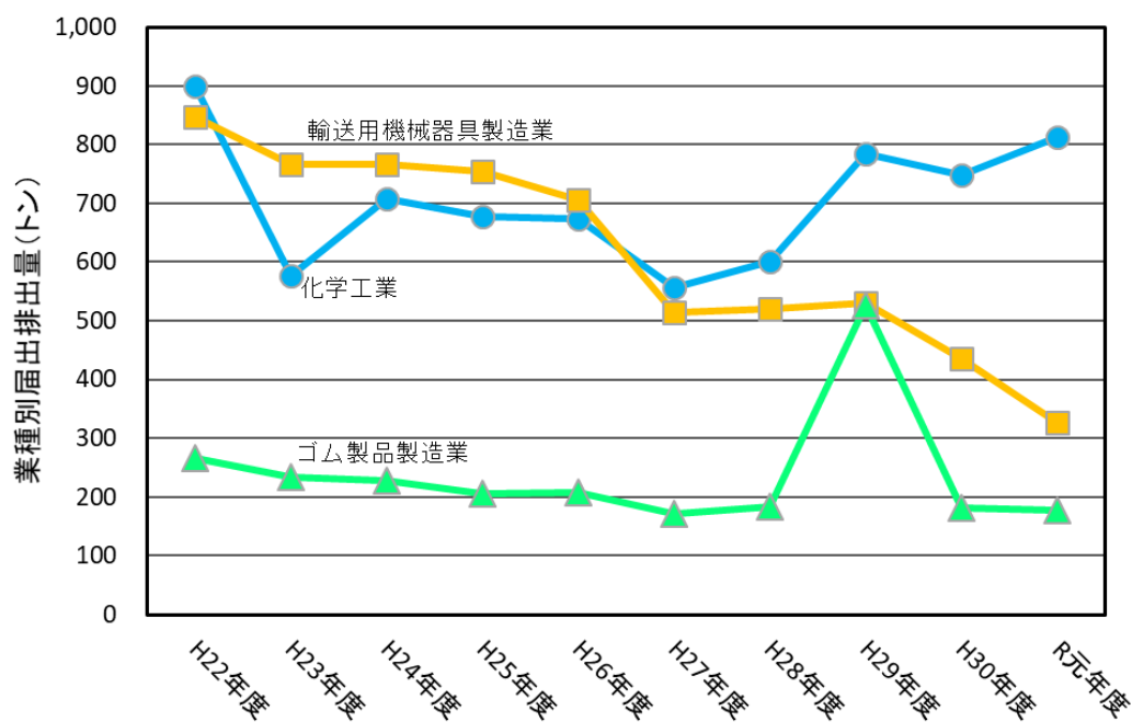
図-2 業種別届出排出量の上位3業種の経年推移
