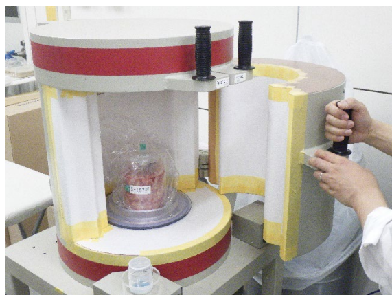
モニタリング検査を行っている機器 (ゲルマニウム半導体検出器)
