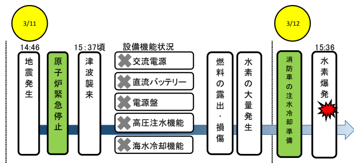
1号機の事故経過
