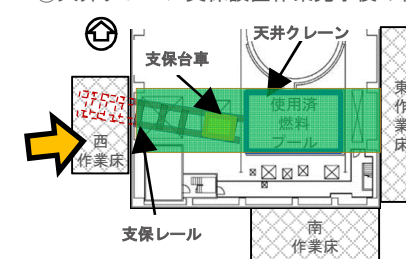
④天井クレーン支保設置作業完了後の状況
