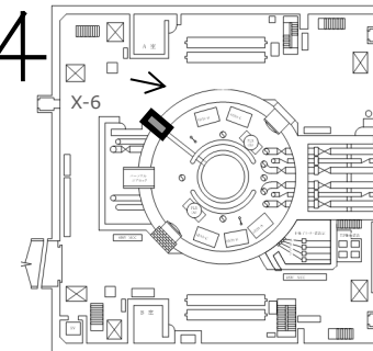
2号機原子炉建屋1階 ペネ配置図
