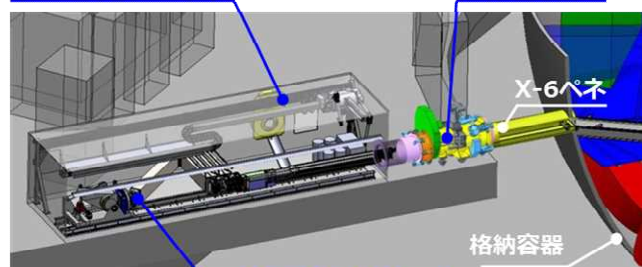
①ロボットアーム
