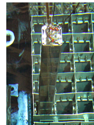
燃料ラックへの装填
