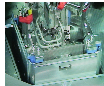
輸送容器からの吊り上げ
