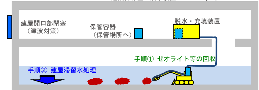
ゼオライト土嚢等の対応方針の概念図
