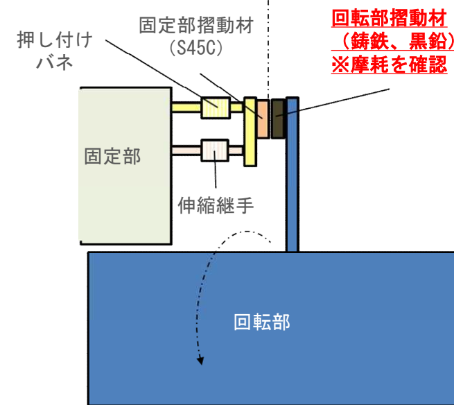
ロータリーキルン シール部（入口側）模式図 （※出口側も同様な構造）
