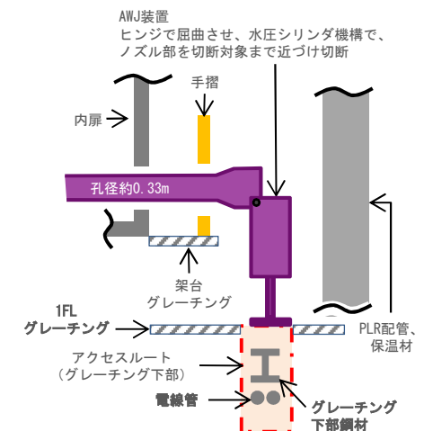
グレーチング切断作業イメージ
