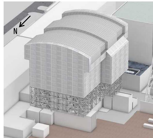
大型カバーの設置イメージ
