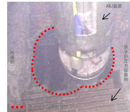
グレーチング切断後写真
