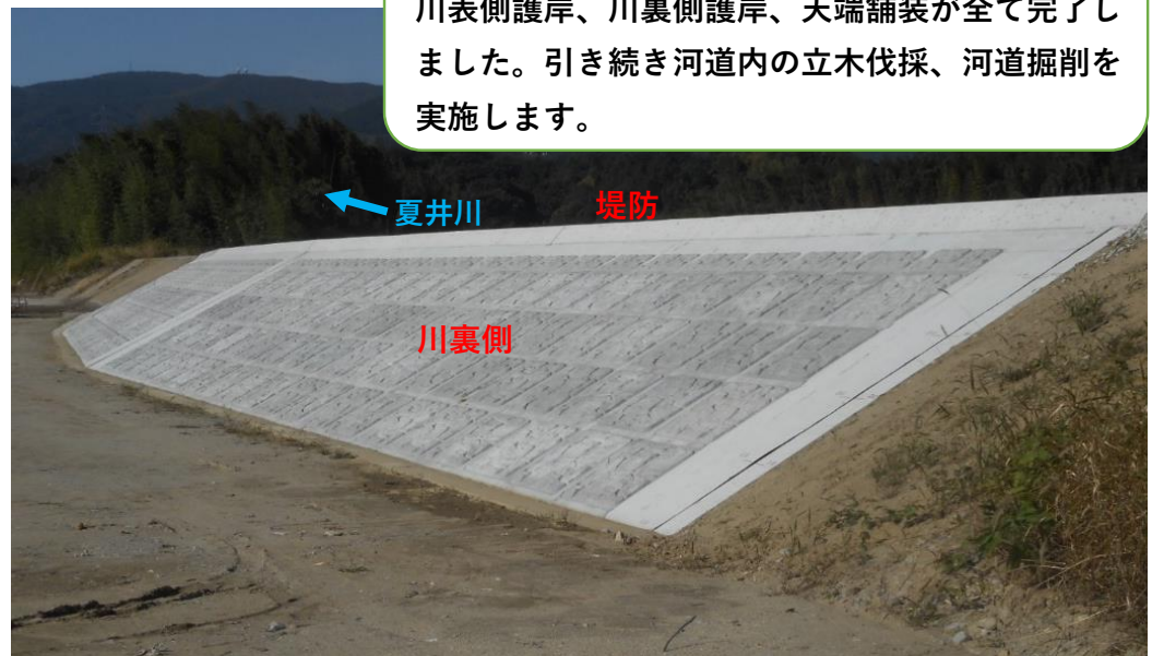
川裏側 コンクリート張ブロック完了 (8月末)
