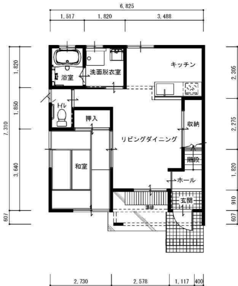
1階平面図
