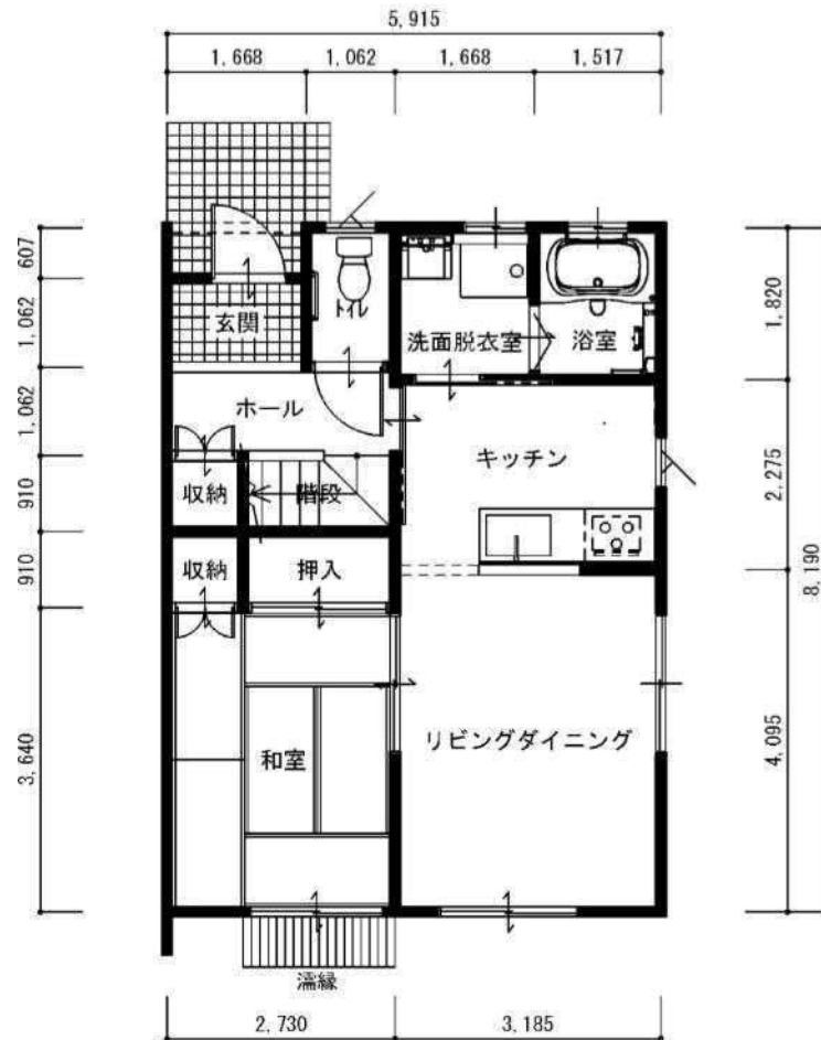
1階 平面図
