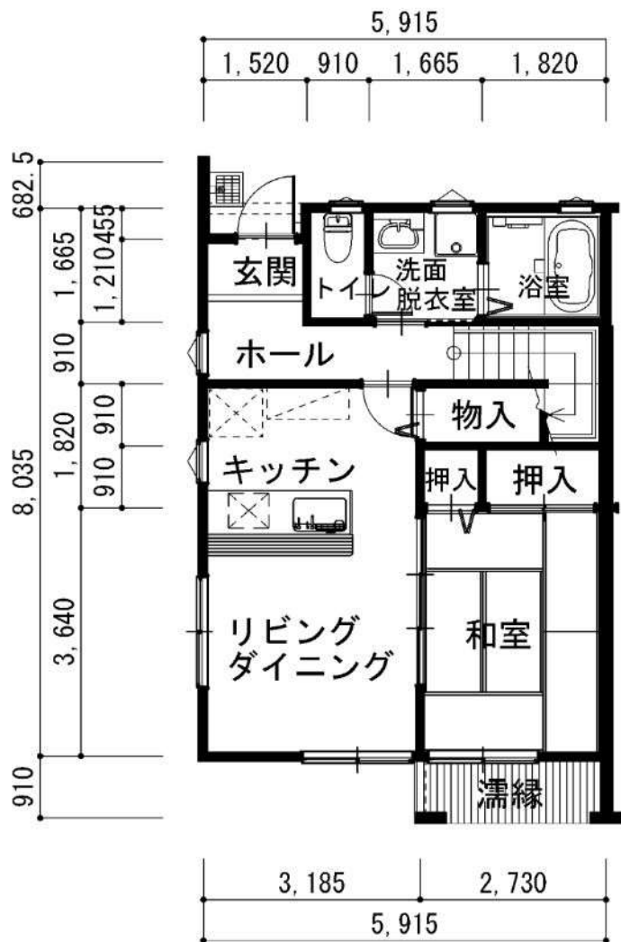
1階平面図
