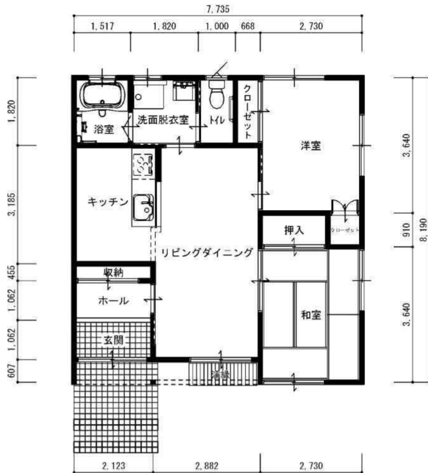
1階平面図
