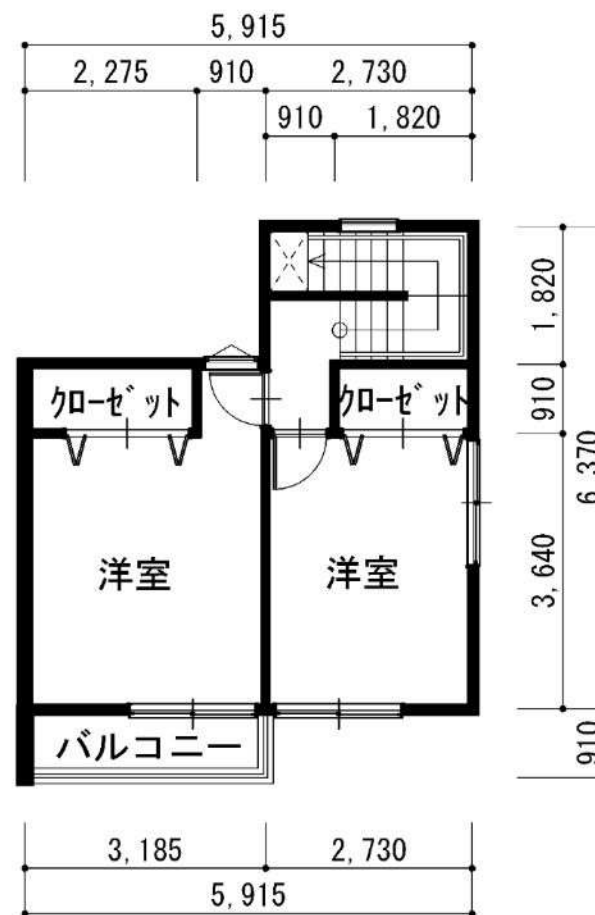
2階平面図
