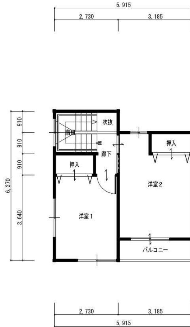
2階平面図 S:1/100
