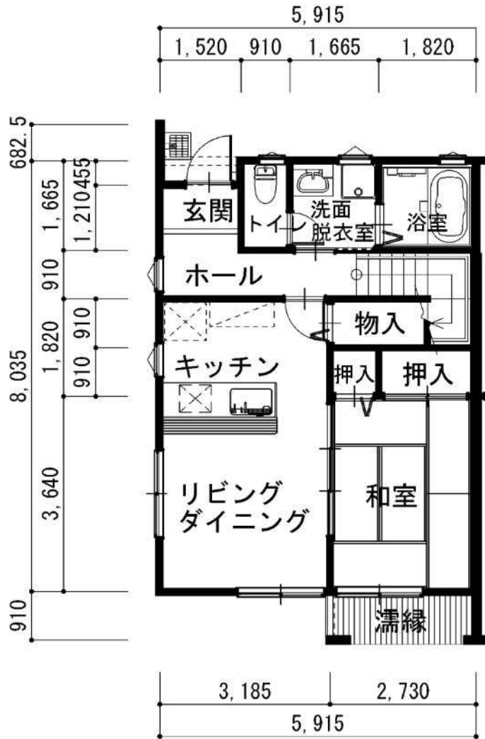
1階平面図
