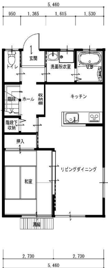
1階平面図 S:1/100
