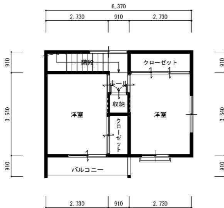
2階平面図
