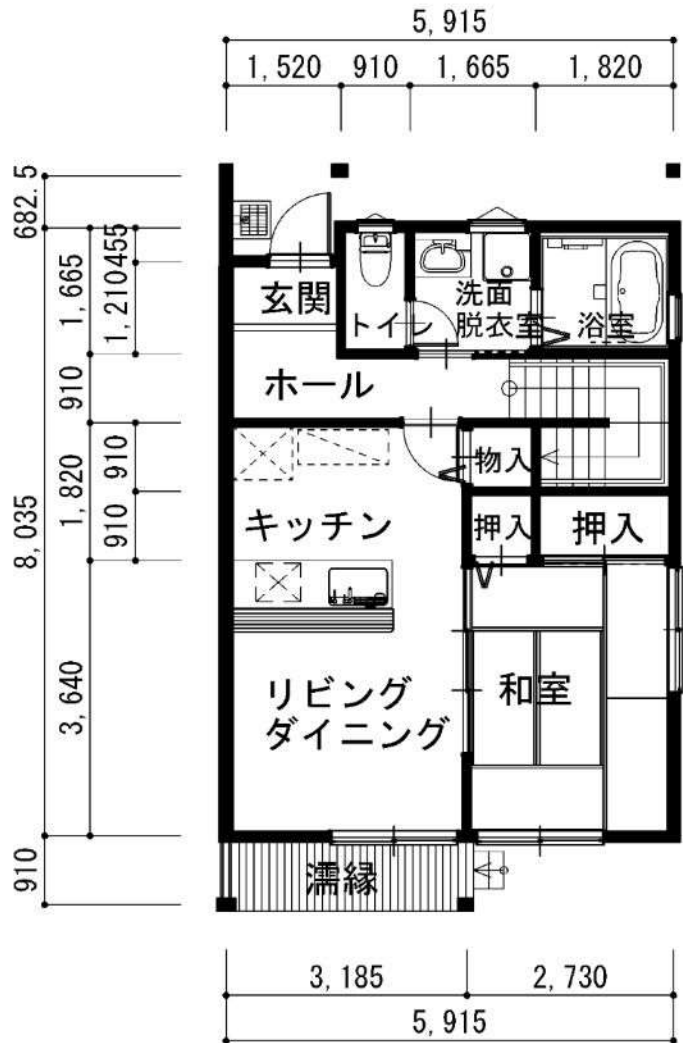
1階平面図
