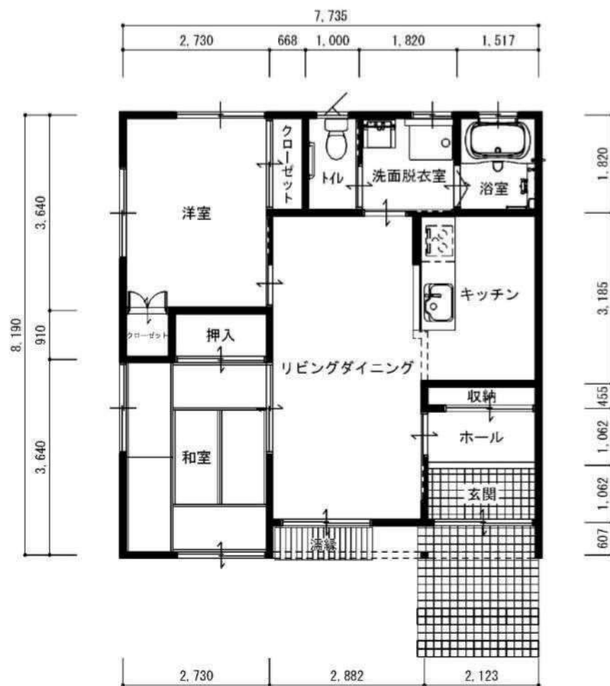
1階平面図
