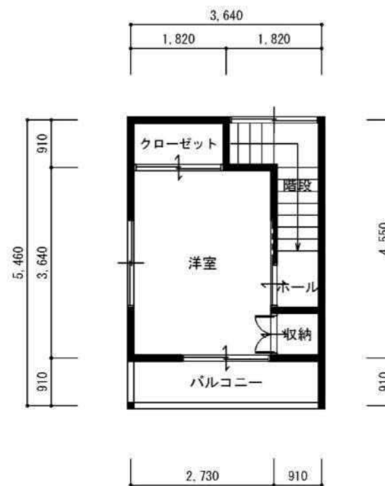
2階 平面図
