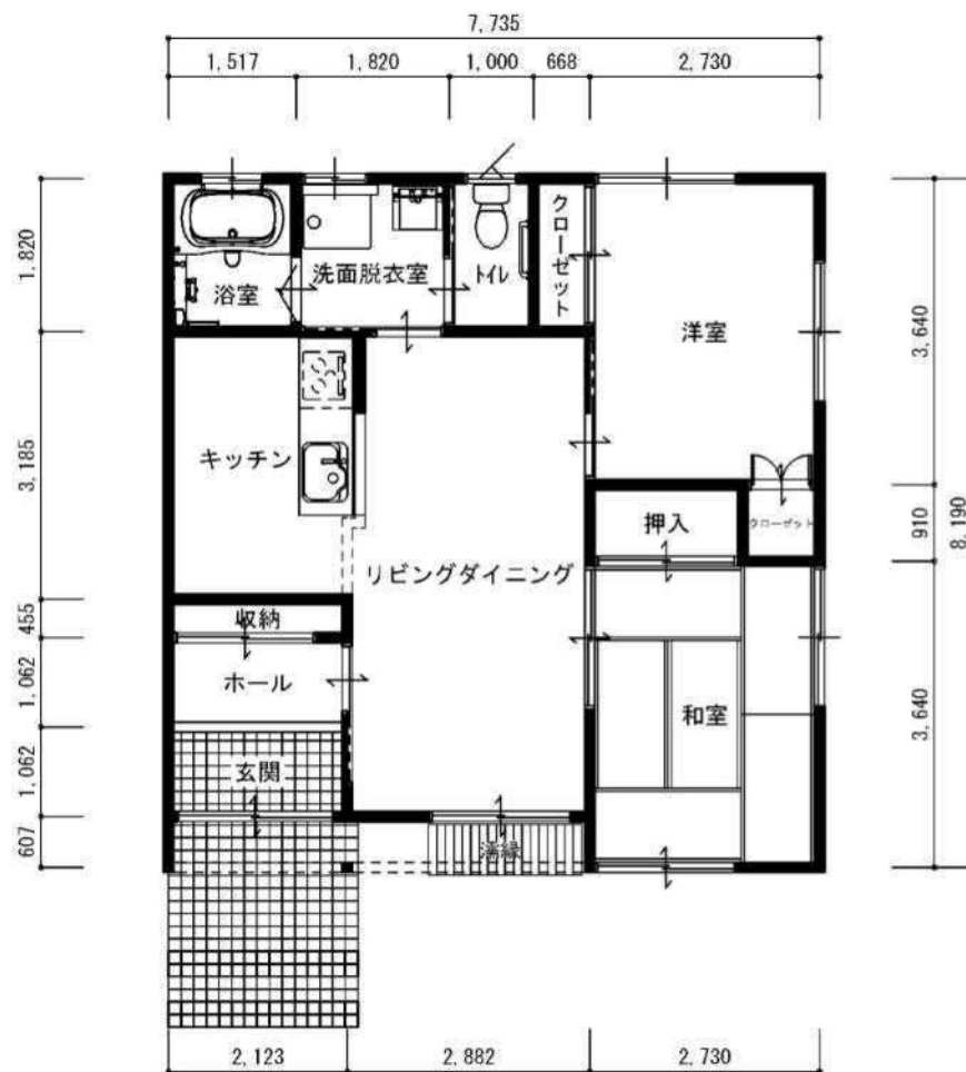
1階平面図
