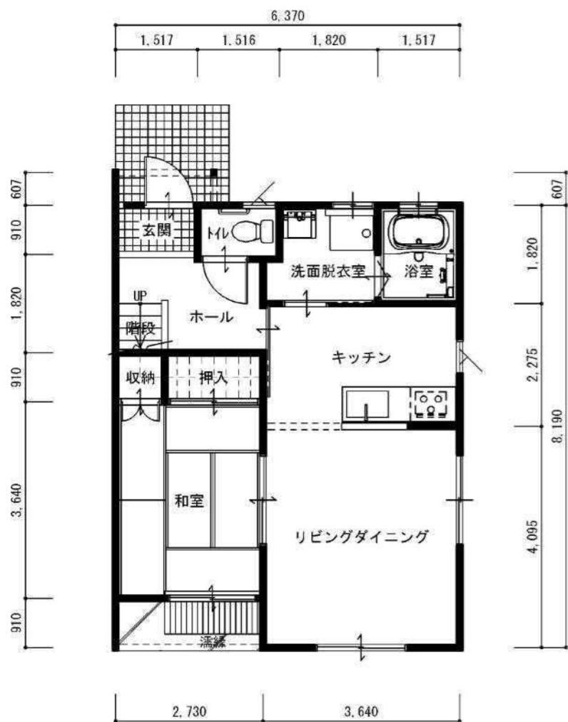
1階平面図
