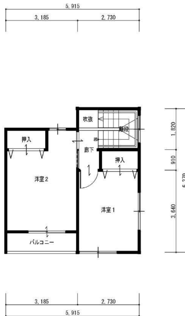
2階平面図 S:1/100
