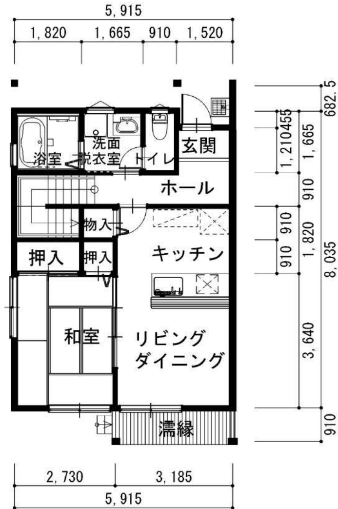
1階平面図
