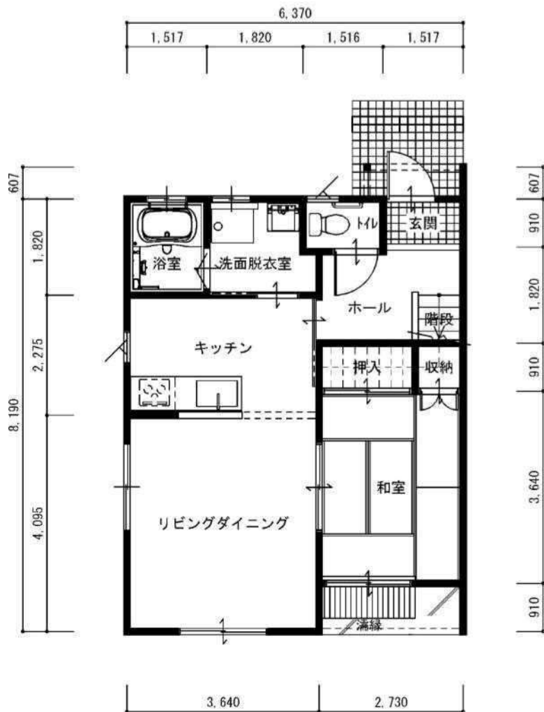
1階平面図
