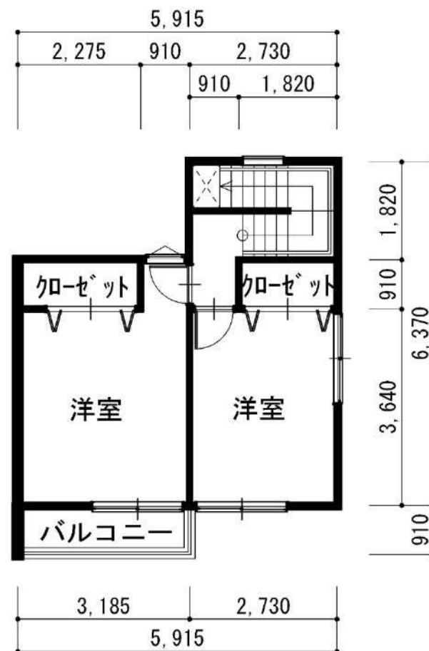
2階平面図
