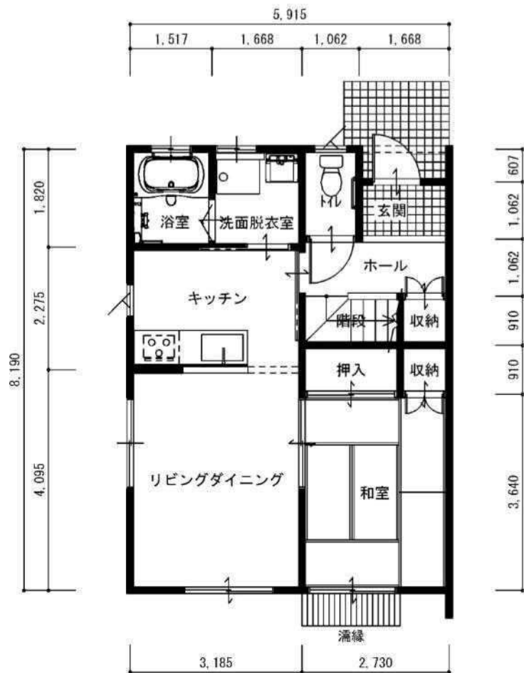
1階 平面図
