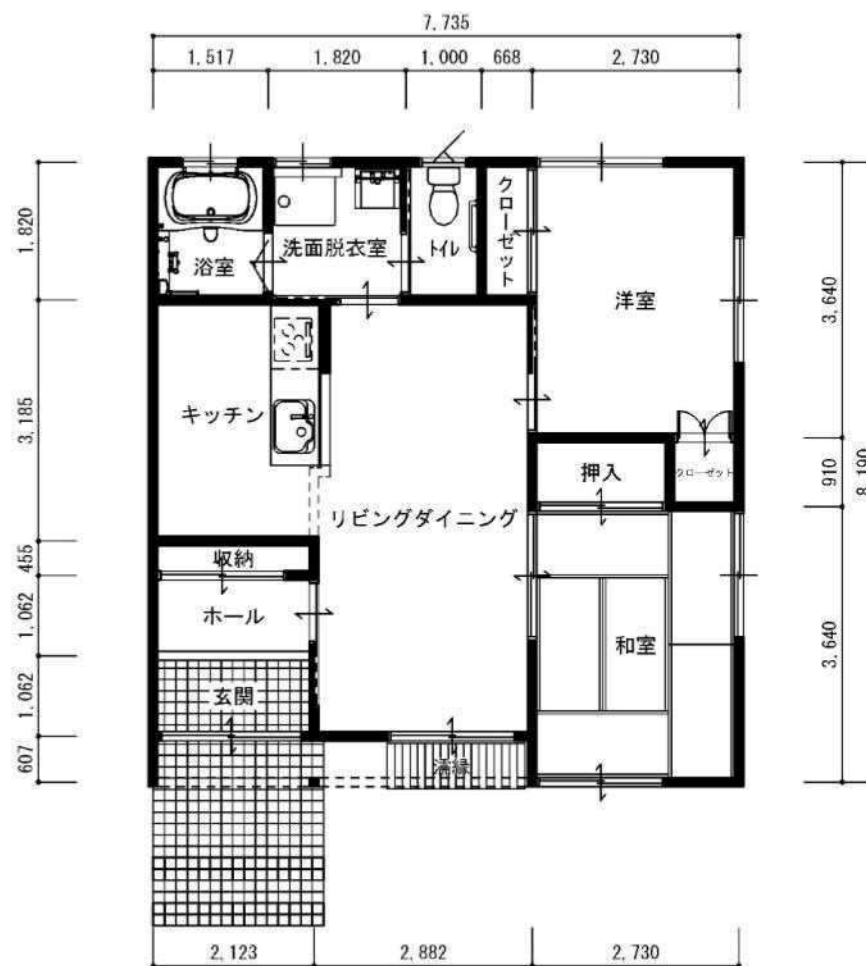
1階平面図
