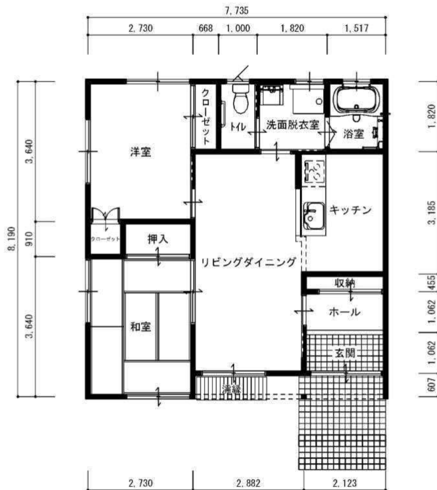
1階平面図
