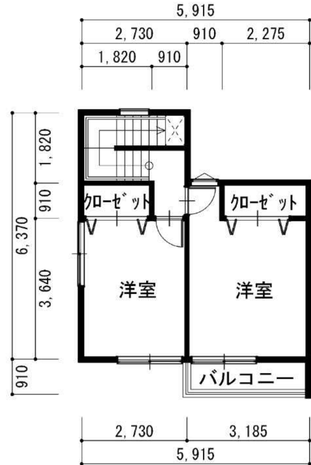
2階平面図
