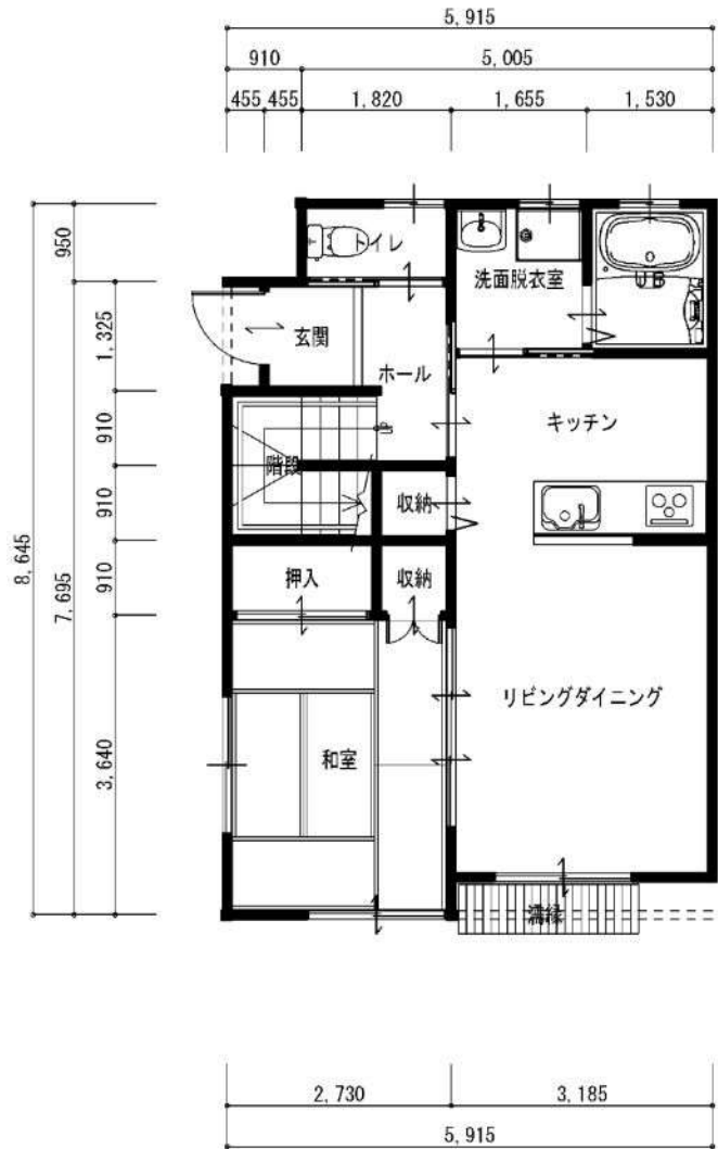
1階平面図 S:1/100
