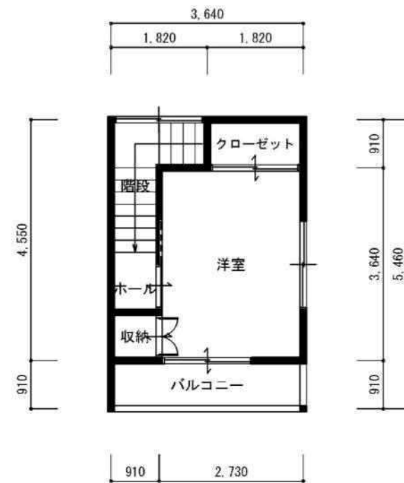
2階 平面図
