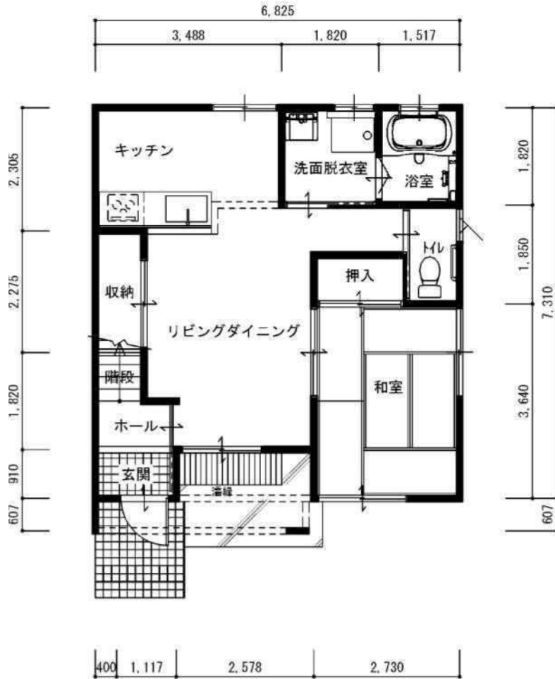
1階平面図
