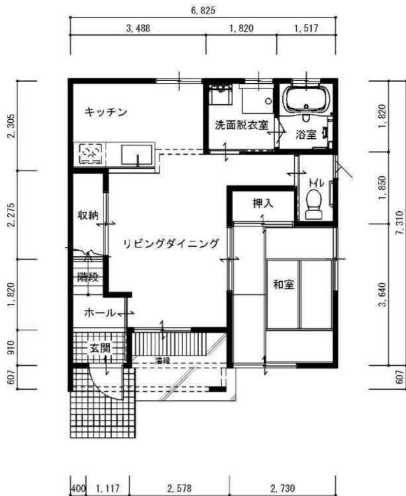
1階平面図
