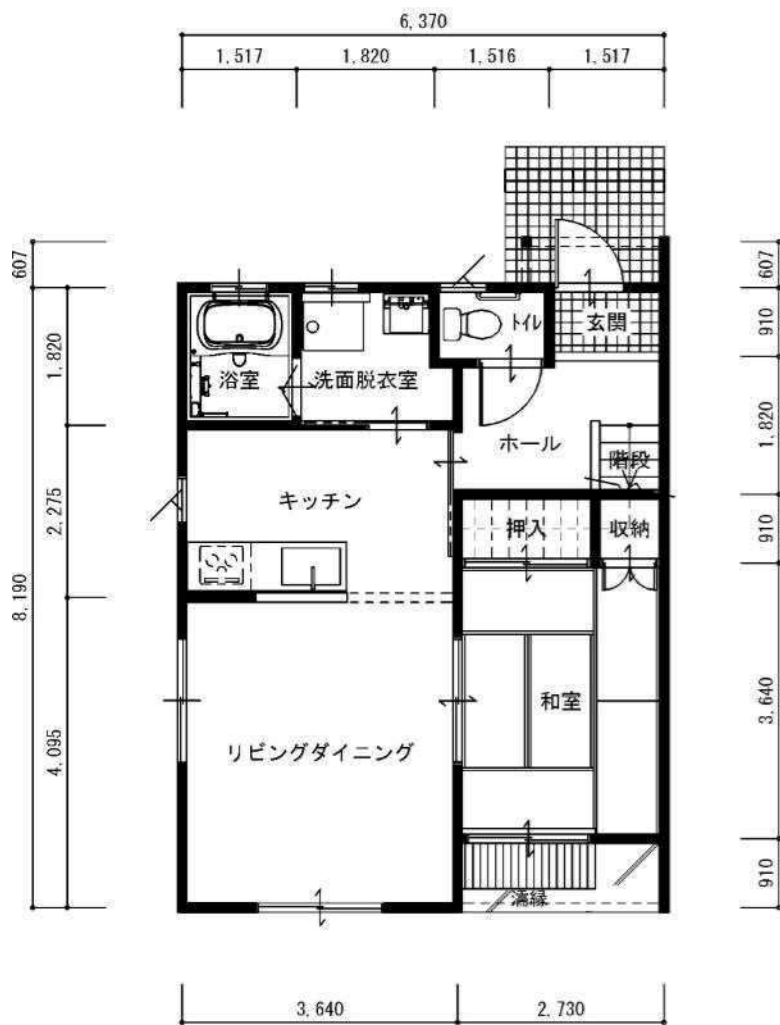
1階平面図
