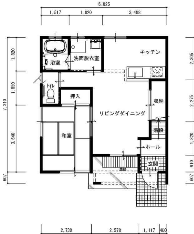
1階平面図
