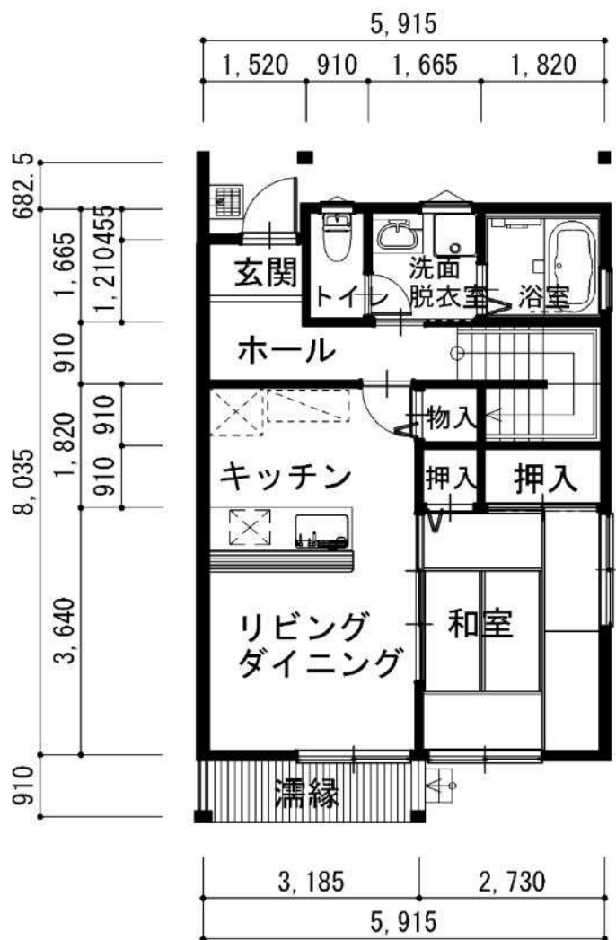
1階平面図
