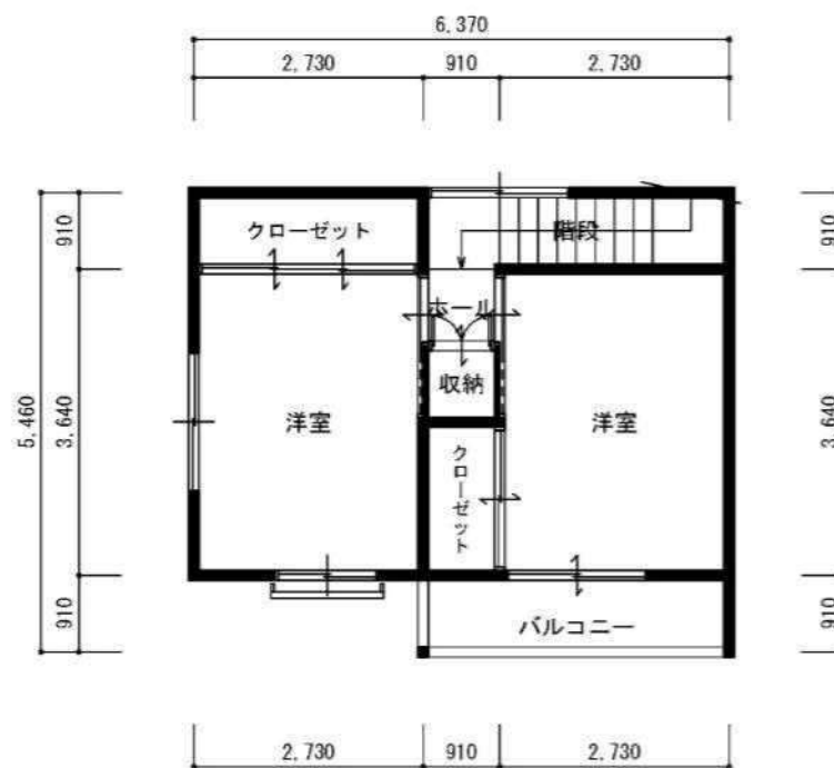
2階平面図
