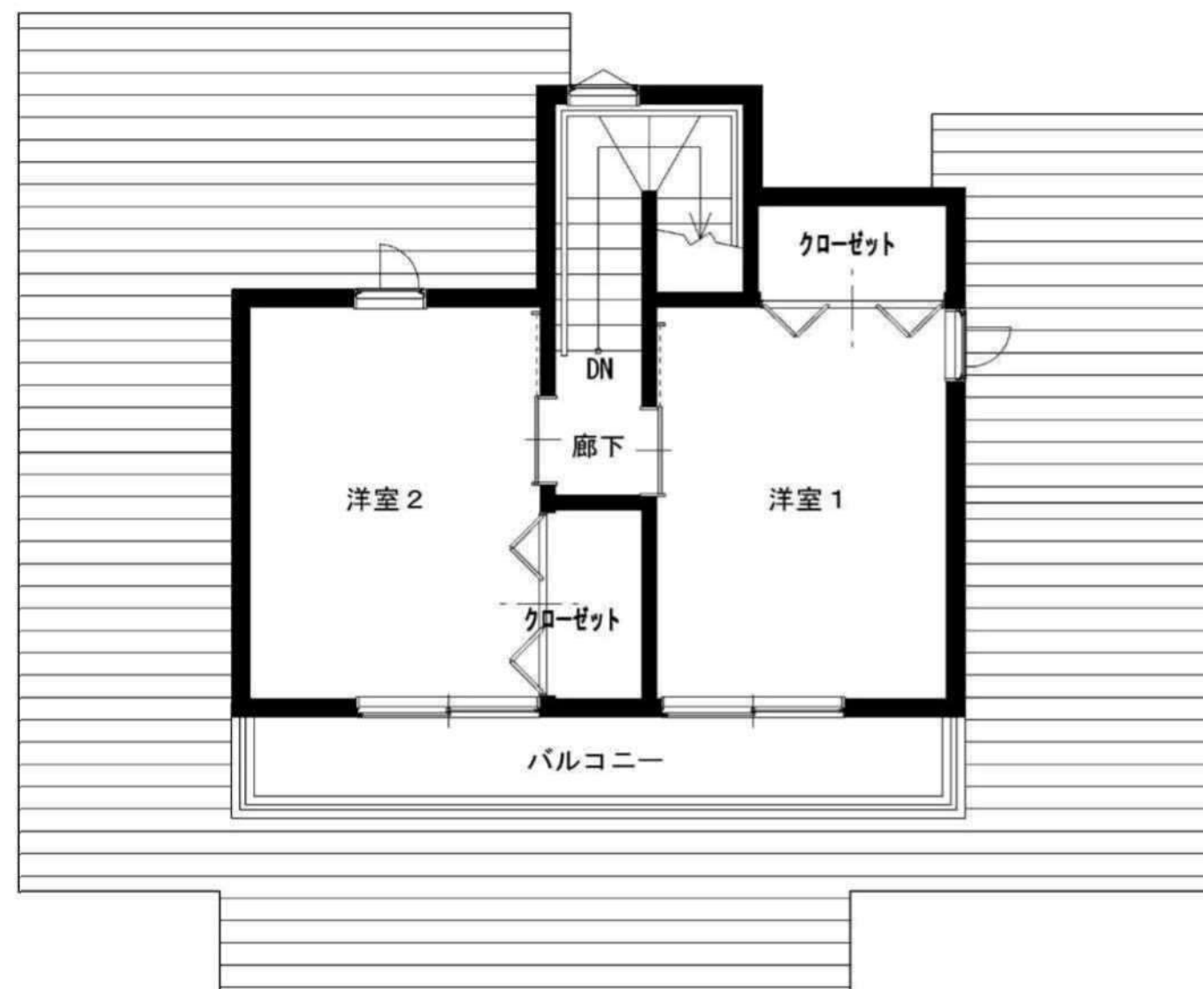
2階平面図
