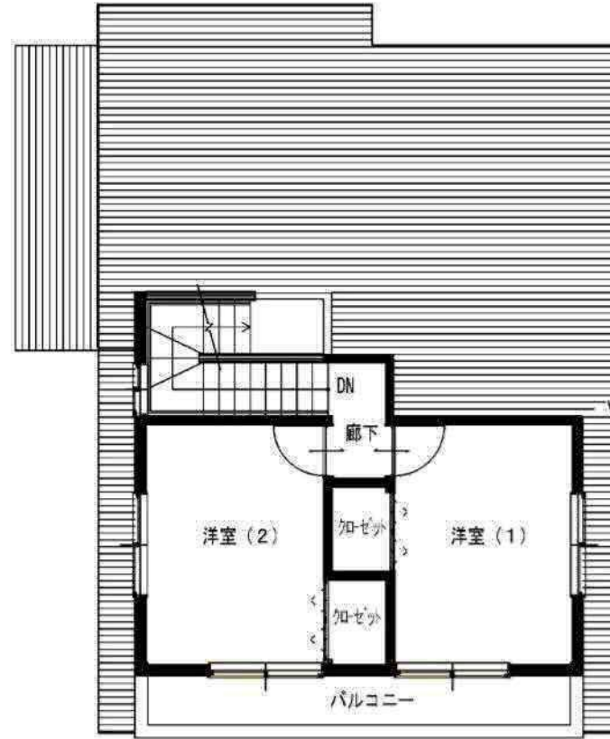
2階平面図
