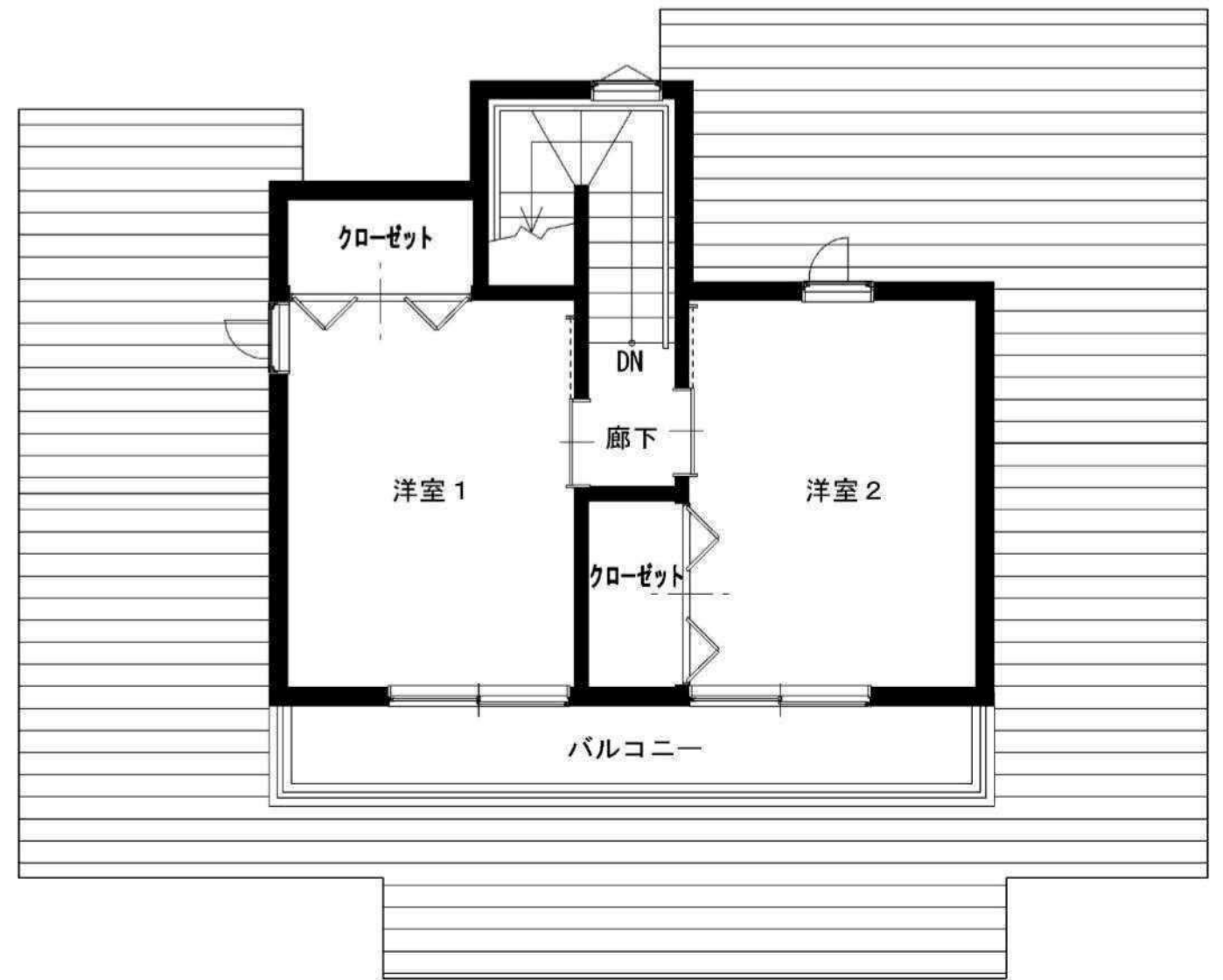
2階平面図
