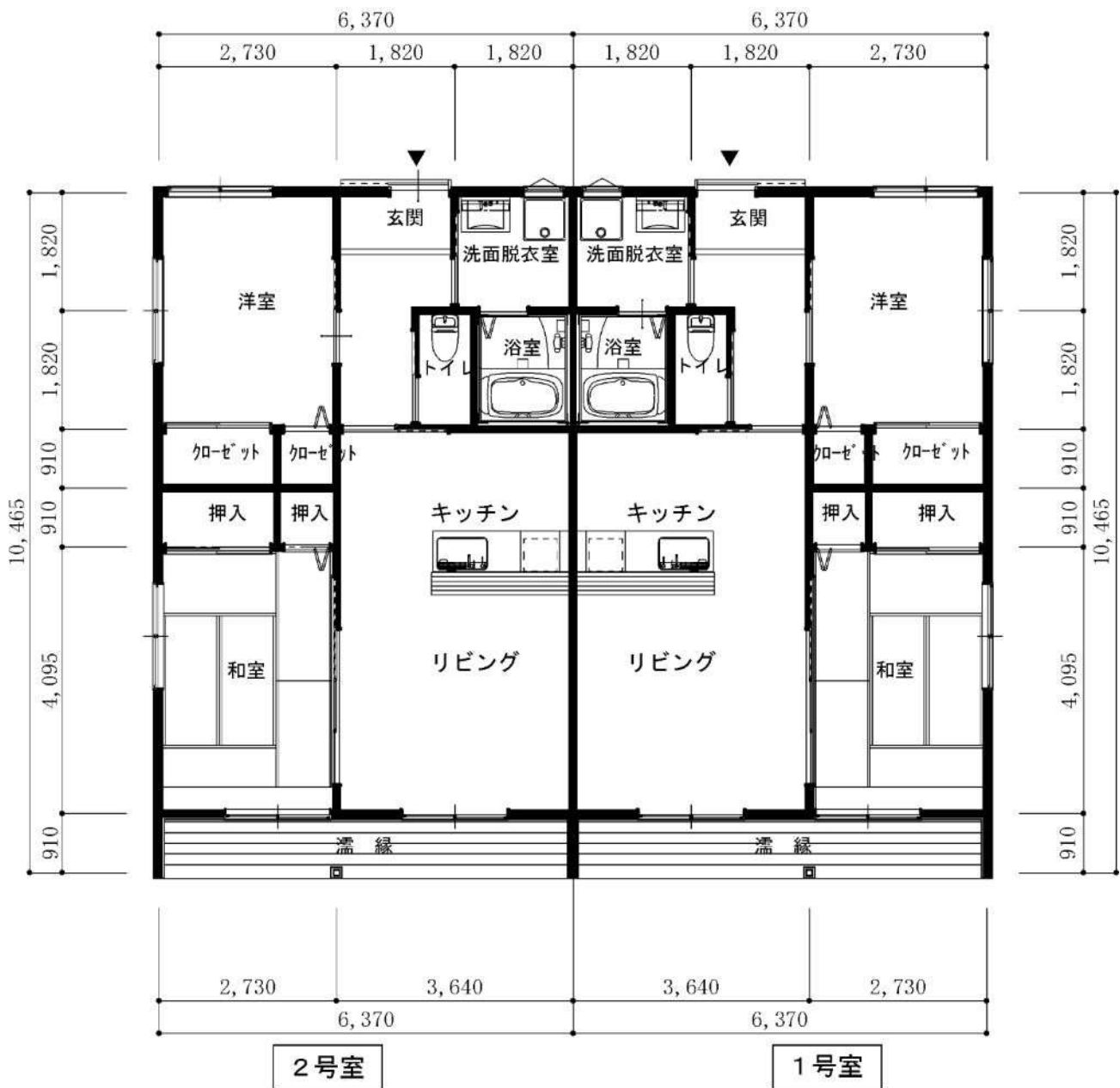
1階平面図
