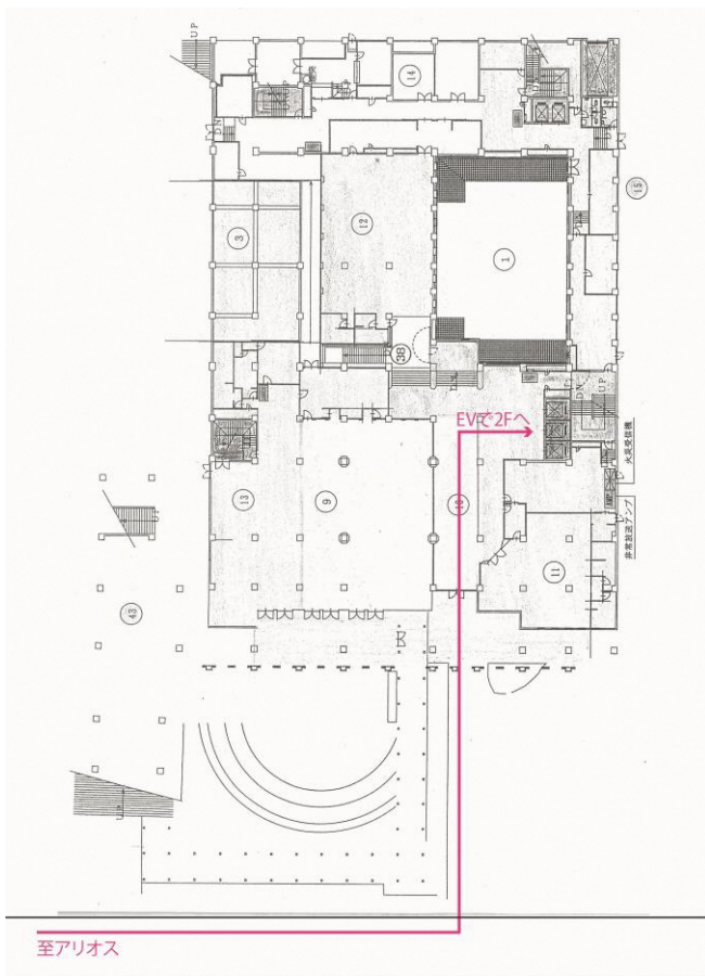
1F 平面図
