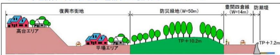
津波への多重防御や高台住宅地の整備などの復興まちづくりのイメージ
