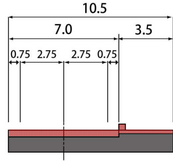
③-③'横断面図(変更案) (W=10.5m)
