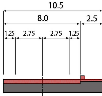
②-②'横断面図(変更案) (W=10.5m)
