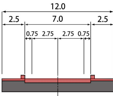
①-①'横断面図 (W=12m)
