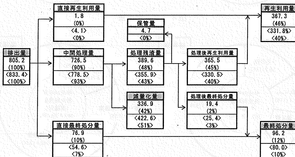
図4-1 産業廃棄物の処理フロー
