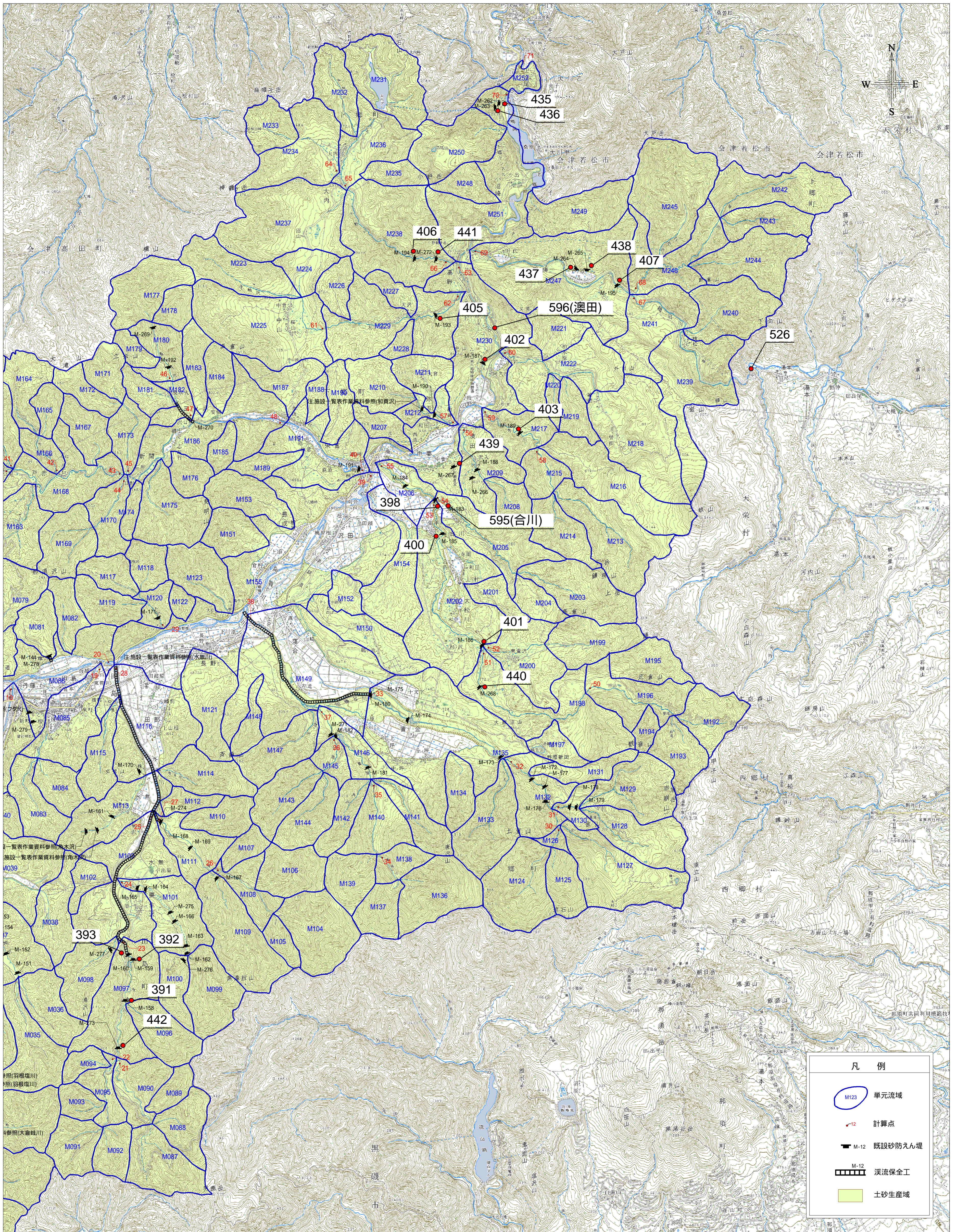
福島県南会津建設事務所 流域分割及び施設位置図-4/7
