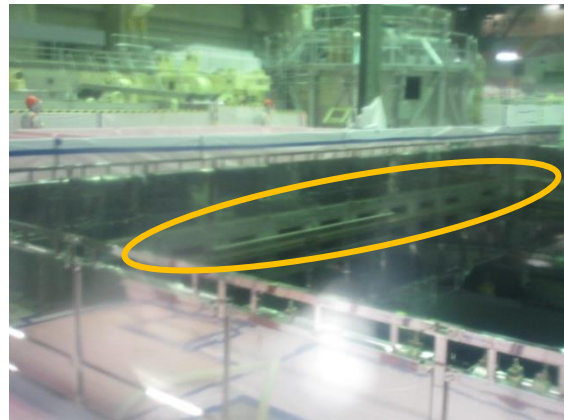
水面の揺れにより水が流入したダクト
