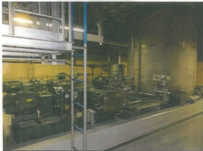
1号機ほう酸水注入系(SLC)のタンクとポンプ
