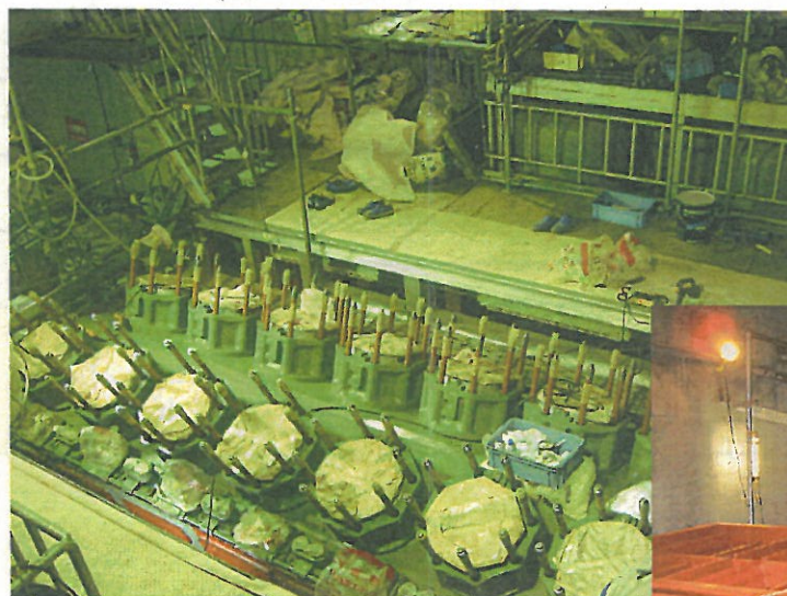
非常用ディーゼル発電設備
