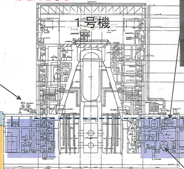
1号機非常用D/G
