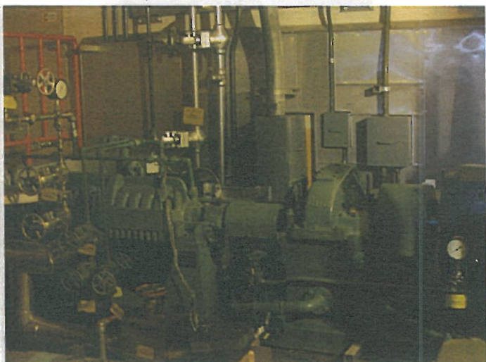
1号機制御棒駆動機構(CRD)ポンプ
